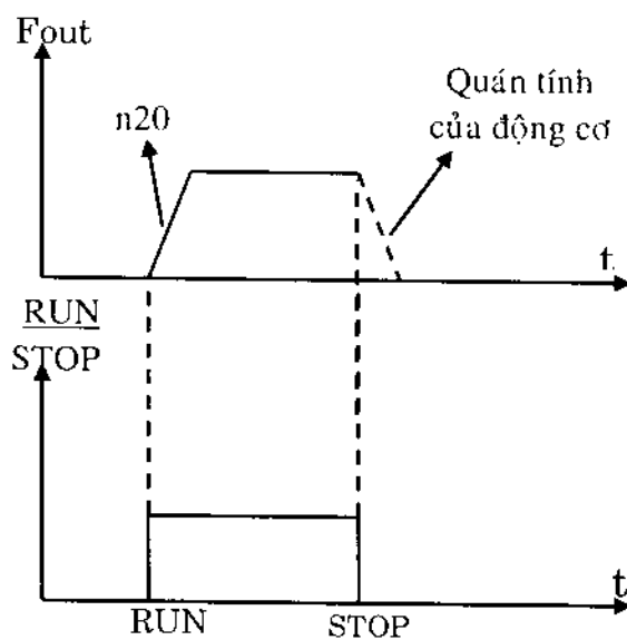
Hình 6.8b: Phương thức ngắt 1
