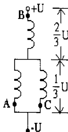
Hình 5.10b: T_2 - T_3 - T_4 dẫn
