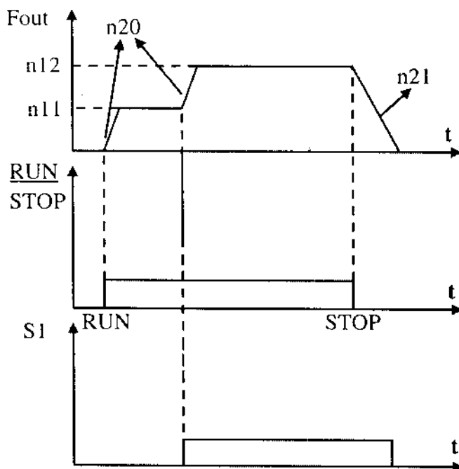
Hình 6.9: Điều khiển hai cấp tốc độ
