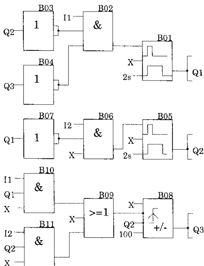
Sơ đồ đóng mở cửa bãi xe tự động theo kiểu FBD
