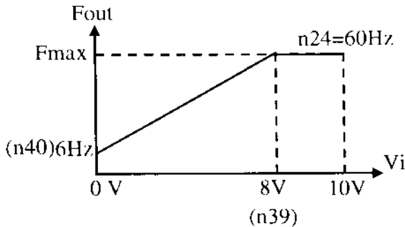
Hình 6.13b: n39 = 0,8 \Rightarrow V_i = 8V
