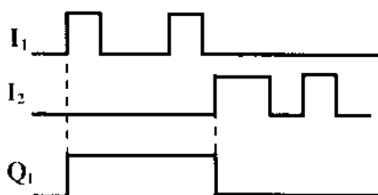
Đáp ứng ngõ vào và ra
