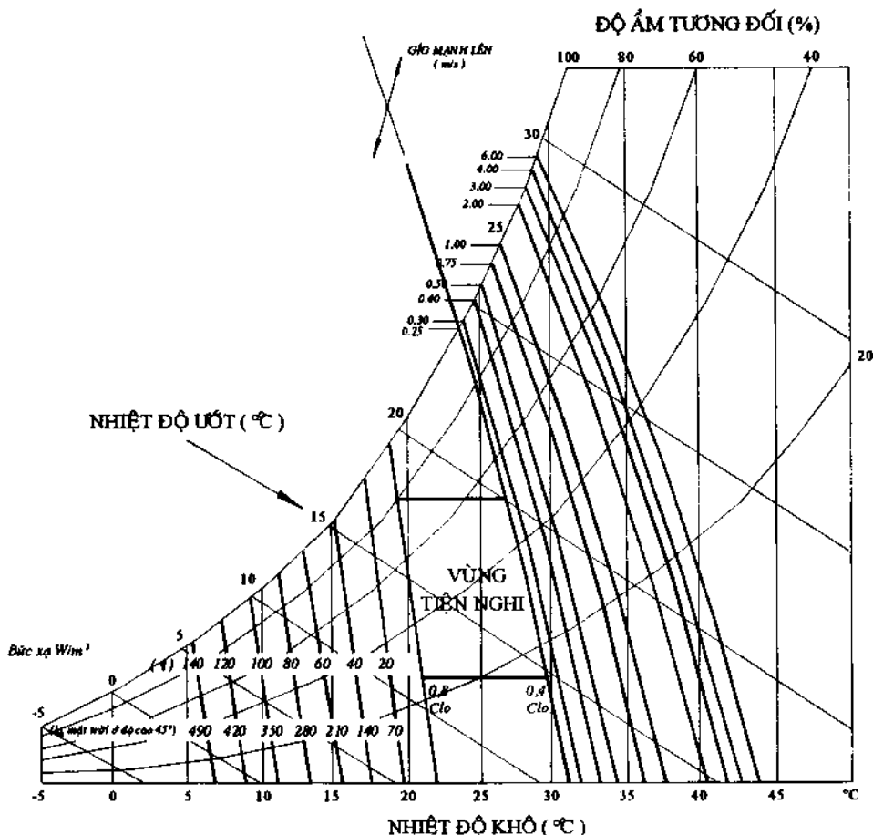
Hình 3.12. Ảnh hưởng của sương ẩm và quạt gió đến vùng tiện nghi
