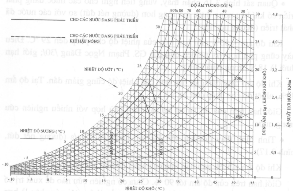
Hình 3.16. Giới hạn vùng tiện nghi khi lặng gió.
