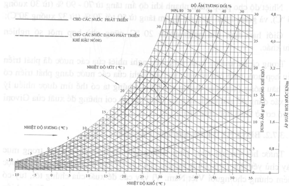
Hình 3.17. Giới hạn vùng tiện nghi khi vận tốc gió là 2 m/s.
