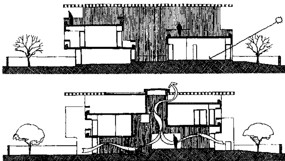
Hình 6.1.9. Nhà Parekh, Ahmedabad, Ấn Độ, KTS Charles Correa.
