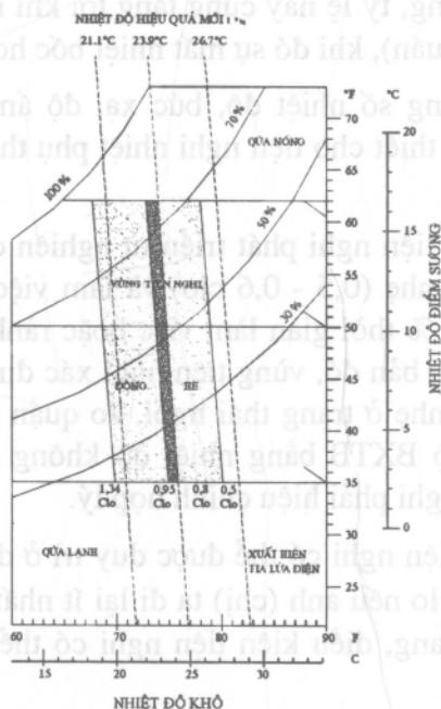
Hình 3.11. Biểu đồ vùng tiện nghi
