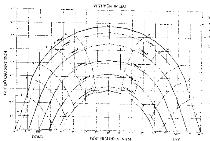
Hình 1.10. BĐMT vẽ theo phép chiếu trụ đứng
