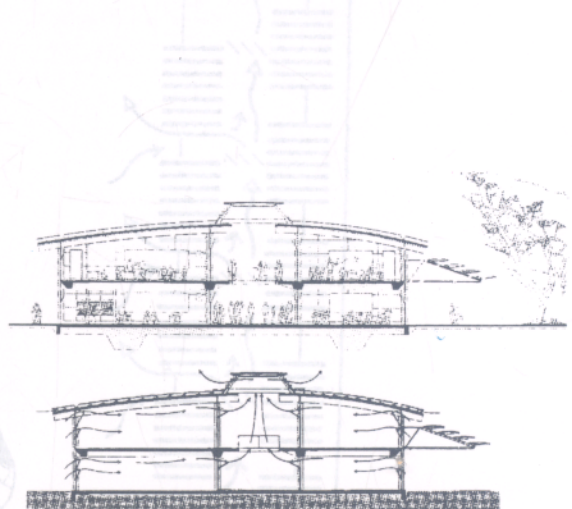
H.7.9c. Mặt cắt ngang
