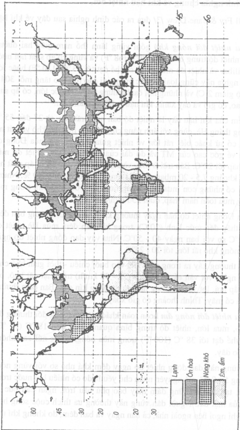
Hình 1.23. Các vùng khí hậu thế giới
