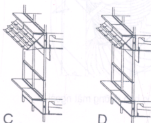
H.7.7c. Kết cấu che nắng
