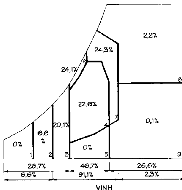
Hình 4.3. Phân tích sinh khí hậu Vinh (cách 1)
