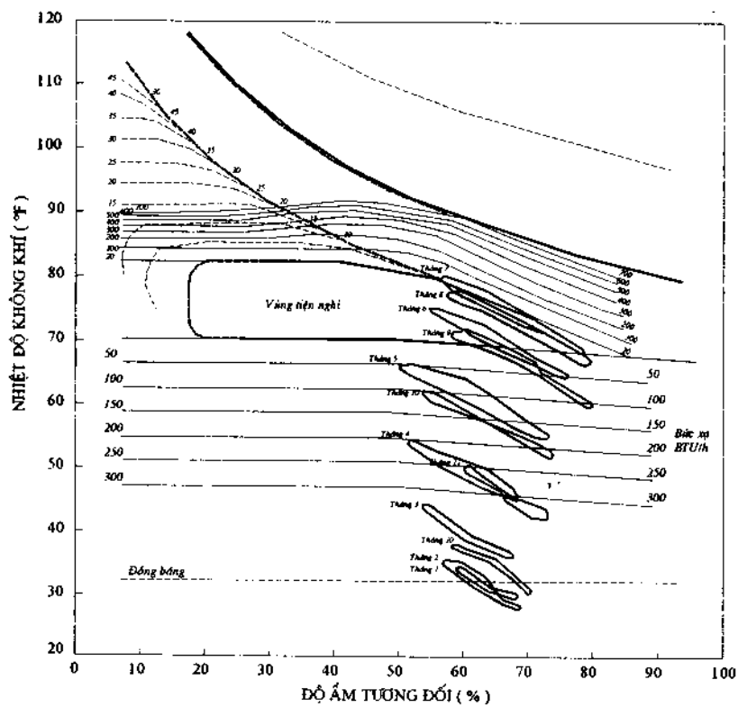
Hình 3.13. Biểu đồ sinh khí hậu của Olgyay
