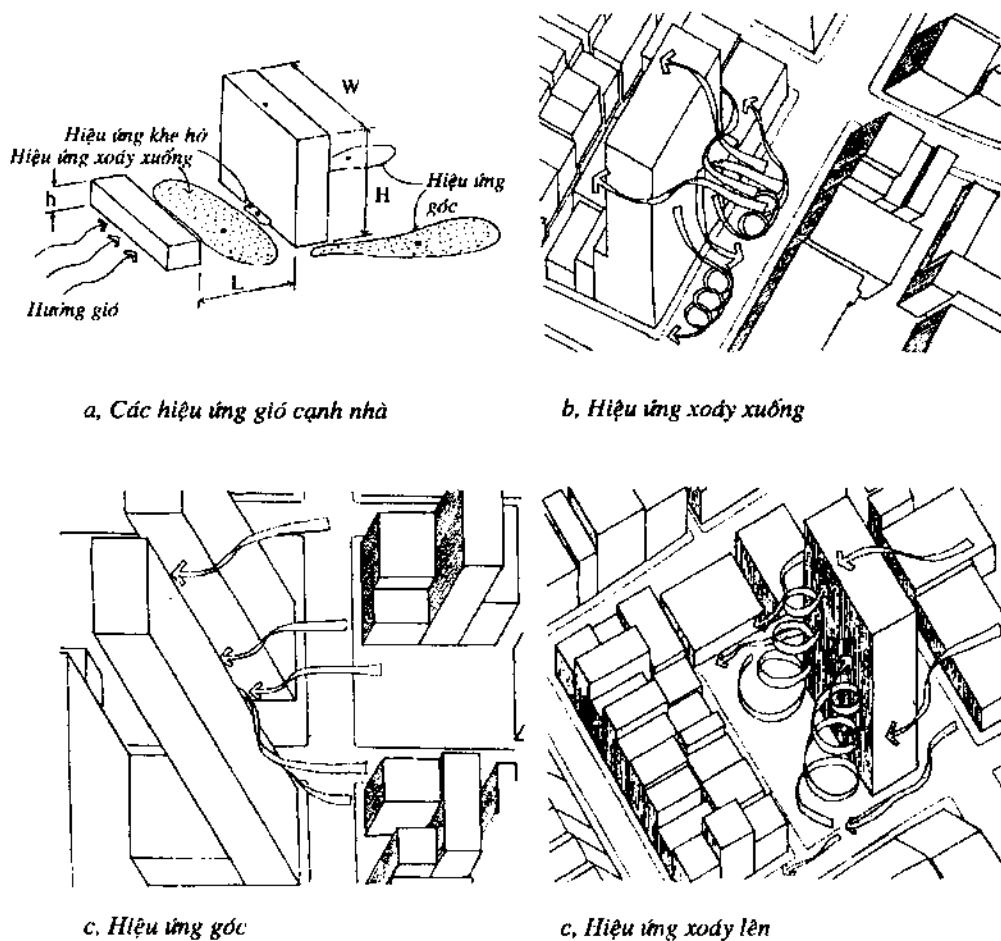
Hình 6.1.6. Các hiệu ứng gió cạnh công trình
