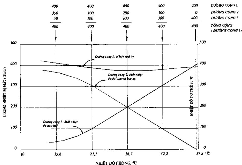
Hình 3.5. Quan hệ giữa nhiệt sinh lý, nhiệt bốc hơi, đối lưu và nhiệt độ phòng.
