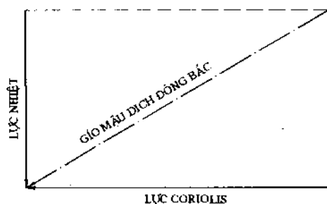
Hình 1.14. Sự hình thành gió Đông Bắc ở phía Bắc xích đạo
