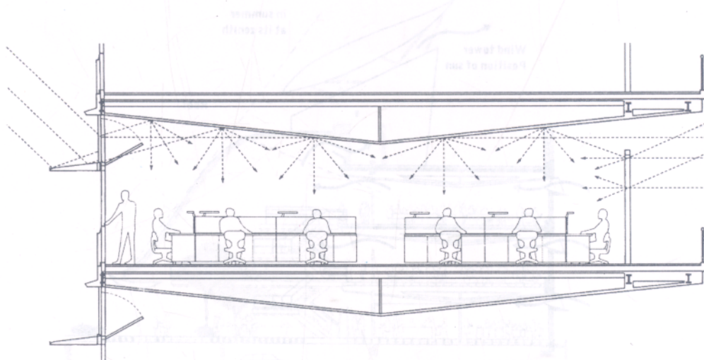
H.7.2d. Trần sử dụng ánh sáng phản xạ
