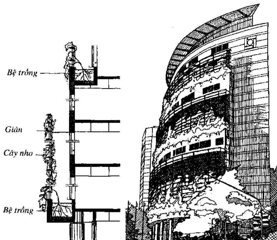
Mặt cắt dọc hướng Tây
