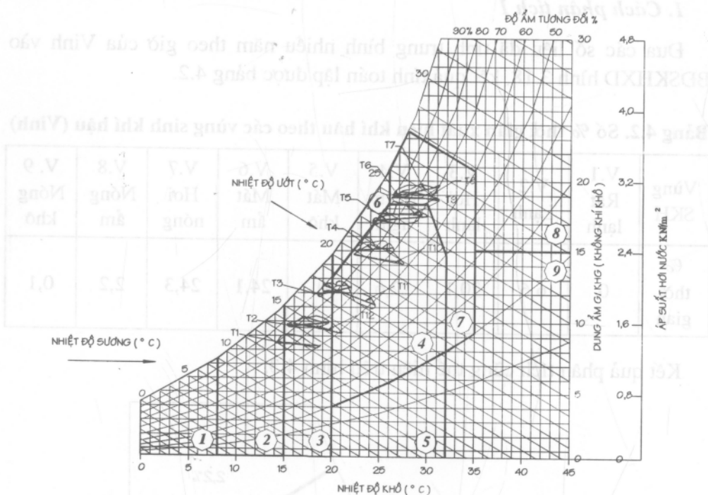
Hình 4.2. Phân tích sinh khí hậu Hà Nội theo biến trình tháng (cách 2 và 3)
