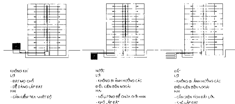
Hình 5.10. Ưu và khuyết điểm của ba loại bơm nhiệt khác nhau
