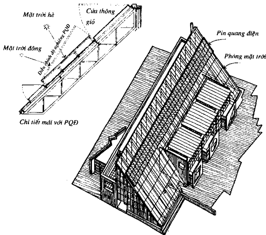
Hình 6.6.3. Nhà trẻ ở Frankfurt, CHLB Đức. KTS Funk & Schroder.
