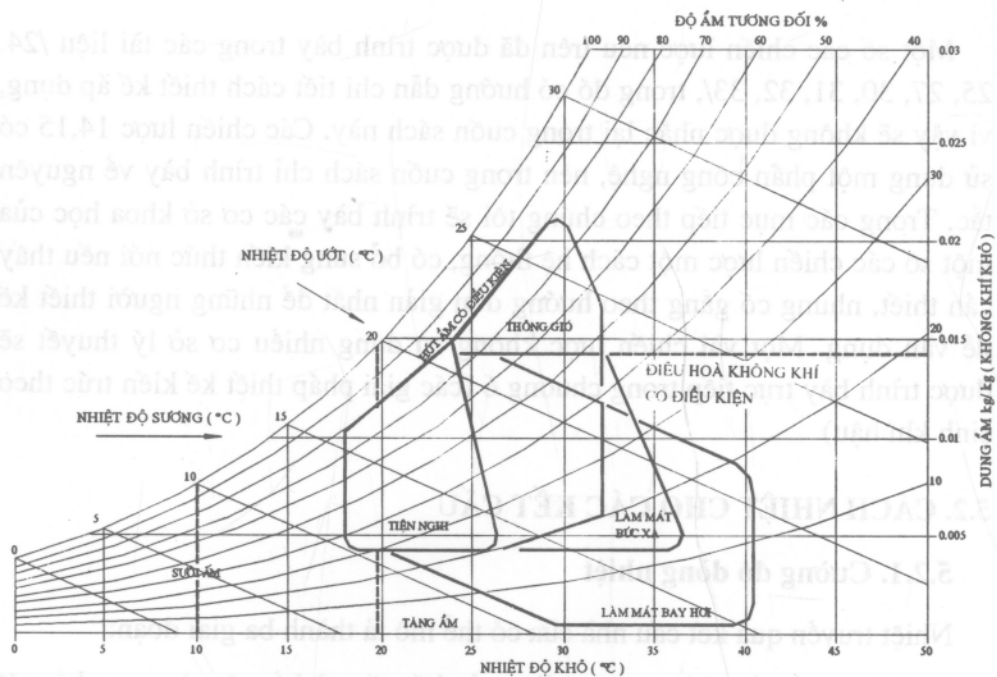
Hình 5.1. Hiệu quả và phạm vi áp dụng các chiến lược thiết kế sinh khí hậu
