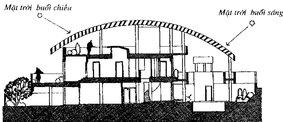
Hình 6.2.1. Nhà mái chống mái ở Kuala Lumpur, Malaysia, của KTS. Ken Yeang.
