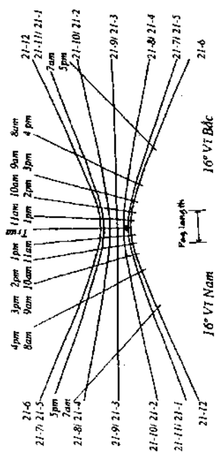
Biểu đồ bóng ở 16°
