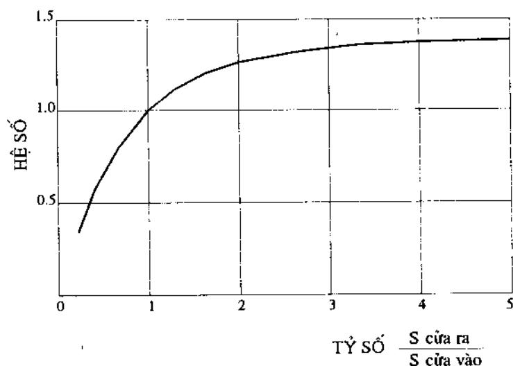
Hình 5.3. Hệ số phụ thuộc tỷ số diện tích cửa thoát gió và cửa đón gió
