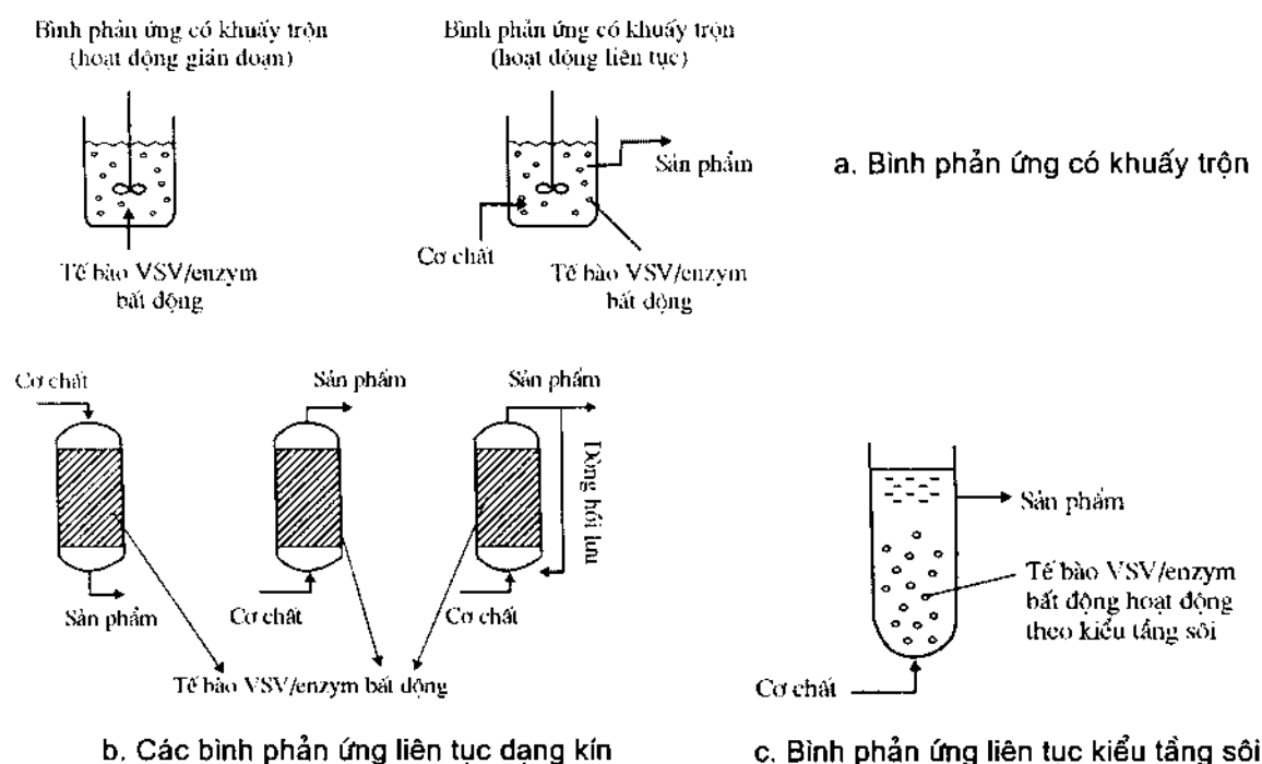
Hình 4.5. Các kiểu bình phản ứng sinh học chứa enzym hoặc tế bào bất động
