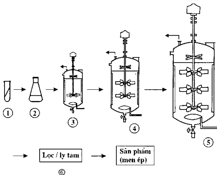
Hình 5.2. Sơ đồ qui trình sản xuất men bánh mì
