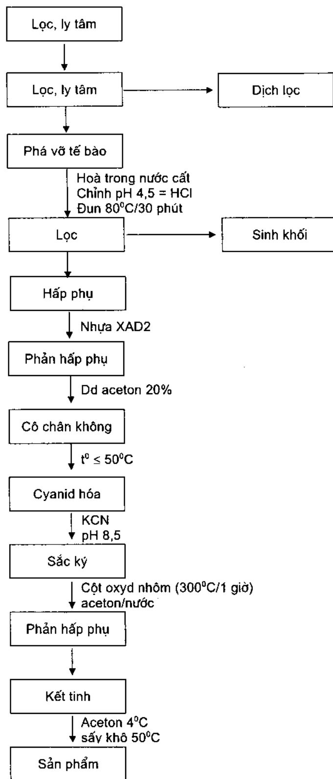
Hình 6.5b. Các công đoạn chiết xuất và tinh chế vitamin B 12 bằng nhựa hấp phụ
