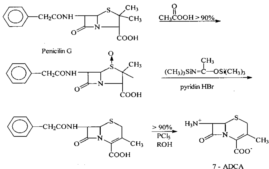
Hình 8.5b. Sơ đồ phản ứng hoá học điều chế 7-ADCA từ penicillin G
