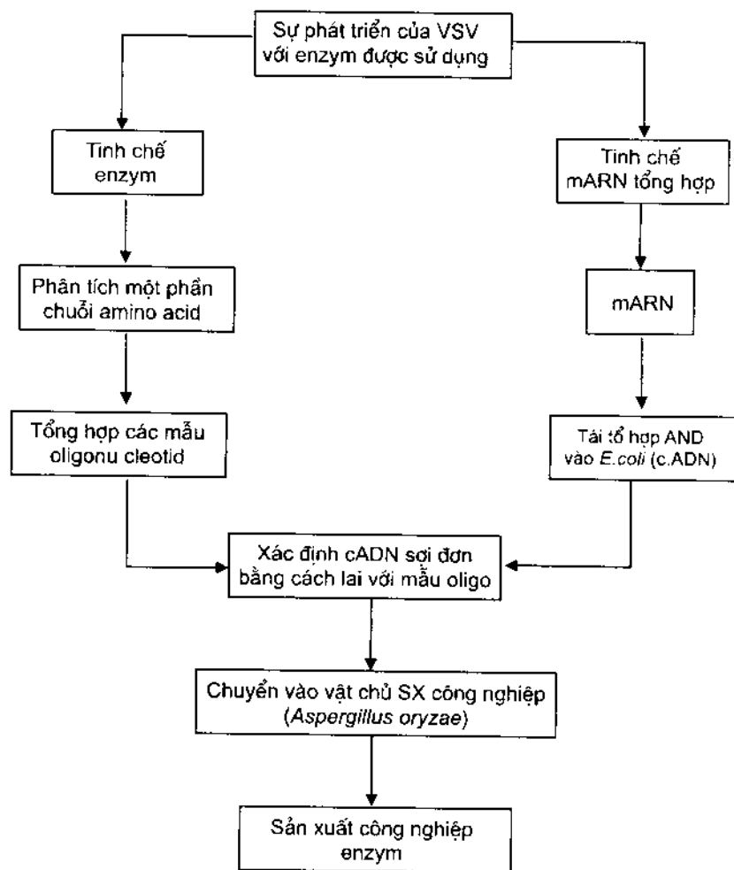
Hình 4.1. Nguyên tắc chuyển gen để tạo enzym
