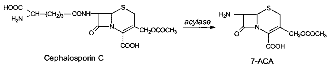
Hình 8.5a. Sơ đồ sản xuất 7-ACA từ cephalosporin C bằng con đường sinh học
