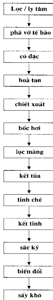
Hình 3.10. Các công đoạn tinh chế sản phẩm
