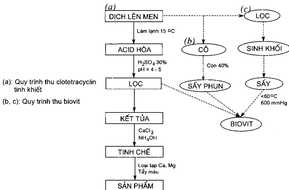
Hình 9.3. Quy trình xử lý dịch lên men clotetracyclin
