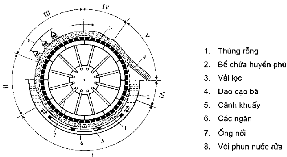
Hình 3.8. Sơ đồ cắt ngang máy lọc chân không hình trống quay
