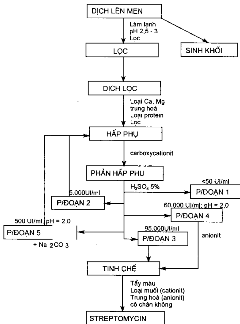
Hình 10.2. Quy trình chiết xuất và tinh chế streptomycin
