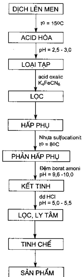
Hình 9.5. Các công đoạn chiết oxytetracyclin bằng dung môi hữu cơ
