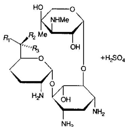
Bảng 10.3. Cấu trúc hoá học của gentamicin theo Dược điển Anh BP 2003
