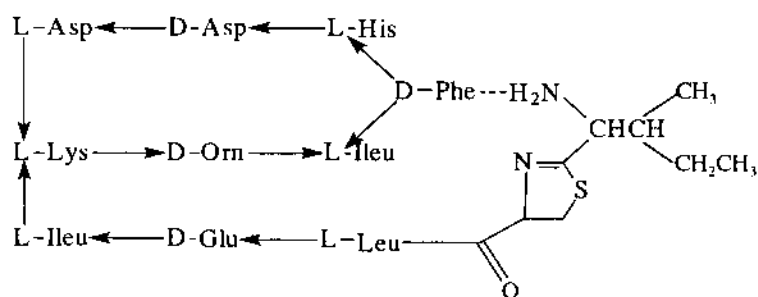
Hình 13.2. Cấu trúc hóa học của phân tử bacitracin A
