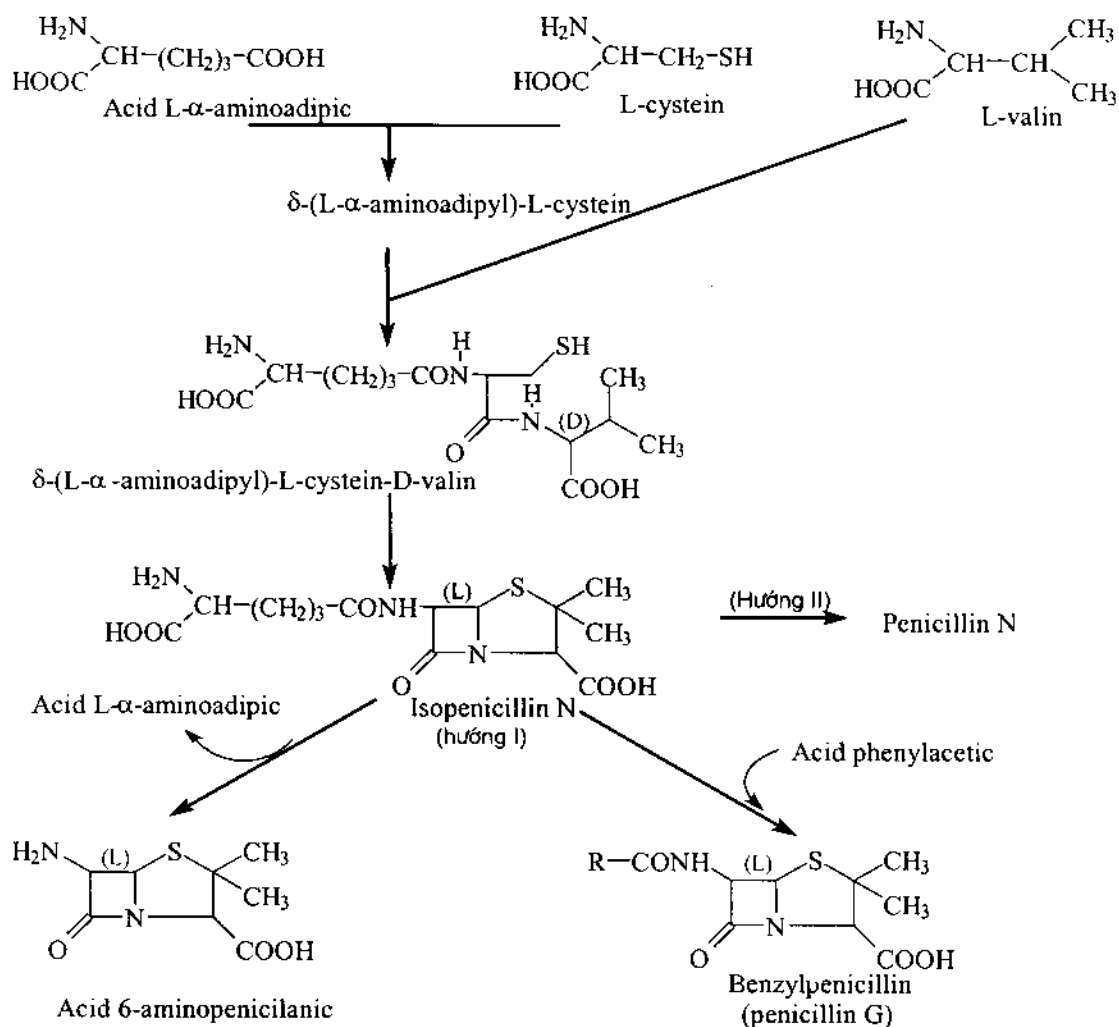
Hình 8.3. Quá trình sinh tổng hợp penicillin từ các amino acid
