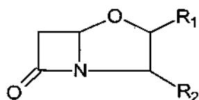
Bảng 8.7. Cấu trúc các kháng sinh clavam tự nhiên
