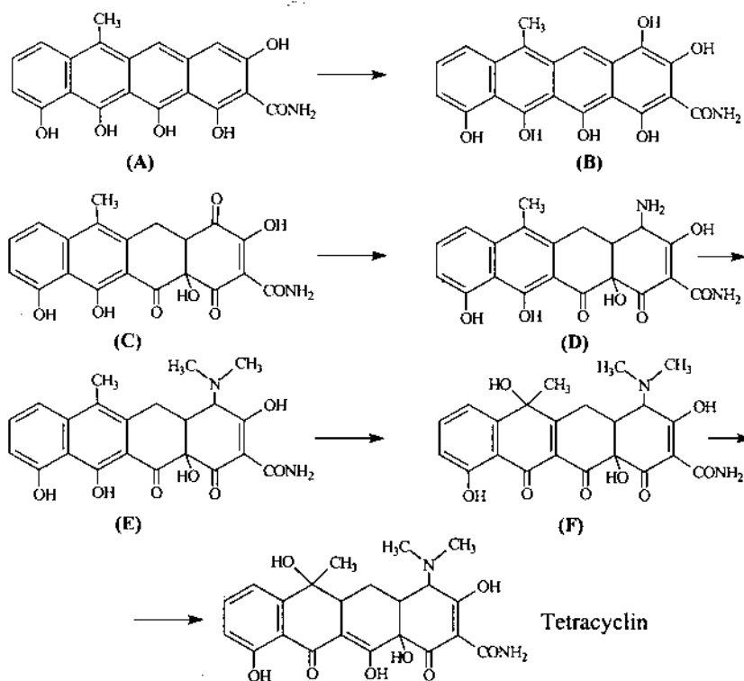
Hình 9.1. Cơ chế sinh tổng hợp tetracyclin từ pretetramid (A)
