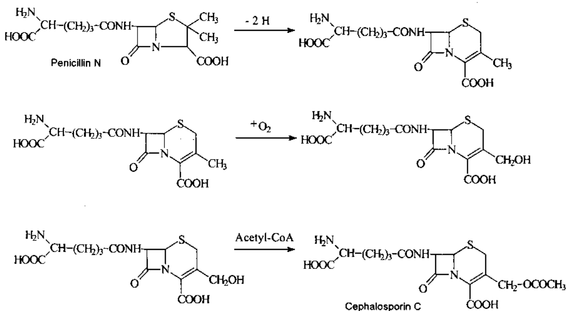
Hình 8.4. Cơ chế sinh tổng hợp cephalosporin C (giai đoạn cuối từ penicillin N)
