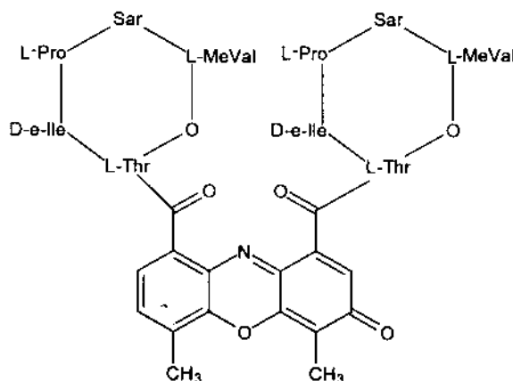
Hình 12.1. Cấu trúc actinomycin D
