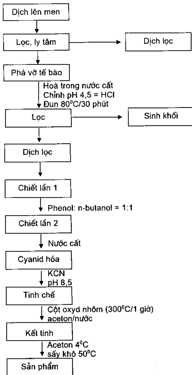
Hình 6.5a. Các công đoạn chiết xuất và tinh chế vitamin B 12 bằng dung môi hữu cơ
