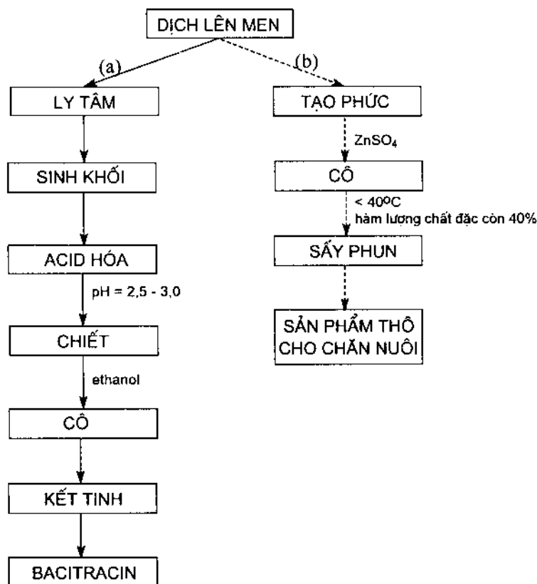
Hình 13.3. Quy trình chiết xuất bacitracin trong y học (a) và trong chăn nuôi (b)
