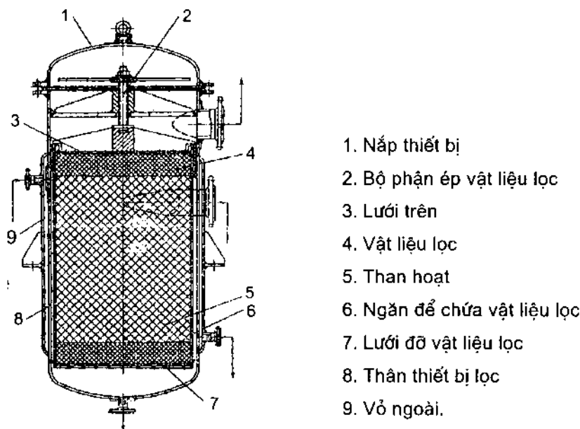
Hình 3.6. Thiết bị lọc khí vô trùng
