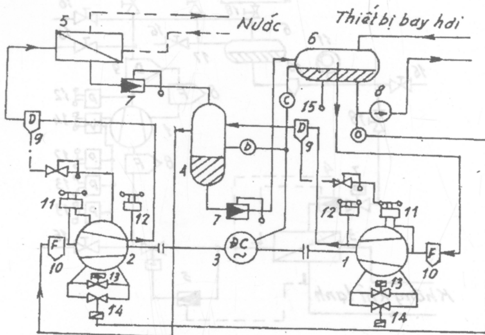
Hình 26. Sơ đồ đơn giản tổ hợp máy nén bình ngưng \text{NH}_3 , 2 cấp nén
