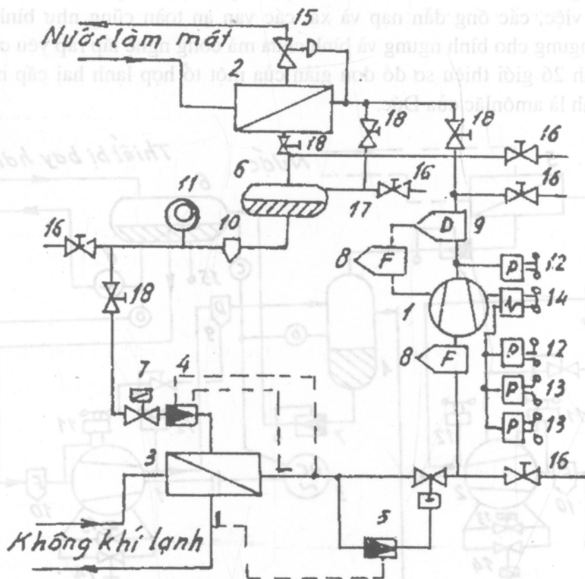
Hình 25. Sơ đồ máy lạnh một cấp điều hoà không khí trên tàu thủy của Đức
