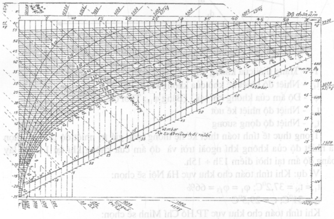
Hình 1. Đồ thị h - d (Entanpi - Độ chứa hơi) của không khí ẩm
