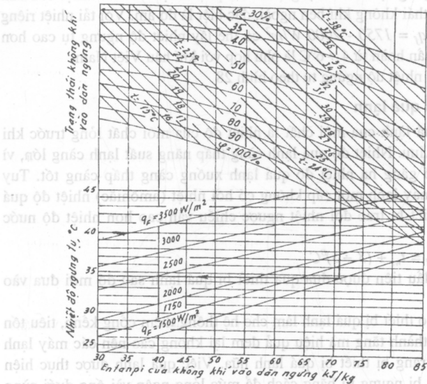
Hình 28. Đồ thị xác định nhiệt độ ngưng tụ cho dàn ngưng tươi
