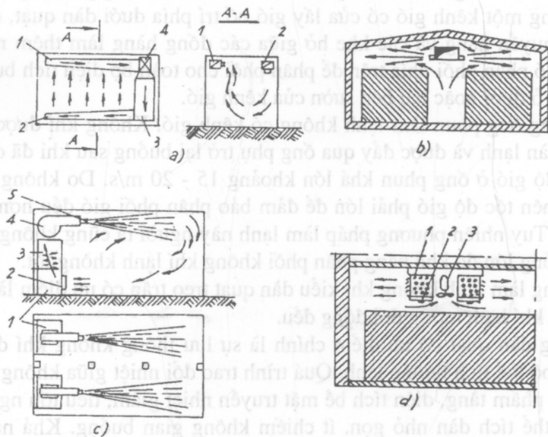
Hình 17. Sơ đồ hệ thống tuần hoàn không khí
