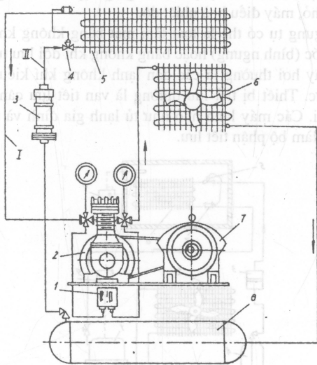
Hình 19. Sơ đồ hệ thống lạnh dùng máy nén hở
