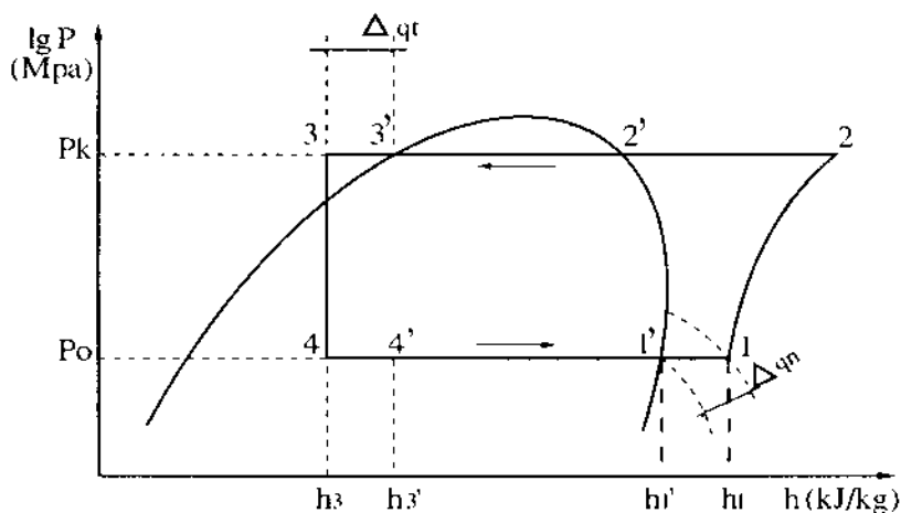
b, Hình 29. Chu trình một cấp amôniac
