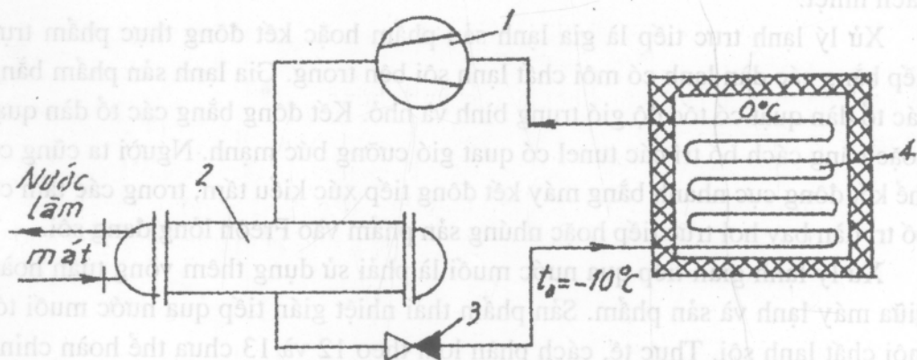
Hình 14. Sơ đồ đơn giản làm lạnh buồng trực tiếp
