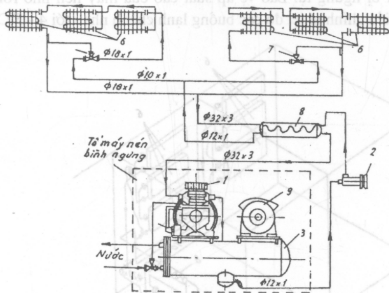
Hình 20. Sơ đồ hệ thống lạnh dùng máy nén AK-ΦB6
