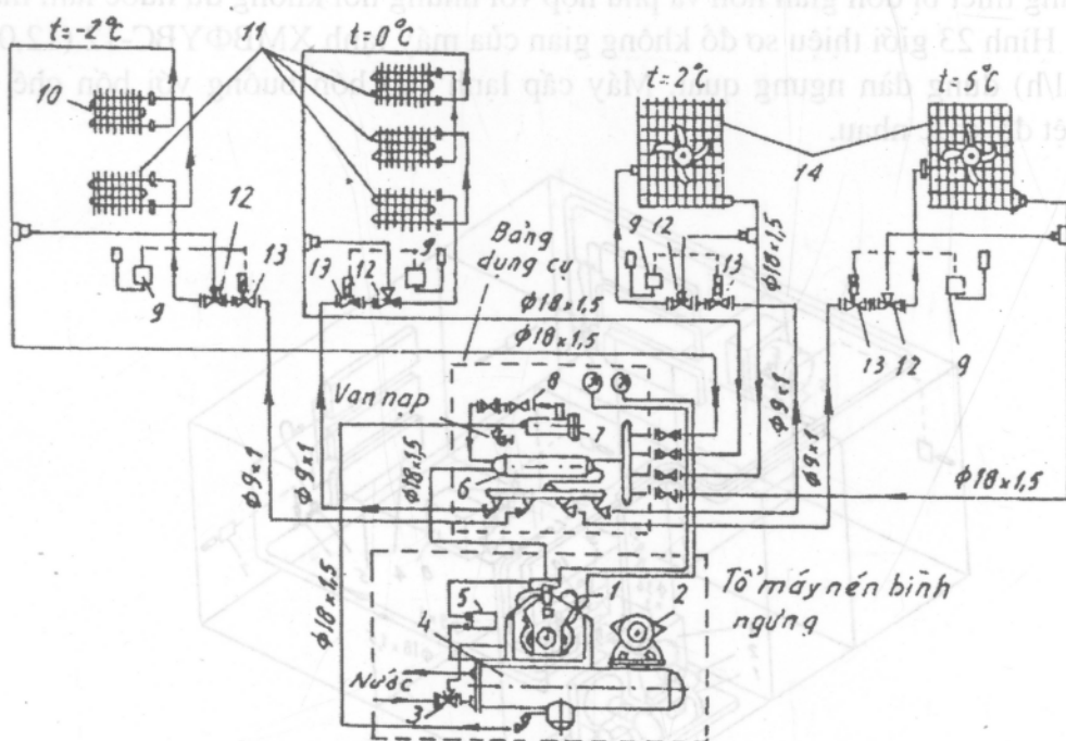
Hình 22. Sơ đồ nguyên lý máy lạnh XM-PY8
