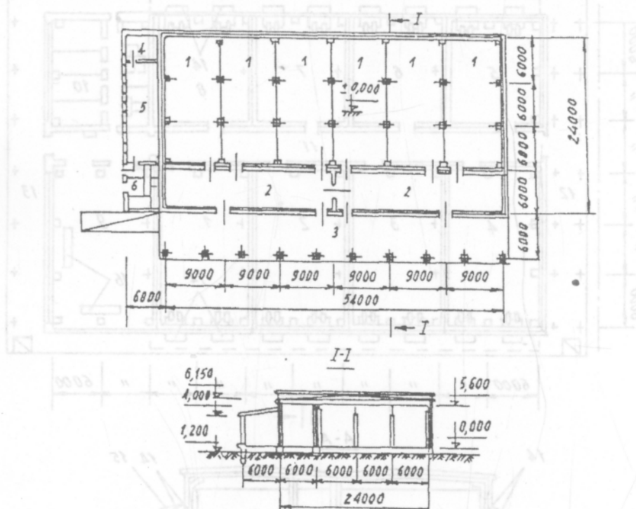
Hình 6. Mặt bằng kho lạnh rau quả và rượu vang 700t
