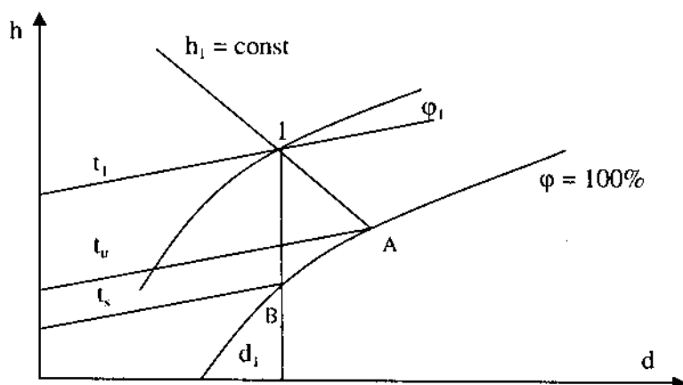
Hình 2a. Phương pháp xác định các giá trị nhiệt độ nhiệt kế ướt t_w và nhiệt độ đọng sương t_s của không khí ẩm trên đồ thị h - d .
