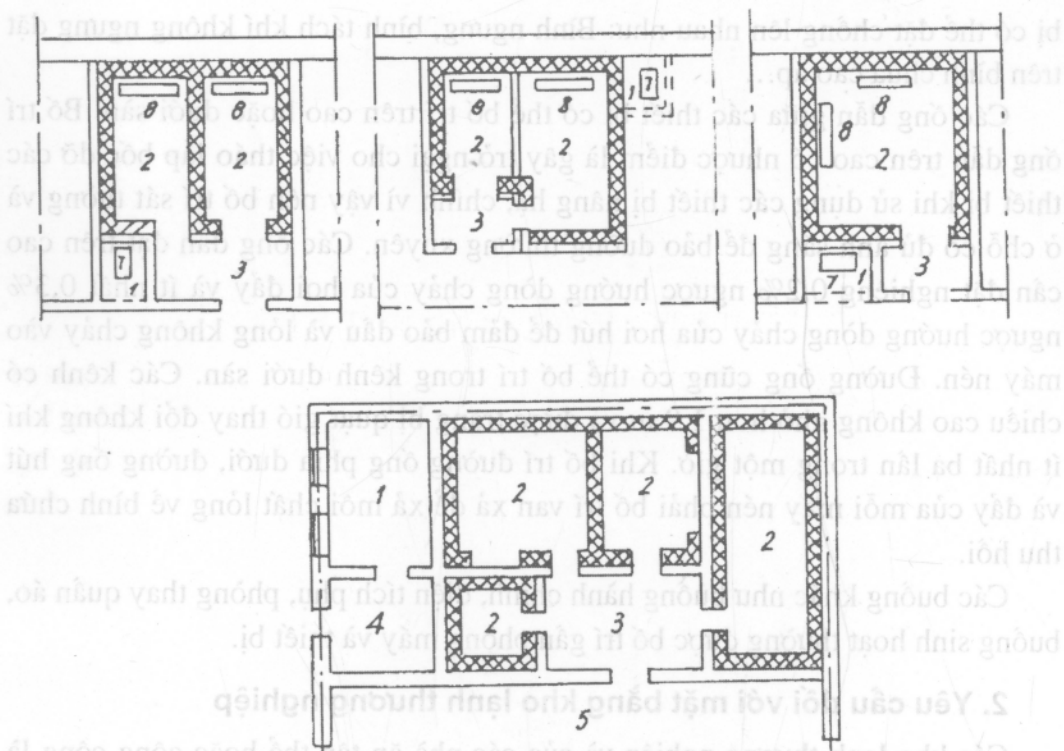
Hình 9. Một số phương án mặt bằng kho lạnh thương nghiệp
