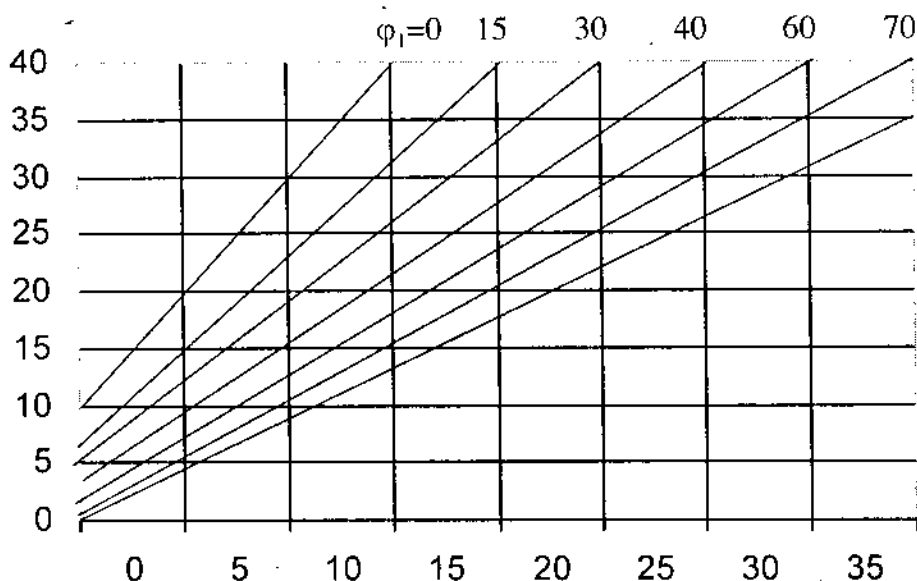
Hình 2b. Sự phụ thuộc của nhiệt độ nhiệt kế ướt vào nhiệt độ không khí t_{kk} và độ ẩm tương đối \varphi_0
