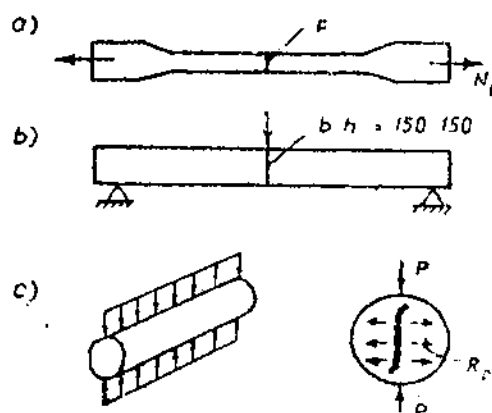
Hình 3.2. Mẫu xác định
