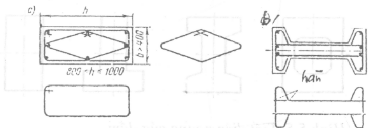
Hình 5.7. Cốt đai
