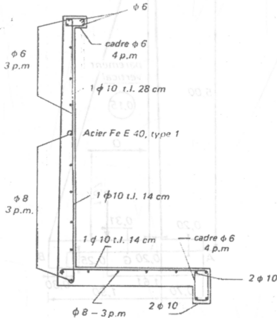
Hình 1.2. Sơ đồ bố trí cốt thép
