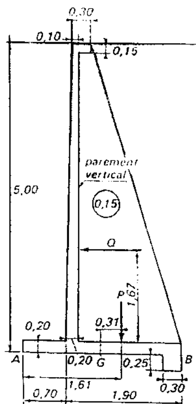
Hình 2.1. Tường chắn có tường ốp
