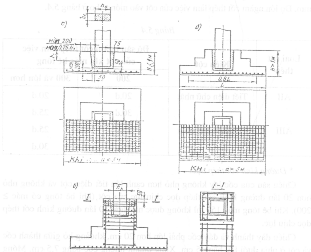
Hình 5.24. Móng bê tông cốt thép nguyên khối dưới cột lắp ghép
