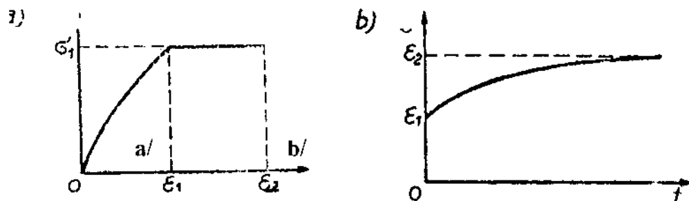
Hình 3.4. Biến dạng của bê tông do tải trọng tác dụng dài hạn a/ Đồ thị ứng suất biến dạng b/ Đồ thị biến dạng theo thời gian
