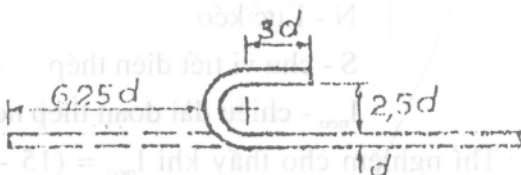
Hình 3.7. Kích thước móc neo
