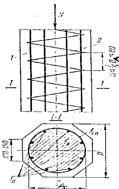
Hình 5.2. Cột có cốt xiên
