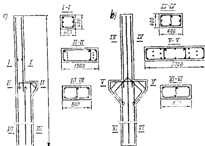
Hình 5.20. Cột chịu nén lệch tâm
