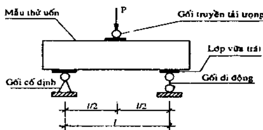
Hình 1.3. Mẫu thử uốn
