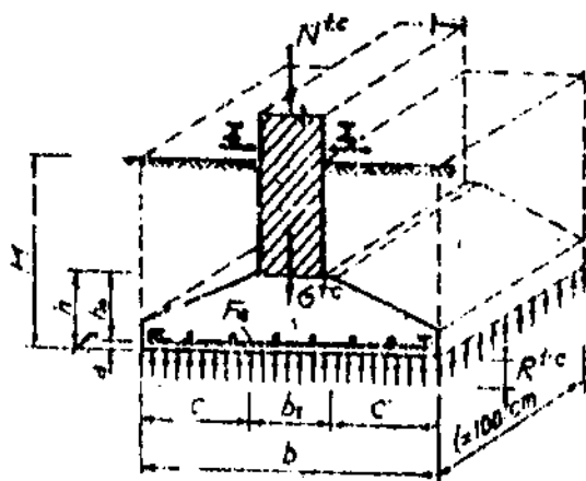
Hình 5.25. Sơ đồ tính toán
