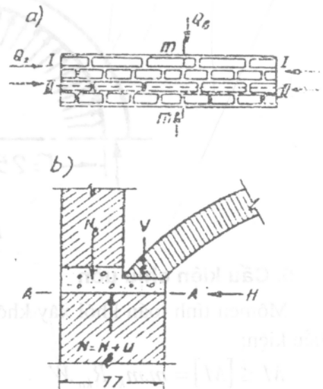
Hình 2.6. Khối xây chịu cắt
