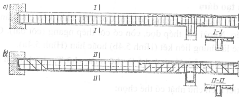
Hình 5.4. Dầm bê tông cốt thép
