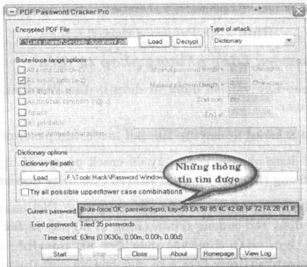
Hình 3.41: Những thông tin tìm được.
