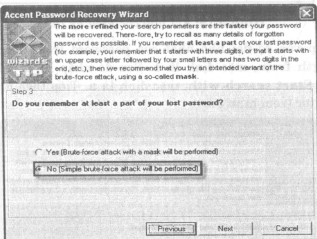
Hình 3.18: Thực hiện crack bằng Brute-force.
