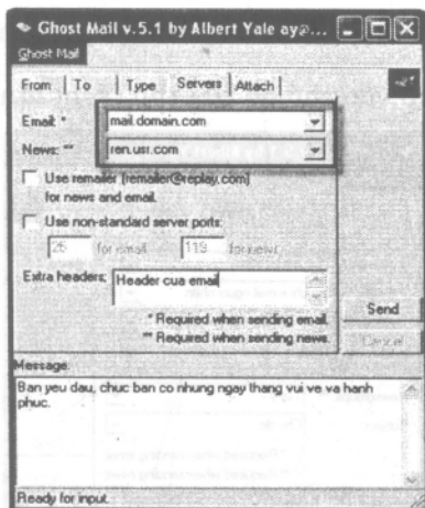
Hình 1.13: Những thiết lập trong thẻ Servers.
