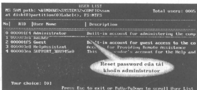
Hình 2.15: Loại bỏ password Administrator.
