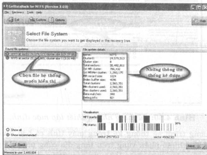
Hình 4.32: Những thông tin thống kê được.
