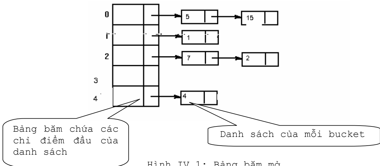
Hình IV.1: Bảng băm mở
