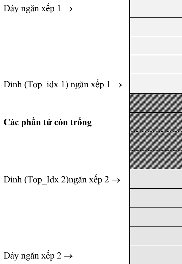
Hình vẽ mảng chứa 2 ngăn xếp
