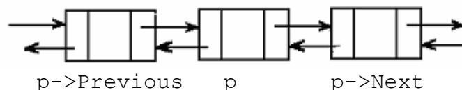
Hình II.17: Danh sách trước khi thêm phần tử x
