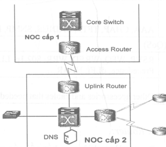
Hình 3: Sơ đồ kết nối thiết bị của NOC cấp 2
