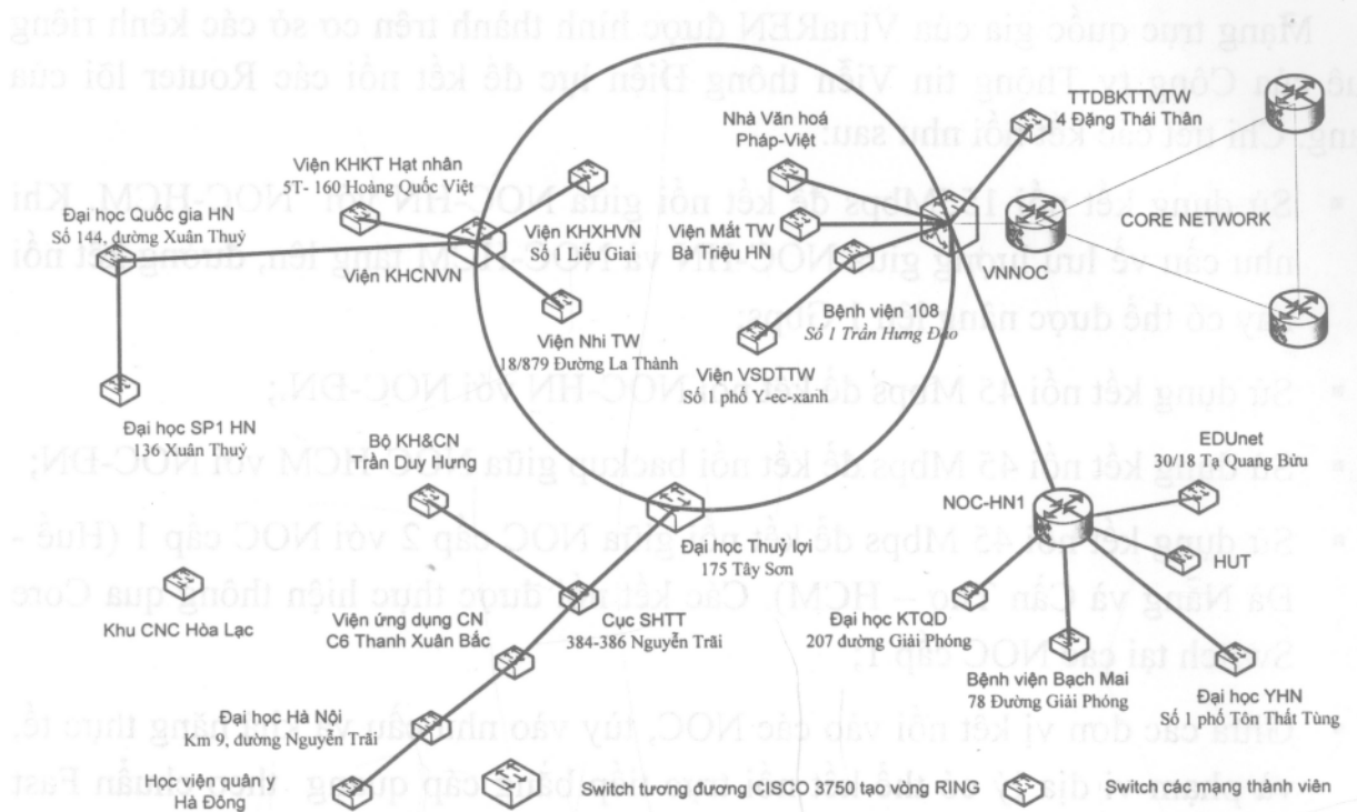
Hình 5: Kết nối cáp quang tại thành phố Hà Nội
