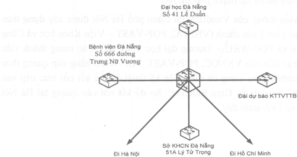
Hình 6: Sơ đồ kết nối cáp quang tại thành phố Đà Nẵng
