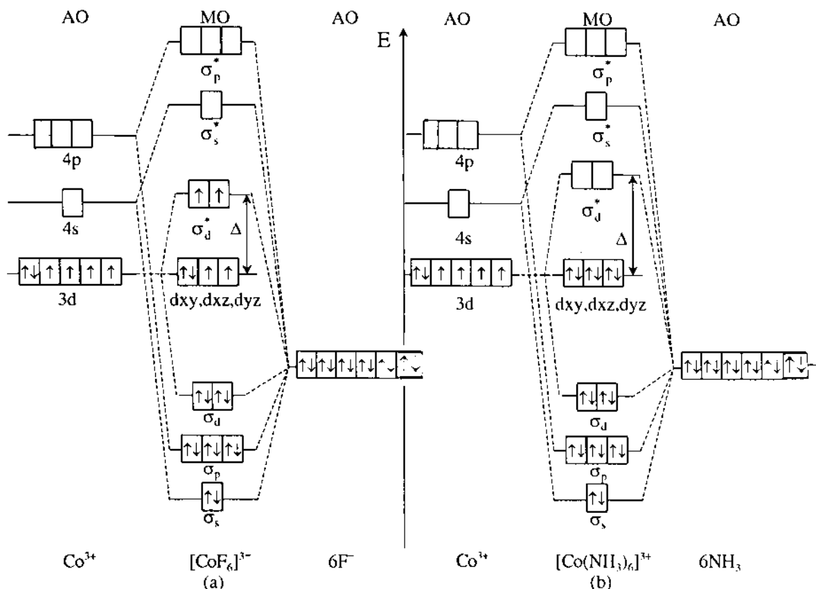
Hình 3.56. Sơ đồ các mức năng lượng MO của các phức chất [CoF_6]^{3-} cao spin (a) và [Co(NH_3)_6]^{3+} thấp spin (b).
