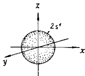
Hình 2.16. Cấu trúc electron của nguyên tử liti.
