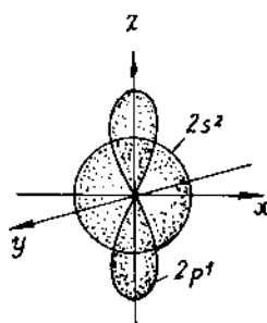
Hình 2.18. Cấu trúc electron của nguyên tử bo.
