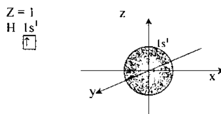
Hình 2.14. Cấu trúc electron của nguyên tử hydro.
