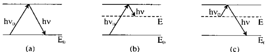
Hình 4.17. Các trường hợp tán xạ:
