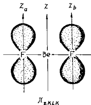
Hình 3.43. MO \pi_{LK} 3 tâm trong BeF_2 .
