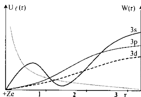
Hình 2.12. Sự phụ thuộc U_\ell(r) và W(r) .
