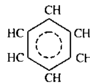
Hình 3.24. Các AO không lai hóa trong phân tử C_6H_6 .
