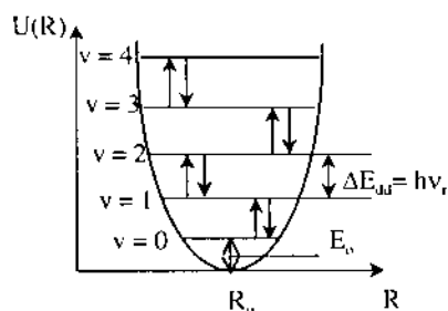
Hình 4.10. Dao động điều hòa.
