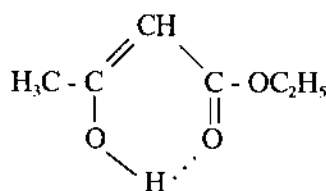
enol
