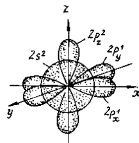
Hình 2.21. Cấu trúc electron của nguyên tử oxy.
