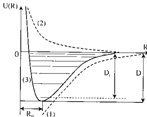
Hình 3.2. Sự phụ thuộc U(R) vào R .
