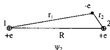
Hình 3.31. Hệ H_2^+ khi electron ở gần hạt nhân 2.
