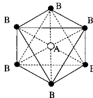
Hình 3.29. Lai hóa d^2sp^3 .
