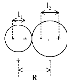
Hình 3.5. Phân cực hóa ion.
