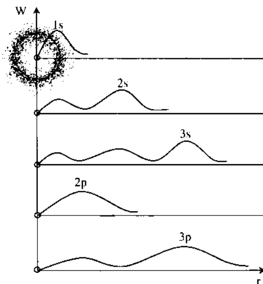
Hình 2.6. Sự phụ thuộc W(r) vào r .
