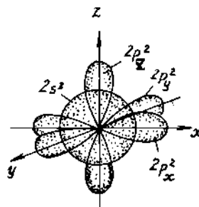
Hình 2.23. Cấu trúc electron của nguyên tử neon.
