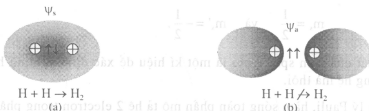
Hình 3.12. Sự phân bố mật độ electron khi hai electron có: a. có spin phản song song; b. có spin song song.
