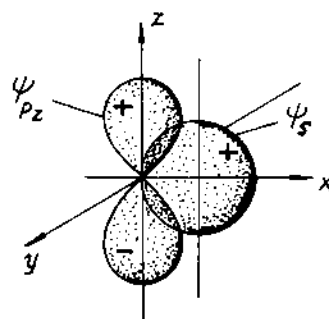
Hình 2.4. Tính chất trực giao của \psi_{pz} và \psi_s .
