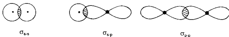
Hình 3.16. Liên kết \sigma .
