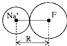
Hình 3.3. Phân tử ion \text{Na}^+\text{F}^- .
