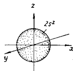
Hình 2.17. Cấu trúc electron của nguyên tử beri.
