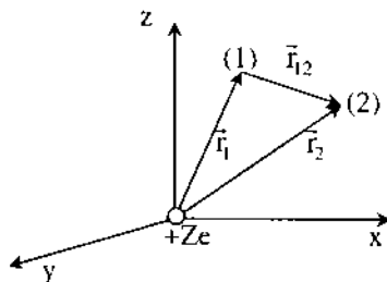
Hình 2.11. Tương tác trong nguyên tử He.
