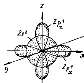
Hình 2.19. Cấu trúc electron của nguyên tử cacbon.
