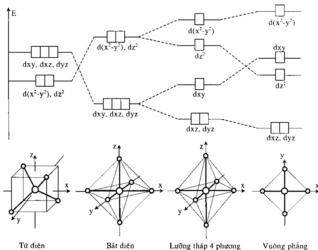
Hình 3.53. Sơ đồ tách mức năng lượng các orbital d trong một số trường ligan.
