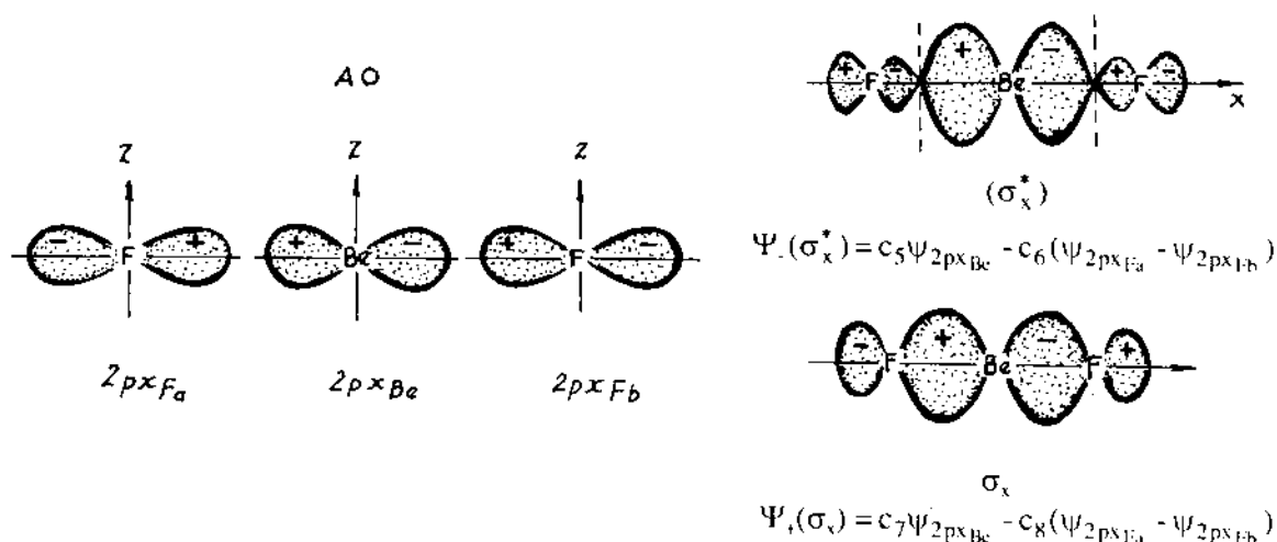
Hình 3.42. Sơ đồ tạo thành MO \sigma_x và \sigma_x^* trong BeF_2 .
