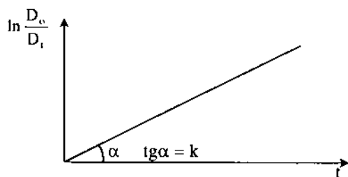
Hình 4.14. Xác định hằng số tốc độ phản ứng.
