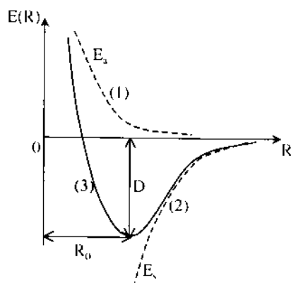
Hình 3.11. Sự phụ thuộc E vào R .
