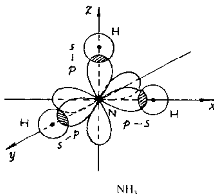
Hình 3.14. Xen phủ s-p trong phân tử NH_3 .
