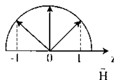
Hình 2.7. M_z mômen động lượng M của các electron p ( \ell = 1; m = 0, \pm 1 ).
