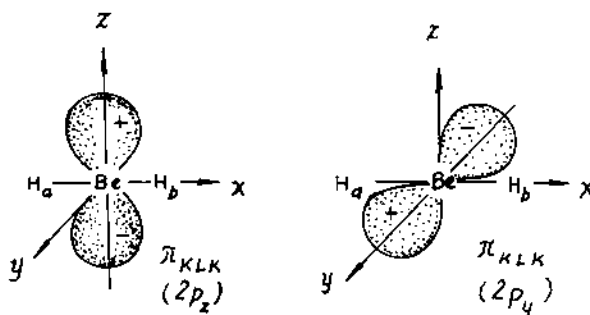
Hình 3.39. Các MO \pi_{\text{KLK}} trong phân tử \text{BeH}_2 .
