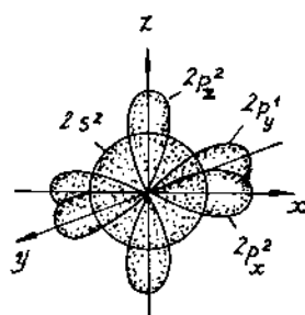
Hình 2.22. Cấu trúc electron của nguyên tử flo.
