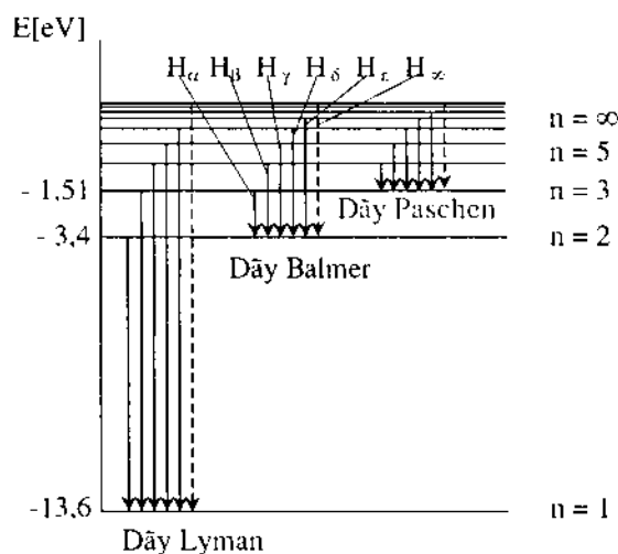
Hình 2.2a. Các mức năng lượng và các bước chuyển dời electron trong nguyên tử hydro
