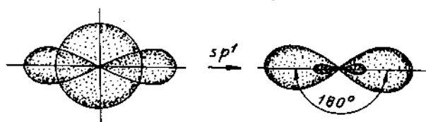
Các orbital (s+p)
