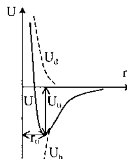
Hình 3.7. Sự phụ thuộc U vào r .
