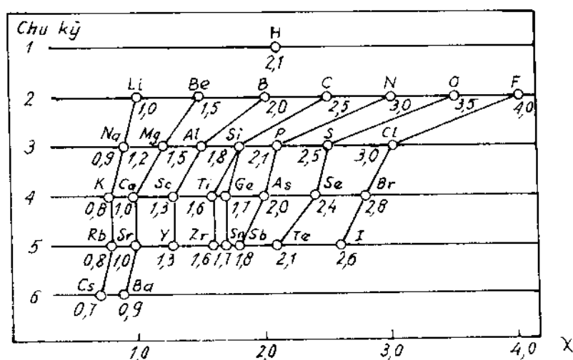
Hình 3.1. Độ âm điện của các nguyên tố.
