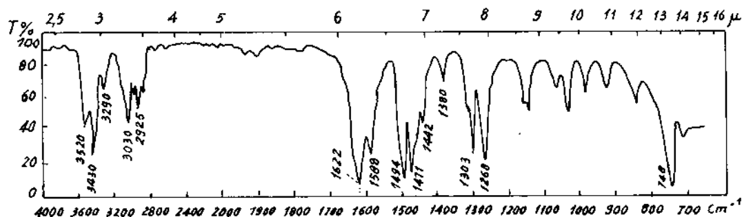
Hình 4.13. Phổ hồng ngoại của C 7 H 9 N.
