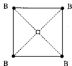
Hình 3.28. Lai hóa dsp^2 .
