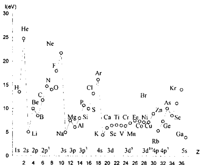
Hình 2.24. Sự phụ thuộc năng lượng ion hóa vào số thứ tự nguyên tố.
