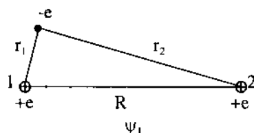
Hình 3.30. Hệ H_2^+ khi electron ở gần hạt nhân 1.
