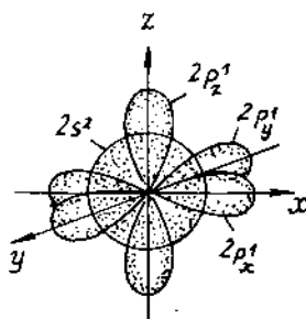
Hình 2.20. Cấu trúc electron của nguyên tử nitơ.
