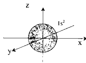
Hình 2.15. Cấu trúc electron của nguyên tử heli.
