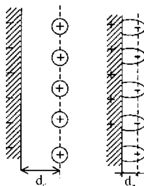
Hình 3.6. Các lớp điện tích kép.
