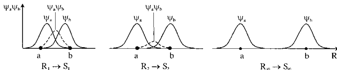
Hình 3.10. Sự phụ thuộc S vào R.
