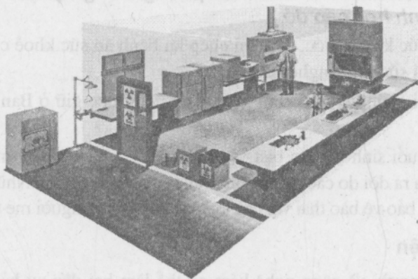
Hình 1.3. Một phòng thí nghiệm an toàn sinh học cấp độ 2 điển hình.
