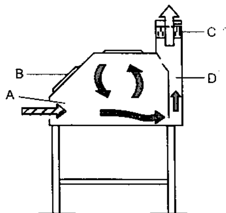
Hình 2.1. Sơ đồ hoạt động của tủ an toàn sinh học loại I
