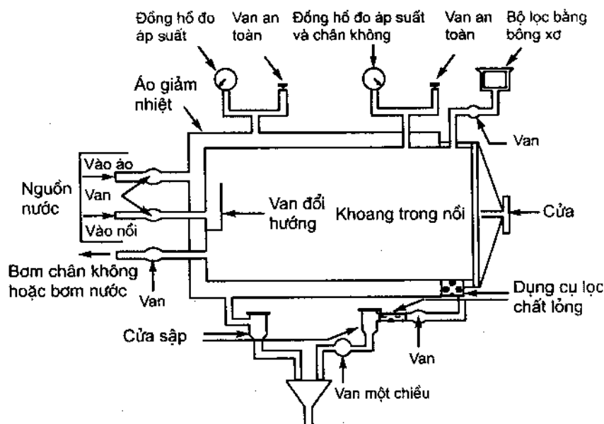
Hình 3.1. Nồi khử trùng hơi thay thế trọng lực
