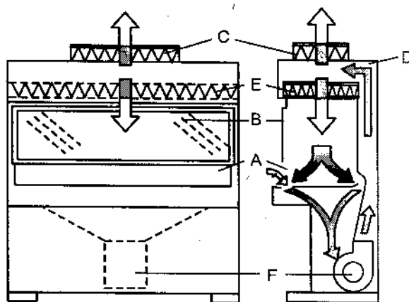
Hình 2.2. Sơ đồ tổng quát các BSC loại IIA1 A. Cửa mở trước; B. Kính chắn; C. Lọc HEPA thoát; D. Ống thoát tổng; E. Lọc HEPA cấp khí; F. Quạt thổi.
