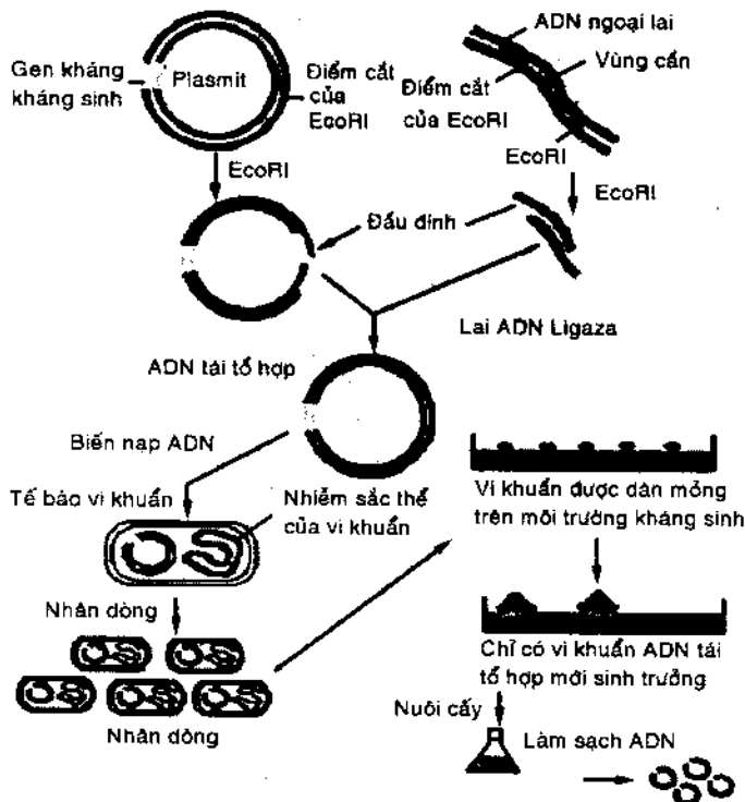
Hình 11.1. Minh họa dưới dạng sơ đồ việc nhân dòng ADN
