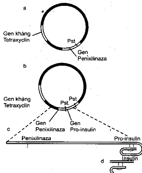
Hình 11.2. Tổng hợp insulin ở E. coli (Nguồn: Sinh học phân tử, Barroso G.)
