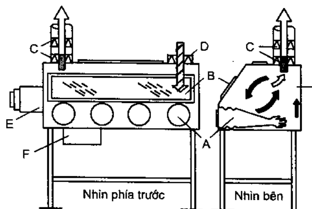
Hình 2.4. Sơ đồ cấu tạo của tủ an toàn sinh học loại III (hộp để găng)
