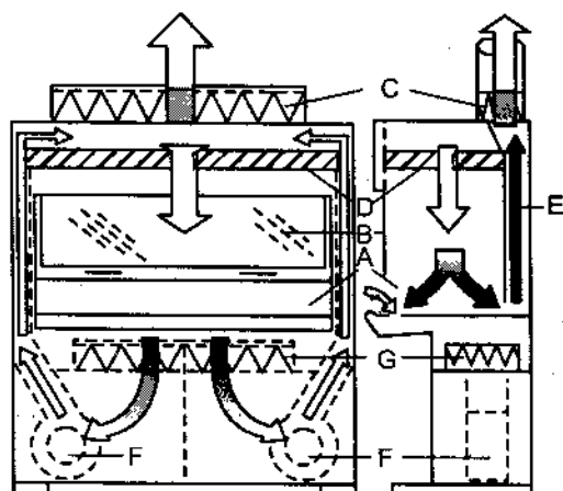
Hình 2.3. Sơ đồ hoạt động của tủ an toàn sinh học loại IIB1
