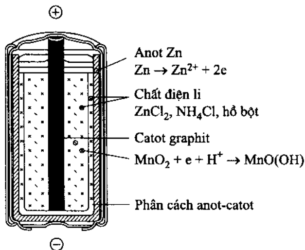
Hình 6.6. Sơ đồ cấu tạo của pin khô.
