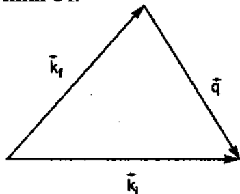
Hình 54. Vectơ sóng tới \vec{k}_i , vectơ sóng tán xạ \vec{k}_f và vectơ sóng \vec{q} .
