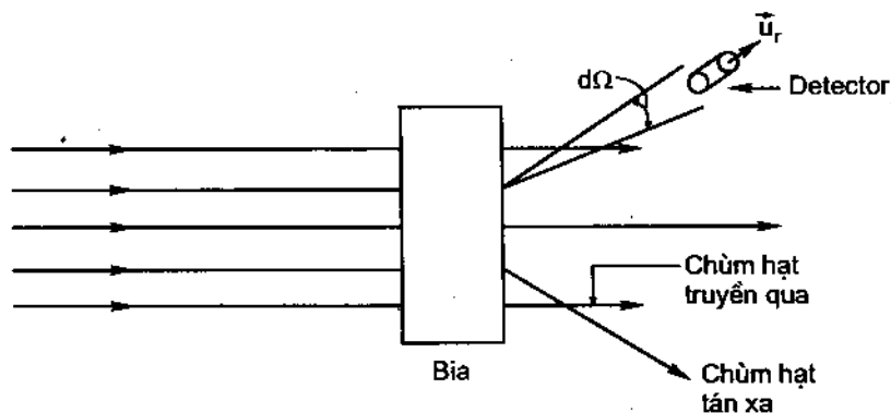
Hình 53. Thí nghiệm tán xạ ba chiều. Máy quan sát hạt đối diện góc khối d\Omega .
