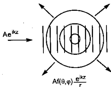
Hình 52. Sơ đồ tóm tắt của một thí nghiệm tán xạ ba chiều chỉ ra sóng phẳng tới và sóng cầu đi khỏi (tán xạ).
