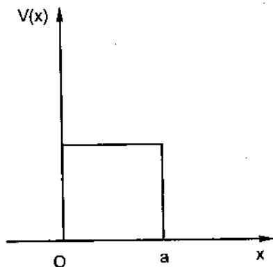
Hình 51. Hàng rào thế bề rộng a trong một thí nghiệm tán xạ một chiều.
