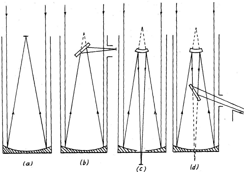
Hình 2. Bốn loại kính thiên văn phản xạ :
