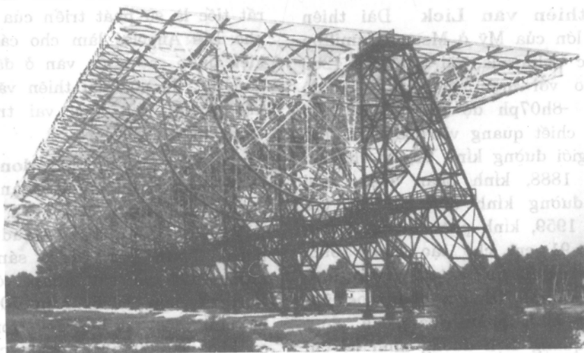
Anten di động của kính thiên văn vô tuyến của đài thiên văn Pari ở Nançay.
