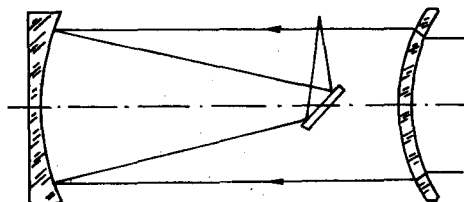
Sơ đồ nguyên lý hệ kính Maksutov.
