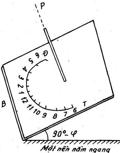
Hình 1. Đồng hồ Mặt Trời kiểu xích đạo.
