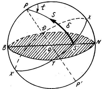
Hệ tọa độ xích đạo 1.
