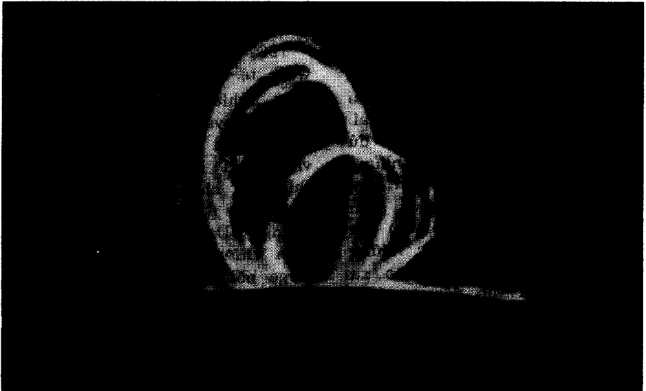
Tai lửa Mặt Trời.
