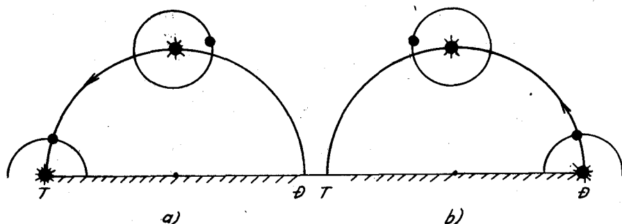
Sao Hôm (a) và Sao Mai (b).
