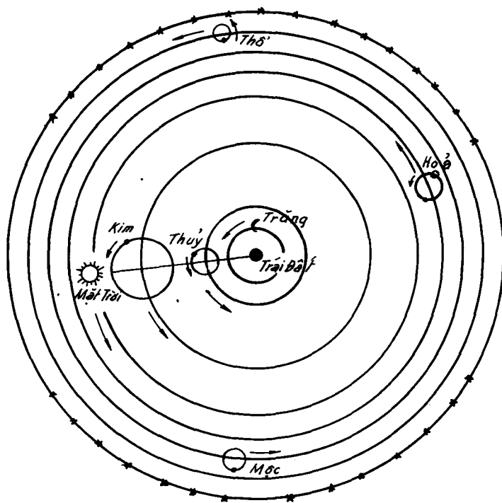
Mô hình địa tâm.
