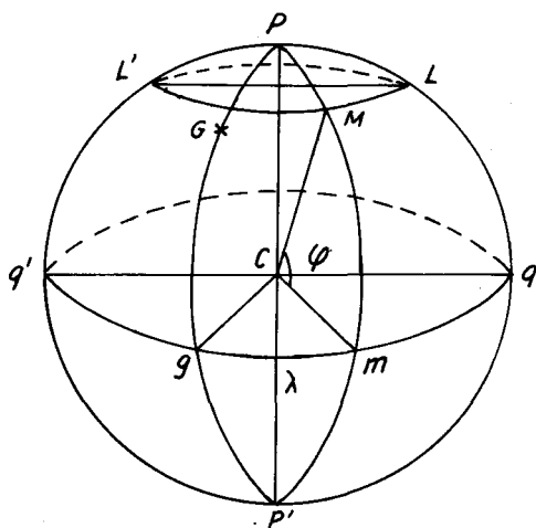
Hệ tọa độ địa lý.
