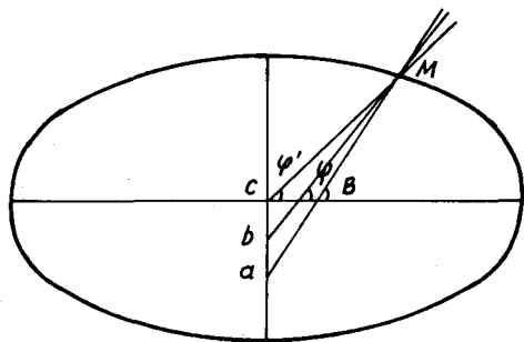
Elipsoit Trái Đất.
