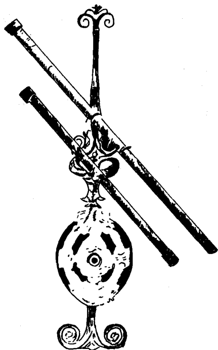
Kính thiên văn đầu tiên do Galilei chế tạo.
