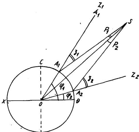
Hình 4. Thị sai ngày.
