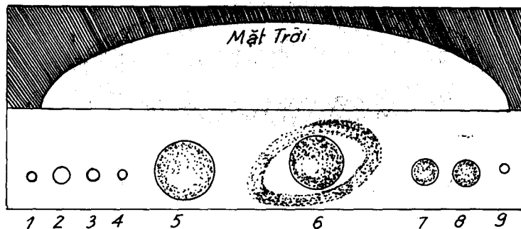
So sánh kích thước của Mặt Trời và các hành tinh : 1. Thủy Tinh ; 2. Kim Tinh ; 3. Trái Đất ; 4. Hỏa Tinh ; 5. Mộc Tinh ; 6. Thổ Tinh ; 7. Thiên Vương Tinh ; 8. Hải Vương Tinh ; 9. Diêm Vương Tinh.
