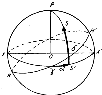
Hệ tọa độ xích đạo 2.
