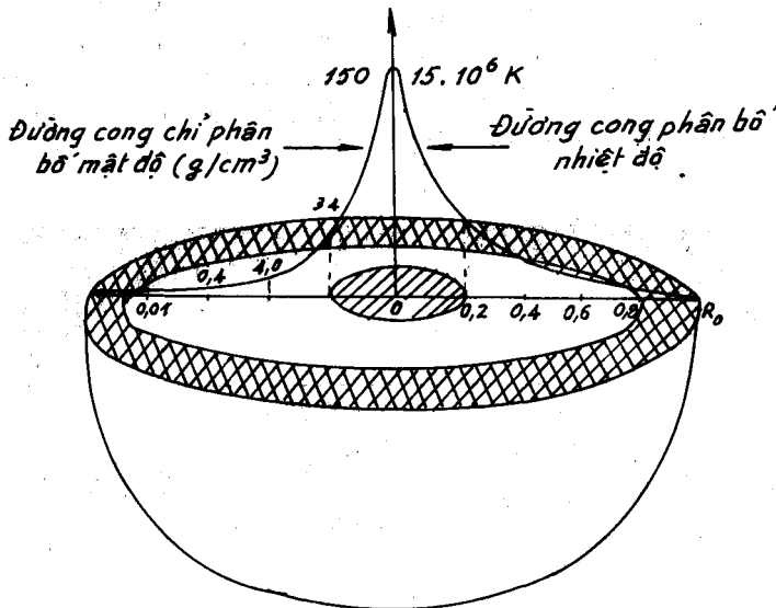
Cấu trúc, phân bố mật độ và nhiệt độ trong Mặt Trời.
