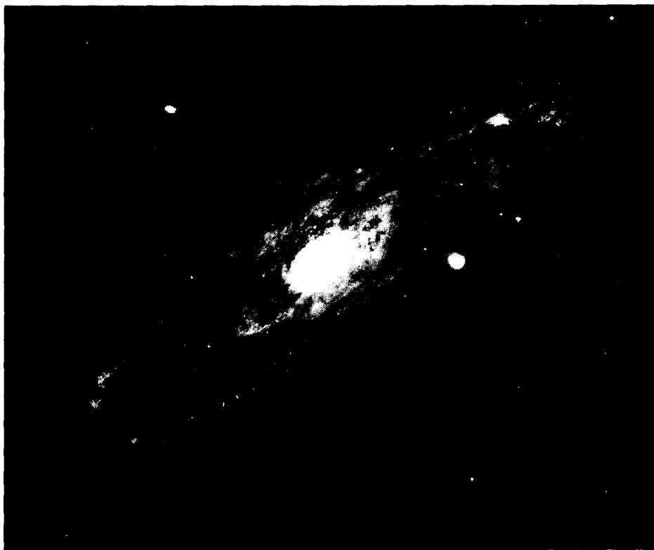
Thiên hà Tiên nữ M31
