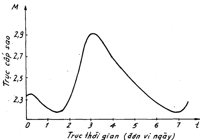
Đồ thị biến thiên độ sáng của sao co gián - \delta chòm Thiên Vương .
