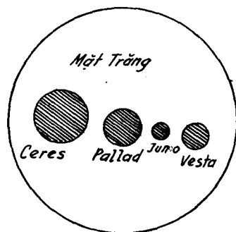
Kích thước các tiểu hành tinh lớn so với Mặt Trăng.
