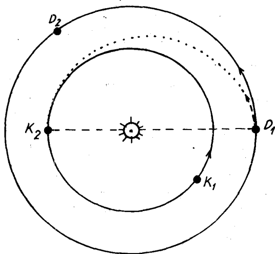
Elip chuyển tiếp từ Trái Đất D_1 đến Kim Tinh K_2 . D_1 và K_1 là vị trí của Trái Đất và Kim Tinh khi bắt đầu phóng tàu. D_2 và K_2 là vị trí của chúng khi con tàu tiến đến Kim Tinh. Đường đi theo lý thuyết là mất 142 ngày. ☼ là Mặt Trời.
