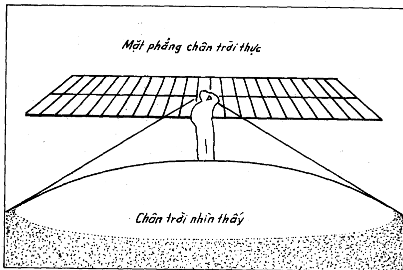
Chân trời thực và chân trời nhìn thấy.
