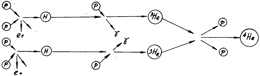
Chu trình proton - proton.
