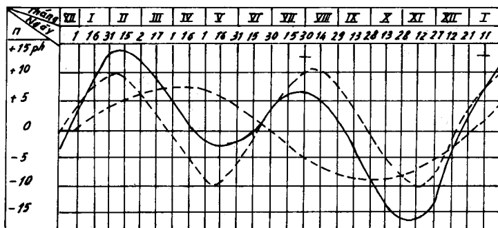
Đồ thị phương trình thời gian.
