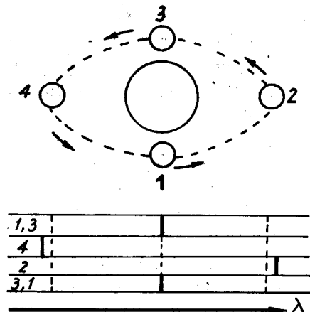
Hiệu ứng Doppler : Quỹ đạo một sao đôi quang phổ và sự dịch chuyển của vạch phổ do chuyển động của sao vệ tinh.
