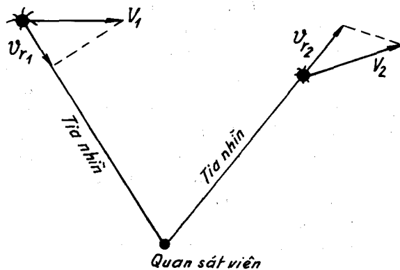
Vận tốc tia ( v_{r1} và v_{r2} ).
