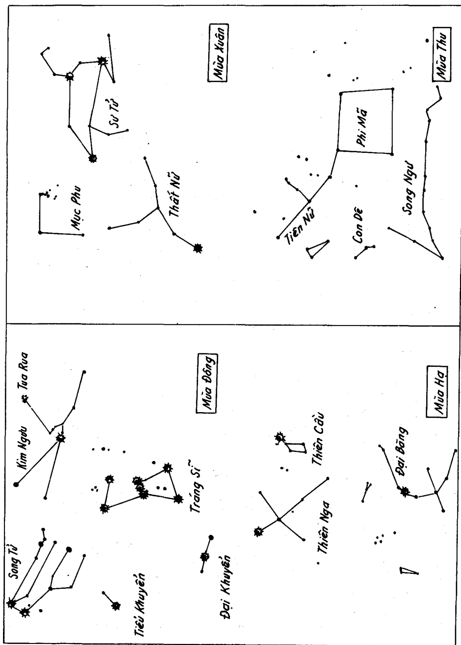
Những chòm sao chính nhìn thấy trong bốn mùa (ở Bắc bán cầu).
