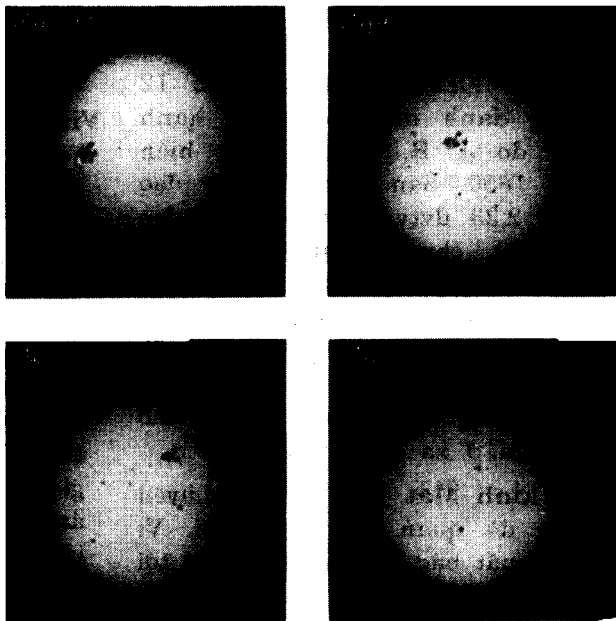
Vết đen Mặt Trời.
