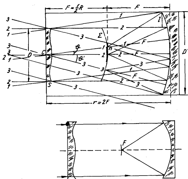
Hệ kính Schmidt.
