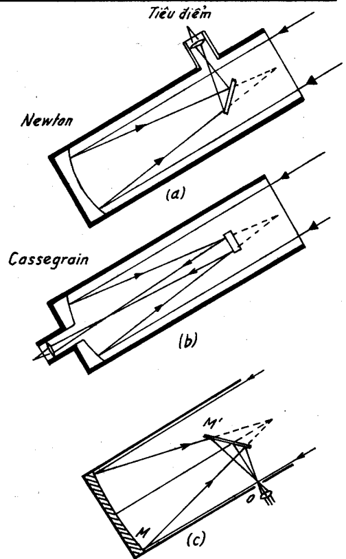
Hệ kính Newton.
