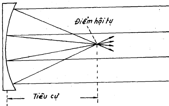
Hình 1. Kính thiên văn phản xạ.
