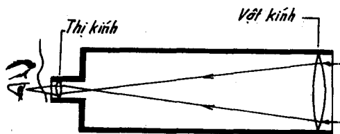
Hệ kính Galilei.
