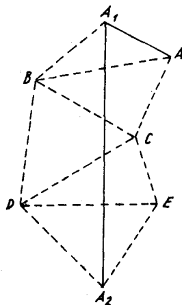
Sơ đồ tam giác đạc.
