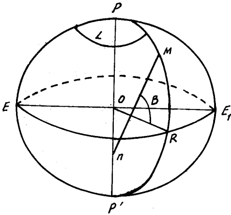
Hệ tọa độ trắc địa.
