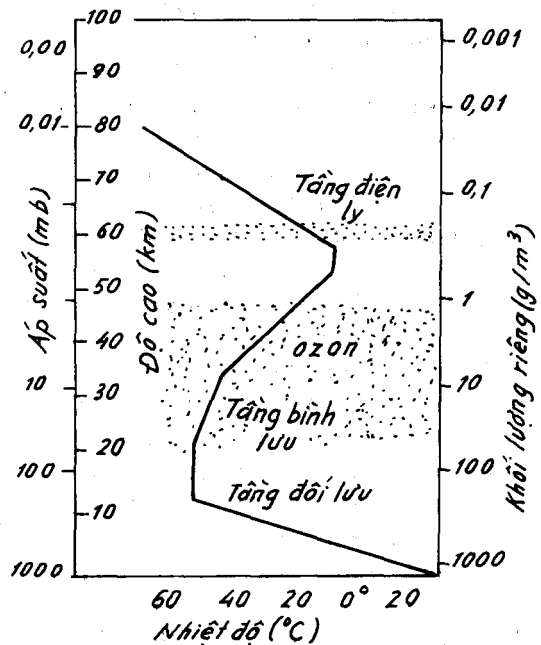
Cấu tạo của khí quyển.
