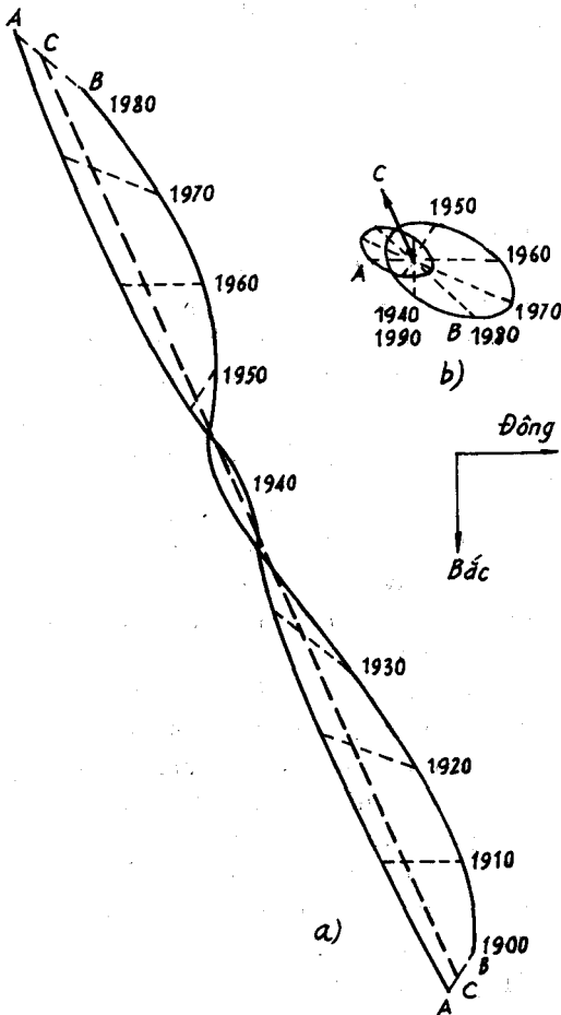
Sao đôi vật lý. a) Chuyển động của sao đôi Thiên Lang. Quỹ đạo của sao chính (A), của sao vệ tinh (B) và của khối tâm (C) đối với các sao lân cận. b) Quỹ đạo chuyển động của sao (A) và (B) quanh khối tâm chung (C).
