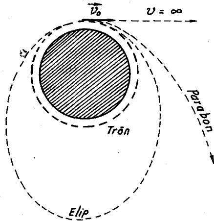
Các tốc độ vũ trụ.
