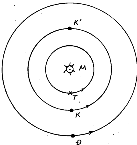
Vị trí Kim Tinh (K) và Thủy Tinh (T) giao hội trong với Mặt Trời (M). Vị trí Kim Tinh (K') giao hội trên với Mặt Trời (M).
