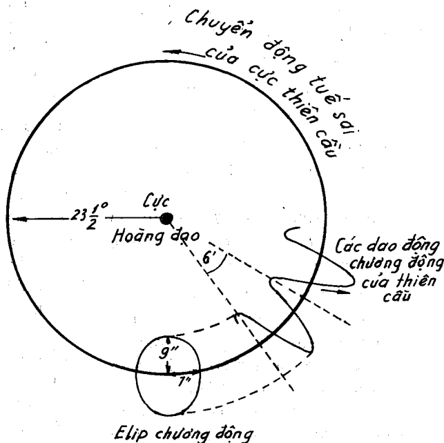
Hình 2. Chuyển động tuế sai của thiên cực.
