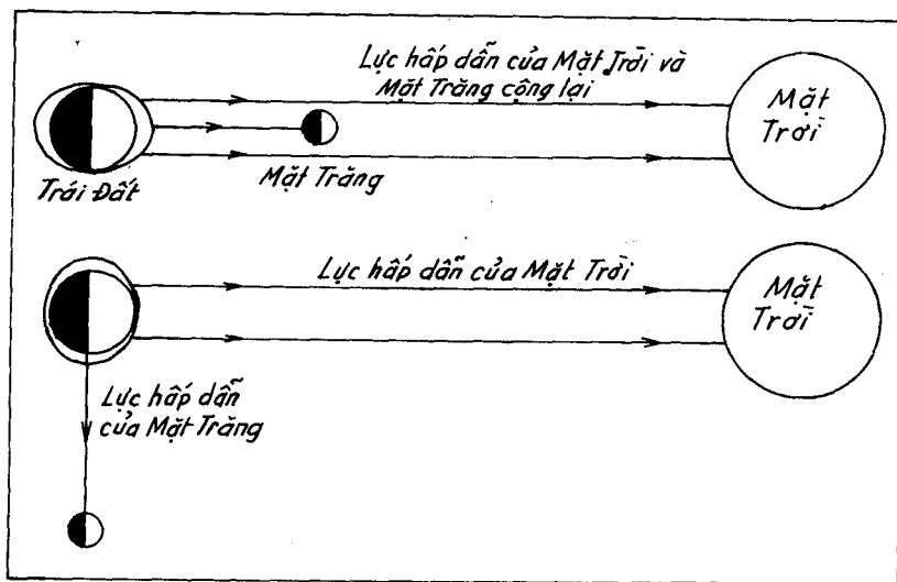
Triều cường (trên) và triều nhược (dưới).
