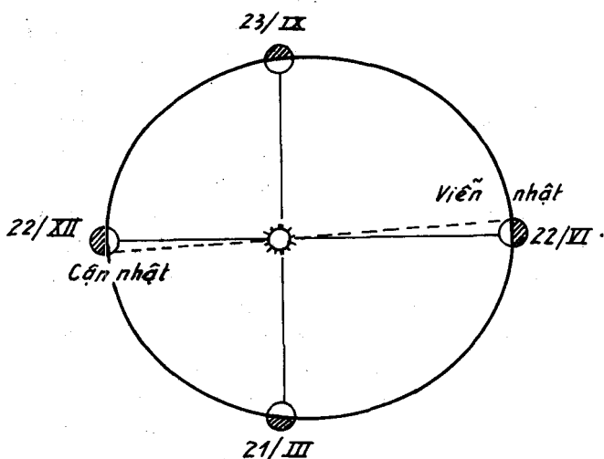
Trái Đất chuyển động xung quanh Mặt Trời theo quỹ đạo elip.
