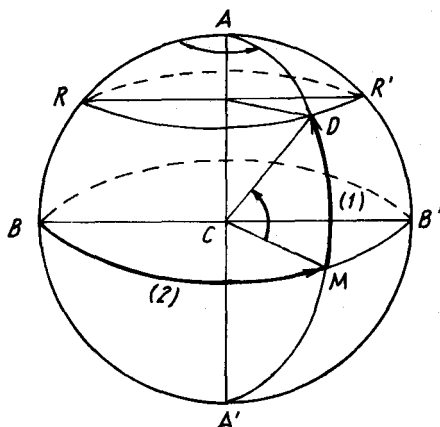
Hệ tọa độ mặt cầu.
