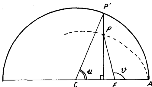
Góc cận điểm thực v , góc cận điểm tâm sai u .
