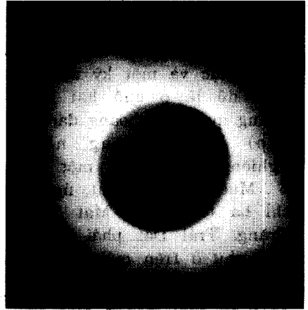
Nhật thực toàn phần ngày 24/10/1995, tại Phan Thiết (ảnh do Phan Văn Đồng và Nguyễn Phúc Giác Hải chụp).
