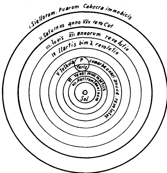
Hệ nhật tâm Copernic. Hình từ cuốn " De Revolutionibus Orbium Coelestium ", của ông xuất bản năm 1543.
