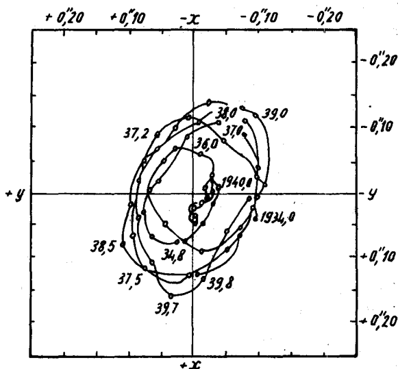
Sự di chuyển của cực tức thời từ năm 1934,0 đến năm 1940,0.
