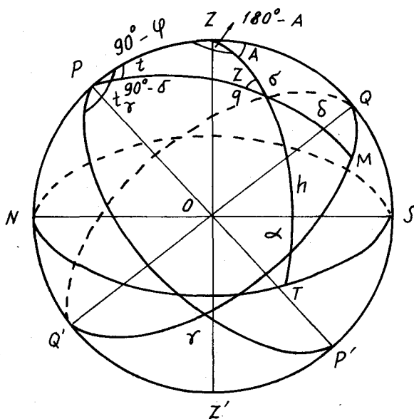
Cách vẽ tam giác định vị của thiên thể.
