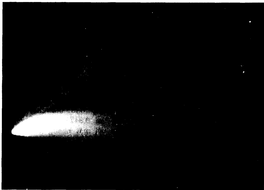
Sao chổi Hale - Bopp, ngày 12/3/1997.
