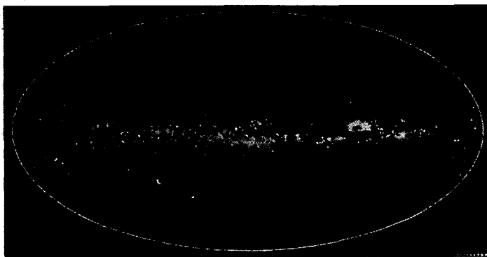
Dải Ngân Hà (ảnh của đài thiên văn Lund, Thụy Điển).
