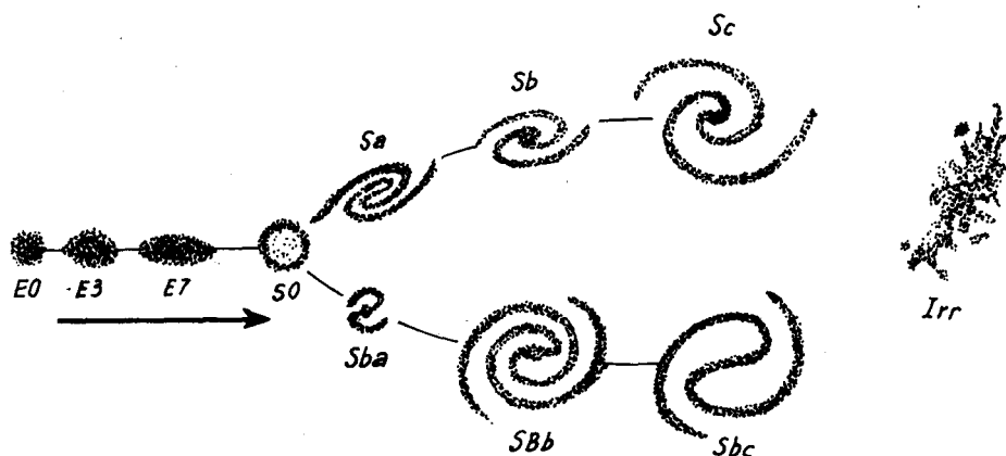
Họa đồ tiến hóa các thiên hà theo Hubble.
