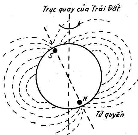
Từ quyển của Trái Đất.
