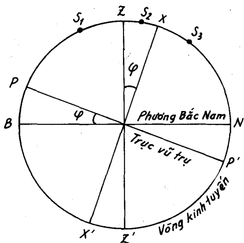
Sự qua kinh tuyến trên.
