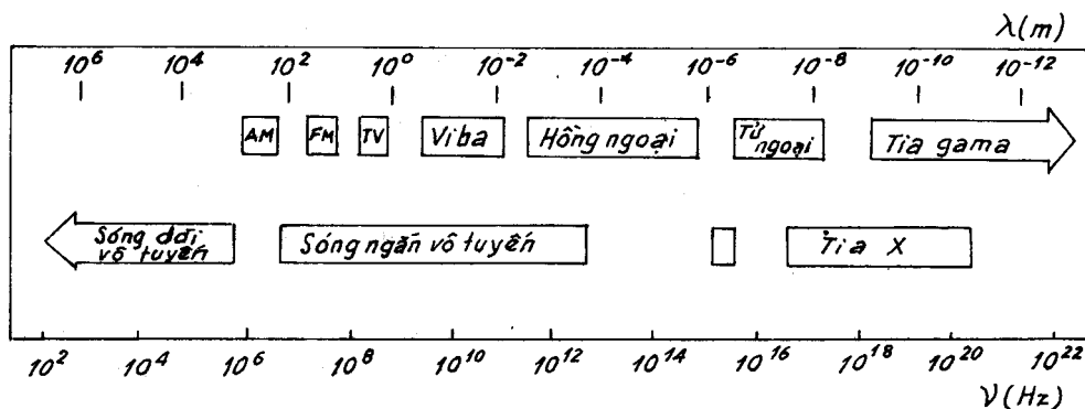
Sơ đồ phổ điện từ.
