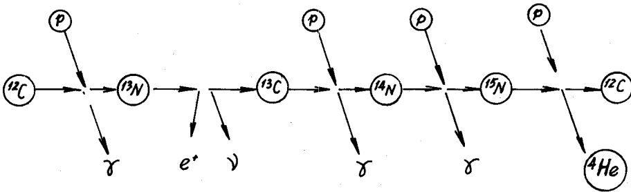
Chu trình cacbon.
