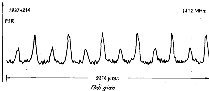
Pulsar : Xung sóng vô tuyến tần số 1412 MHz của pulsar PSR 1937 + 214.
