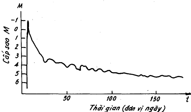
Đồ thị biến thiên độ sáng (cấp sao tuyệt đối M ) của sao mới V1500 Thiên Nga 1975 trong 150 ngày kể từ khi bùng sáng.
