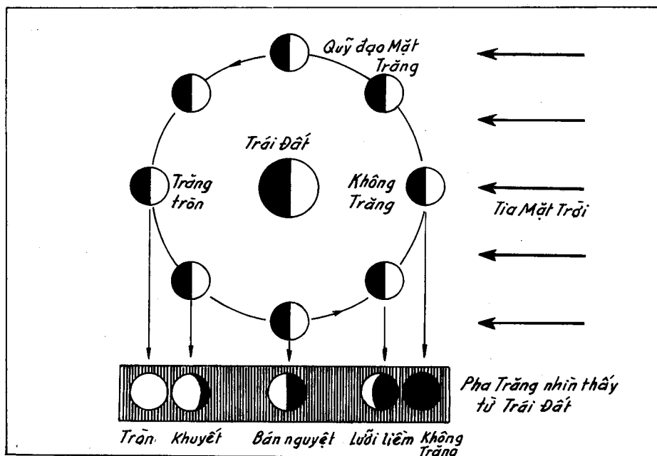
Các pha trăng nhìn thấy từ Trái Đất.
