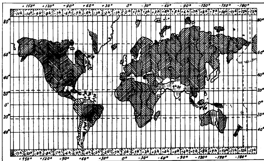
Ranh giới của 24 múi giờ.
