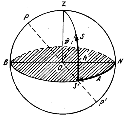
Hệ tọa độ chân trời.
