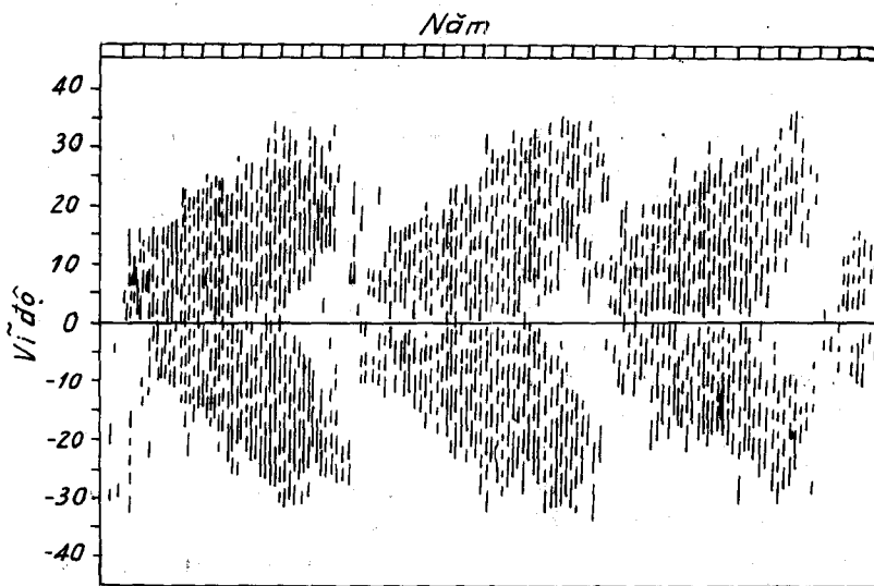
Họa đồ hình bướm.
