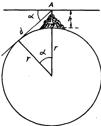
Một trong các phương pháp xác định kích thước của Trái Đất.
