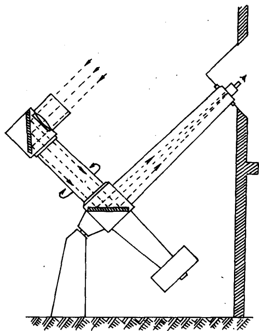
Kính phản xạ Coudé.
