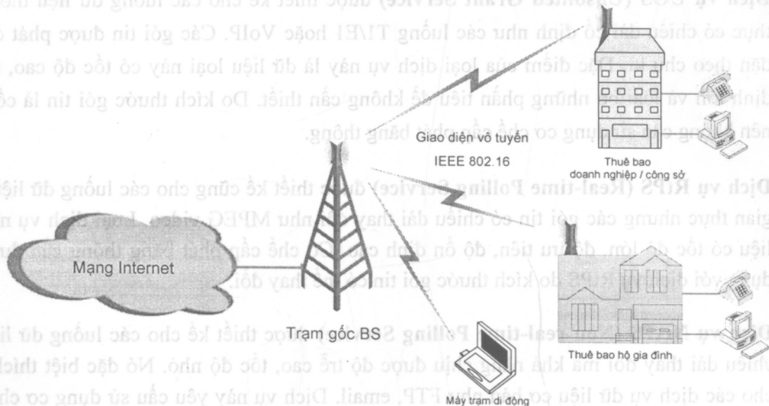
Hình 4.21. Ứng dụng WiMAX cho mạng truy nhập.
