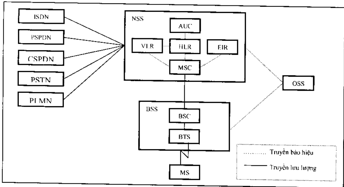
Hình 2.2. Các thành phần của mạng GSM.
