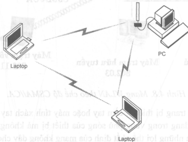
Hình 4.7. Mạng WLAN cấu hình theo chế độ độc lập (tùy biến) – Ad-hoc mode.
