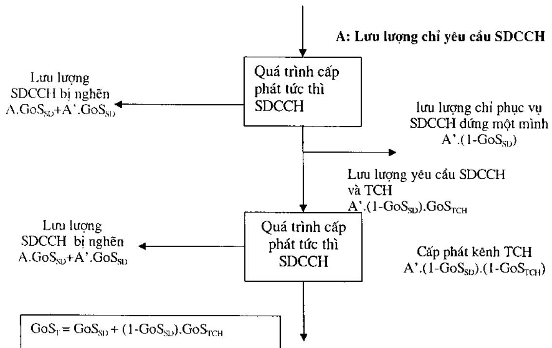
Hình 2.28. Sơ đồ thiết lập cuộc thoại.
