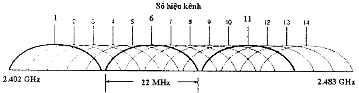
Hình 4.11. Cấp phát kênh theo chuẩn 802.11b/g
