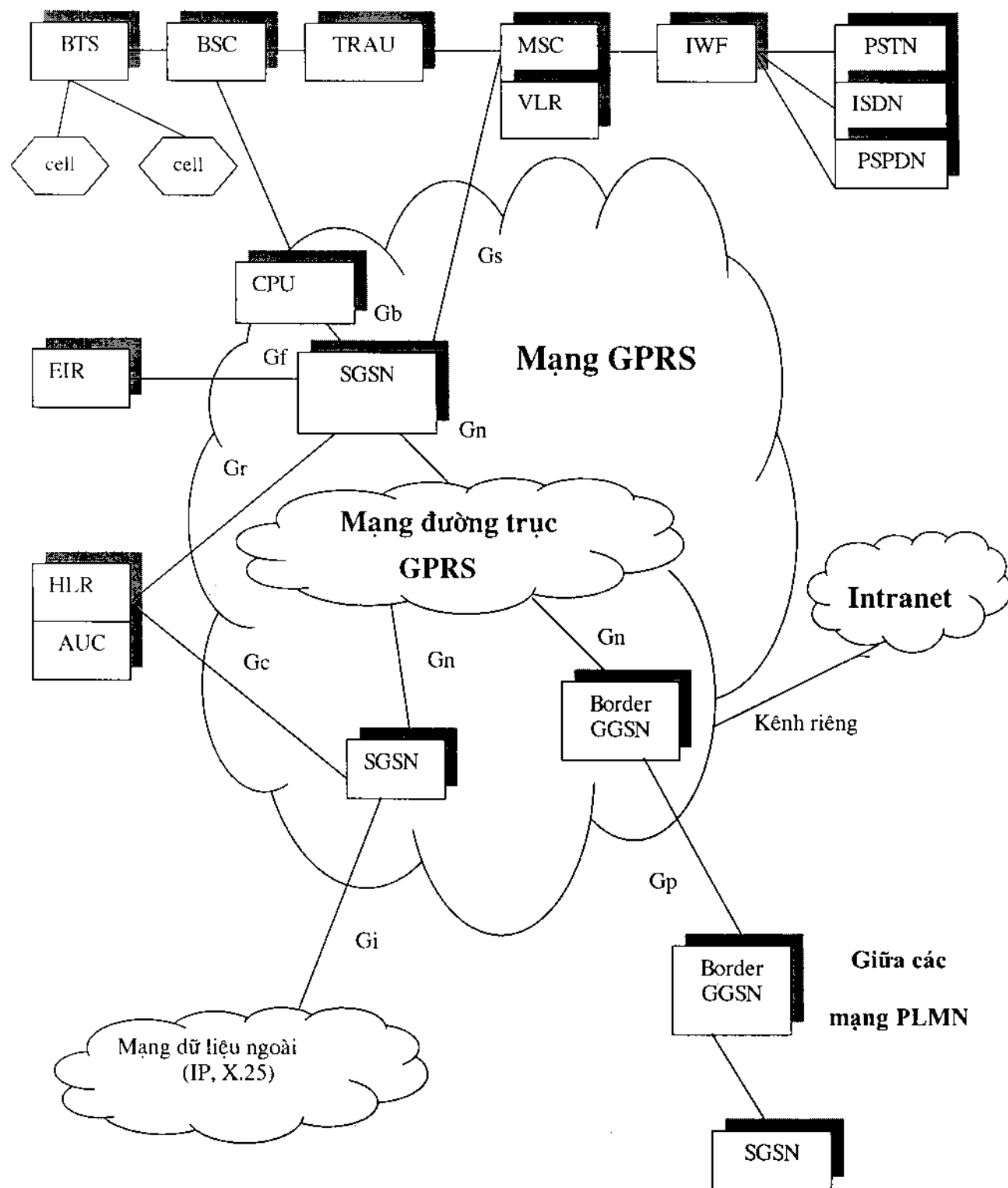
Hình 2.30. Các thành phần chính trong hệ thống GPRS
