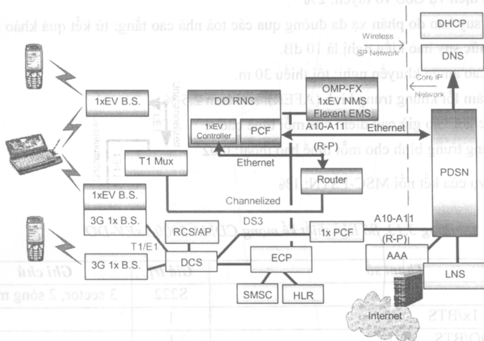
Hình 3.23. Giải pháp mạng kết hợp 1x và EV-DO của Lucent.
