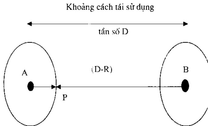
Hình 2.20. Sơ đồ tính C/I.
