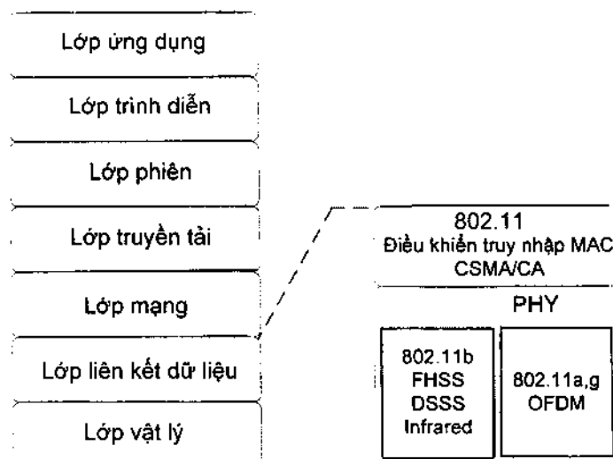
Hình 4.10. Mô hình giao thức IEEE 802.11
