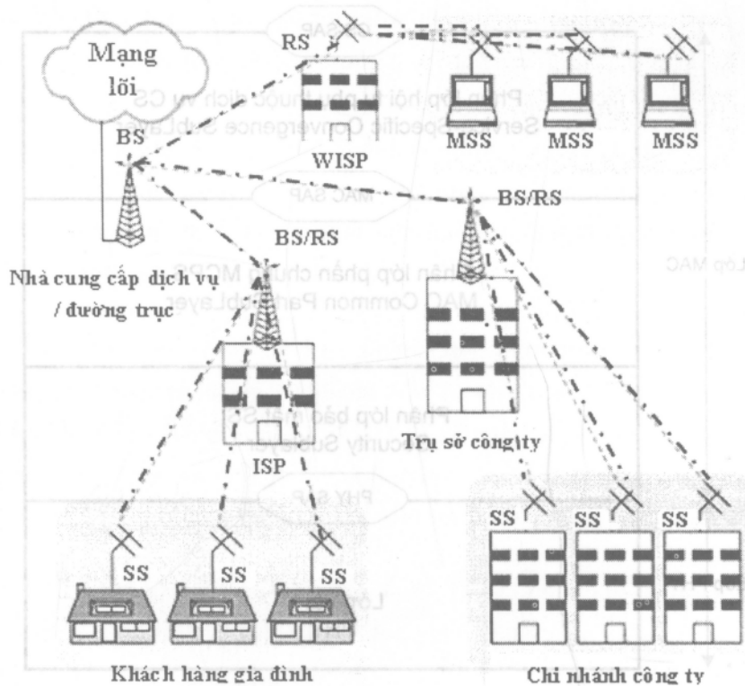
Hình 4.18. Cấu hình mạng WiMAX.
