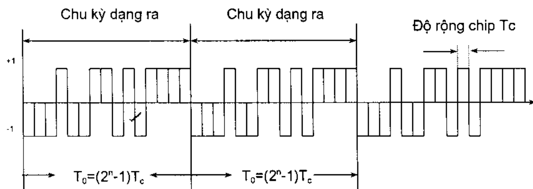
Hình 3.8. Dạng ra của bộ 4 tầng có hồi tiếp tuyến tính.
