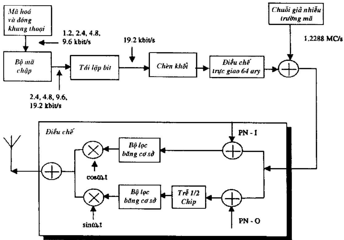
Hình 1.7. Điều chế tài thông chiều đi của cdmaOne.
