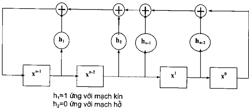
Hình 3.9. Bộ thanh ghi dịch hồi tiếp tuyến tính n tầng.
