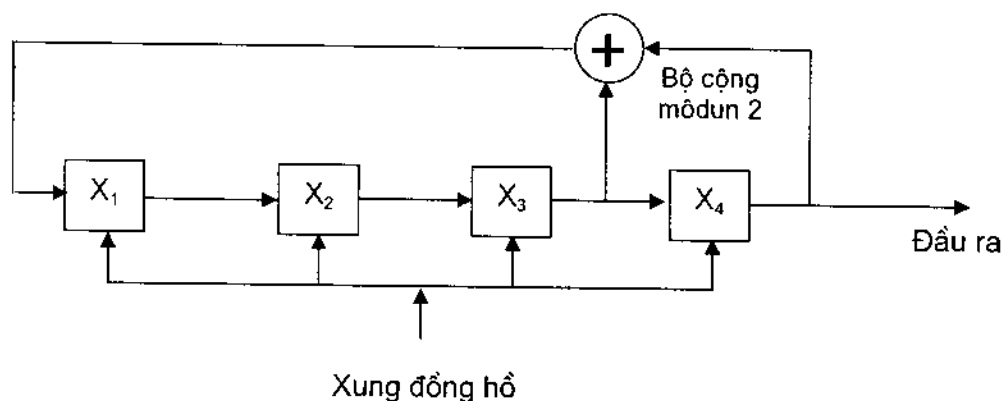
Hình 3.7. Bộ 4 thanh ghi có hồi tiếp tuyến tính.
