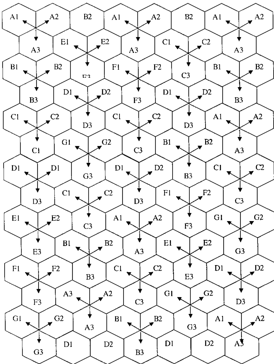
Hình 2.23. Mẫu tái sử dụng tần số 7/21.
