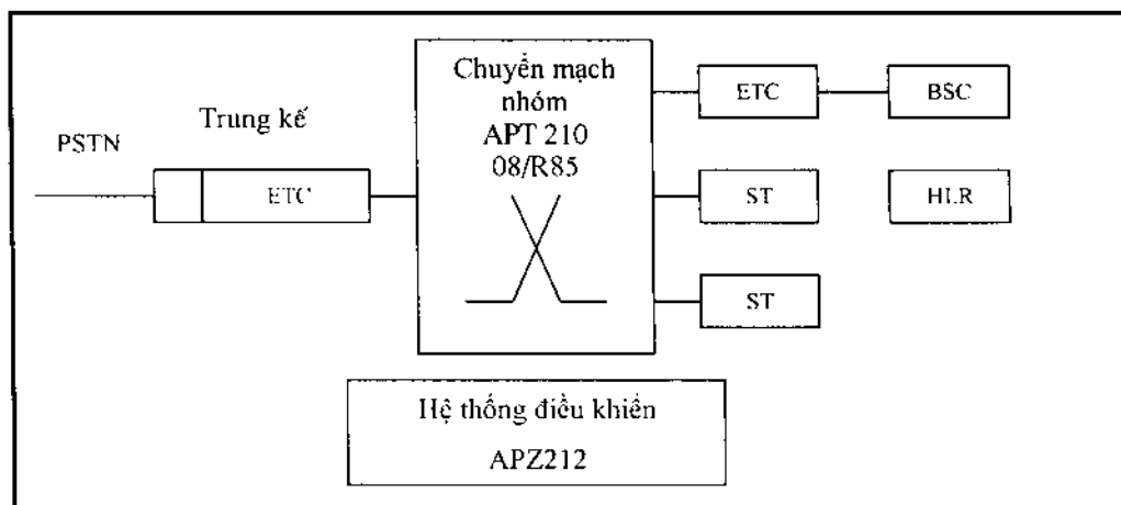
Hình 2.3. Cấu trúc của MSC/VLR
