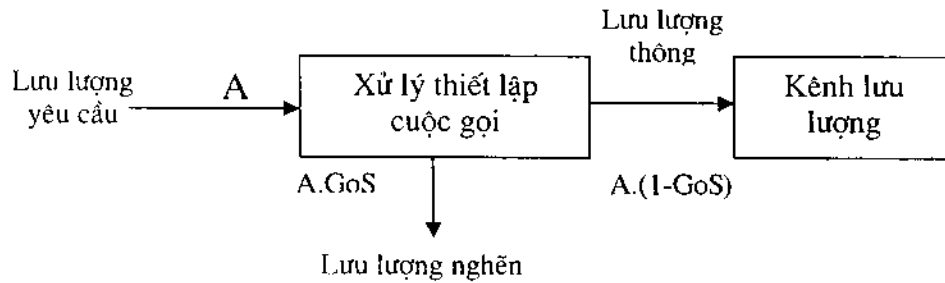
Hình 2.27. Sơ đồ lưu lượng.
