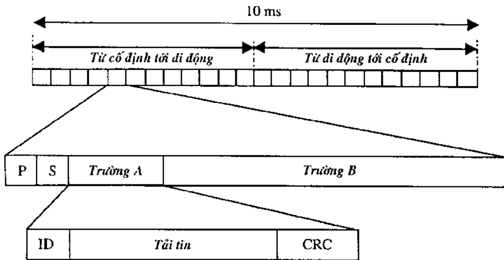
Hình 1.11. Cấu trúc khung DECT.
