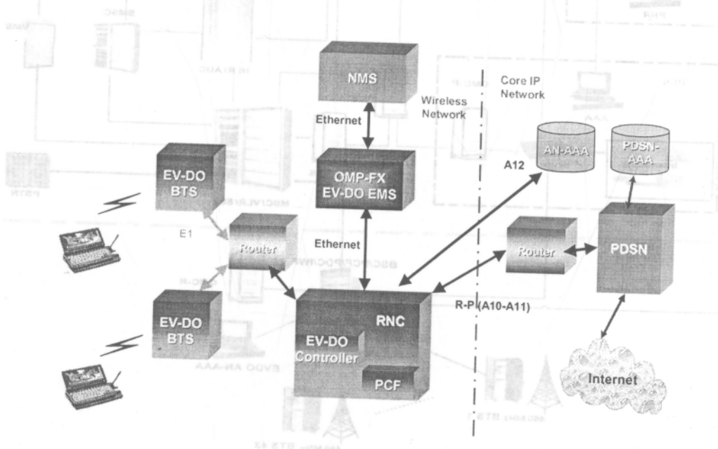
Hình 3.22. Giải pháp mạng 1xEV-DO độc lập của Lucent.
