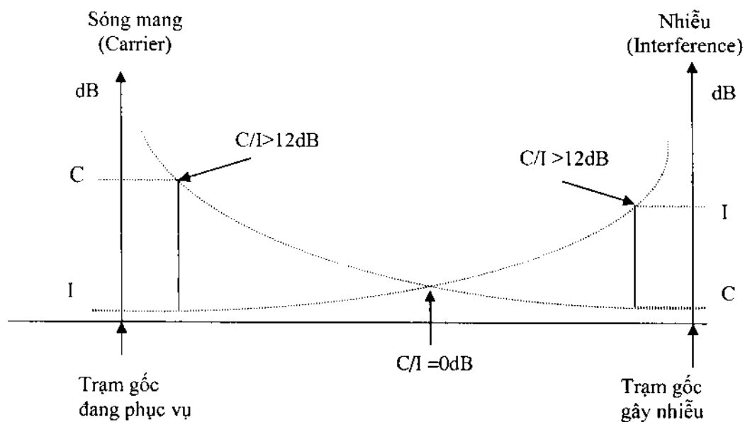
Hình 2.18. Tỷ số C/L.
