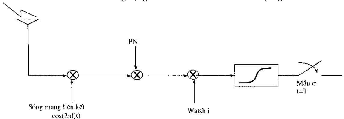
Hình 3.11. Ứng dụng của hàm Walsh và mã bù ở trạm gốc.
