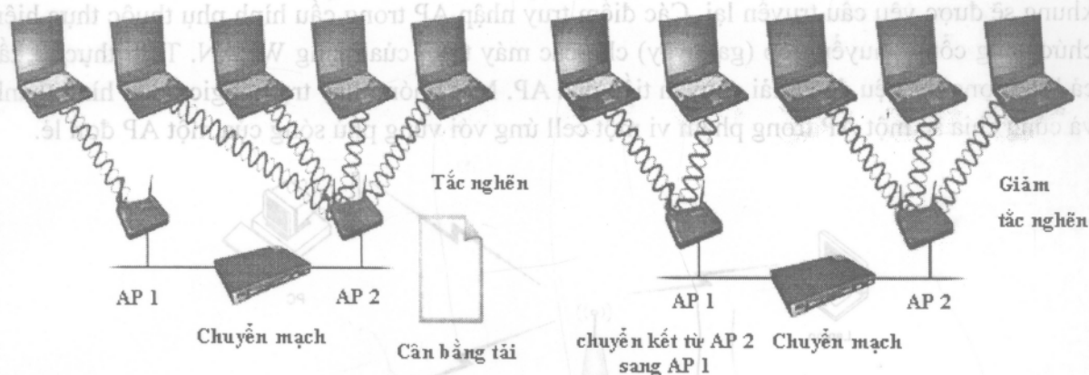
Hình 4.4. Thực hiện cân bằng tải tại AP.
