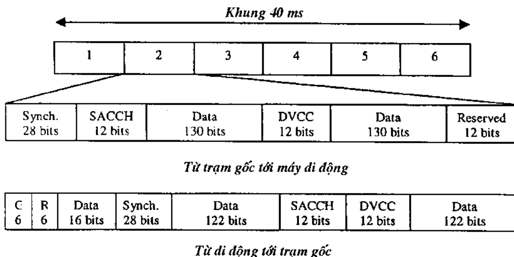
Hình 1.6. Cấu trúc khe thời gian D-AMPS.
