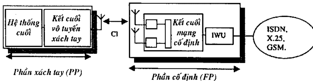
Hình 1.12. Cấu trúc mạng DECT.
