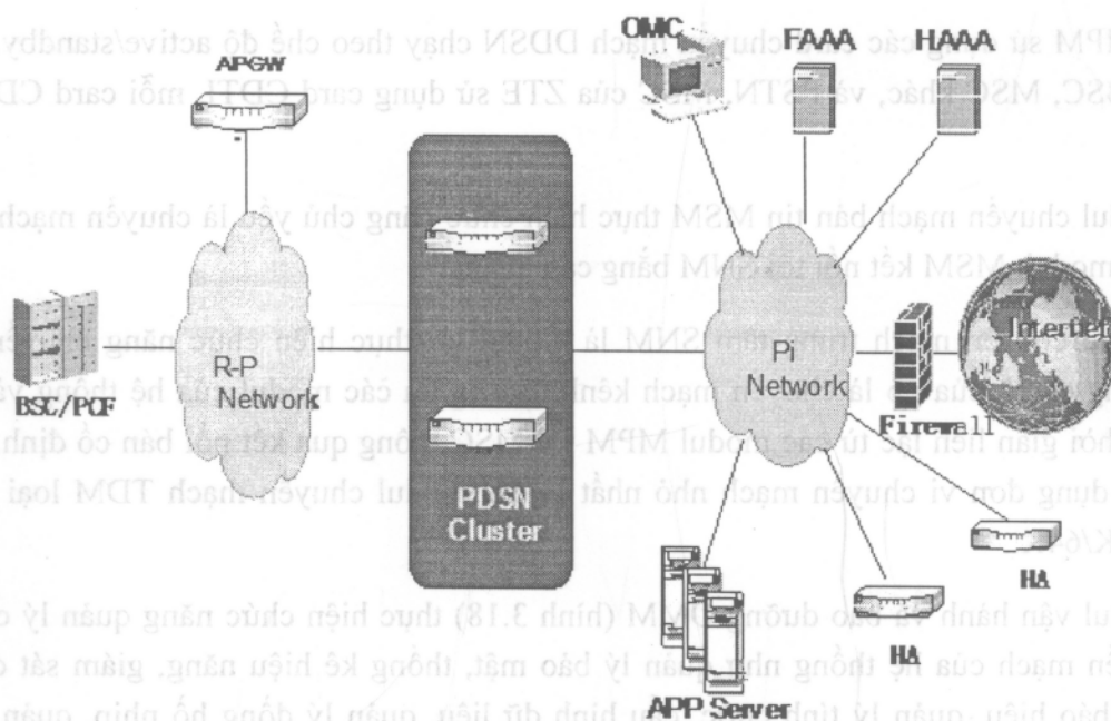
Hình 3.19. Giải pháp dữ liệu gói cho CDMA 2000 1xEV-DO của ZTE.
