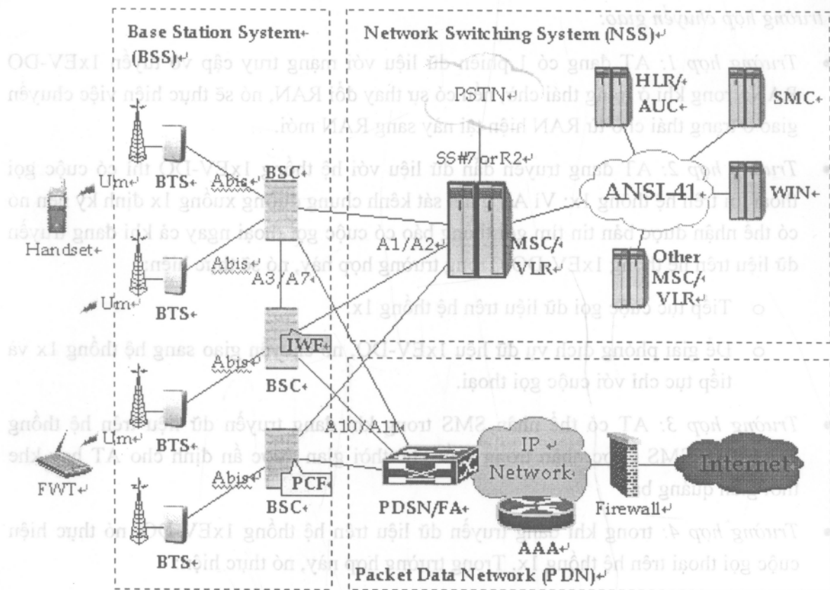
Hình 3.15. Kiến trúc mạng CDMA 2000 1xEV-DO của ZTE.
