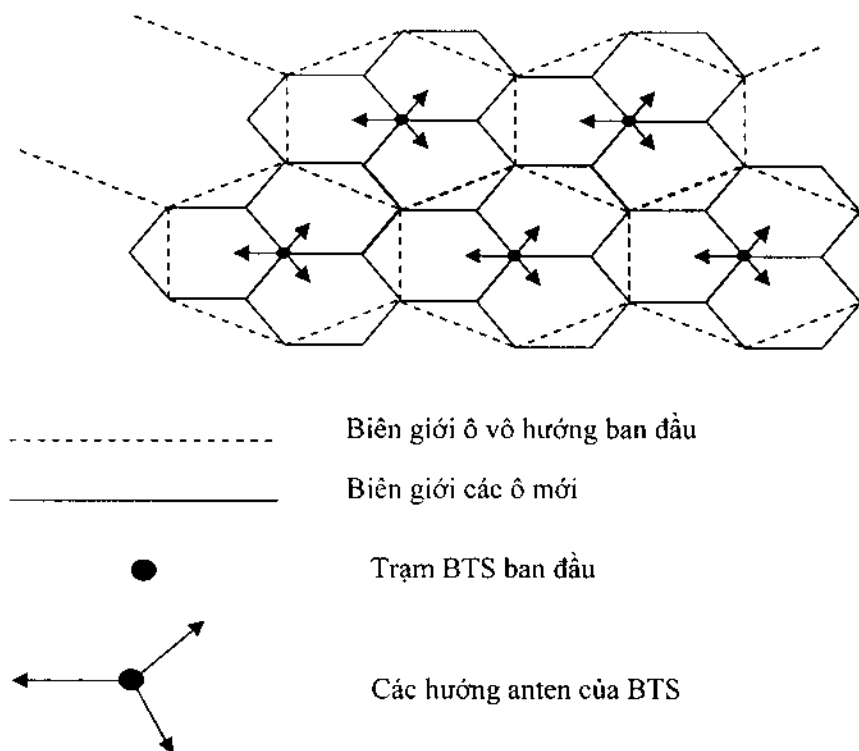
Hình 2.25. Chia cell giai đoạn 1.
