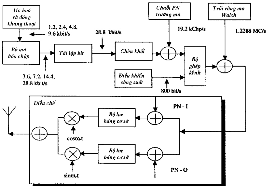
Hình 1.8. Điều chế tải thông hướng về của cdmaOne.
