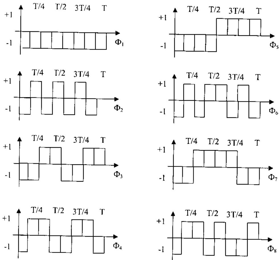
Hình 3.13. Các báo hiệu của các hàm Walsh.
