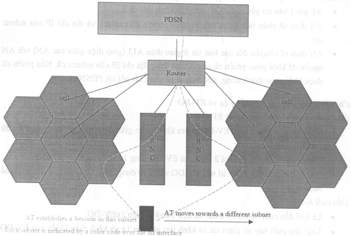
Hình 3.14. Minh họa quá trình chuyển giao ở trạng thái chờ.
