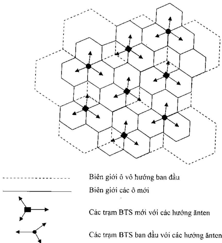
Hình 2.26. Chia cell giai đoạn 2 (1:4).
