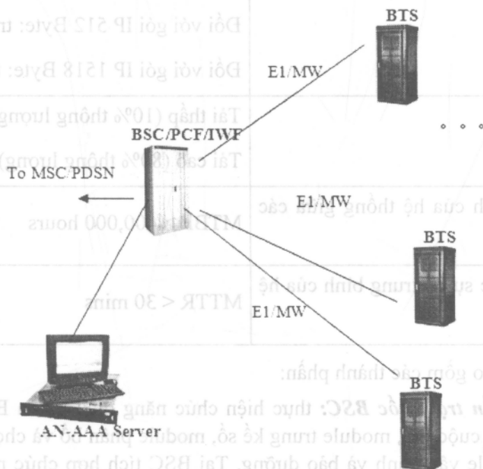
Hình 3.20. Giải pháp mạng truy cập CDMA 2000 1xEV-DO của ZTE.
