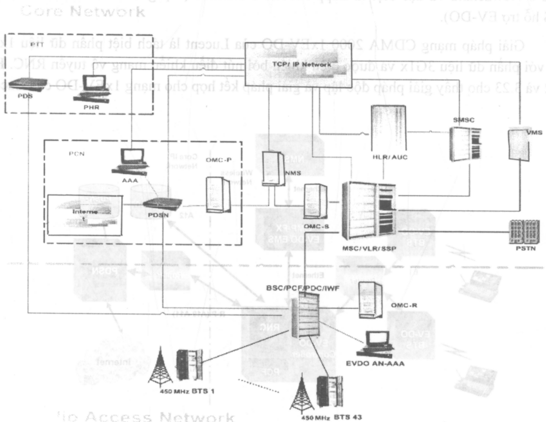
Hình 3.21. Sơ đồ mạng CDMA 2000 1xEV-DO.
