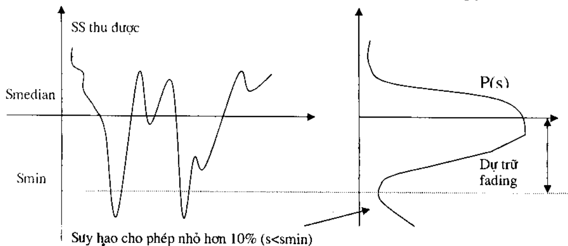
Hình 2.13. Dự trữ fading chậm.
