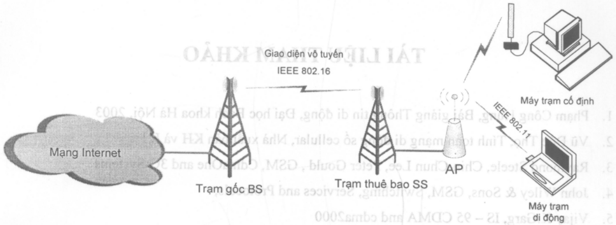
Hình 4.23. Ứng dụng WiMAX kết hợp với Wi-Fi.
