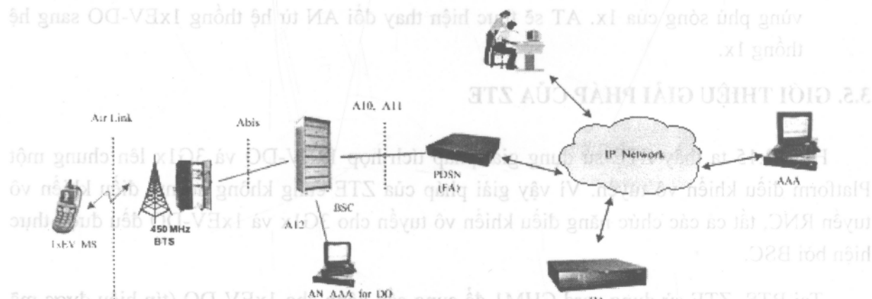
Hình 3.16. Lưu lượng EV-DO và 1x tới BSC, PDSN cùng 1 đường.
