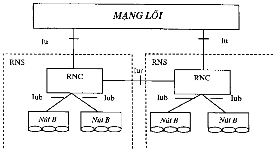
Hình 1.17. Cấu trúc mạng UTRAN.
