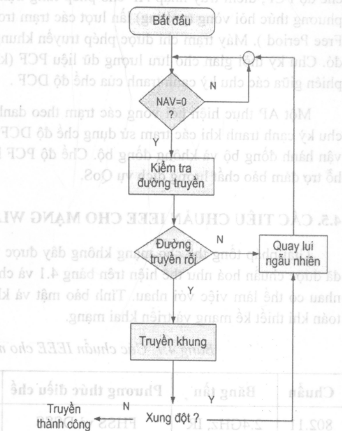
Hình 4.9. Nguyên tắc hoạt động theo chế độ DCF
