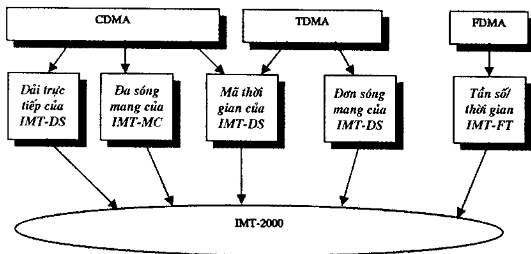
Hình 1.13. Họ các hệ thống sóng radio của IMT-2000.
