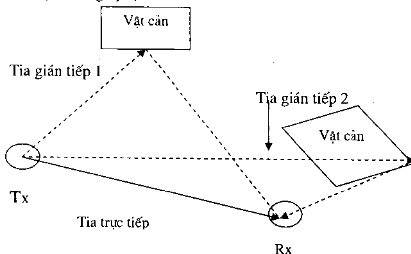
Hình 2.14. Truyền sóng tới nhiều tia, nguyên nhân gây phân tán thời gian.
