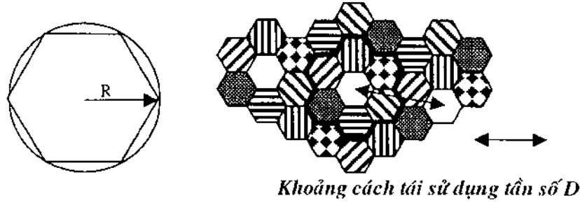
Hình 1.1. Mẫu 7 tế bào sử dụng lặp tần.
