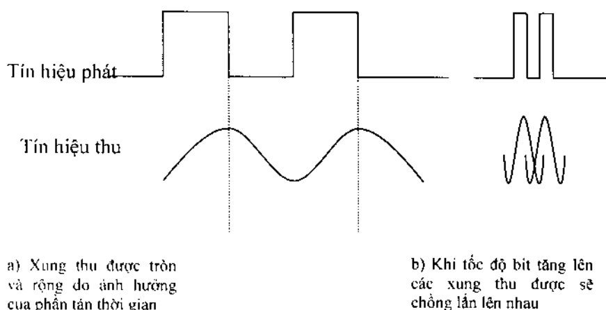
Hình 2.16. Nhiễu giữa các ký tự.
