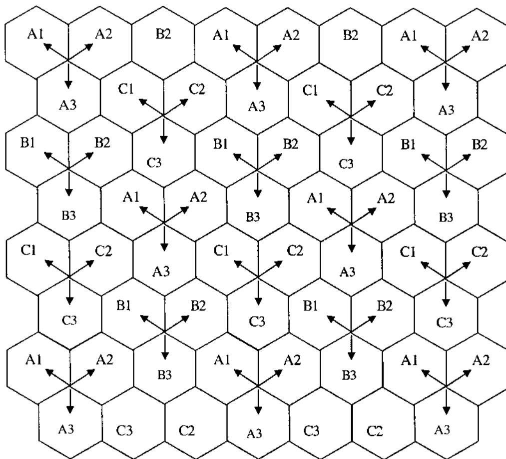
Hình2.21. Mẫu tái sử dụng tần số 3/9.
