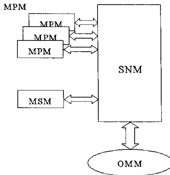
Hình 3.17. Kiến trúc phần cứng của MSC/VLR.
