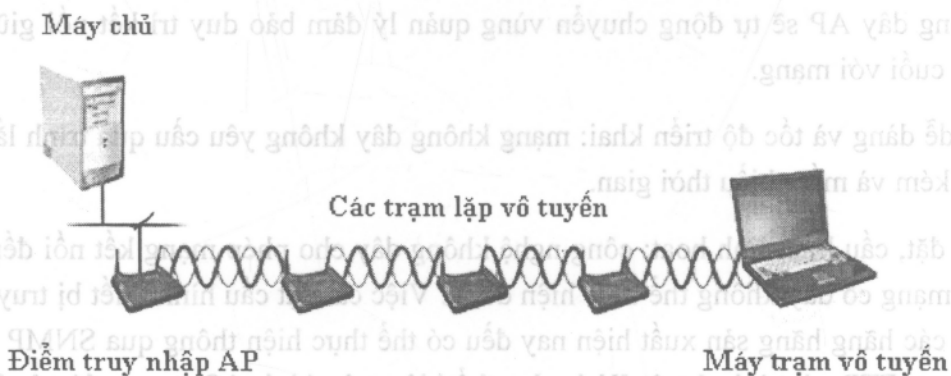
Hình 4.3. Cấu hình điểm truy nhập AP thực hiện chức năng chuyển tiếp.
