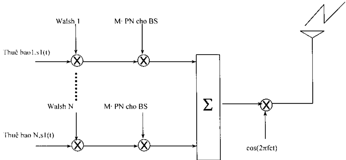
Hình 3.11. Ứng dụng của hàm Walsh và mã bù ở trạm gốc.
