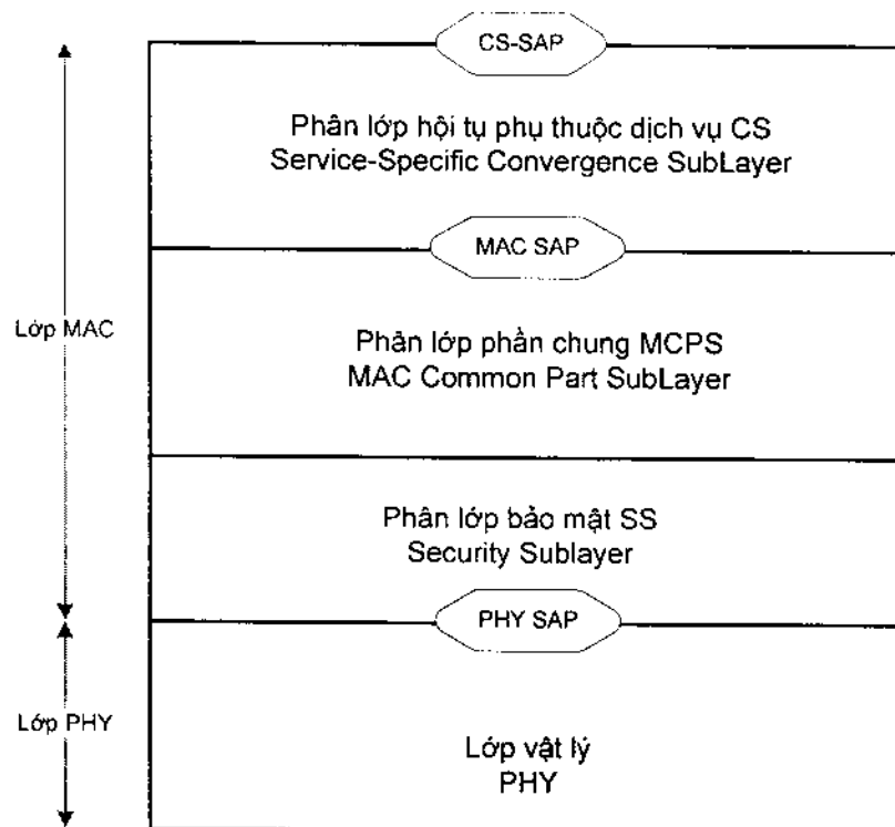
Hình 4.19. Mô hình cấu trúc giao thức của IEEE 802.16.
