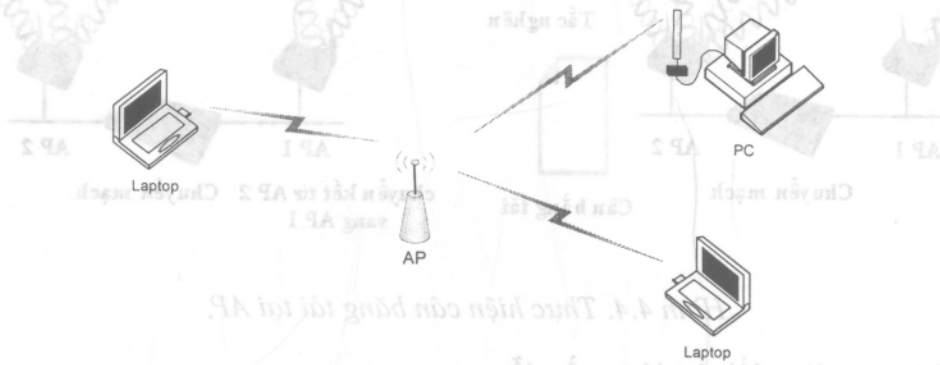
Hình 4.5. Mạng WLAN cấu hình theo chế độ phụ thuộc - infrastructure mode.
