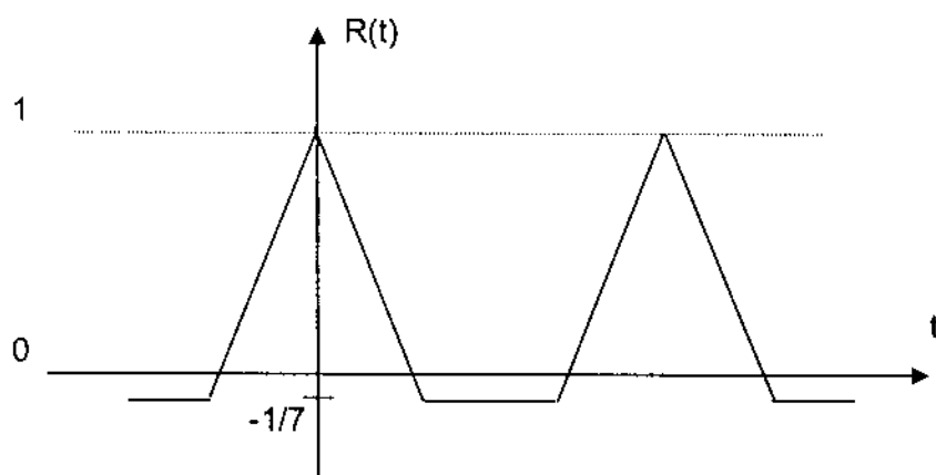
Hình 3.10. Hàm tự tương quan của bộ gồm ba tầng và các đường hồi tiếp tuyến tính.
