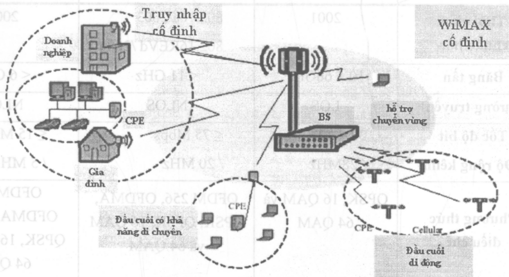
Hình 4.17. Các hướng ứng dụng được chuẩn hóa bởi WiMAX.
