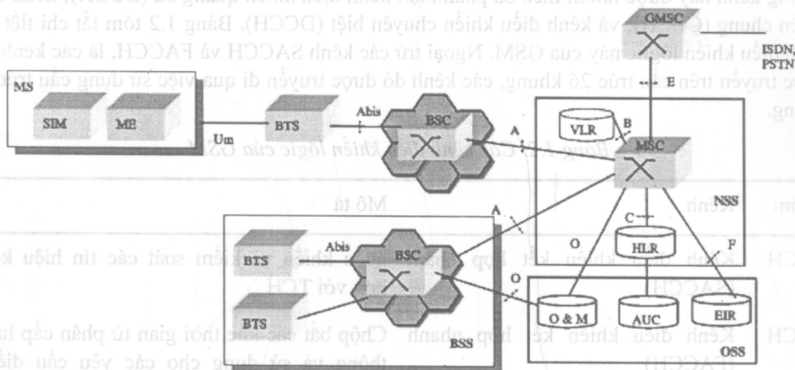
Hình 1.5. Cấu trúc mạng đơn giản hoá của GSM.
