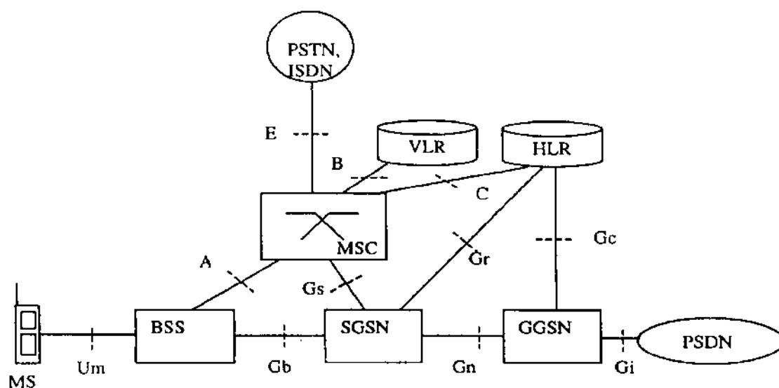
Hình 1.9. Cấu trúc mạng dịch vụ vô tuyến gói chung GPRS.
