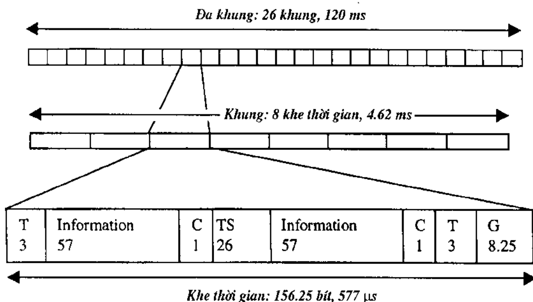
Hình 1.3. Cấu trúc 26 khung TDMA của GSM.
