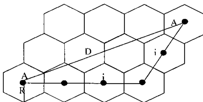
Hình 2.19. Khoảng cách tái sử dụng tần số.
