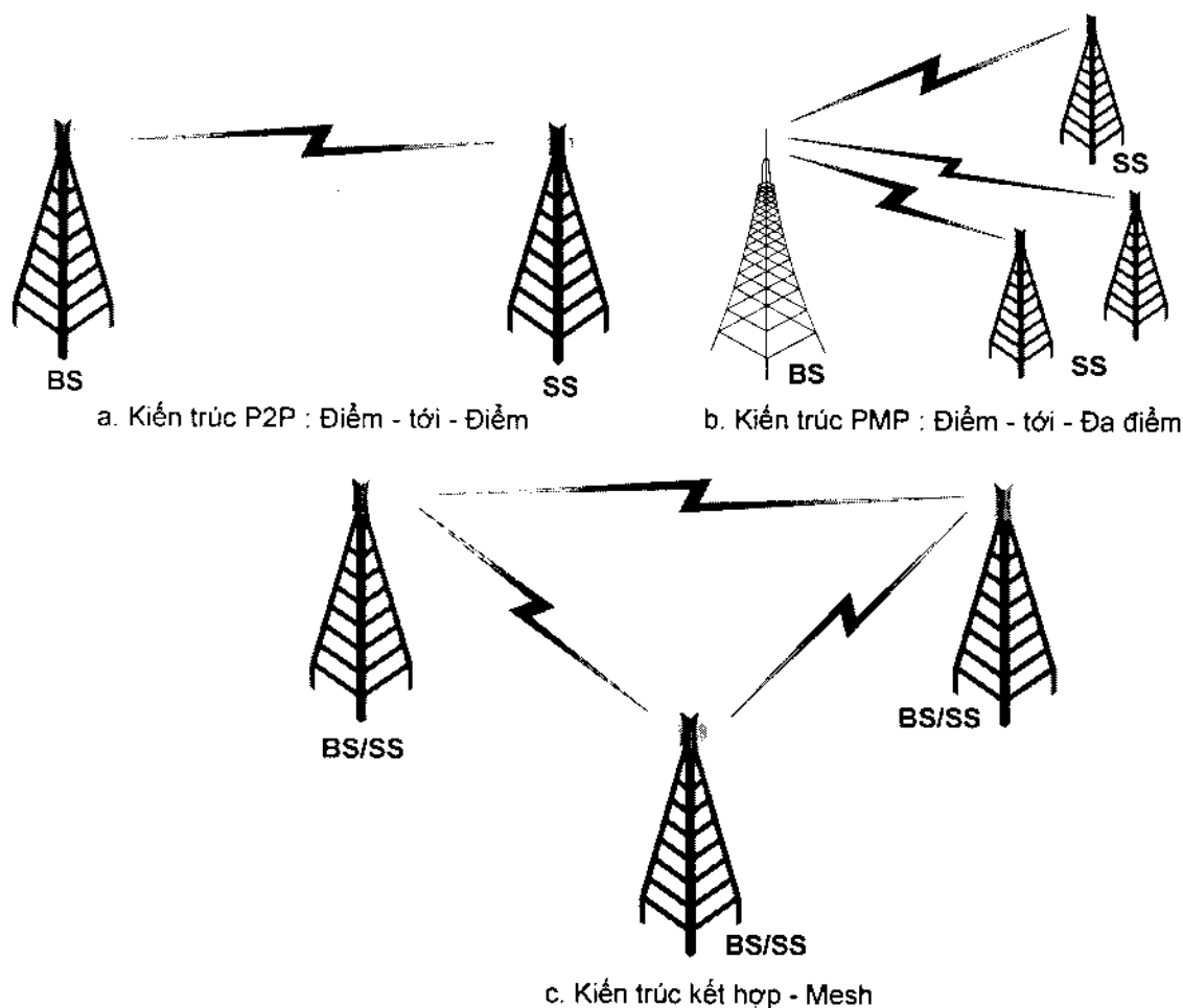
Hình 4.20. Các mô hình kiến trúc kết nối BS và SS.
