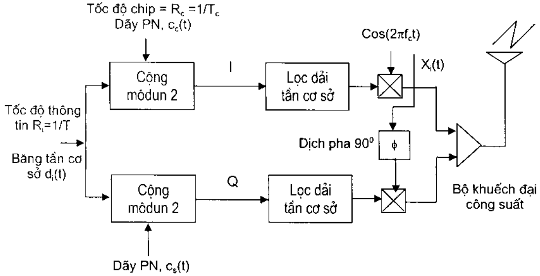
Hình 3.4. Hệ thống DSSS với máy phát QPSK.
