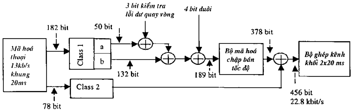
Hình 1.4. Bộ mã âm thoại toàn tốc của GSM.
