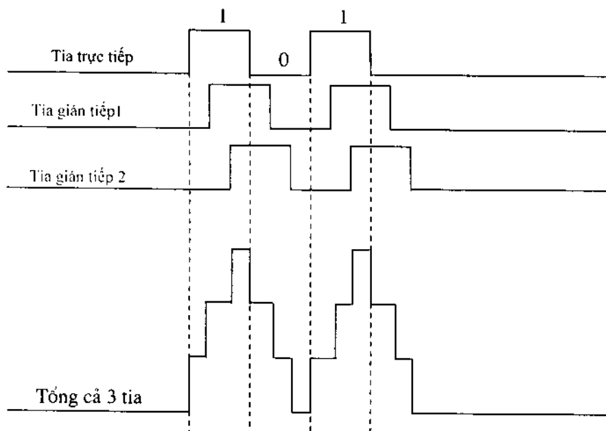
Hình 2.14. Truyền sóng tới nhiều tia, nguyên nhân gây phân tán thời gian.
