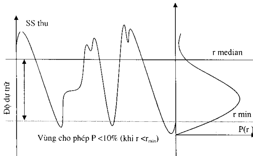
Hình 2.12. Dự trữ fading chậm.
