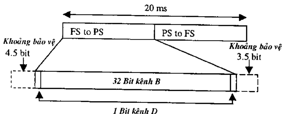
Hình 1.10. Cấu trúc khung của CT-2.
