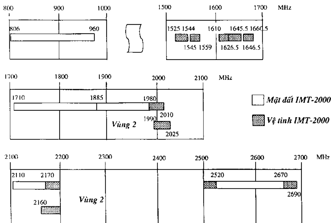
Hình 1.14. Phân phối quang phổ của IMT-2000.
