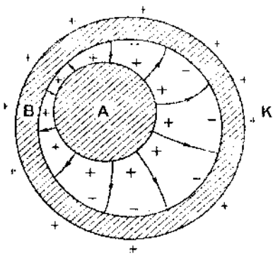
Hình 2.4. Điện hưởng toàn phần
