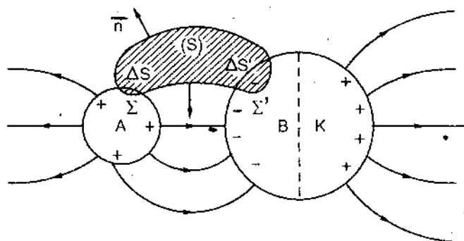
Hình 2.3. Hiện tượng điện hướng
