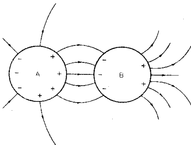
Hình 2.5. Hệ vật dẫn tích điện cân bằng
