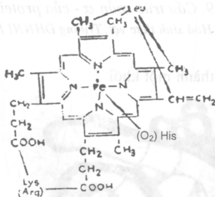
Hình 12. Cấu tạo của phân tử hemôglôbin
