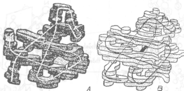
Hình 11. Cấu trúc bậc bốn của phân tử hemôglôbin
