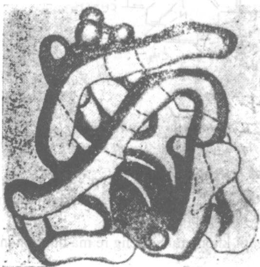
Hình 10. Cấu trúc bậc ba của phân tử miôglôbin
