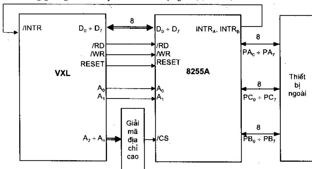
Hình 5.8. Phối ghép 8086 với 8255A
