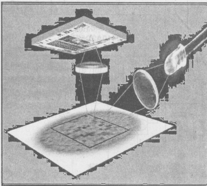
Hình 7.5. Hệ thống quang trong chuột quang
