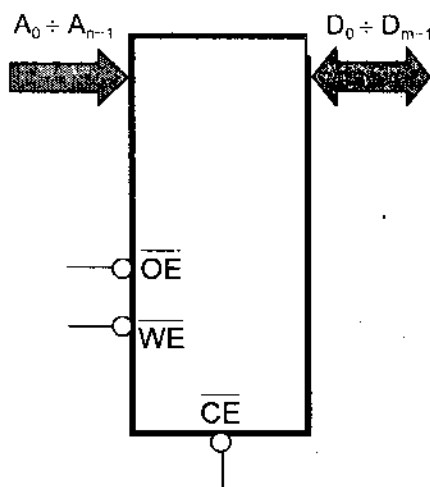
Hình 4.9. Sơ đồ cấu trúc chung của mạch nhớ RAM
