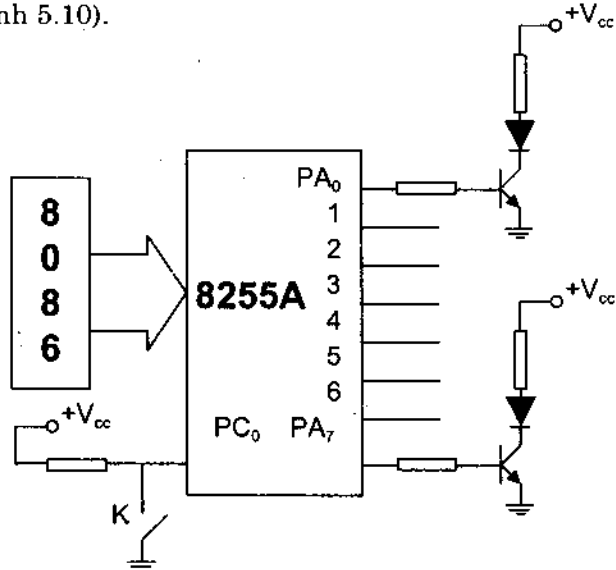
Hình 5.10. 8255A điều khiển các LED tắt/mở theo khoá K
