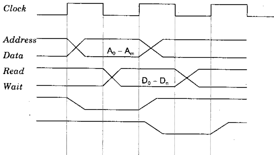
Hình 4.18. Minh họa một chu trình BUS đơn giản
