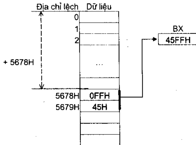
Hình 3.3. Mô tả lệnh MOV BX,[5678H]
