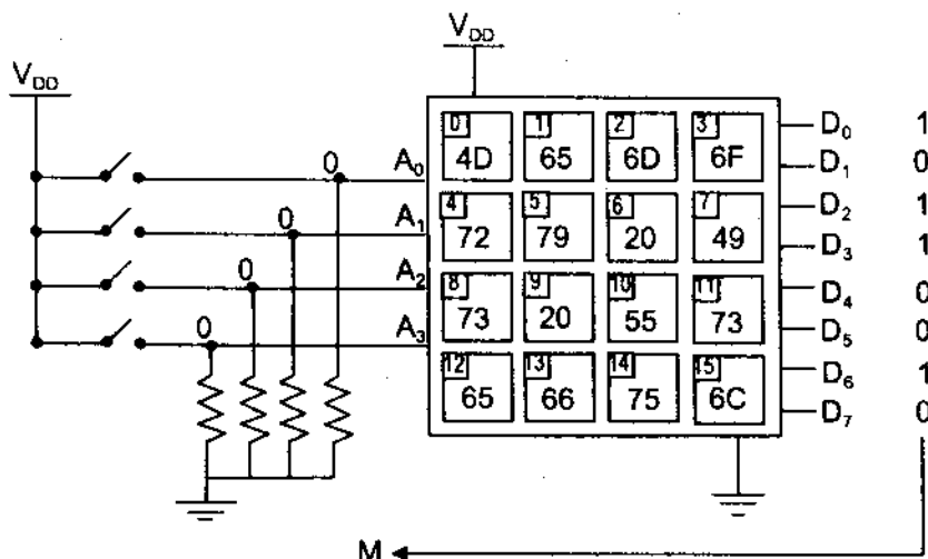
Hình 4.2. ROM (16×8bit)
