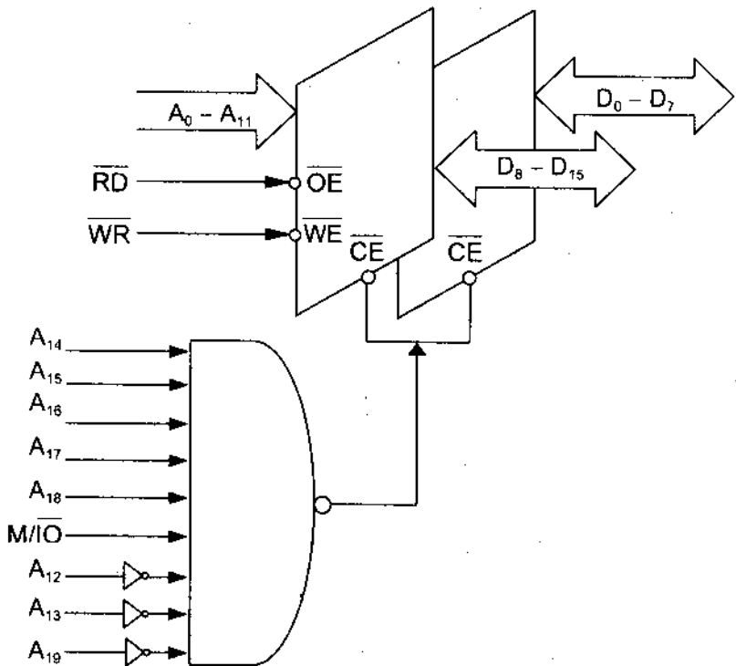
Hình 4.11. Sơ đồ mạch giải mã ví dụ 2
