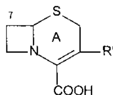
Cephem (Vòng A có 6 cạnh, không bão hoà)
