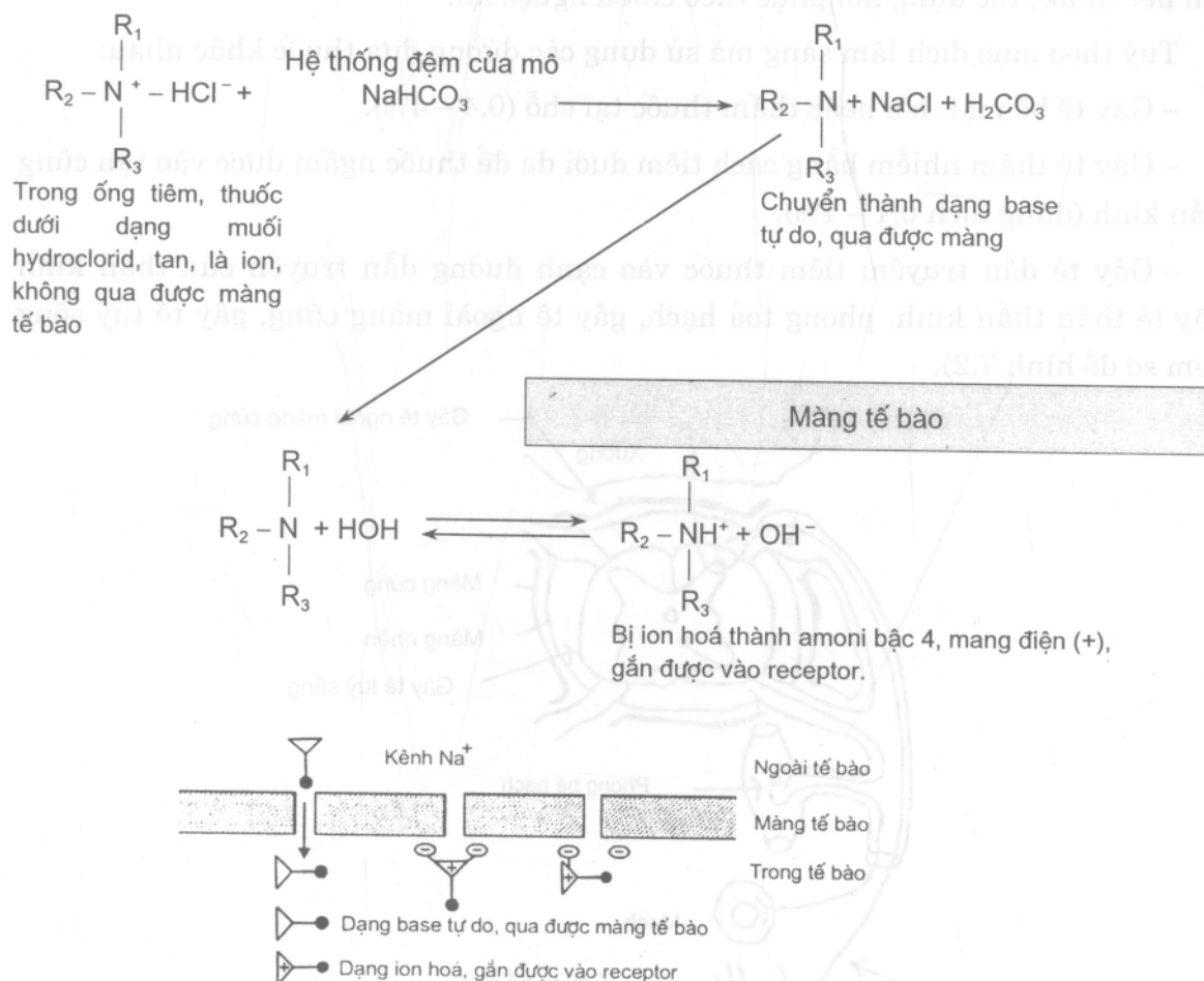
Hình 7.1. Quá trình thâm nhập của thuốc tê qua màng tế bào để gắn vào receptor
