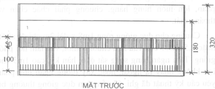
Hình 23: Sơ đồ thiết kế kiểu chuồng lợn đục giồng
