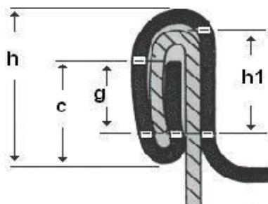
Hình V - 21. Mặt cắt ngang mối ghép
