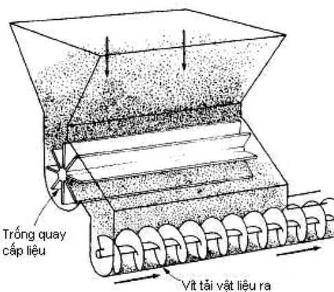
Hình IV- 6. Trống định lượng
