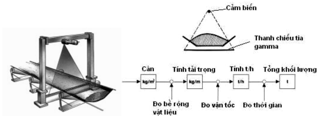
Hình IV- 4. Đo lường cung cấp bằng tia gamma
