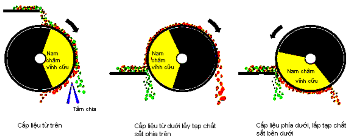
Hình III - 15. Trống quay tách tạp chất sắt từ
