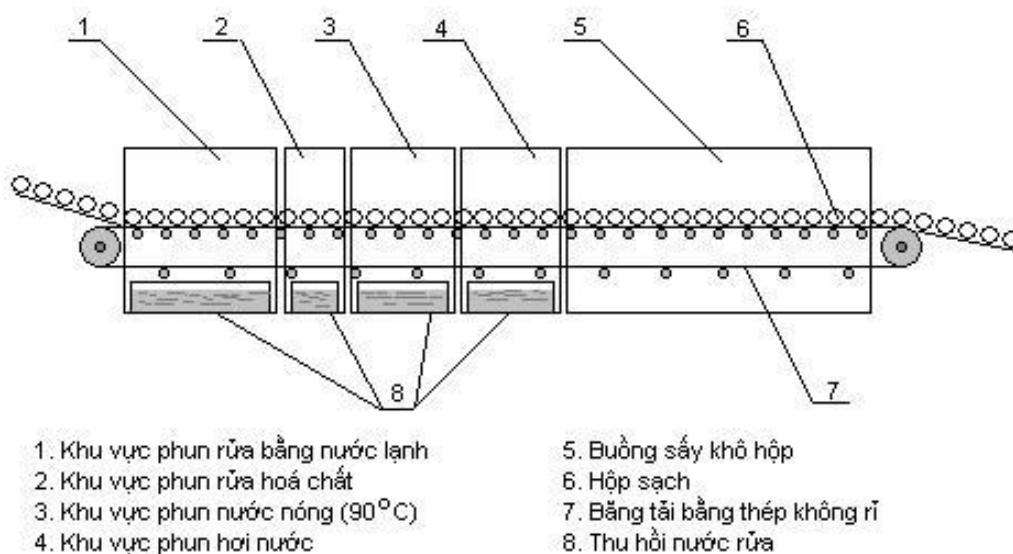
Hình II- 1. Máy rửa hộp sắt kiểu băng chuyền
