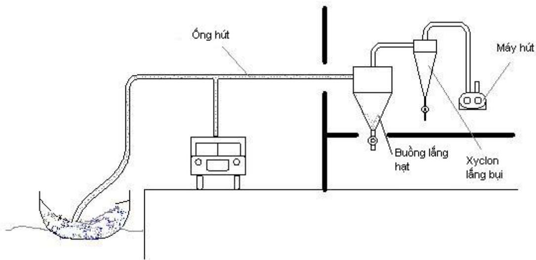
Hình 1 - 9. Hệ thống vận chuyển hạt bằng khí động
