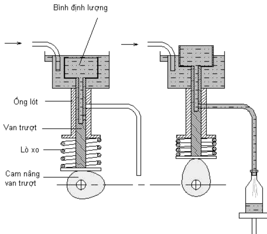
Hình VI - 3. Cơ cấu rót chính xác có bình lường-van trượt
