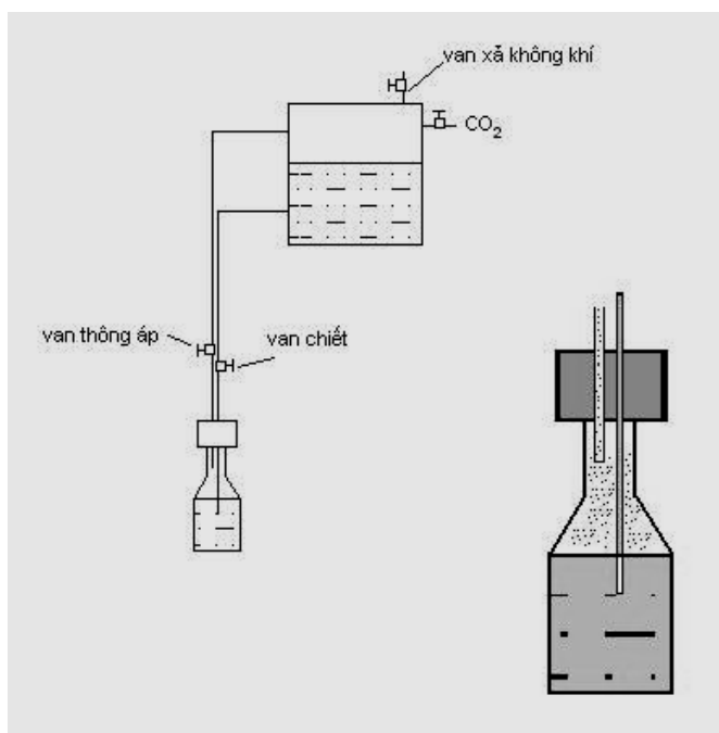
Hình VI - 4. Cơ cấu rót đẳng áp
