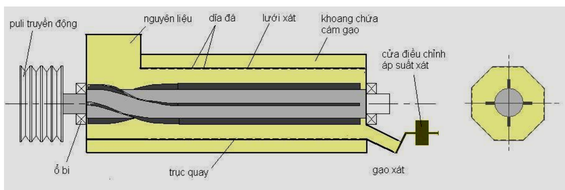
Hình V- 8. Máy xát trục vít
