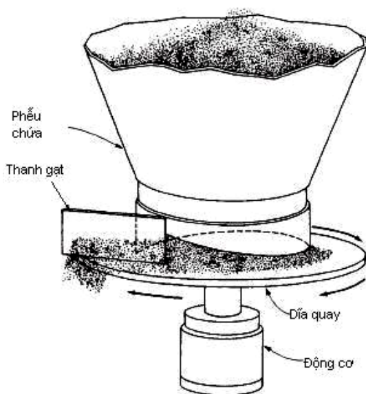
Hình IV- 5. Dĩa định lượng
