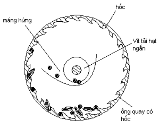
Hình III - 7. Ống phân loại hạt ngắn
