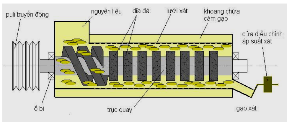
Hình V- 5. Máy sát nhiều đĩa đá
