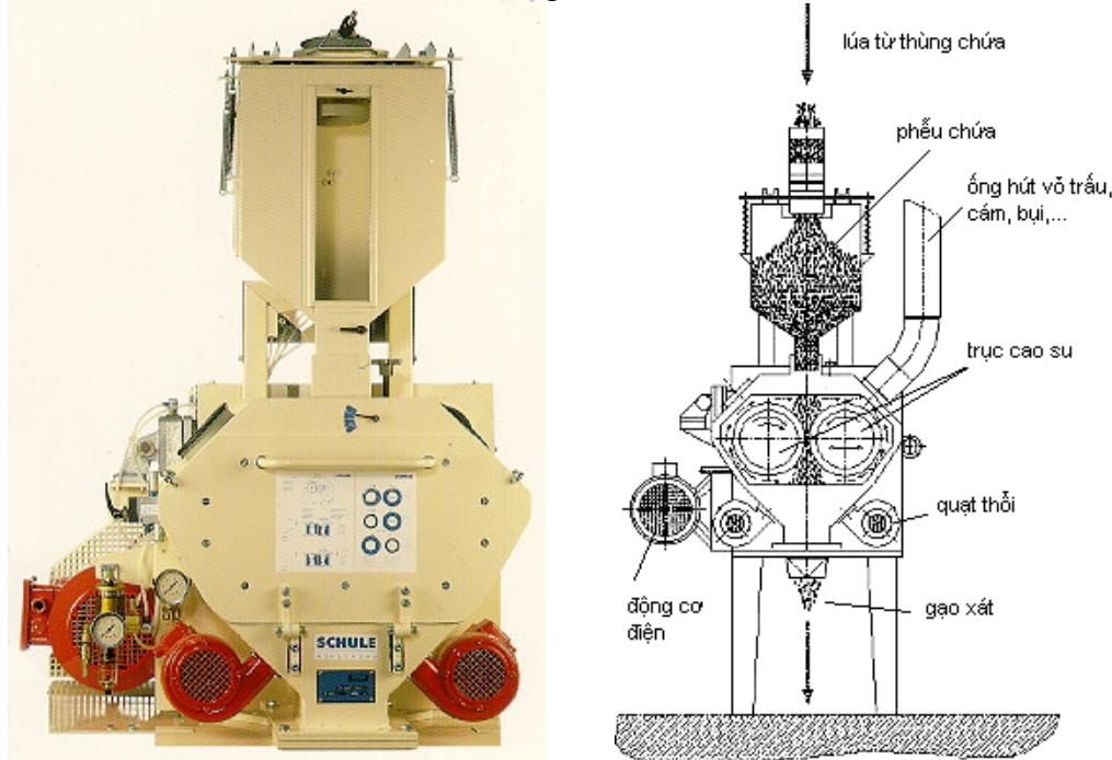
Hình V- 2. Máy xay 2 trục cao su
