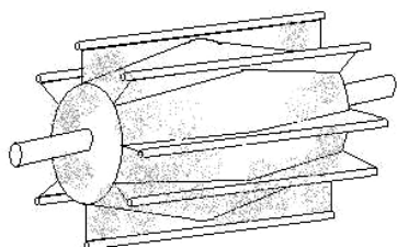
Hình I - 7. Puli căng dạng cánh chống nghiền nát vật liệu
