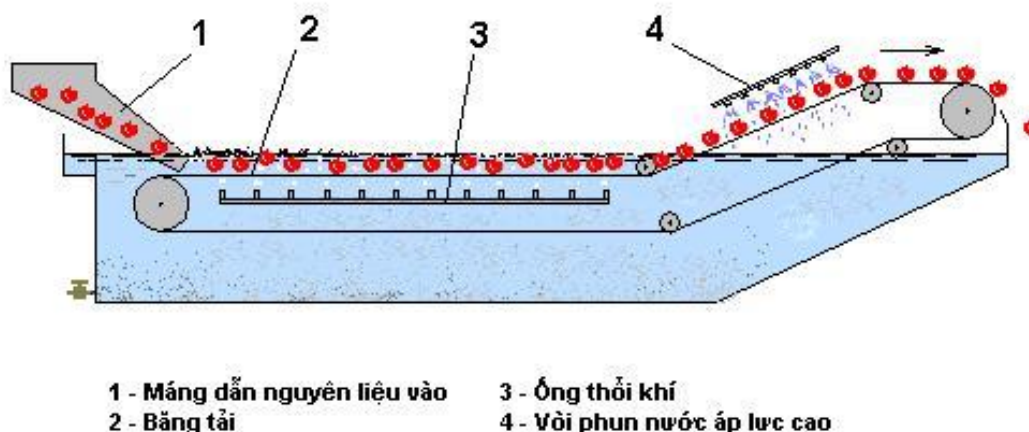
Hình II- 5. Máy rửa băng chuyền
