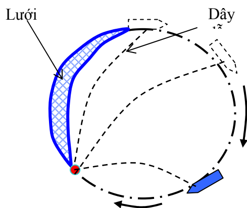
H 8.3 - Dây dẫn được thả khi bắt đầu thả lưới
