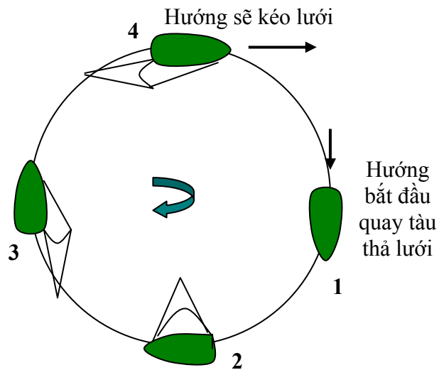
H 5.4 - Sơ đồ thả lưới bằng mạn tàu
