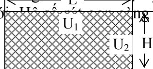
H 2.2 - Hệ số rút gọn ngang U_1 và hệ số rút gọn đứng U_2
