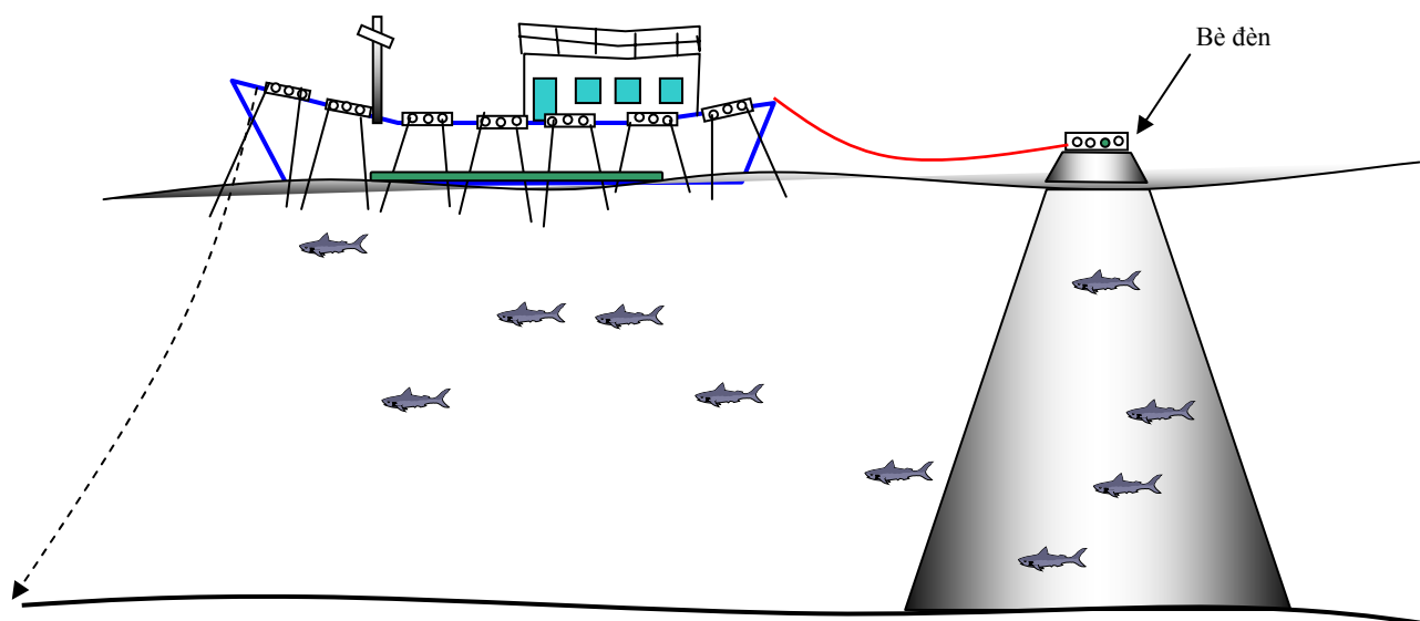
H 10.4 - Hệ thống chiếu sáng trên tàu lưới vây kết hợp ánh sáng
