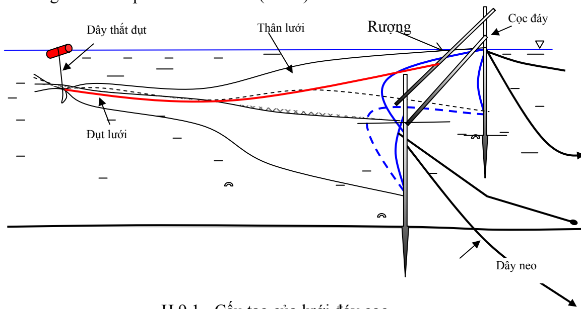
H 9.1 - Cấu tạo của lưới đáy cọc
