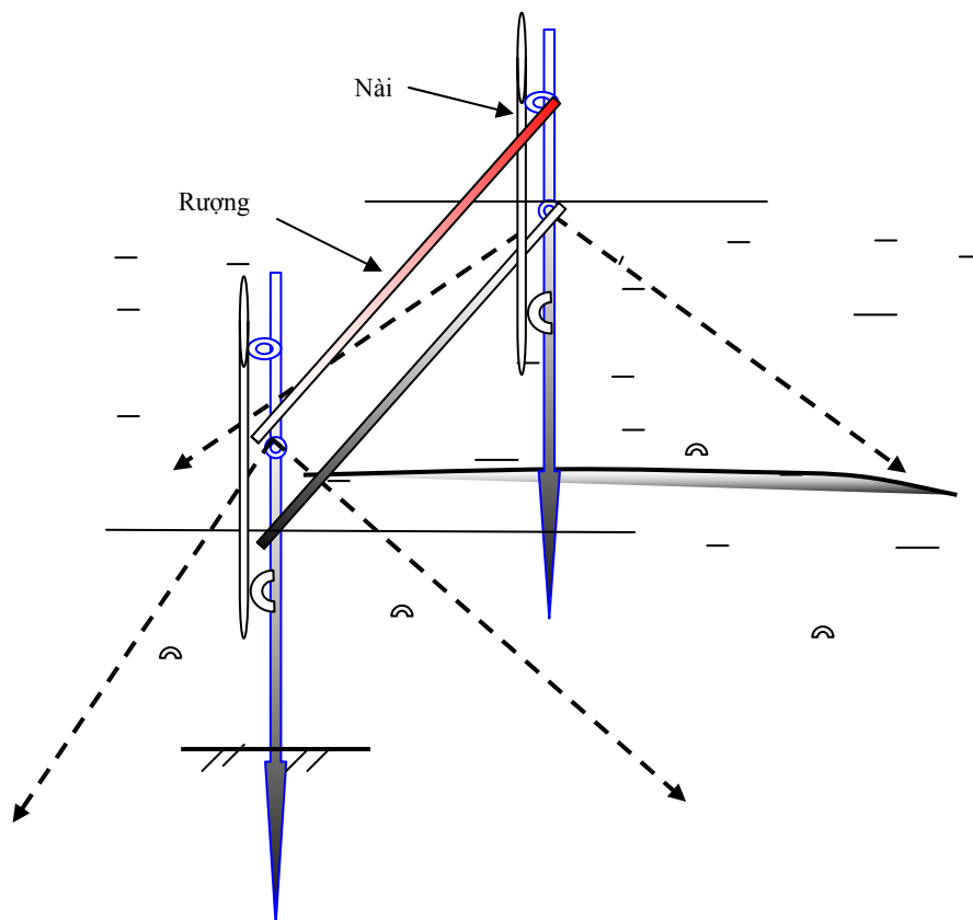
Hình 9.3 - Cọc lưới đáy
