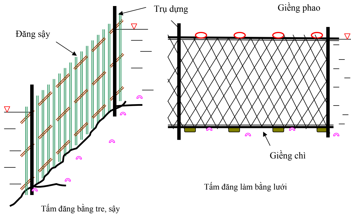
H 7.1 - Các dạng tấm đăng
