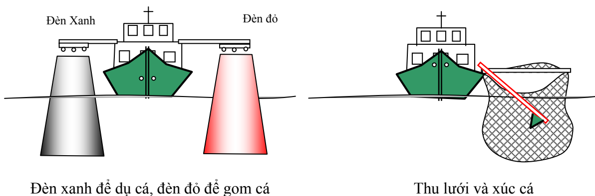
10.5 - Hệ thống khai thác lưới vó mạn tàu
