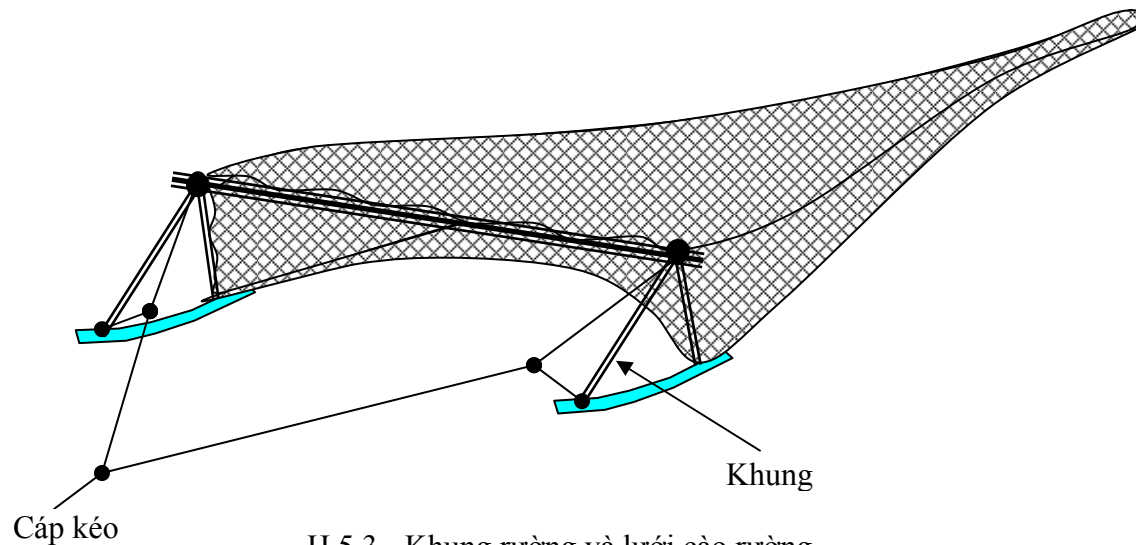
H 5.3 - Khung rường và lưới cào rường
