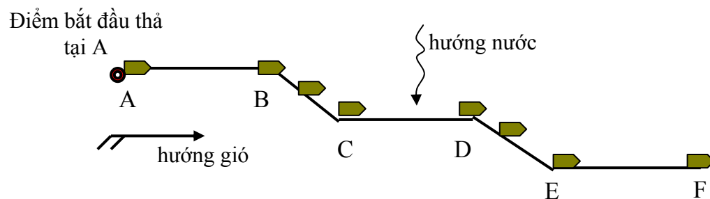
H 4.8 - Thả lưới theo kiểu zig-zag
