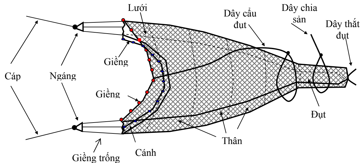
H 5.1 - Hình dạng tổng thể của lưới kéo
