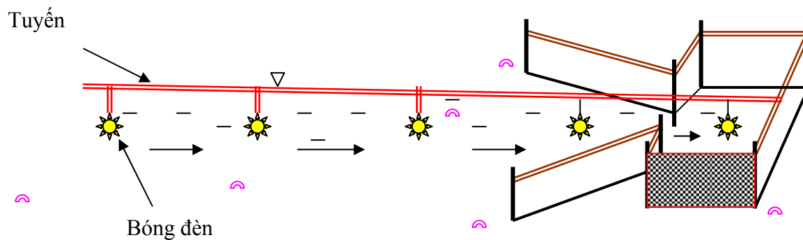
H 7.6 - Nguồn sáng bằng bóng đèn điện chịu áp lực nước
