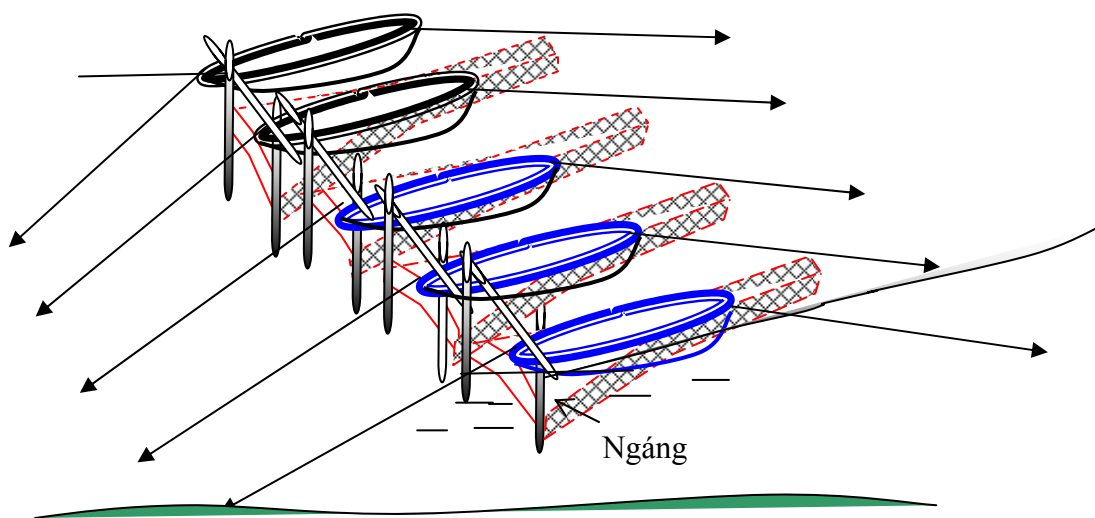
H 9.5 - Bè lưới đáy
