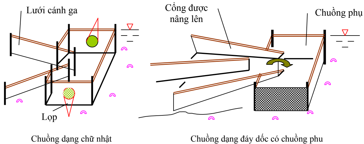
H 7.2 - Hình dạng chuồng lưới đăng
