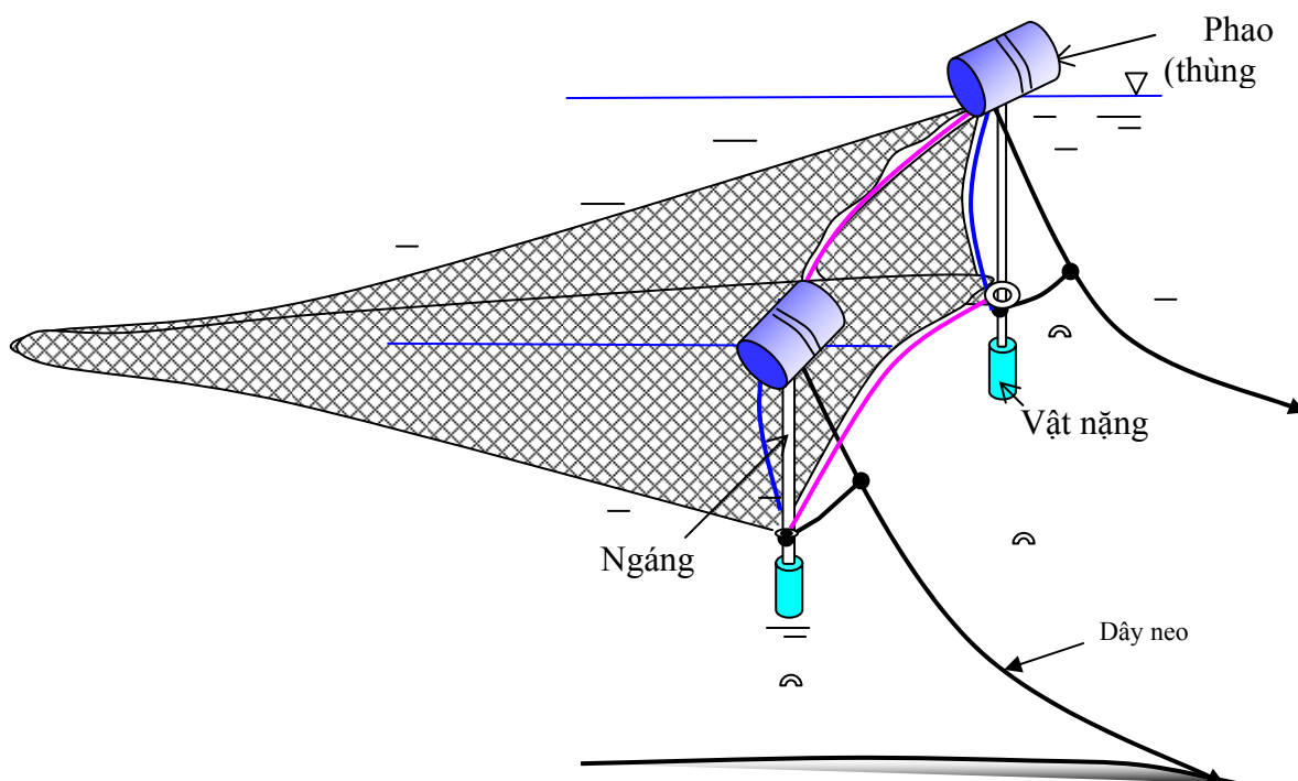
H 9.4 - Neo ngáng và phao nổi lưới đáy
