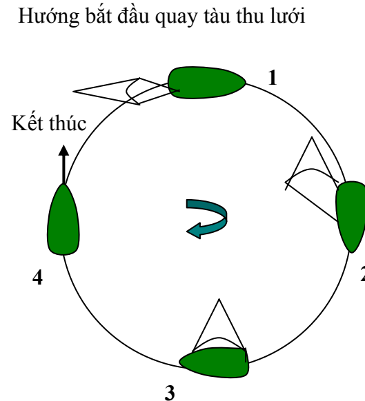
H 5.5 - Sơ đồ thu lưới bằng mạn tàu
