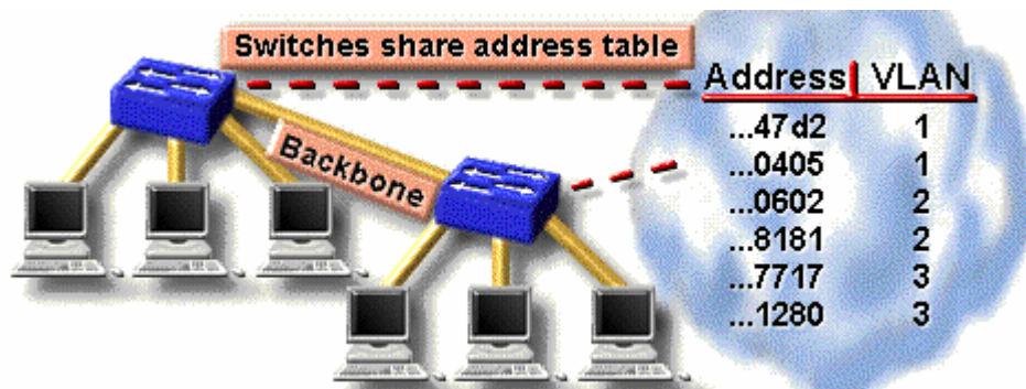
Hình 6.1 – VLAN sử dụng cơ chế lọc khung
