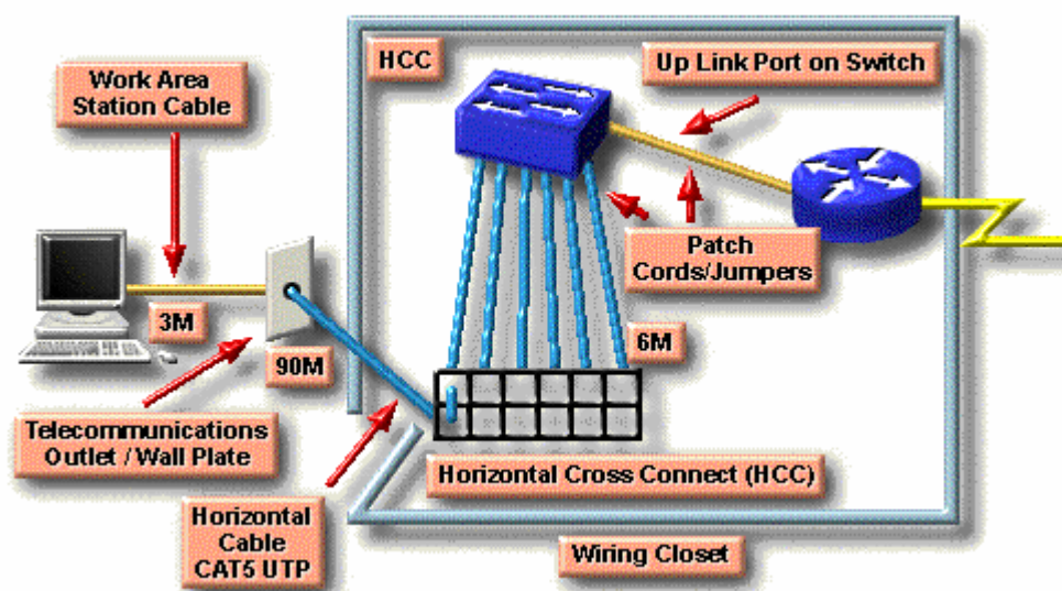
Hình 9.2 – Sử dụng HCC patch panel trong MDF
