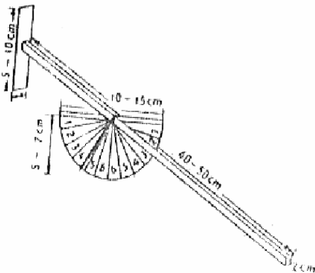
Hình 10.2. Thước đo độ nghiêng lá
