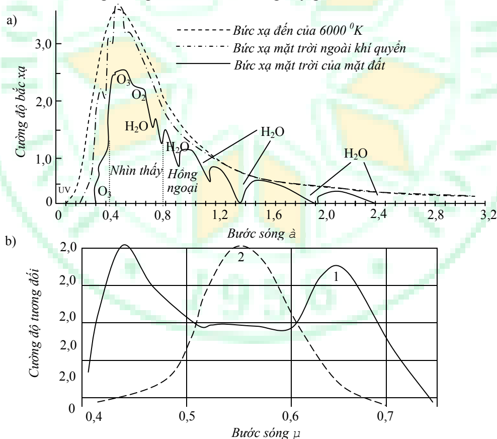
Hình 2.2. Quang phổ bức xạ mặt trời (a). So sánh đường cong quang phổ quang hợp của lúa mì và độ cảm giác nhìn thấy tương đối (b)
