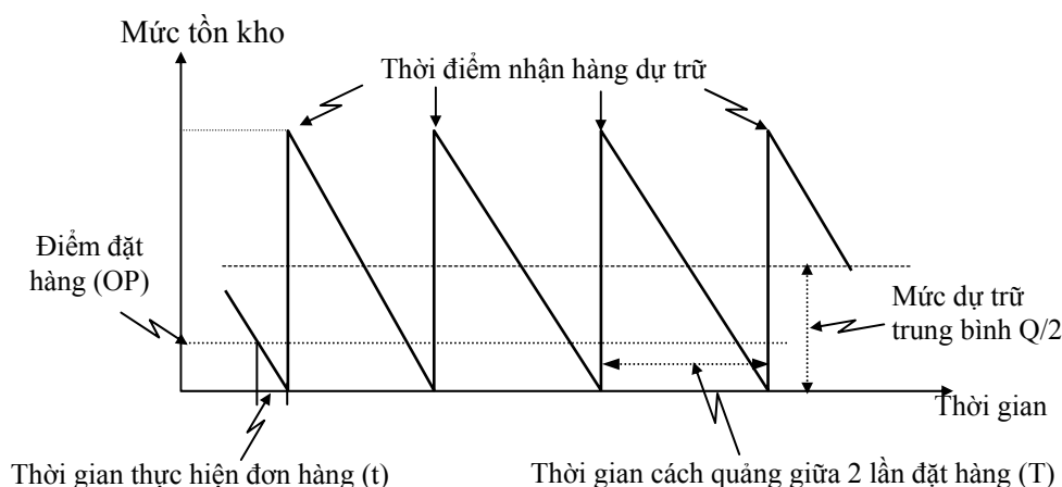
Sơ đồ 7.2a: Mô hình EOQ
