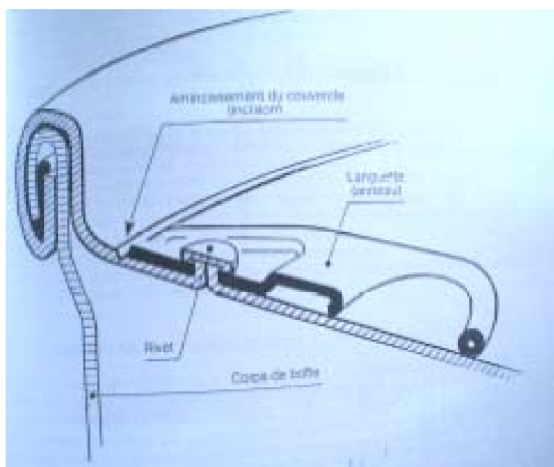
Hình 3.7. Mặt cắt ngang của hộp đã ghép kín
