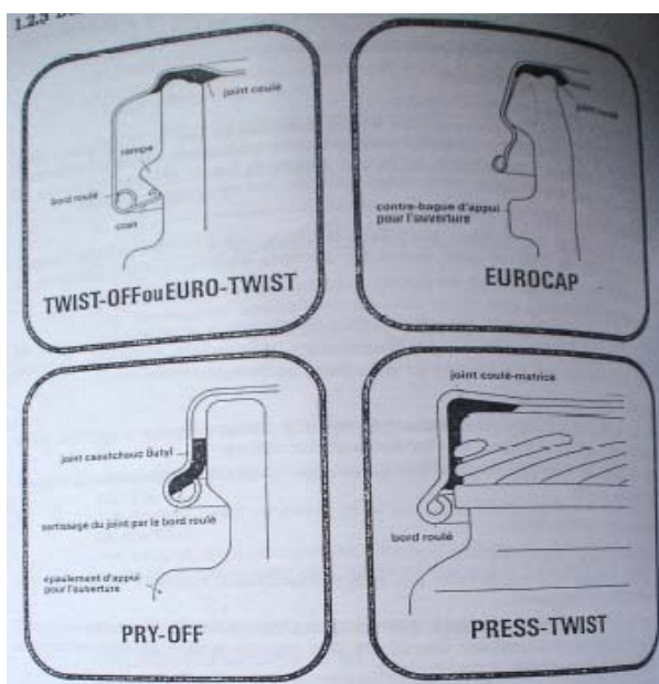
3.3. Kiểu nắp bao bì thủy tinh
