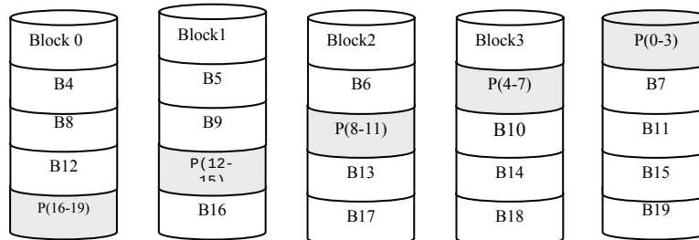
Hình V.13: RAID 5
