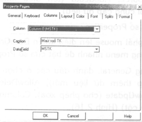
Hình 2.17. Trang Columns trong cửa sổ Property Pages của DataGrid.
