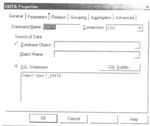
Hình 2.35. Cửa sổ Properties của Command.
