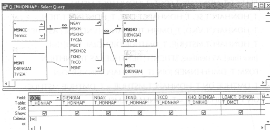
Hình 4.13. Query Q_INHHDNHAP.
