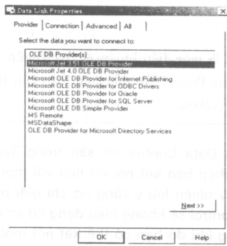
Hình 2.12. Trang Provider.
