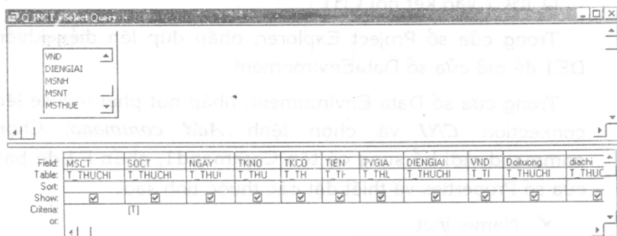
Hình 3.16. Query Q_INCT.
