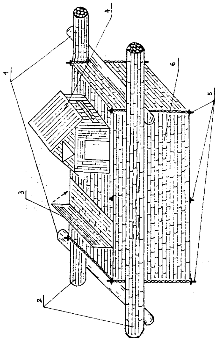
1. Đà-ké 2. Phao 3. Cửa lồng 4. Nhà bảo vệ 5. Trụ lồng
