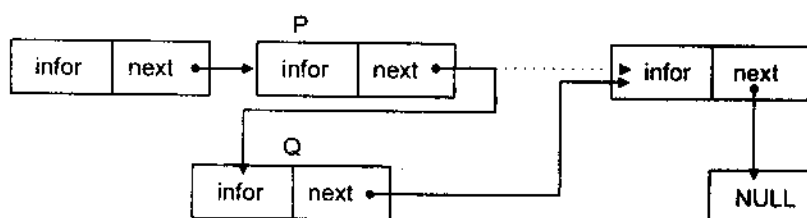
Hình 4.6. Phép thêm phần tử vào giữa danh sách liên kết đơn
