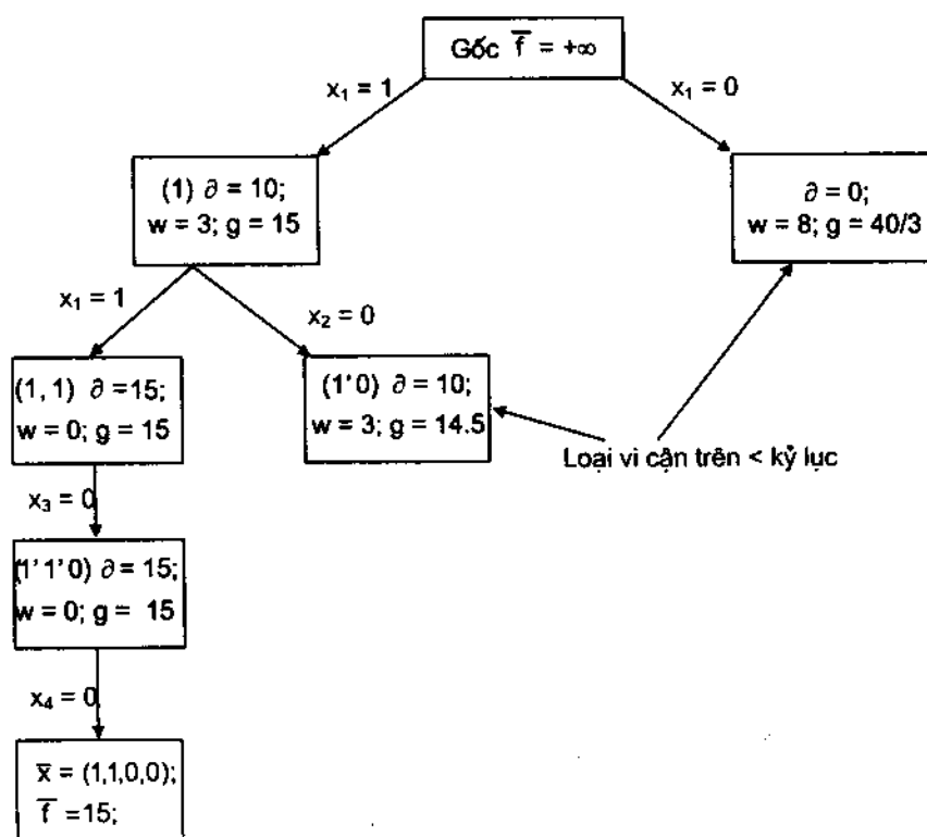
Hình 3.5. Giải bài toán cái túi theo thuật toán nhánh cận.
