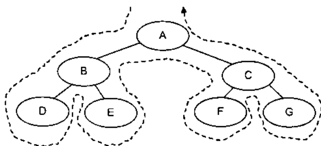
Hình 5.13 Mô tả phương pháp duyệt cây nhị phân
