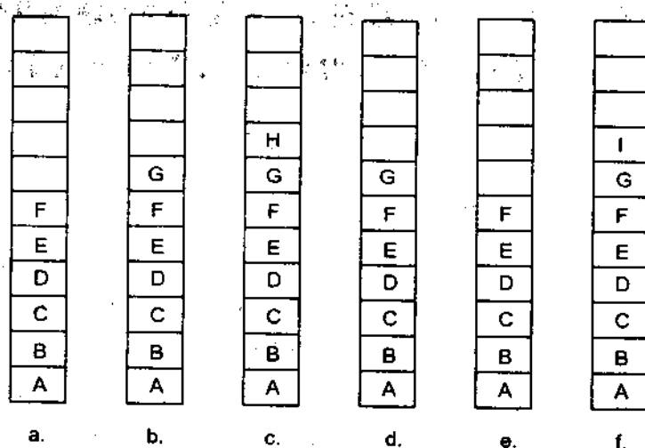
Hình 4.1 Sự thay đổi của stack thông qua các thao tác thêm và bớt đỉnh trong stack
