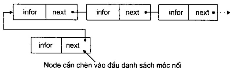
Hình 4.4. Thêm đỉnh mới vào đầu danh sách móc nối đơn
