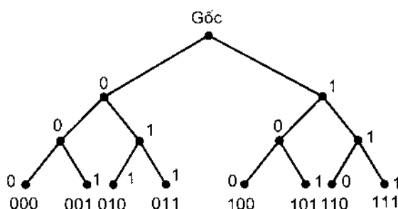
Hình 3.2. Cây tìm kiếm lời giải liệt kê dãy nhị phân độ dài 3
