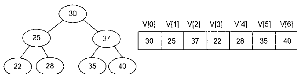
Hình 5.7. Lưu trữ kế tiếp của cây nhị phân
