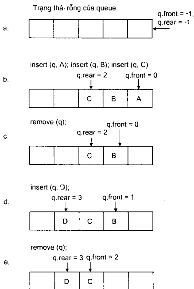
Hình 4.2 Các thao tác trong hàng đợi
