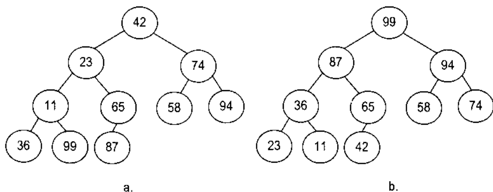
Hình 7.1 Tìm kiếm theo giải thuật Heap Sort
