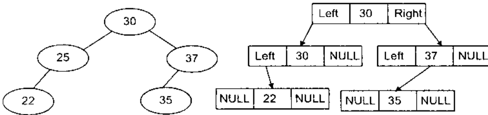
Hình 5.10 Biểu diễn cây nhị phân bằng danh sách móc nối
