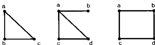
Hình 6.18. Đồ thị Hamilton G_3 , nửa Hamilton G_2 và G_1 .
