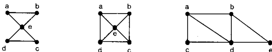
Hình 6.15. Đồ thị vô hướng G_1 , G_2 , G_3 .
