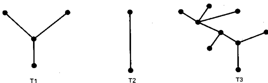
Hình 6.20 Rừng gồm 3 cây T_1, T_2, T_3 .
