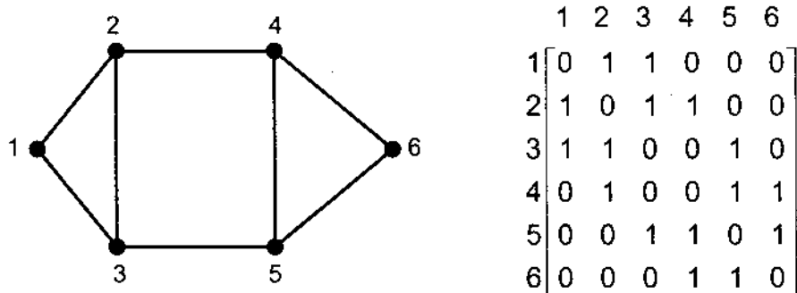
Hình 6.9. Đồ thị vô hướng G
