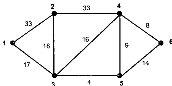
Hình 6.21. Đồ thị vô hướng liên thông G = \langle V, E \rangle
