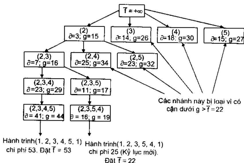
Hình 3.6. Cây tìm kiếm lời giải bài toán người du lịch.
