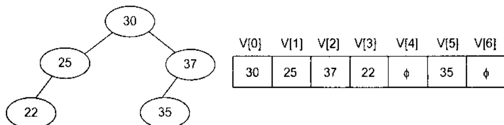
Hình 5.8. Lưu trữ kế tiếp của cây nhị phân không đầy đủ
