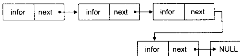
Hình 4.5. Thêm node mới vào cuối danh sách.
