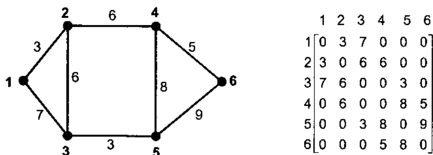
Hình 6.11. Đồ thị trọng số G
