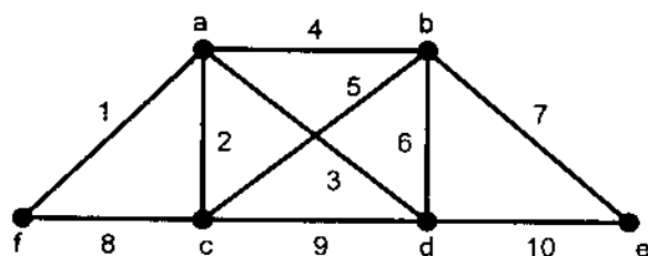
Hình 6.17. Đồ thị vô hướng G .
