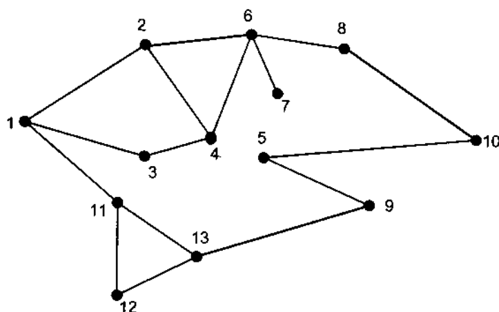
Hình 6.12. Đồ thị vô hướng G
