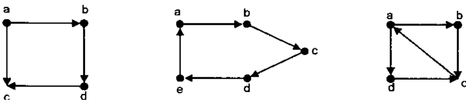
Hình 6.16. Đồ thị có hướng H_1 , H_2 , H_3 .
