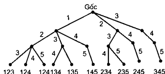
Hình 3.3. Cây liệt kê tổ hợp chập 3 từ {1, 2, 3, 4, 5}
