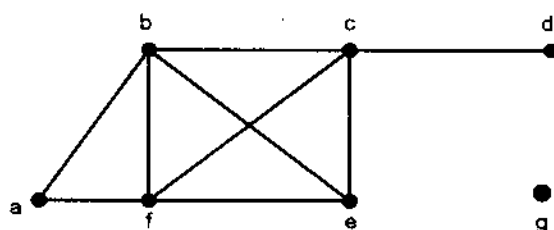
Hình 6.6 Đồ thị vô hướng G
