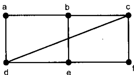
Hình 6.8. Đường đi trên đồ thị
