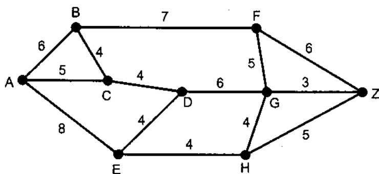
Hình 6.22. Đồ thị trọng số G
