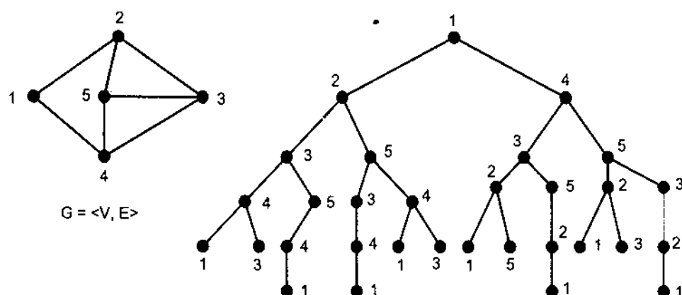
Hình 6.19. Cây tìm kiếm chu trình Hamilton.
