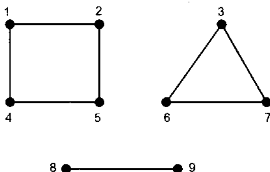
Hình 6.14. Đồ thị vô hướng G .
