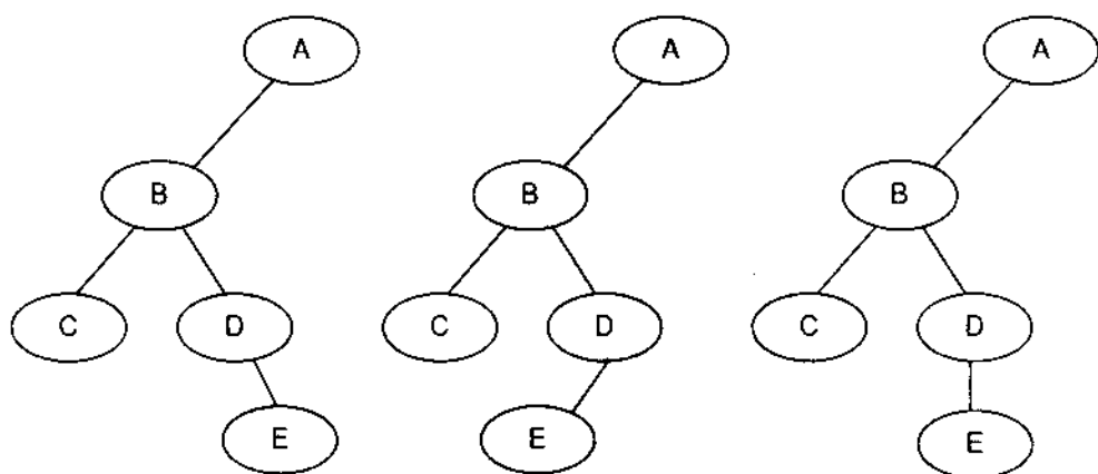
Hình 5.3 Các cây nhị phân
