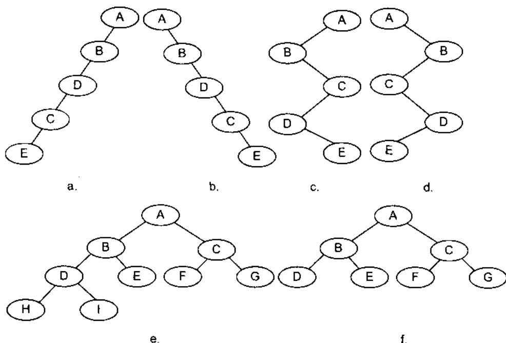
Hình 5.4 Các cây nhị phân có dạng đặc biệt
