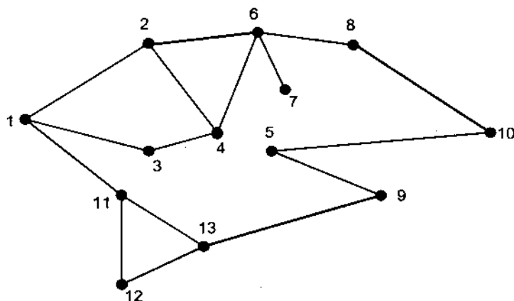
Hình 6.13 Đồ thị vô hướng G
