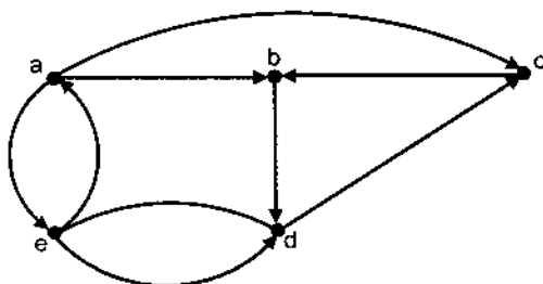
Hình 6.7. Đồ thị có hướng G .
