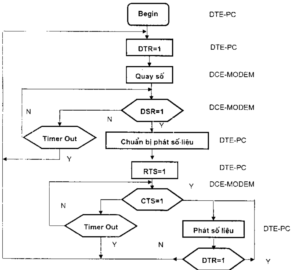
Hình 6.4. Lưu đồ thuật toán của quá trình thu/ phát
