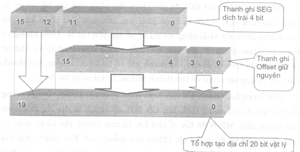
Hình 1.4. Minh họa cách tính địa chỉ ngăn nhớ từ địa chỉ Segment và địa chỉ offset (minh họa cho bộ VXL 80286)
