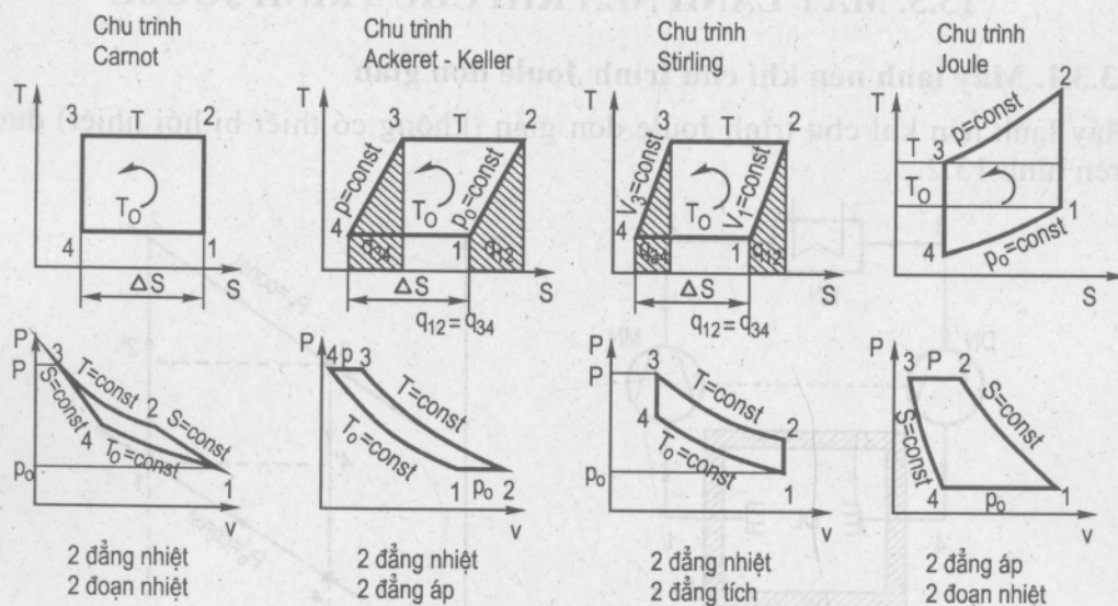
Hình 13.1 : Các chu trình có thể của máy lạnh nén khí.
