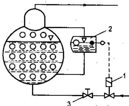
Hình 14.13 : Hệ thống điều chỉnh cấp lỏng 2 vị trí theo mức lỏng.
