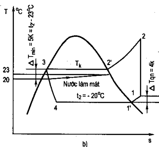
Hình 5.17 : Chu trình a và b trên đồ thị T-s.
