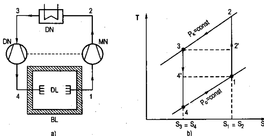
Hình 13.2 : Máy lạnh nén khí chu trình Joule.
