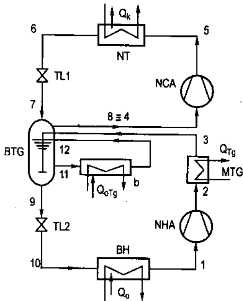
Hình 6.6 : Chu trình 2 cấp 2 chế độ bốc hơi dùng cho \text{NH}_3 a) Thiết bị bay hơi áp thấp p_o ; t_o b) Thiết bị bay hơi trung gian p_{tg} ; t_{tg}
