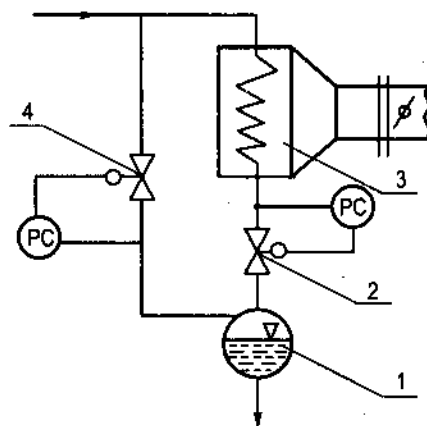
Hình 14.7 : Điều chỉnh áp suất ngưng tụ bằng dàn ngưng giải nhiệt gió.
