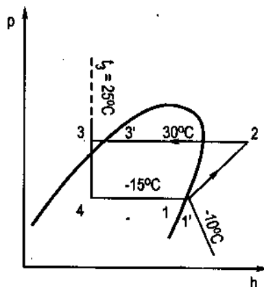
Hình 4.11 : Biểu diễn chu trình trên đồ thị lgp-h.
