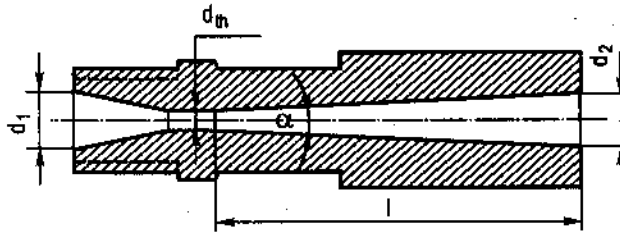
Hình 12.5 : Ống phun hơi.
