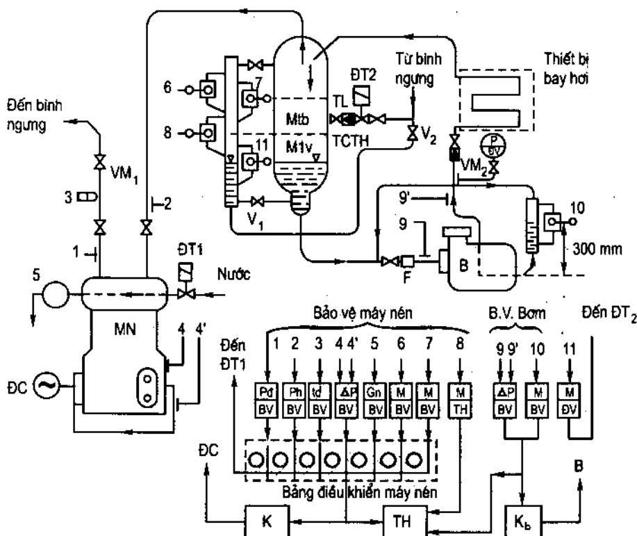
Hình 14.17 : Sơ đồ bảo vệ máy nén và bơm amôniac.
