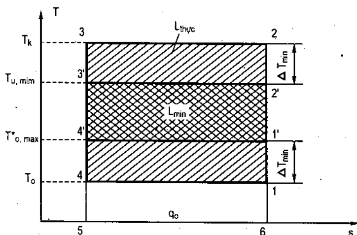
Hình 5.11 : Tổn thất do quá trình trao đổi nhiệt không thuận nghịch ở thiết bị ngưng tụ và bay hơi.
