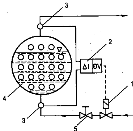
Hình 14.11 : Sơ đồ điều chỉnh cấp lỏng hai vị trí (ĐV) theo tín hiệu nhiệt độ \Delta t .
