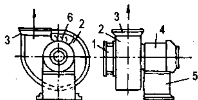
Hình 10.15 : Quạt ly tâm.
