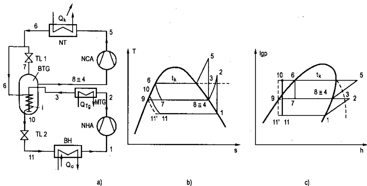
Hình 6.4 : Chu trình hai cấp, hai tiết lưu, bình trung gian ống xoắn dùng cho \text{NH}_3
