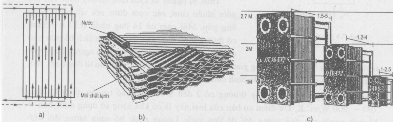
Hình 7.8 : TBNT kiểu tấm (panen)
