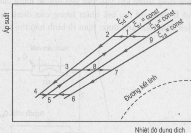
Hình 11.11 : Chu trình máy lạnh hấp thụ H_2O/LiBr tác dụng kép trên đồ thị \lg p - 1/T .
