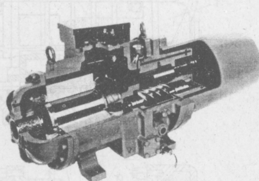
Hình 4.26c : Máy nén trục vít kiểu 2 trục (bóc cắt) của Hitachi.
