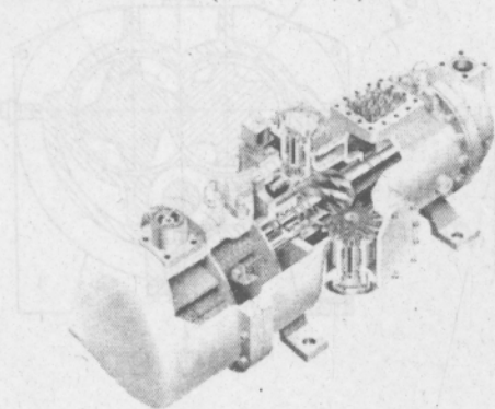
Hình 4.26b : Máy nén trục vít nửa kín có 1 trục (bóc cắt) của Daikin
