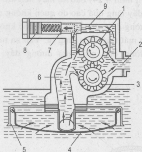
Hình 4.25 : Bơm dầu
