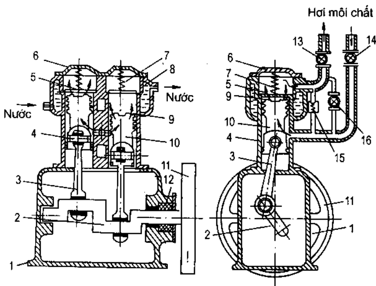
Hình 4.14 : Nguyên lí cấu tạo máy nén hơi, 2 xi lanh đứng, thuận đồng
