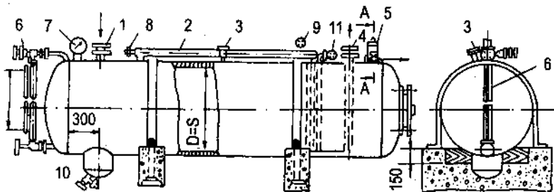
1 - Môi chất lỏng vào ; 2 - Bình tách khí không ngưng ; 3 - Đường cân bằng hơi ; 4 - Lỏng ra ; 5 - Van an toàn ; 6 - Mức lỏng kế ; 7 - Áp kế ; 8 - Vẽ đường hút ; 9 - Xả khí qua nước ; 10 - Xả dầu ; 11 - Tiết lưu lỏng vào 2.
