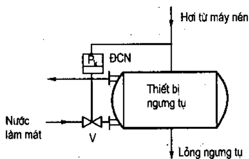
Hình 14.4 : Điều chỉnh lưu lượng nước làm mát.
