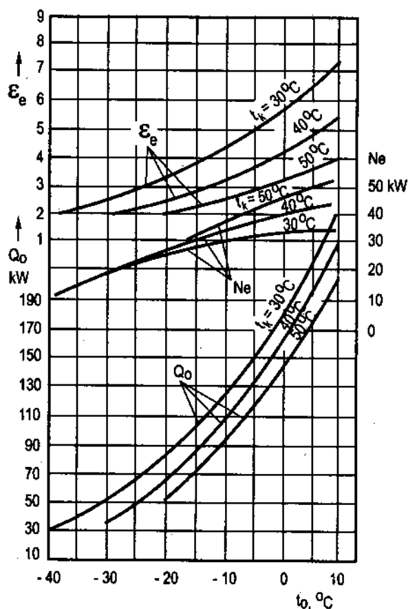
Hình 5.15 : Các đường đặc tính hoặc sự phụ thuộc của Q_o , N_e , \epsilon vào t_o và t_k của máy nén P80 (8 xi lanh, d = 76\text{mm} , S = 66\text{mm} , môi chất R22).
