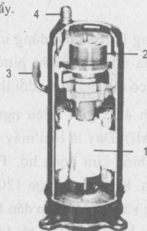
Hình 4.33 : Hình ảnh một máy nén xoắn ốc tách vỏ 1 – Động cơ ; 2 – Băng xoắn động và tĩnh (pittông và xi lanh) ; 3 – Ống hút ; 4 – Ống đẩy.
