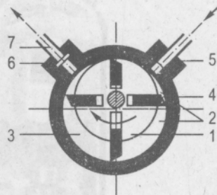
Hình 4.28 : Nguyên tắc làm việc của máy nén rôto tấm trượt
