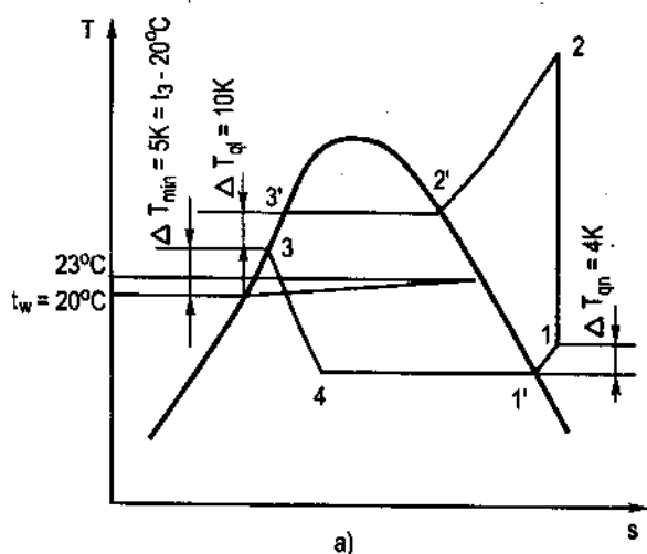
Hình 5.17 : Chu trình a và b trên đồ thị T-s.
