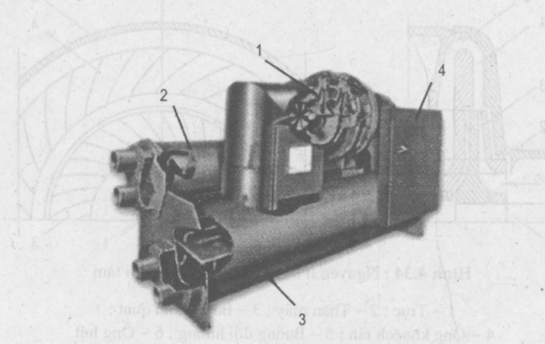
Hình 4.35 : Chiller làm lạnh nước, giải nhiệt nước, máy nén li tâm CentraVac của Trane (Mi) dùng cho điều hoà không khí trung tâm
