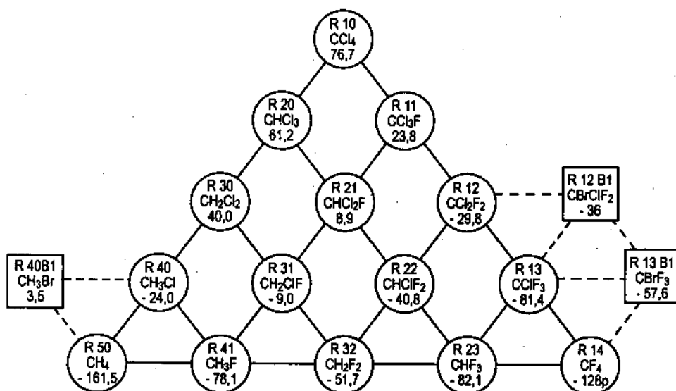
Hình 3.10 : Các chất dẫn xuất từ metan \text{CH}_4 .
