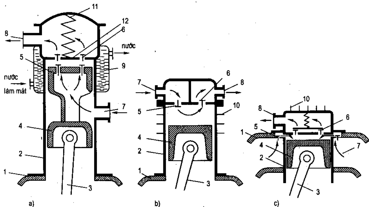
Hình 4.12 : a) Máy nén thuận dòng
