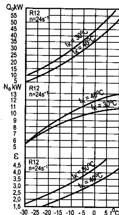
Hình 4.10 : Đặc tính máy nén hay quan hệ giữa năng suất lạnh Q_o , công suất hữu ích N_e và các hệ số lạnh lý thuyết \epsilon vào nhiệt độ bay hơi và ngưng tụ t_k của máy nén FV20.
