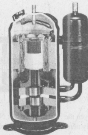
Hình 4.30b : Máy nén rôto đôi (twin rotary) của Toshiba – Carrier dùng cho PAC (Packaged Air Conditioner).
