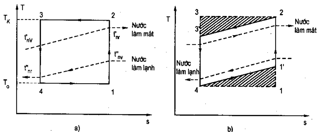
Hình 3.1 : a) Chu trình Carnot 1-2-3-4 ; b) Chu trình Lorenz 1'-2-3'-4 Công tiết kiệm được của chu trình Lorenz so với Carnot
