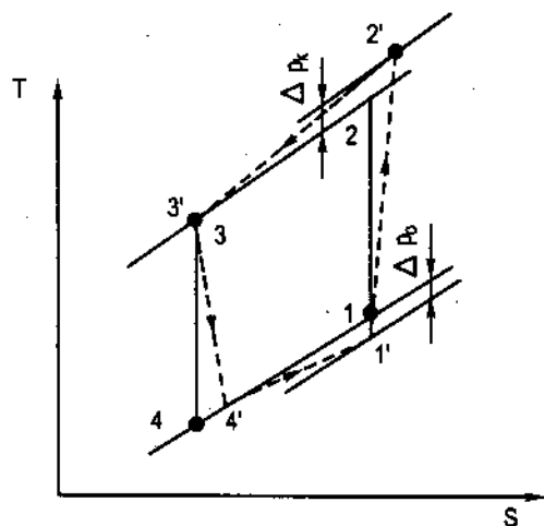
Hình 13.3 : Chu trình thực với tổn thất áp suất.
