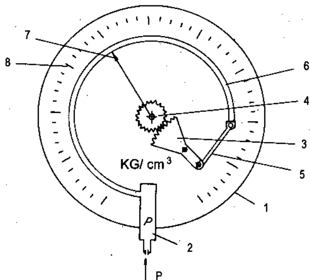
Hình 10.20 : Áp kế.
