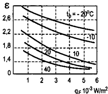
Hình 8.17 : Biểu đồ xác định hệ số \epsilon a – Đối với R22 b – Đối với R12
