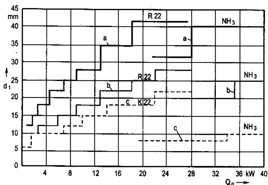
Hình 10.21 : Đường kính ống phụ thuộc loại môi chất và năng suất lạnh Q_0 .
