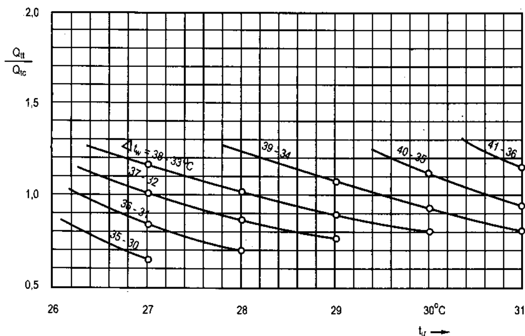
Hình 9.2 : Sự phụ thuộc của năng suất lạnh thấp vào nhiệt độ ướ t_u và nhiệt độ nước vào ra khỏi tháp với giả thiết hiệu nhiệt độ nước vào ra là 5K không đổi.
