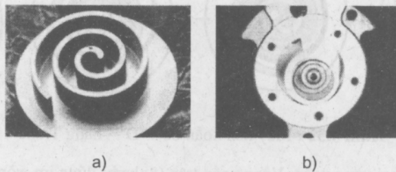
Hình 4.31 : a) Hình dáng pittông và xi lanh dạng băng xoắn máy nén xoắn ốc ;
