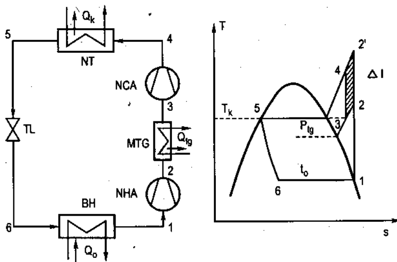
Hình 6.1 : Chu trình hai cấp nén, một tiết lưu làm mát trung gian không hoàn toàn
