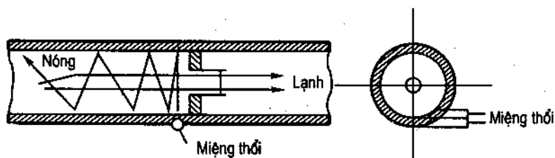
Hình 2.4 : Ống xoáy.
