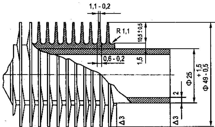
Hình 7.14 : Ống hai kim loại có cánh trong TBNT làm mát bằng không khí
