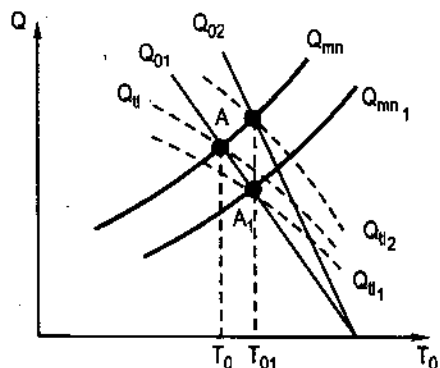
Hình 14.1 : Xác lập nhiệt độ sôi trong thiết bị bay hơi của hệ thống lạnh.
