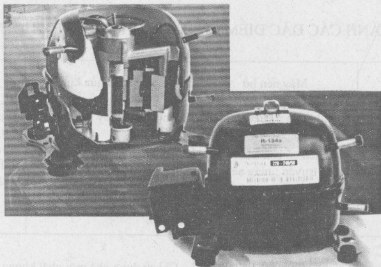
Hình 4.17b : Hình cắt và hình dáng bên ngoài một kiểu máy nén kín của Tecumseh dùng cho tủ lạnh gia đình (máy nén bố trí phía trên động cơ phía dưới).
