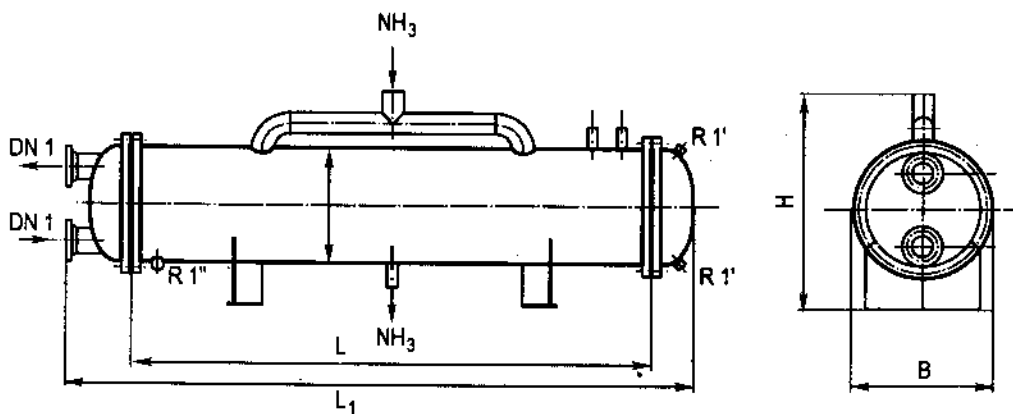
Hình 7.4 : Bình ngưng ống chùm của hãng Guntner
