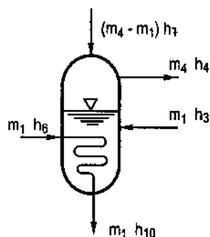
Hình 6.5 : Cân bằng entanpy ở bình trung gian có ống xoắn.
