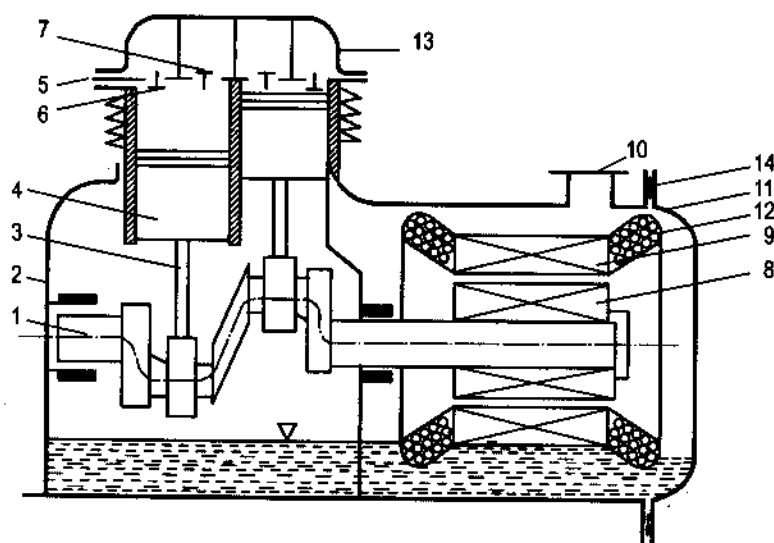
Hình 4.16a : Nguyên lí cấu tạo máy nén nửa kín
