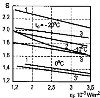
Hình 8.17 : Biểu đồ xác định hệ số \epsilon a – Đối với R22 b – Đối với R12
