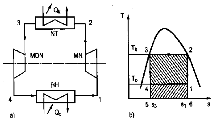
Hình 5.1 : Chu trình Carnot ngược chiều
