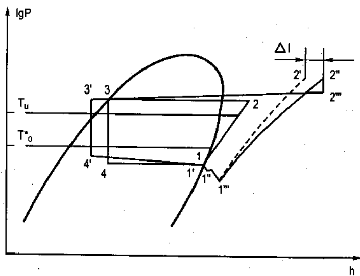
Hình 5.12 : Chu trình thực với các tổn thất cơ bản.
