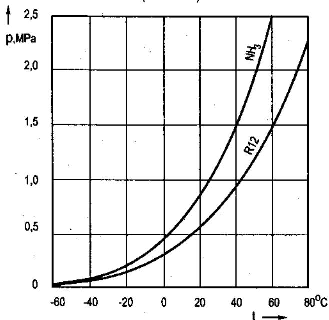
Hình 3.2 : Đường cong áp suất hơi của R12 và R717 ( \text{NH}_3 )
