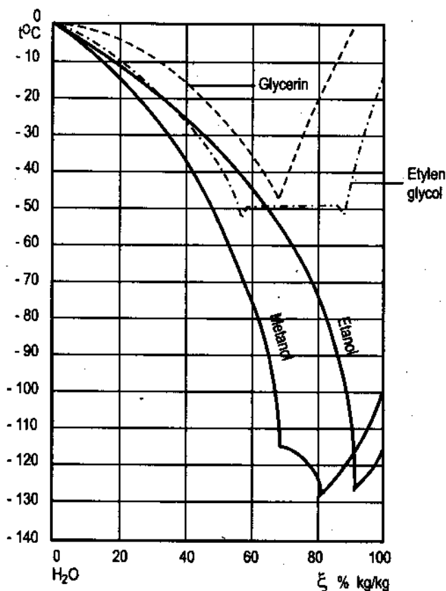
Hình 3.13 : Đường đông băng của các dung dịch chất hữu cơ và nước.
