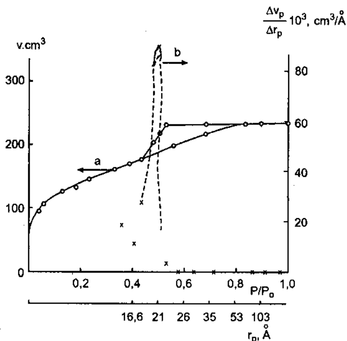
Hình 62.7. Sự hấp phụ \text{N}_2 ở -195^\circ\text{C} , trên \text{Al}_2\text{O}_3 ;
