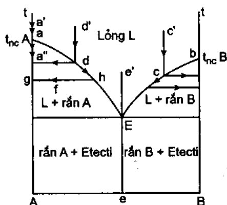
Hình 47.2. Biểu đồ nóng chảy của hệ hai cấu tử có điểm ectecti và không tạo thành dung dịch rắn (kiểu I)
