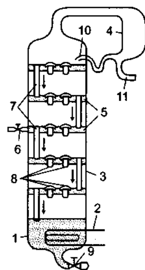
Hình 37.8. Sơ đồ cột tinh cất
