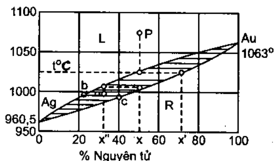
Hình 47.5. Biểu đồ nóng chảy của hệ vàng – bạc tạo thành dung dịch rắn ở mọi tỉ lệ (kiểu II).
