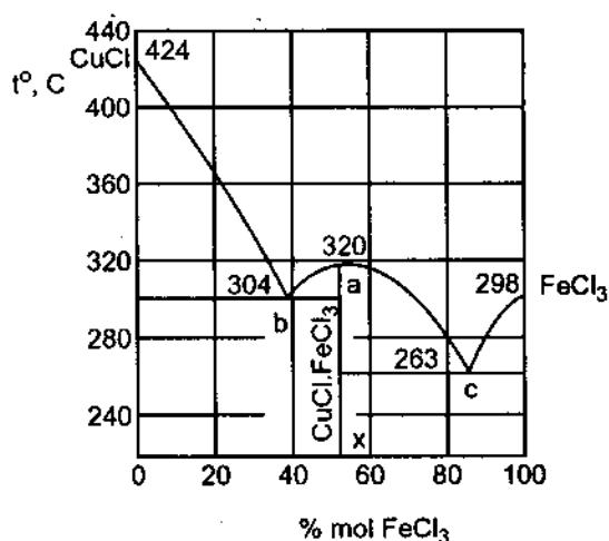
Hình 47.9. Biểu đồ nóng chảy của hệ \text{CuCl} - \text{FeCl}_3 tạo thành hợp chất hoá học có điểm nóng chảy toàn đẳng (kiểu IV).
