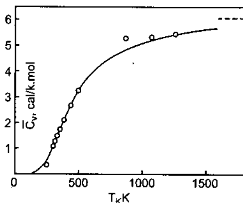
Hình 56.2. Sự phụ thuộc nhiệt dung của kim cương vào nhiệt độ o - giá trị thực nghiệm - hàm Einstein - - - giá trị giới hạn theo định luật Dulong Petit.
