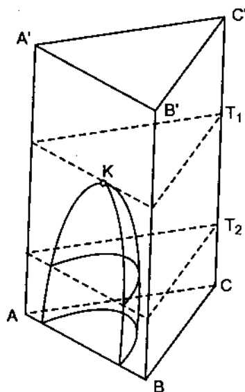
Hình 48.8. Biểu đồ thể tích về tính tan của hệ ba chất lỏng A, B và C (A và B hoà tan hạn chế)
