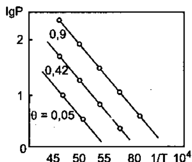
Hình 58.6. Các đường đẳng lượng hấp phụ etan trên muội graphite ở các độ che phủ \theta khác nhau.
