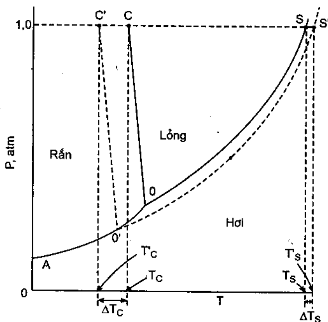
Hình 41.1. Biểu đồ pha của nước.
