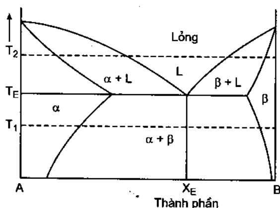
Hình 49.1. Biểu đồ pha của hệ hai cấu tử hoà tan hạn chế ở pha rắn.
