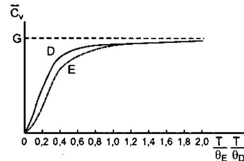
Hình 56.5. Sự phụ thuộc nhiệt dung của các đơn chất rắn vào nhiệt độ.
