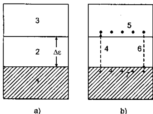
Hình 57.16. Sơ đồ vùng năng lượng
