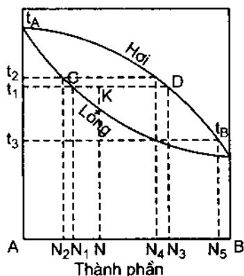
Hình 37.6. Biểu đồ nhiệt độ sôi – thành phần của hệ hai cấu tử
