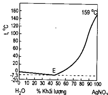
Hình 47.3. Biểu đồ nóng chảy của hệ nước – bạc nitrat.
