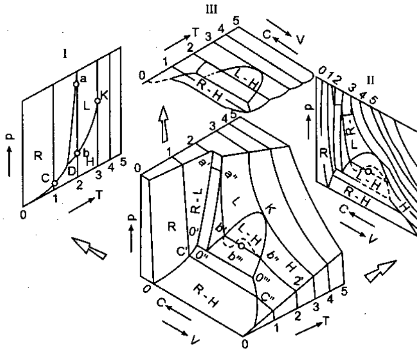
Hình 46.2. Biểu đồ pha (3 chiều) của \text{CO}_2 và hình chiếu của nó lên các mặt phẳng P-T (I), P-V (II) và V-T (III). Các đường 1, 2, 3, 4, 5 là các đường đẳng nhiệt.
