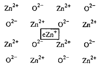
Hình 57.7. Sự thừa cation \text{Zn}^{2+} trong ZnO làm xuất hiện electron tự do trong tinh thể.
