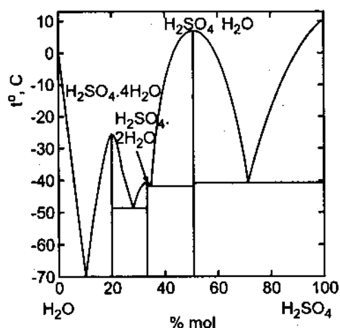
Hình 47.10. Biểu đồ nóng chảy của hệ nước - axit sunfuric tạo thành nhiều hợp chất hoá học.
