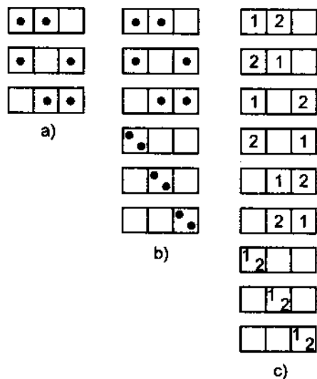
Hình 52.4. Sự phân bố các hạt theo các ô : (a) – Các hạt fermion ; (b) – Các hạt bozon ; (c) các hạt cổ điển (Các con số đánh dấu hạt thứ nhất và thứ hai).
