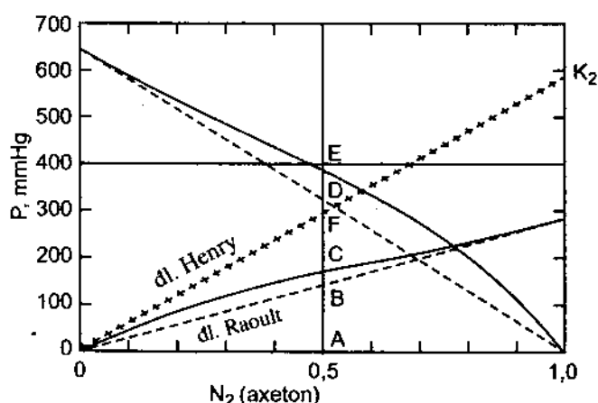
Hình 43.2. Áp suất hơi riêng phần trên dung dịch ete – axeton ở 30°C.
