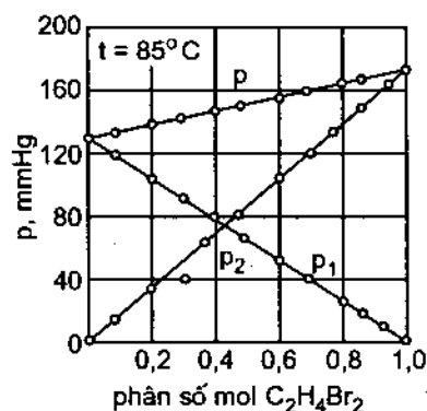
Hình 36.3. Áp suất hơi của dung dịch dibromopropan – dibrometan
