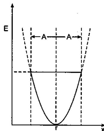
Hình 53.2. Năng lượng dao động phụ thuộc khoảng cách x
