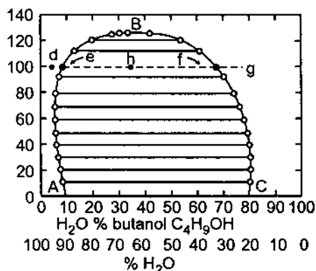
Hình 38.1. Ảnh hưởng của nhiệt độ đến tính tan tương hỗ của hệ n – butanol – nước
