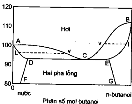
Hình 38.4. Biểu đồ nhiệt độ sôi - thành phần của hệ n -butanol - nước ở 1 atm
