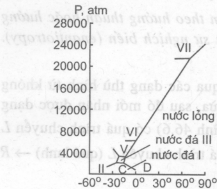
Hình 46.4. Biểu đồ pha của nước ở áp suất cao.
