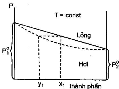
Hình 37.1. Thành phần pha lỏng và pha hơi cân bằng của hỗn hợp hai cấu tử.
