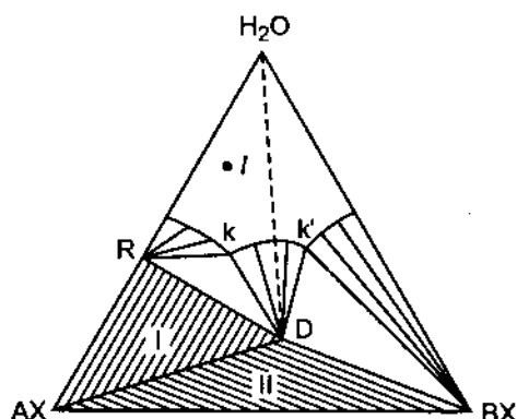
Hình 48.6. Biểu đồ pha tam giác của hệ AX - BX - H_2O tạo thành muối hidrat ( R ) và hợp chất hoá học ( D )
