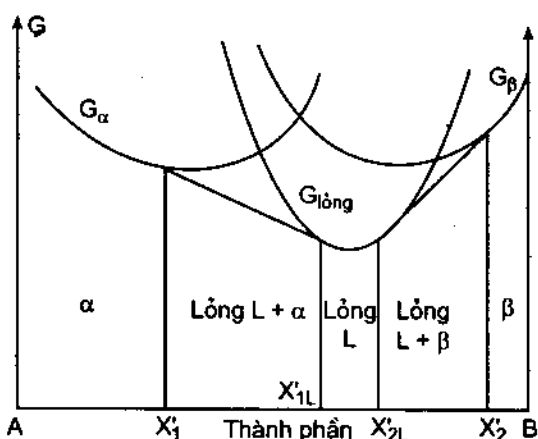
Hình 49.3. Biểu đồ thế đẳng áp của hệ hai cấu tử được biểu diễn trên hình 49.1 tại nhiệt độ T_2 > T_E .
