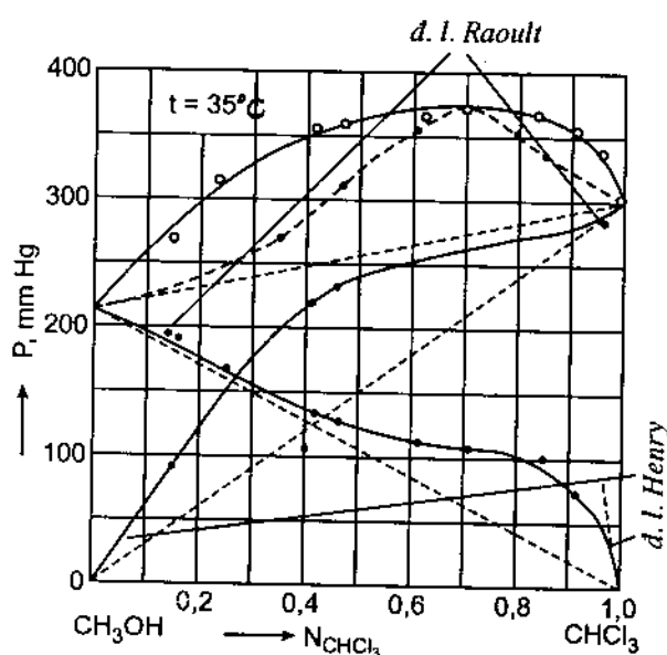
Hình 40.1. Biểu đồ áp suất hơi - thành phần của hệ metanol - cloroform (minh họa vùng áp dụng các định luật Raoult và Henry).
