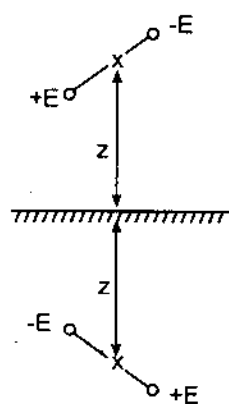
Hình 58.1. Lưỡng cực và ảnh của nó qua bề mặt kim loại
