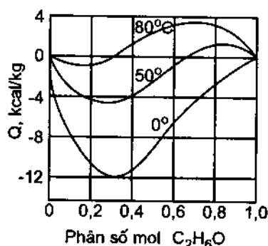
Hình 36.7. Nhiệt hình thành dung dịch \text{C}_2\text{H}_5\text{OH}-\text{H}_2\text{O}
