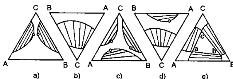
Hình 48.9. Một số trường hợp về tính tan hạn chế của hệ 3 chất lỏng.
