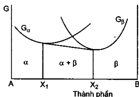
Hình 49.2. Biểu đồ thế đẳng áp của hệ hai cấu tử được biểu diễn trên hình 49.1 tại nhiệt độ T_1 < T_E .
