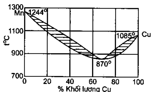
Hình 47.6. Biểu đồ nóng chảy của hệ mangan – đồng có điểm cực tiểu trên đường nóng chảy (kiểu II').
