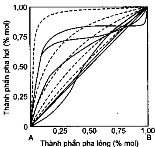
Hình 37.3. Thành phần pha lỏng và pha hơi cân bằng của các hệ khác nhau.
