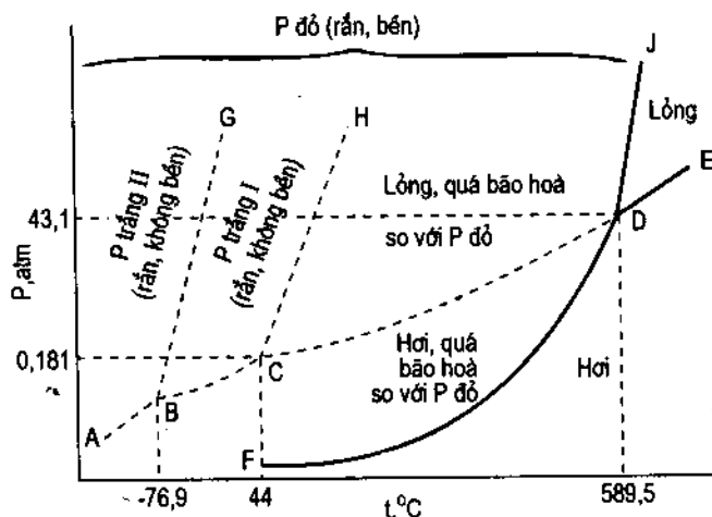
Hình 46.8. Biểu đồ pha của photpho
