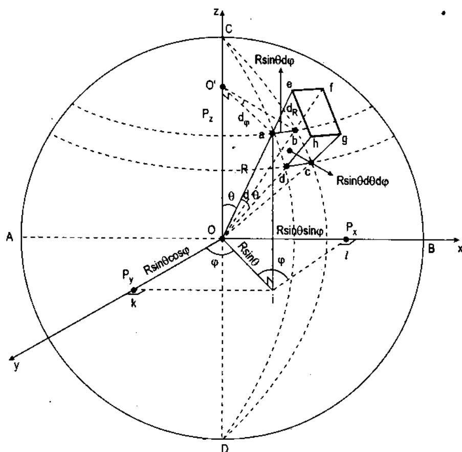
Hình 51.1. Chuyển toạ độ vuông góc thành toạ độ cầu. R – bán kính hình cầu (vector bán kính); \varphi – độ kinh tính từ kinh tuyến đi qua trục y ; \theta – độ vĩ tính từ cực C ; dR = ae ; d\theta = \widehat{aOd} ; d\varphi = \widehat{aOb} ; i – hình chiếu của a trên mặt yOx ; O_i = O'a = R \sin \theta ; ab = R \sin \theta d\varphi ; ad = R d\theta ; p_y = Ok = R \sin \theta \cos \varphi ; p_x = Oi = R \sin \theta \sin \varphi ; p_z = OO' = R \cos \theta ; S(abcd) = ab \times ad = R^2 \sin \theta d\theta d\varphi ; thể tích v(abcdefgh) = Sdr = R^2 \sin \theta d\theta d\varphi dR (toạ độ cầu) = dp_x dp_y dp_z (toạ độ vuông góc).
