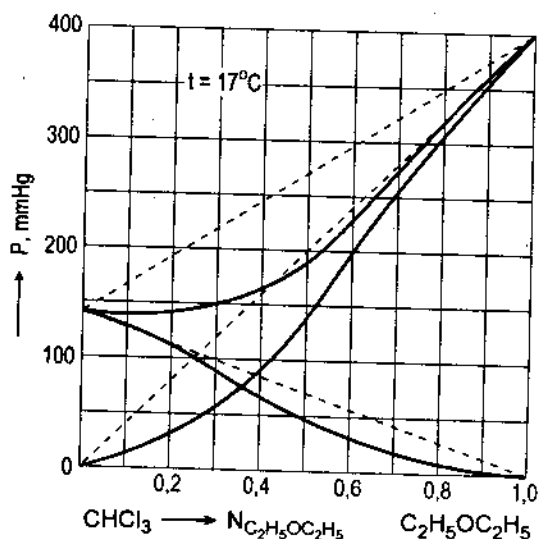
Hình 36.5. Áp suất hơi của dung dịch không lí tưởng (sai lệch âm)
