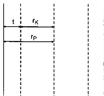
Hình 62.6. Mao quản hình trụ có bán kính Kelvin r_k và bán kính thực r_p .
