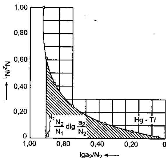
Hình 43.4. Xác định hoạt độ của dung môi (Hg) theo sự phụ thuộc của hoạt độ chất tan (TI) vào nồng độ (ví dụ 3).
