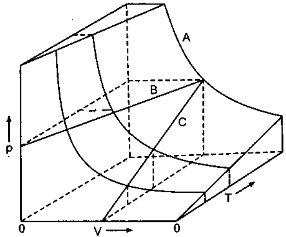
Hình 46.1. Tương quan giữa các biến số P, V, T đối với khí lí tưởng
