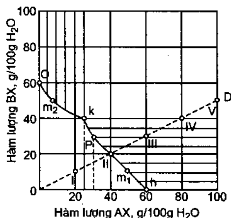
Hình 48.4. Biểu đồ vuông góc của hệ AX - BX - H_2O
