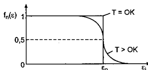
Hình 57.18. Hàm phân bố Fermi – Dirak đối với electron.
