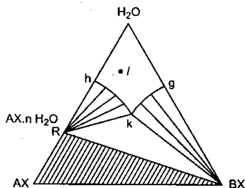
Hình 48.5. Biểu đồ pha tam giác của hệ AX - BX - H_2O tạo thành muối hidrat ( R ) kết tinh
