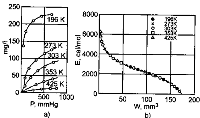
Hình 62.8. Các đường đẳng nhiệt hấp phụ \text{CO}_2 trên than hoạt tính ở các nhiệt độ khác nhau (a) và đường cong đặc trưng tương ứng (b)
