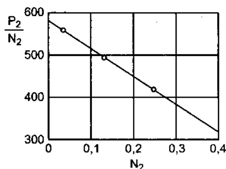
Hình 43.3. Tính hệ số Henry đối với axeton ( K_2 ) trong dung dịch ete – axeton
