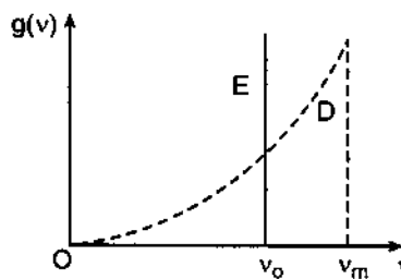
Hình 56.4. Hàm phân bố tần số theo thuyết Einstein (đường đậm E) và theo thuyết Debye (đường chấm chấm D)
