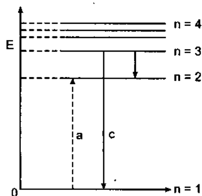
Hình 53.1. Các mức năng lượng electron
