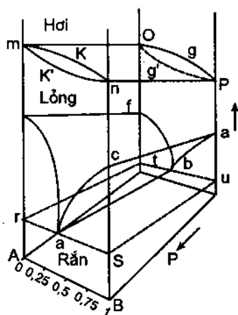
Hình 47.1. Biểu đồ pha thể tích của hệ hai cấu tử có điểm ectecti và không tạo thành dung dịch rắn.
