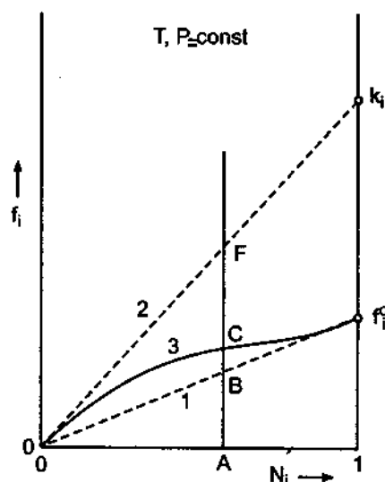
Hình 43.1. Sự phụ thuộc hoạt áp vào nồng độ (1) Theo định luật Raoult (2) Theo định luật Henry (3) Hoạt áp thực.
