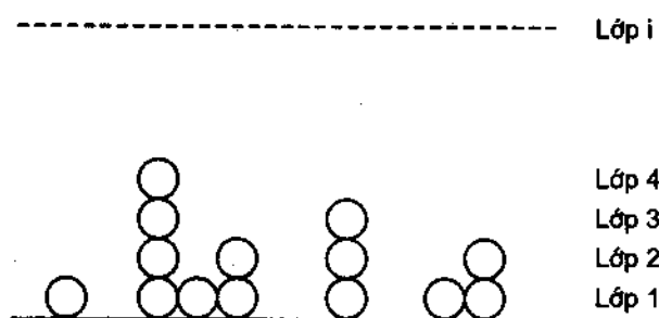
Hình 59.5. Mô hình hấp phụ vật lý nhiều lớp theo lý thuyết BET.
