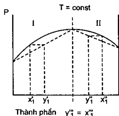
Hình 37.4. Thành phần pha lỏng và pha hơi của dung dịch không lí tưởng có điểm đẳng phí (thành phần y'''_1 = x'''_1 )
