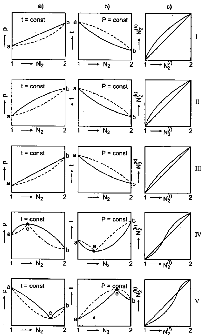
Hình 37.5. Các kiểu biểu đồ cân bằng lỏng - hơi của hệ hai cấu tử
