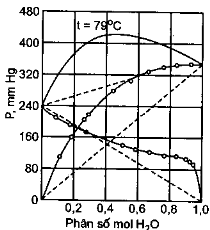
Hình 36.6. Áp suất hơi của dung dịch \text{C}_2\text{H}_5\text{N}-\text{H}_2\text{O}
