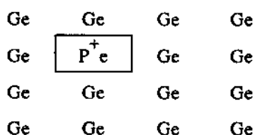
Hình 57.9. Tinh thể gecmani chứa photpho là bán dẫn electron (loại n)
