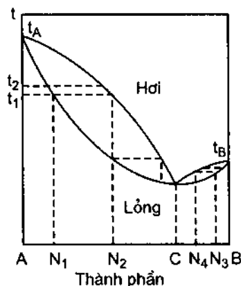
Hình 37.7. Biểu đồ nhiệt độ sôi – thành phần của hệ hai cấu tử có điểm đẳng phí (thành phần c)
