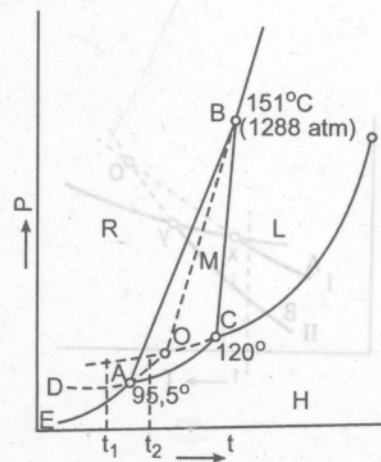
Hình 46.6. Biểu đồ pha của lưu huỳnh.
