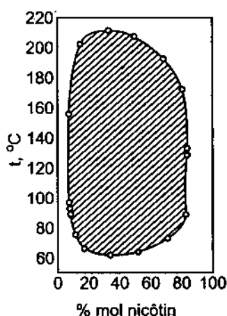
Hình 38.2. Sự hoà tan hạn chế của hệ nicotin – nước.
