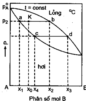
Hình 37.2. Biểu đồ áp suất hơi – thành phần của hệ hai cấu tử.
