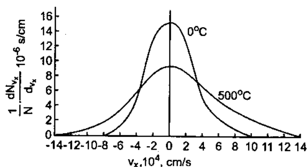
Hình 51.3. Sự phân bố các phân tử nitơ theo một thành phần tốc độ ( v_x ) ở các nhiệt độ khác nhau.
