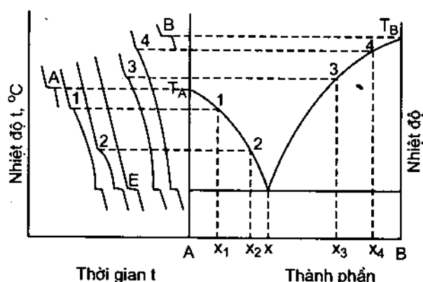
Hình 49.4. Xây dựng biểu đồ nóng chảy bằng phương pháp phân tích nhiệt
