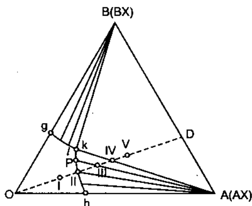
Hình 48.3. Biểu đồ pha tam giác của hệ AX - BX - H_2O
