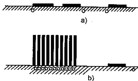
Hình 60.3. Sự định hướng các phân tử hoạt động bề mặt trong lớp hấp phụ (a) – màng khí ; (b) – màng ngưng tụ.
