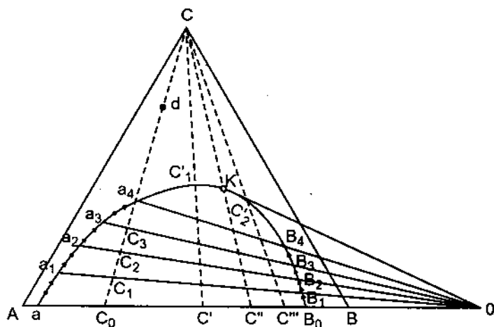
Hình 48.7. Biểu đồ hoà tan của hệ ba chất lỏng A, B và C (A và B hoà tan hạn chế)
