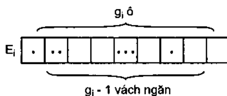
Hình 52.2. Quy luật phân bố Bose – Einstein.
