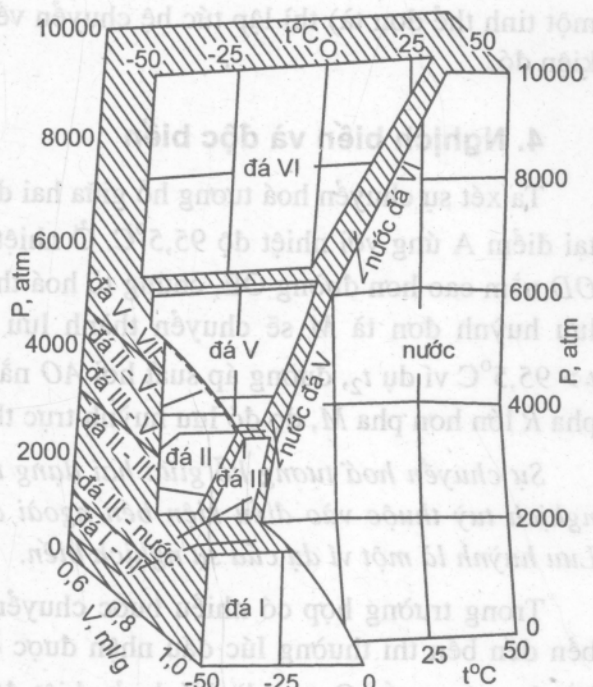
Hình 46.5. Biểu đồ pha (3 chiều) của nước.
