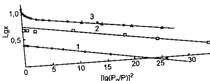
Hình 62.9. Các đường đẳng nhiệt hấp phụ benzen và nitơ trên than hoạt tính theo tọa độ của phương trình Dubinin; 1, 2. hấp phụ benzen ở 20°C trên hai loại than hoạt tính khác nhau; 3. hấp phụ nitơ ở -195°C trên than hoạt tính, x biểu diễn bằng mmol/g.
