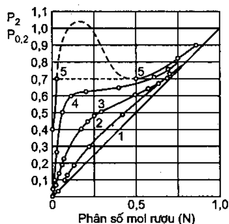
Hình 38.3. Áp suất hơi tương đối của các rượu khác nhau trên dung dịch nước ở 25^{\circ}\text{C} 1. dung dịch lí tưởng ; 2. metanol ; 3. etanol ; 4. propanol ; 5. butanol.
