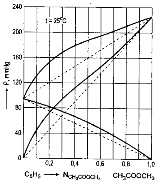
Hình 36.4. Áp suất hơi của dung dịch không lí tưởng (sai lệch dương)
