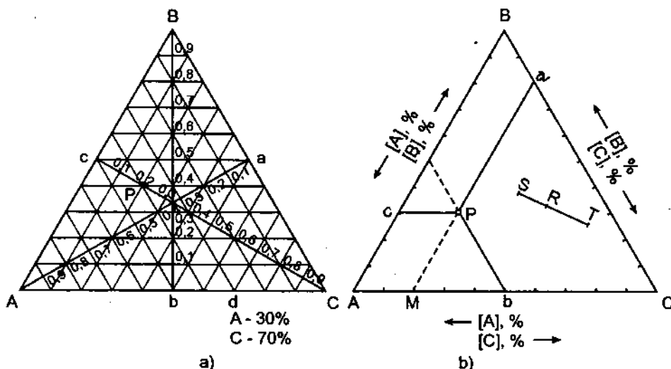
Hình 48.1. Biểu diễn thành phần của hệ ba cấu tử bằng biểu đồ tam giác.
