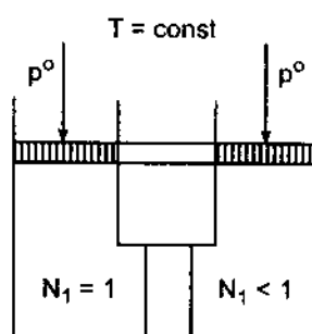
Hình 42.1. Màng bán thấm và áp suất thẩm thấu.
