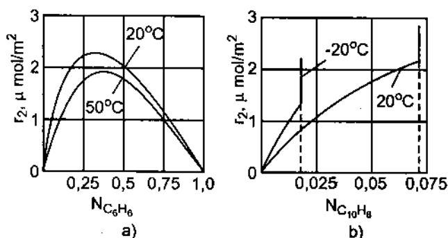
Hình 61.3. Ảnh hưởng của nhiệt độ đến sự hấp phụ trong dung dịch hai cấu tử; (a) Sự hấp phụ của benzen trong dung môi n -hexan (hoà tan hoàn toàn) trên bề mặt \text{SiO}_2 ; (b) Sự hấp phụ của naphthalen trong dung môi n -heptan (hoà tan hạn chế) trên bề mặt \text{SiO}_2 .
