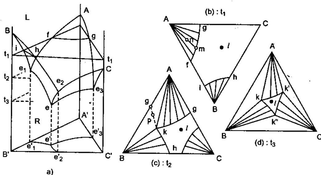
Hình 48.2. Hệ 3 cấu tử không tạo thành dung dịch rắn có điểm etecti bậc 3.
