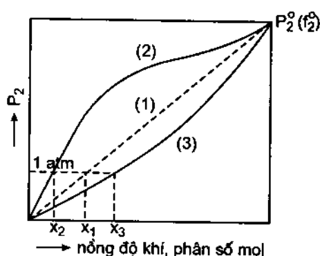
Hình 40.2. Áp suất hơi trên dung dịch lí tưởng (1), sai lệch dương (2) và sai lệch âm (3)
