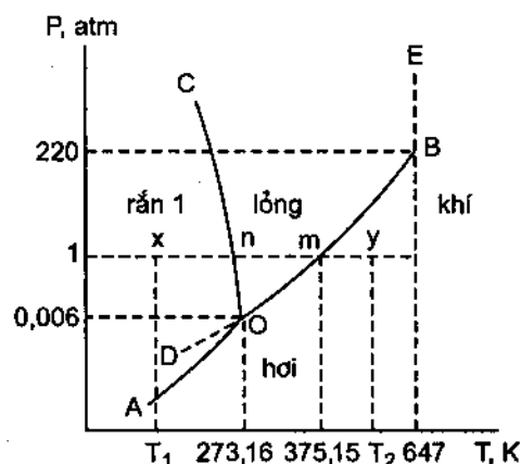
Hình 46.3. Biểu đồ pha (2 chiều) của nước ở vùng áp suất trung bình.
