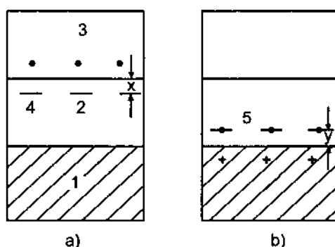
Hình 57.17. Sơ đồ vùng bán dẫn chứa tạp chất cho (a) và nhận (b)
