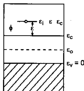
Hình 57.19. Kí hiệu các mức năng lượng :
