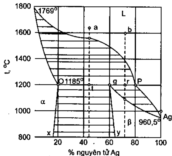
Hình 47.8. Biểu đồ nóng chảy của hệ platin – bạc hoà tan hạn chế ở pha rắn (kiểu III')
