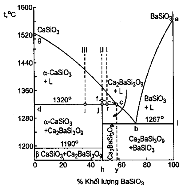
Hình 47.11. Biểu đồ nóng chảy của hệ \text{CaSiO}_3 – \text{BaSiO}_3 tạo thành hợp chất hoá học nóng chảy không toàn đẳng (kiểu V)
