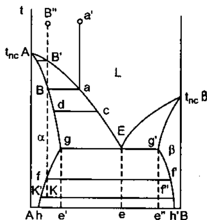
Hình 47.7. Biểu đồ nóng chảy của hệ hai cấu tử hoà tan hạn chế ở pha rắn (kiểu III)
