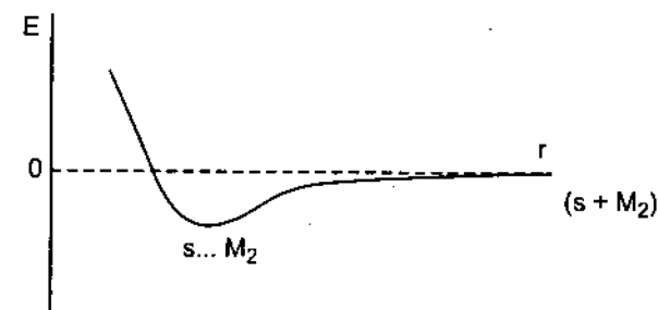
Hình 58.4. Sự hấp phụ vật lí phân tử M_2 trên bề mặt S, E – thế năng, r – khoảng cách.
