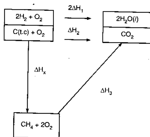
Hình 7-2. Sơ đồ xác định nhiệt tạo thành khí metan.
