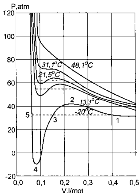
Hình 24-4. Các đường đẳng nhiệt P-V của \text{CO}_2 xây dựng theo phương trình (24.7) với các hằng số a = 3,591^2 \text{ atm/mol}^2 , b = 0,04271/\text{mol} .
