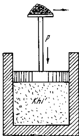
Hình 6-4. Sơ đồ thực hiện công giãn nở khí đoạn nhiệt.
