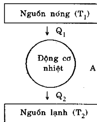
Hình 12-1. Sơ đồ chuyển nhiệt thành công trong động cơ nhiệt làm việc giữa hai nguồn nhiệt.
