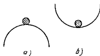
Hình 21.1 Ví dụ về cân bằng cơ học không bền (a) và bền (b).
