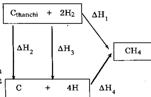
Hình 7-3. Sơ đồ tính sinh nhiệt nguyên tử của metan.
