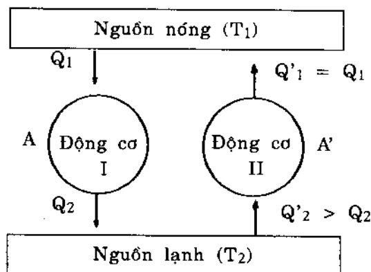
Hình 12-3. Sơ đồ chứng minh định lý Carnot thứ nhất.
