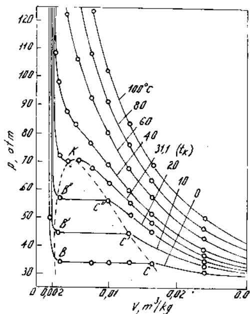
Hình 24.3 Các đường đẳng nhiệt V - P của CO 2 theo các dữ kiện thực nghiệm.
