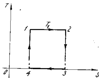
Hình 32-1. Chu trình Carnot biểu diễn trên hệ tọa độ T - S
