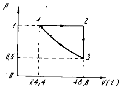
Hình 7-8. Chu trình thuận nghịch trong bài tập 16.
