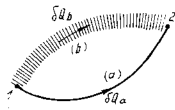
Hình 14-2 Sơ đồ biểu diễn quá trình thuận nghịch (a) và không thuận nghịch (b)
