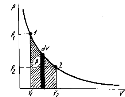
Hình 6-2. Biểu diễn bằng đồ thị công giãn nở đẳng nhiệt khí lí tưởng (diện tích gạch chéo)
