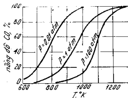
Hình 25-1 Nồng độ cân bằng của CO trong phản ứng C + CO_2 = 2CO
