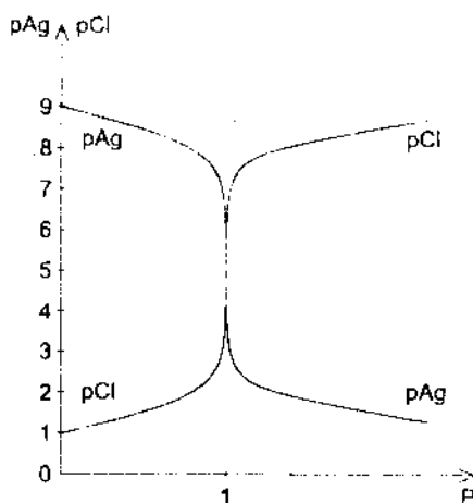
Hình 8.1. Đường chuẩn độ NaCl 0.1 M bằng AgNO_3 0.1 M
