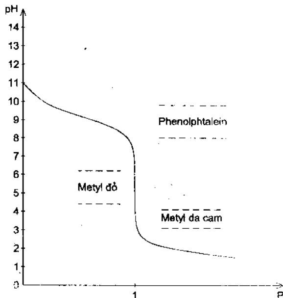
Hình 6.4. Đường chuẩn độ dung dịch NH_3 bằng HCl C \approx C_o = 0,100M
