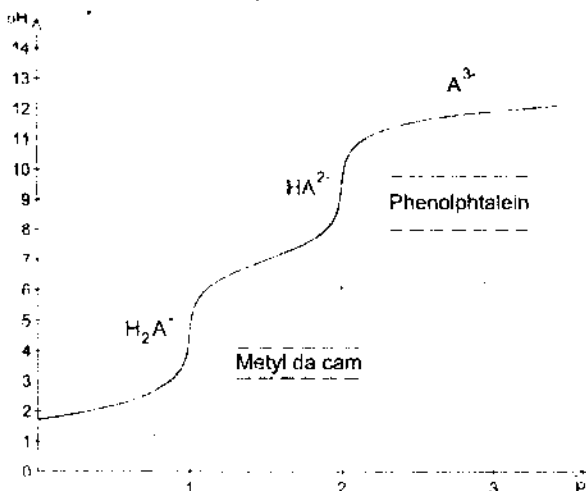
Hình 6.8. Đường chuẩn độ axit H_3A 0,100M bằng XOH 0,100M pK_{a1} = 2,00 ; pK_{a2} = 7,00 ; pK_{a3} = 12,00
