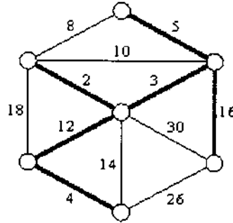
Hình 3. Cây khung nhỏ nhất của đồ thị
