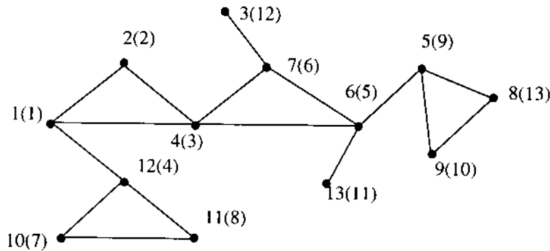
Hình 2. Chỉ số mới (trong ngoặc) của các đỉnh được đánh lại theo thứ tự chúng được thăm trong thuật toán tìm kiếm theo chiều sâu
