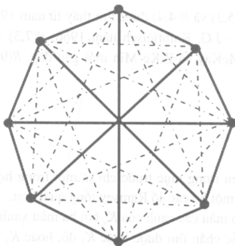
Hình 2. Tô màu K_8
