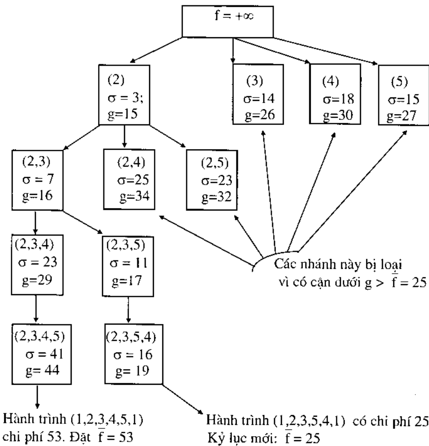
Hình 2. Giải bài toán người du lịch
