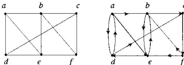
Hình 1. Đường đi trên đồ thị
