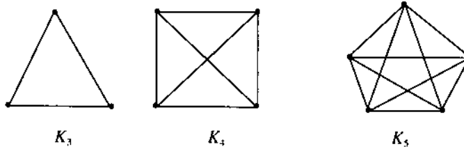
Hình 1. Đồ thị đầy đủ
