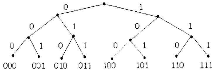
Hình 2. Cây liệt kê dãy nhị phân độ dài 3
