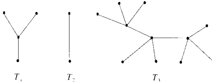
Hình 1. Rừng gồm ba cây T_1, T_2, T_3
