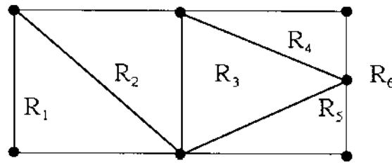
Hình 7. Các miền tương ứng với biểu diễn phẳng của đồ thị
