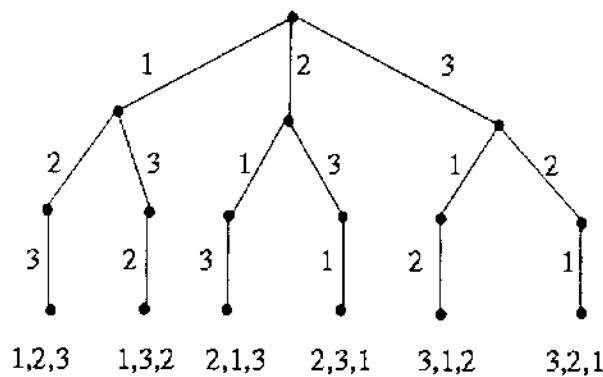
Hình 3. Cây liệt kê các hoán vị của 1, 2, 3.
