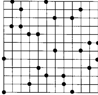
Hình 3. Một lời giải bài toán của bài toán với n = 12
