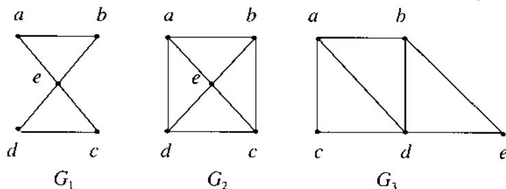
Hình 1. Đồ thị G_1, G_2, G_3
