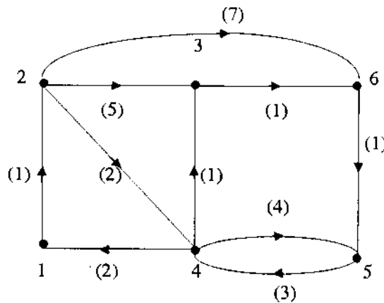
Hình 2. Minh họa thuật toán Dijkstra
