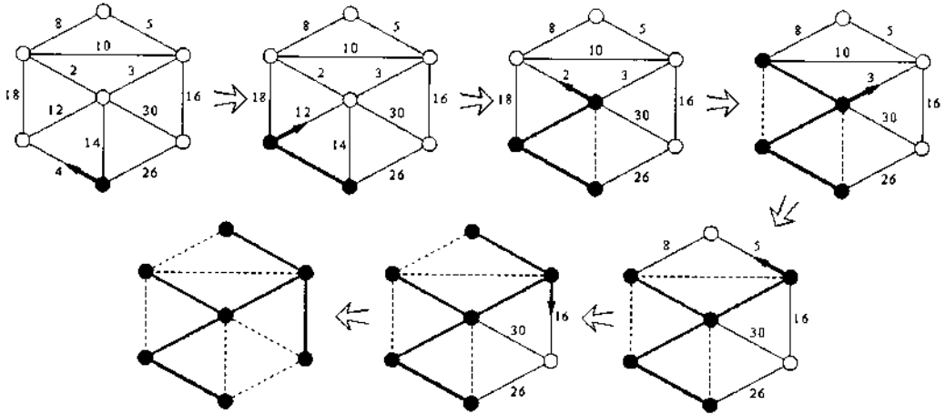
Hình 6. Tìm cây khung theo thuật toán Prim
