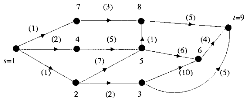
Hình 3. Đồ thị không có chu trình
