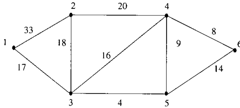
Hình 4. Đồ thị có trọng số
