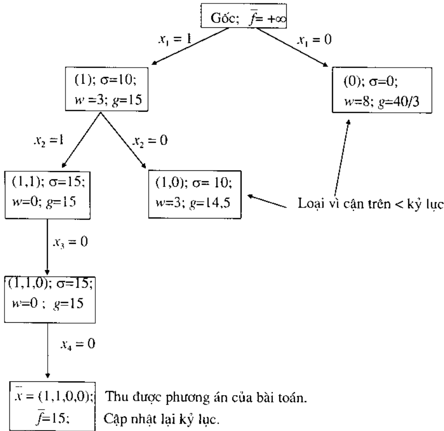
Hình 1. Giải bài toán cái túi bằng thuật toán nhánh cận
