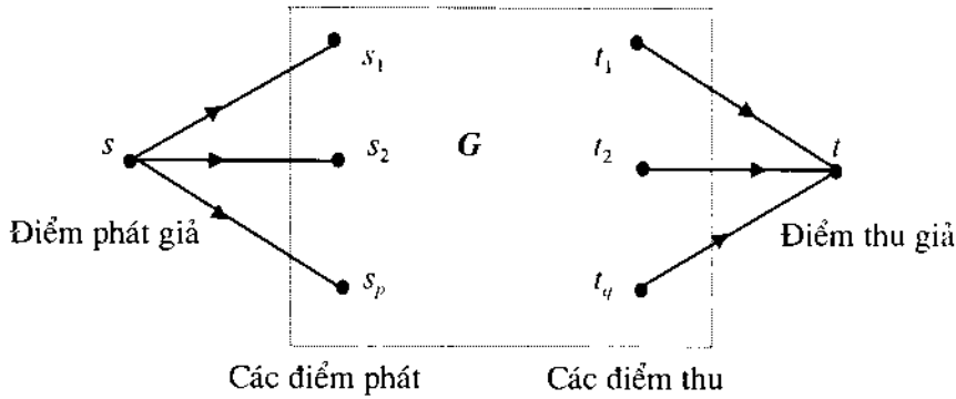
Hình 4. Mạng với nhiều điểm phát và thu
