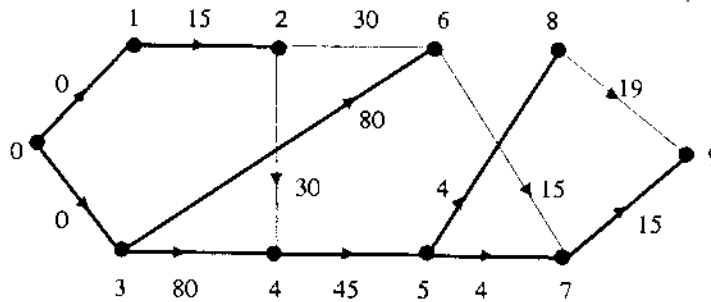
Hình 4. Đồ thị minh họa PERT
