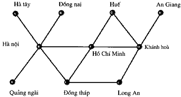
Hình 1. Sơ đồ mạng máy tính
