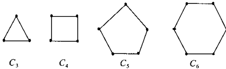
Hình 2. Đồ thị vòng C_3, C_4, C_5, C_6
