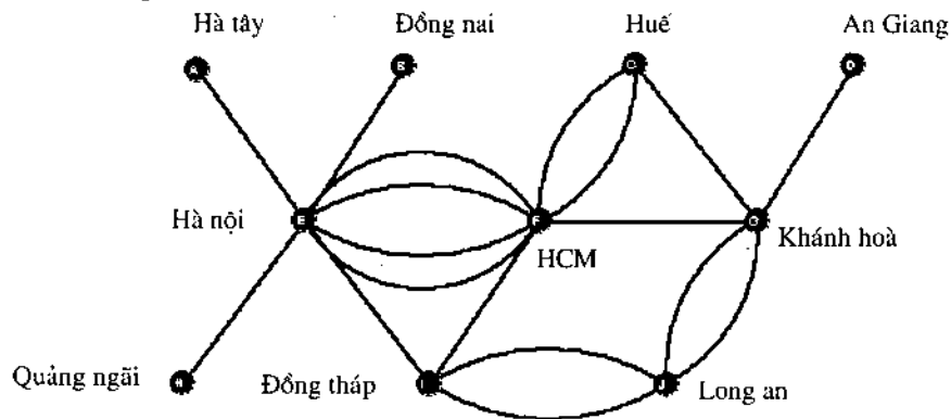
Hình 2. Sơ đồ mạng máy tính với đa kênh thoại
