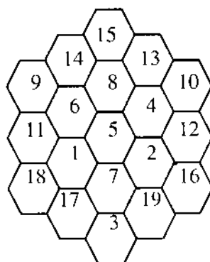
Hình 2. Hình lục giác thần bí
