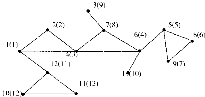
Hình 1. Chỉ số mới (trong ngoặc) của các đỉnh được đánh lại theo thứ tự chúng được thăm trong thuật toán tìm kiếm theo chiều sâu
