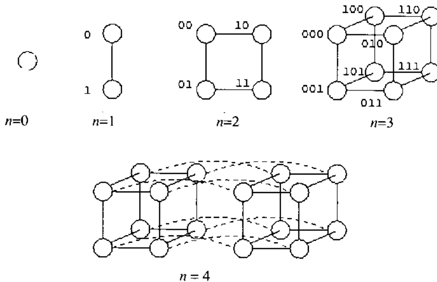
Hình 4. Đồ thị lập phương Q_n
