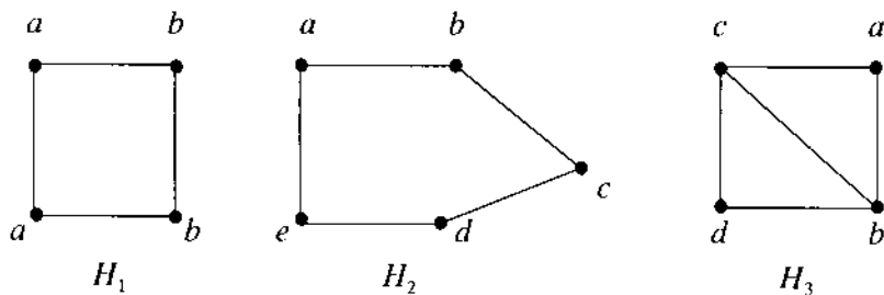
Hình 2. Đồ thị H_1, H_2, H_3
