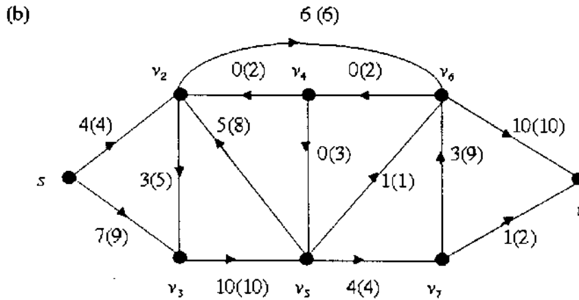
Hình 3. Tăng luồng dọc theo đường tăng
