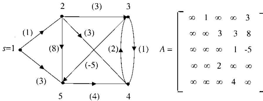
Hình 1. Minh hoạ cho thuật toán Ford - Bellman
