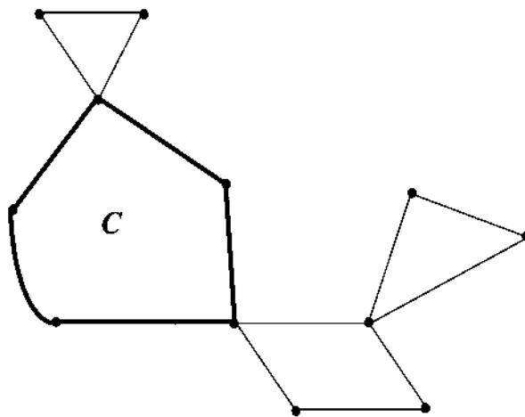
Hình 3. Minh hoạ cho chứng minh định lý 1
