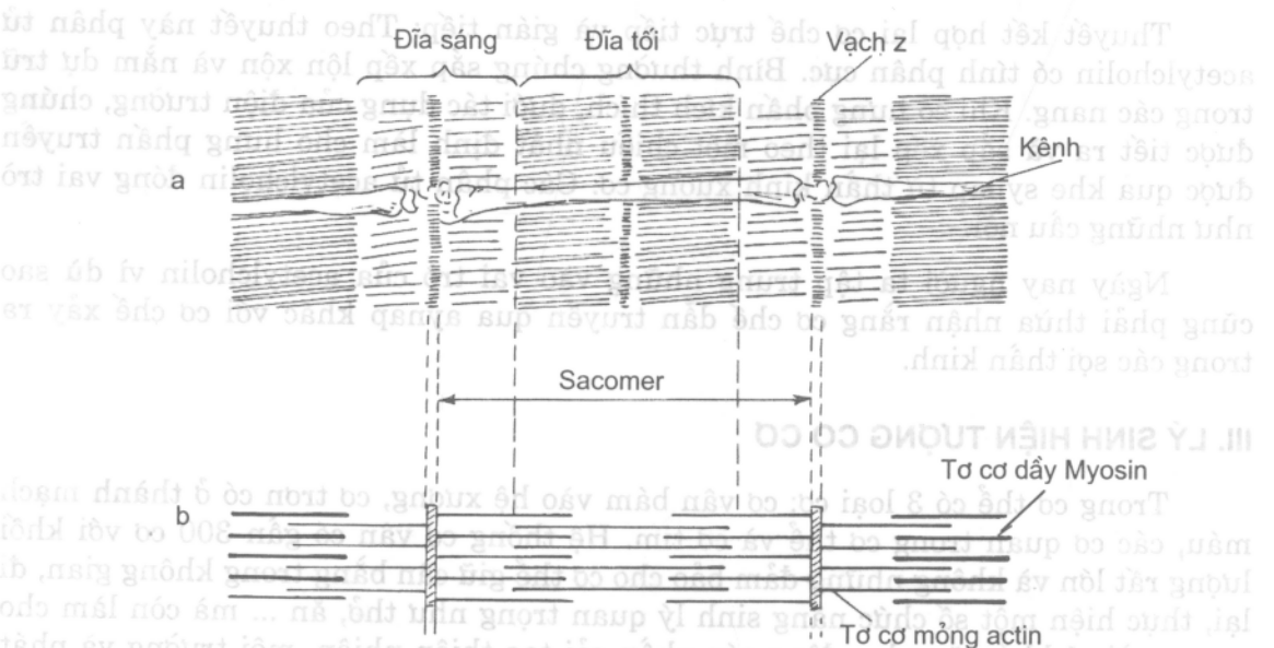
Hình 3.3.2. Hình ảnh cấu trúc Sacomer của cơ trên kính hiển vi điện tử
