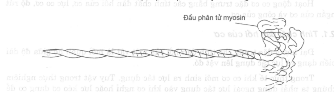
Hình 3.3.5. Cấu trúc không gian của phân tử myosin
