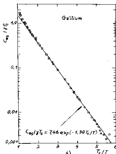
Hình 9.7. Phụ thuộc C_0/\gamma T_c = 7,46 \exp(-1,39T_c/T) của Gali.
