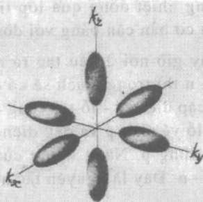
Hình 8.10. Mặt đẳng năng ellipsoid trong Si với m_l/m_t = 5.5
