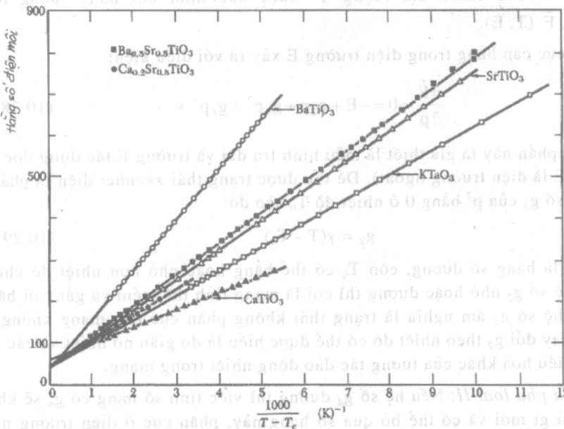
Hình 10.15. Hằng số điện môi theo 1/(T - T_C) ở trạng thái thuận điện T > T_C của perovskite (Theo G. Rupprecht và R.O.Bell).
