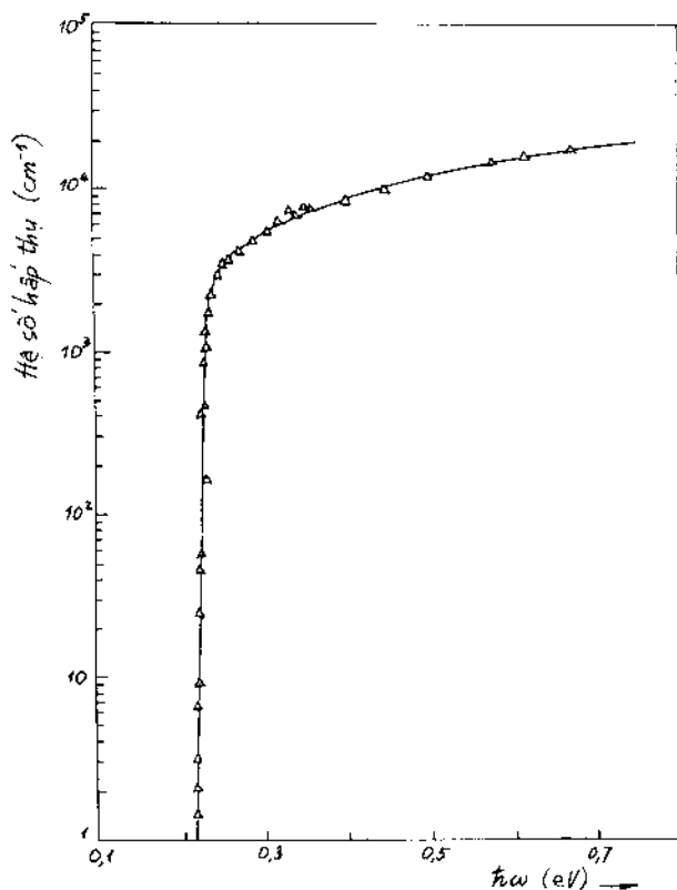
Hình 8.5. Phổ hấp thụ của InSb, quá trình trực tiếp.
