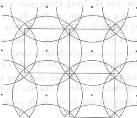
Hình 7.6. Xác định vùng Brillouin theo Harisson cho mạng hai chiều.
