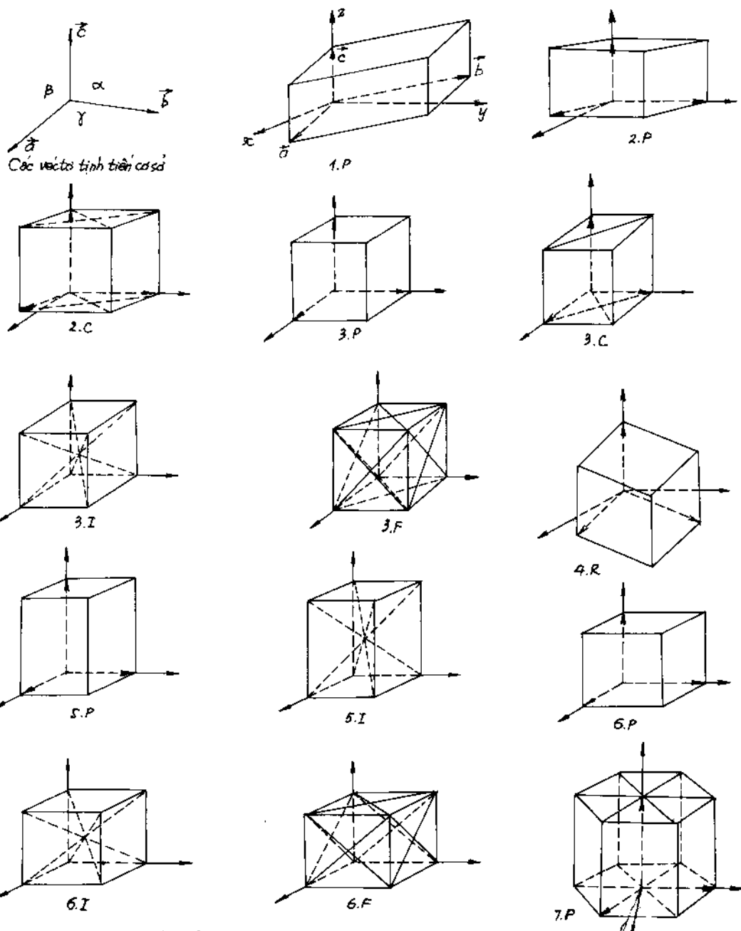
Hình 1.5. Mười bốn kiểu mạng Bravais 3 chiều trong hệ trục tọa độ Đề các, trục tọa độ x, y, z có mũi tên đậm, các vectơ tịnh tiến cơ sở có mũi tên mảnh, tại các nút giao nhau của các đường có cơ sở là 1 nguyên tử (số thứ tự và kí hiệu mạng như bảng trên).
