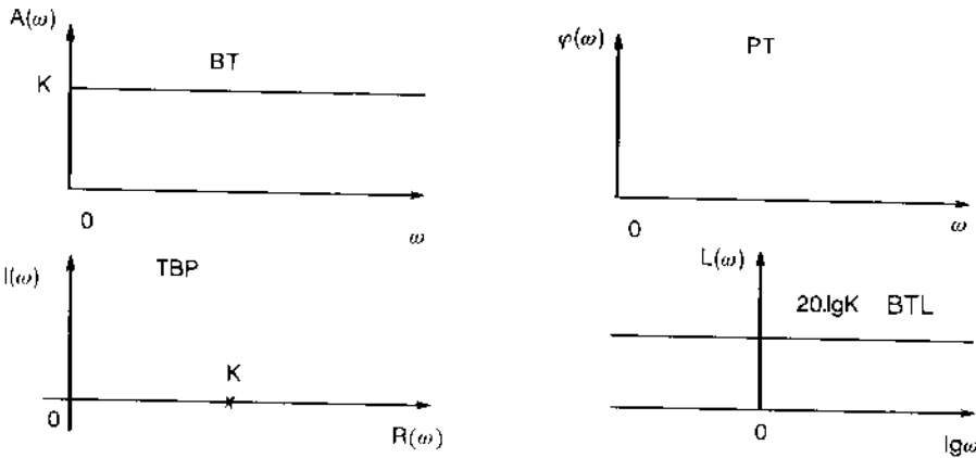
Hình 1-6 Các đặc tính tần số của khâu khuếch đại
