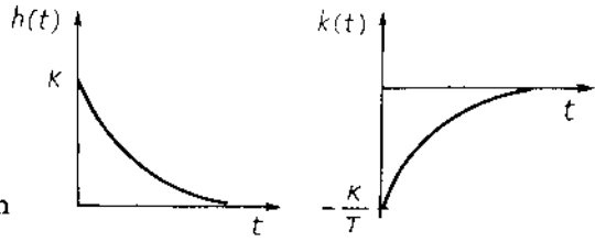
Hình 1-29 Các đặc tính thời gian của khâu vi phân thực
