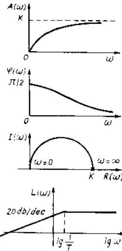
Hình 1-30 Các đặc tính tần số
