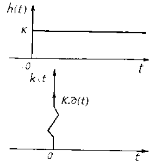
Hình 1-5 Các đặc tính thời gian của khâu khuếch đại
