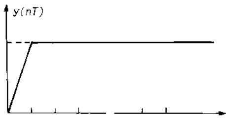
Hình II-23 Quá trình quá độ trong hệ thống tối ưu tác động nhanh
