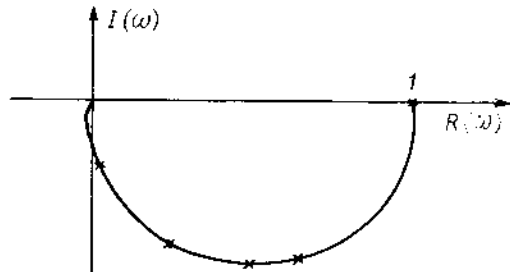
Hình II-4 Đặc tính TBP của W_m(j\omega)/T và của hệ xung hờ
