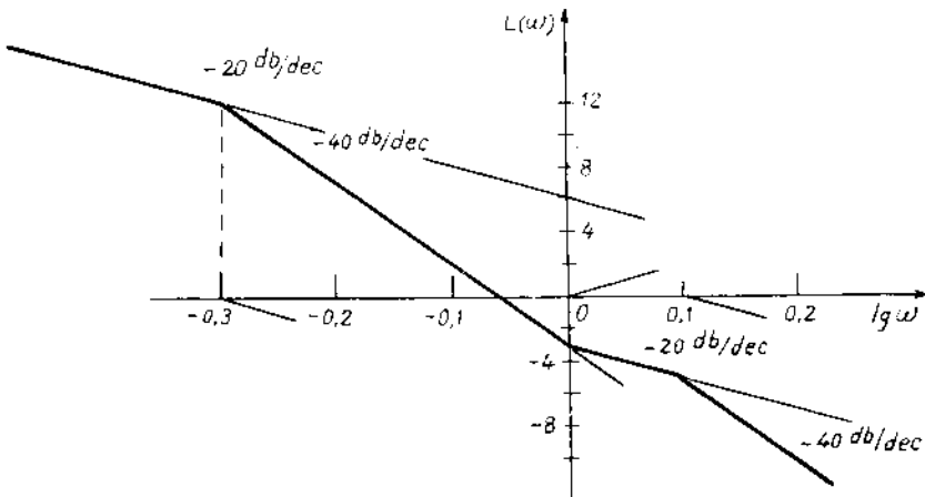
Hình 1-56 Đặc tính BTL (bài 1-2)
