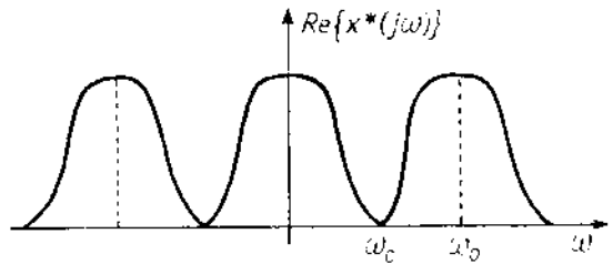
Hình I-8 Phổ của tín hiệu rời rạc khi bảo đảm điều kiện lượng tử hóa của Cachenhicốp
