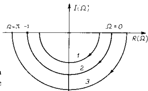
Hình 11-18a Đặc tính TBP của hệ thống hở
