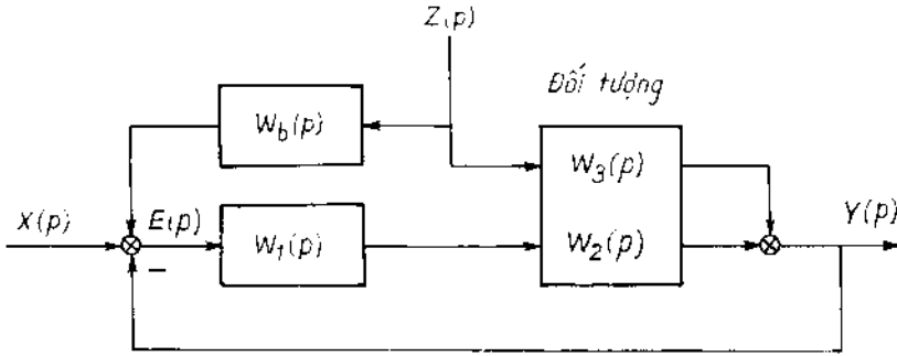
Hình III-21 Xây dựng hệ thống bất biến với nhiễu phụ tải
