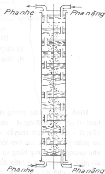
Hình XI.24. Tháp lưới
