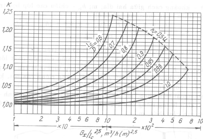
Hình IX.22. Sự phụ thuộc của hệ số K vào tỉ số giữa chiều dài của chảy tràn l_c với đường kính tháp D và tỉ số G_x/l_c^{2.5}
