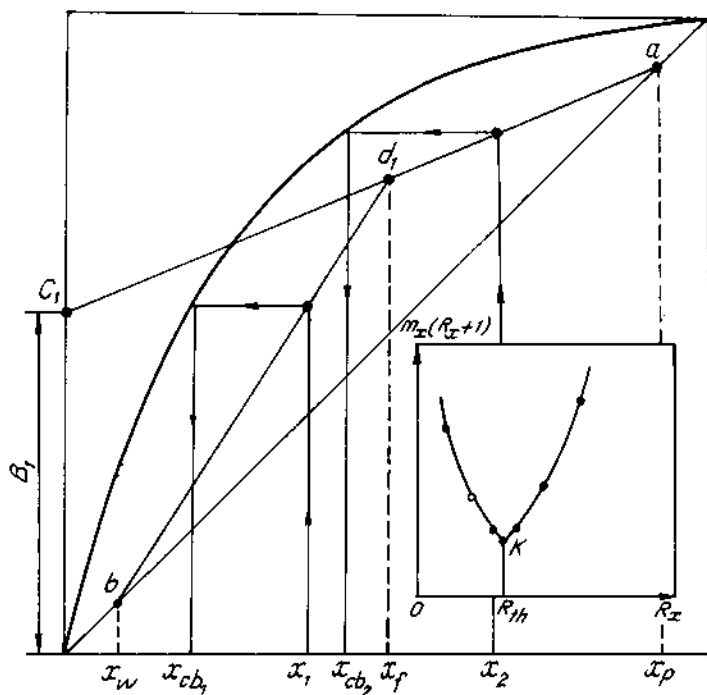
Hình IX.4. Đồ xác định chỉ số hồi lưu thích hợp
