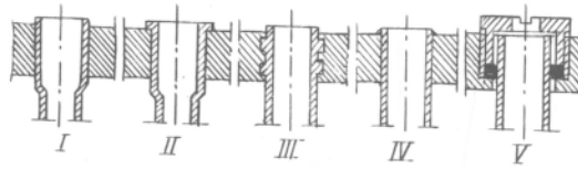
Hình V.28. Cách lắp ống vào mang ống I, II, III- nong ống; IV - hàn; V - ghép bằng ô đệm
