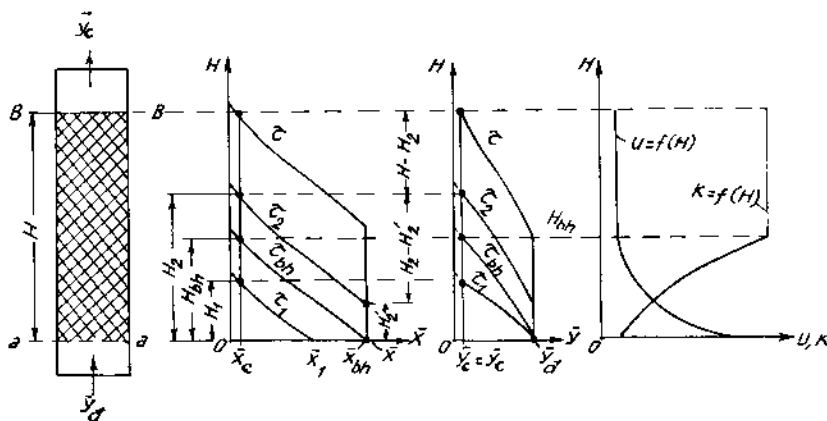
Hình X.4. Sơ đồ của quá trình và trường nồng độ trong lớp chất hấp phụ đứng yên
