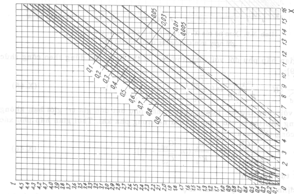
Hình X.7. Quan hệ của t và X khi P = 3 . Các giá trị của \bar{C}_{yc}/\bar{C}_{yd} ghi ngay trên các đường cong của đồ thị
