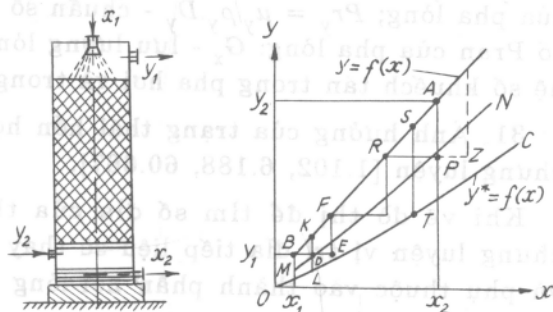
Hình IX.15. Xác định số đơn vị chuyển khối theo số đơn vị thể tích (quá trình hấp thụ)
