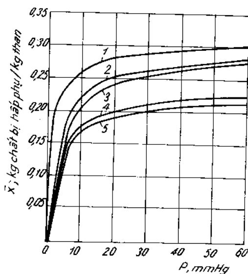
Hình X.1. Đường đẳng nhiệt hấp phụ đối với than hoạt tính: 1- benzen; 2- rượu etylic; 3- rượu etylic ở 25°C; 4- rượu etylic (70%) + ete dietylic 30% ở 20°C; 5- ete dietylic ở 20°C
