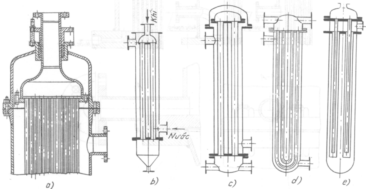
Hình V.33. Các phương pháp dẫn nở tự do:
