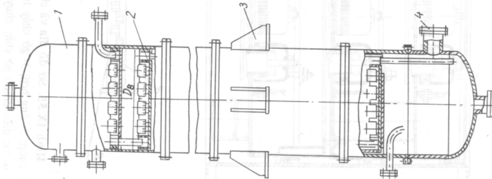
Hình IX.52. Tháp chóp tròn: 1- vỏ; 2- đĩa; 3- tái đun; 4- cửa
