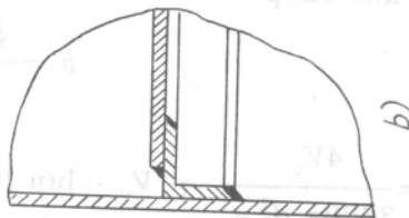
Hình IX.60. Một số phương pháp lắp đĩa và ống cháy chuyển: a) kết cấu giá đỡ đĩa nhỏ thanh trụ; b) ghép chặt đĩa với vành; c) kết cấu đĩa nằm giữa hai mặt bích; d) ghép bằng đệm trung gian; e) ghép bằng kim thủy lực.
