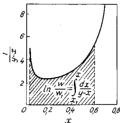
Hình IX.30. Đồ xác định lượng sản phẩm đáy
