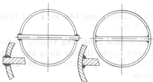
Hình V.38. Chia ngăn dọc phía ngoài
