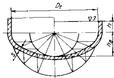
Hình XIII.11. Quan hệ kích thước đáy elip: h_0 = 0,25 D_1 nhưng không bé hơn 0,2 D_1 ; đối với đáy bằng thép cán h \geq 2S , nhưng không bé hơn 25mm
