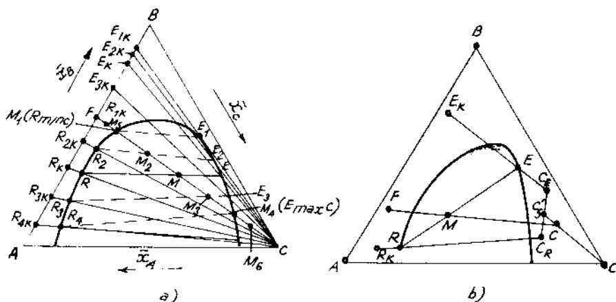
Hình XI.9. Trích ly một bậc trên đồ thị tam giác
