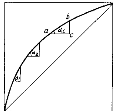
Hình IX.10. Xác định hệ số phân bố m
