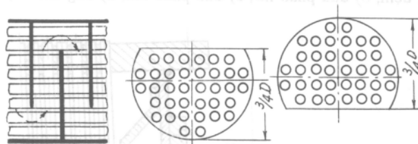
Hình V.36. Ngăn hình viên phân
