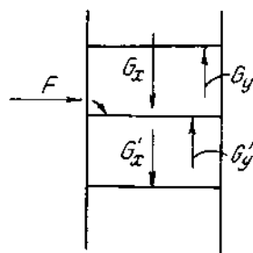
Hình IX.17. Đề thành lập phương trình cân bằng nhiệt lượng của đĩa tiếp liệu
