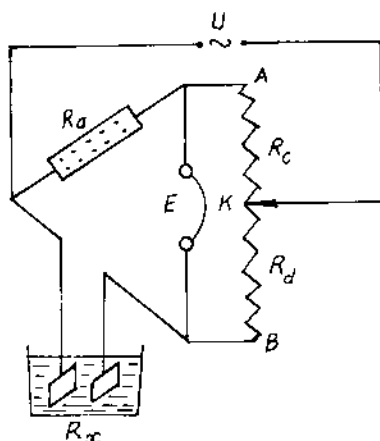
Hình 10-3. Sơ đồ đo điện trở dây dẫn loại 2 theo nguyên tắc cầu Wheastone :
