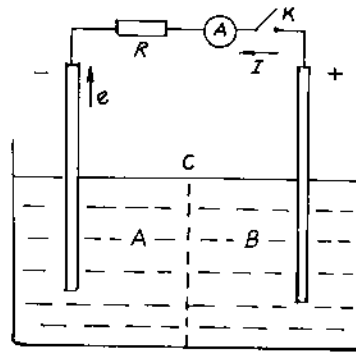
Hình 11-1. Sơ đồ cấu tạo pin hoá học.
