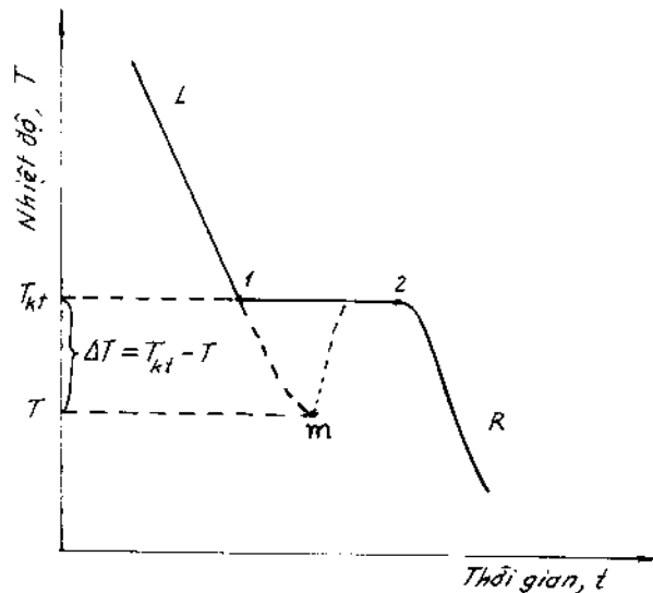
Hình 8-7. Biến thiên nhiệt độ trong quá trình kết tinh.
