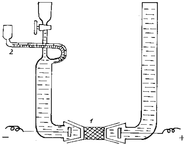
Hình 13-13. Sơ đồ dụng cụ đo \xi bằng hiệu ứng điện thẩm.
