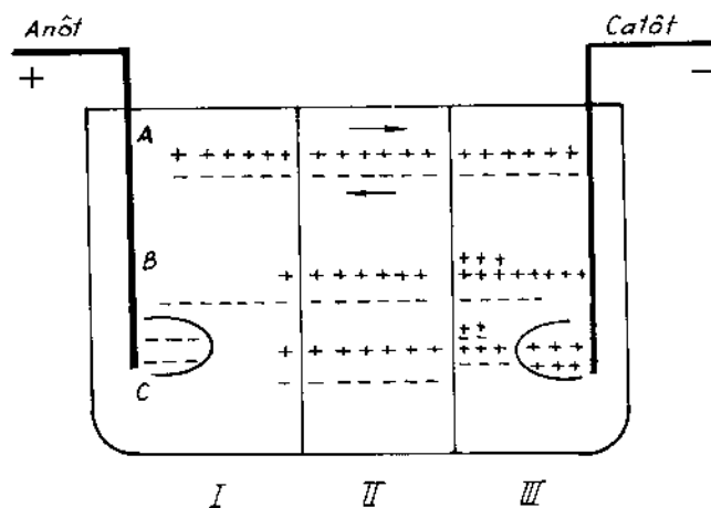
Hình 10-8. Sơ đồ chuyển dịch điện tích của các ion (xác định số chuyển vận theo phương pháp Hittorf).
