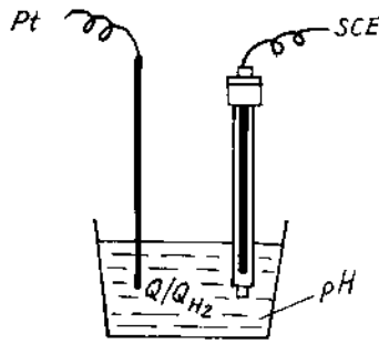
Hình 11-12. Đo pH theo điện cực quinhydron và calomen chuẩn (SCE):
