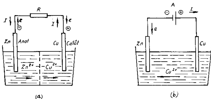
Hình 12-1. Sơ đồ của pin (a) và của bình điện phân (b):
