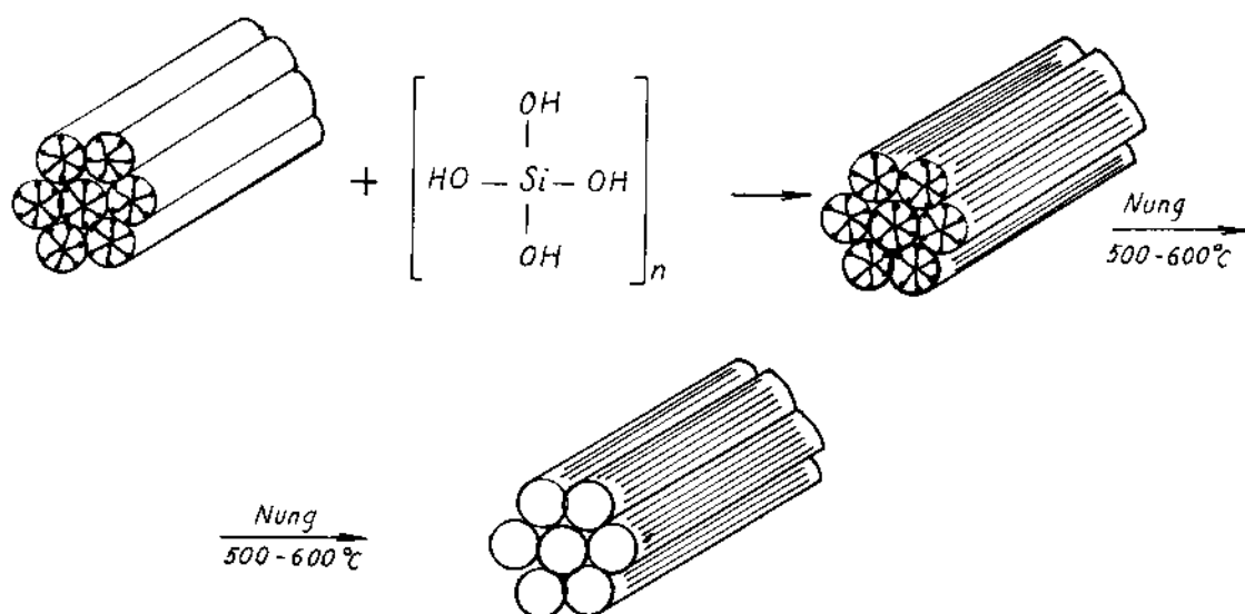
Hình 14-11. Sơ đồ chế tạo vật liệu vô cơ mao quản rộng.
