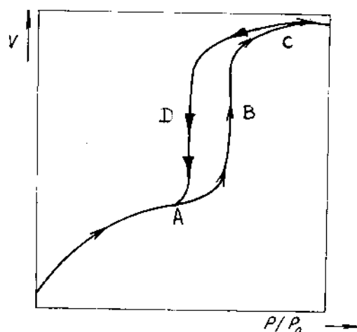
Hình 6-6: Đường hấp phụ (→) và khử hấp phụ (↔) của vật liệu mao quản trung bình.
