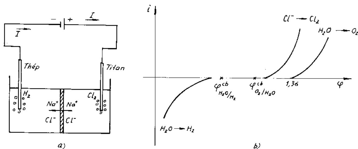
Hình 12-11. (a) Bình điện phân.
