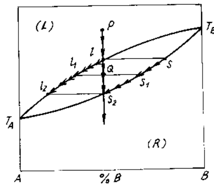
Hình 4-19. Biểu đồ đẳng áp (T - C) của hệ hai cấu tử không tạo thành hợp chất hoá học nhưng tạo thành dung dịch rắn.
