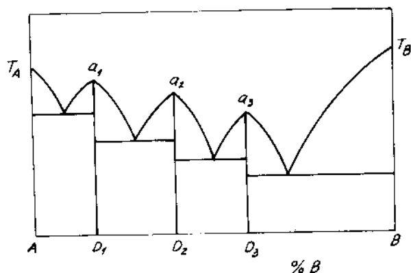
Hình 4-17. Biểu đồ đẳng áp (T - C) của hệ có nhiều hợp chất hoá học bền.
