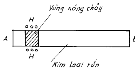
Hình 5-21. Sơ đồ nóng chảy vùng.
