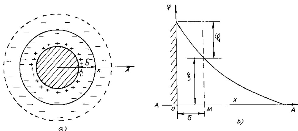
Hình 13-10. Sơ đồ cấu tạo hạt keo (a).
