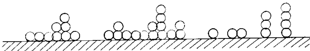
Hình 6-3: Sơ đồ hấp phụ đa lớp (phân tử) theo lý thuyết BET.
