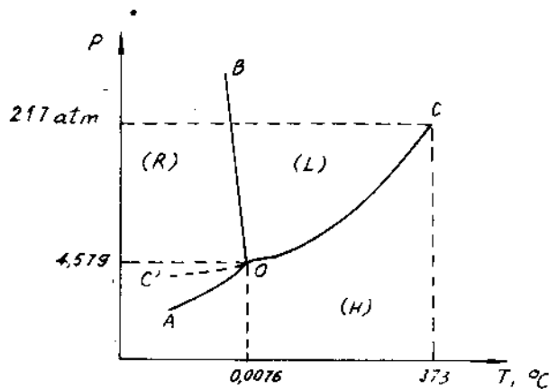
Hình 4-3. Biểu đồ trạng thái ( P - T ) của H_2O ở áp suất thấp.
