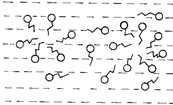
Hình 14-5. Dung dịch đẳng hướng.
