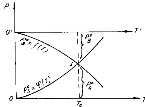
Hình 5-14. Đồ thị dùng để minh họa cách xác định nhiệt độ sôi của hệ hai chất lỏng hoàn toàn không tan lẫn.
