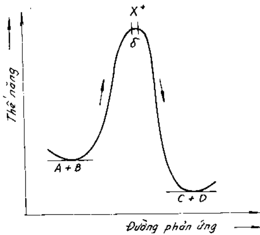
Hình 7-11. Biến thiên thế năng của hệ.
