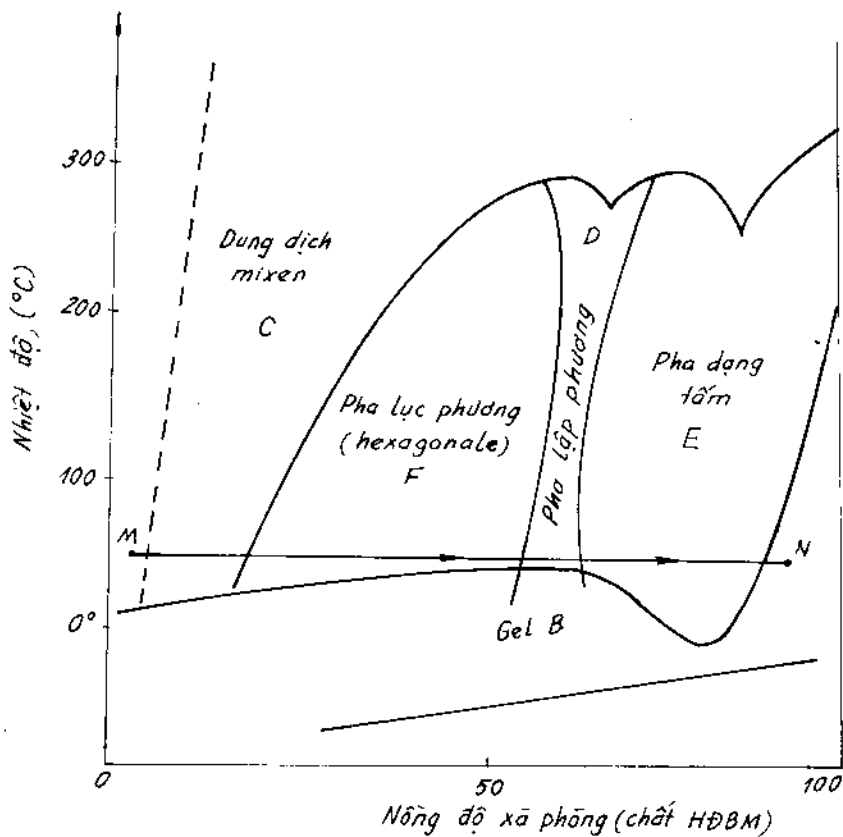
Hình 14-8. Biểu đồ pha của hệ "nước - xà phòng kali".
