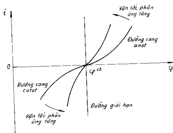
Hình 12-3. Các đường cong phân cực nhanh.
