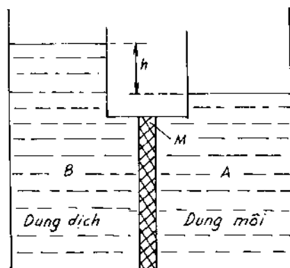
Hình 13-7. Sơ đồ thẩm thấu:
