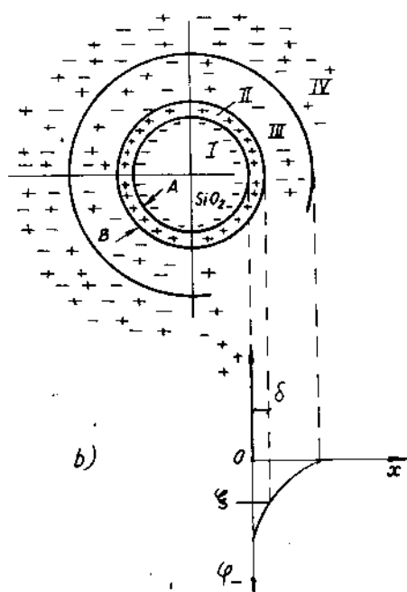
Hình 13-1. Sơ đồ cấu tạo mixen minh hoạ bằng công thức (a) và minh hoạ bằng hình vẽ (b):
