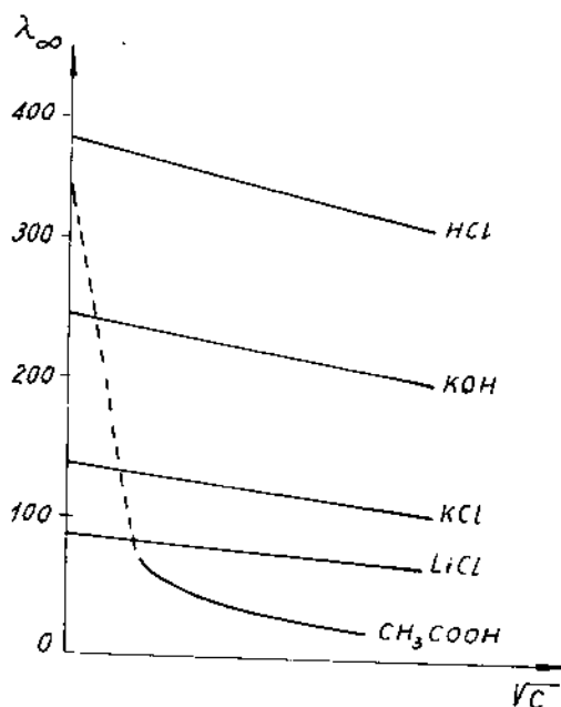
Hình 10-6. Sự phụ thuộc của \lambda vào nồng độ (\sqrt{C}) , (\text{đlg.l}^{-1})^{1/2} .
