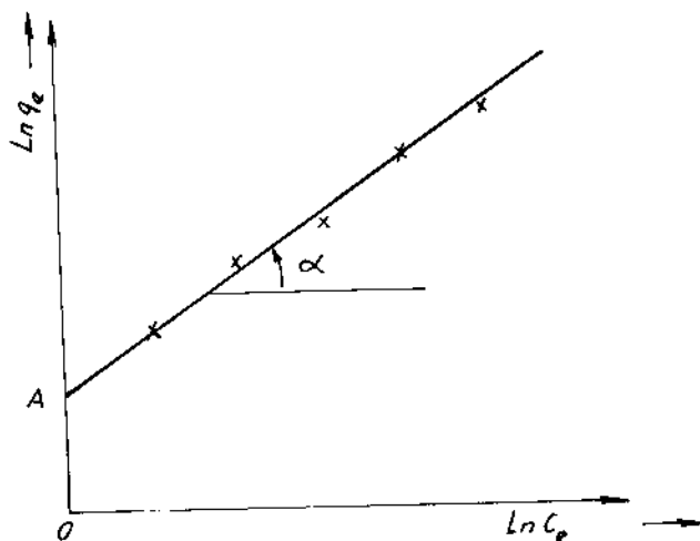
Hình 6-12. Đồ thị Freundlich .
