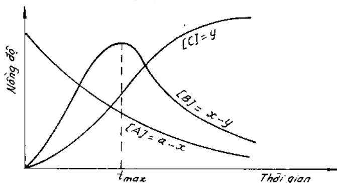
Hình 7-3. Biến thiên nồng độ của các chất trong phản ứng nối tiếp theo thời gian.
