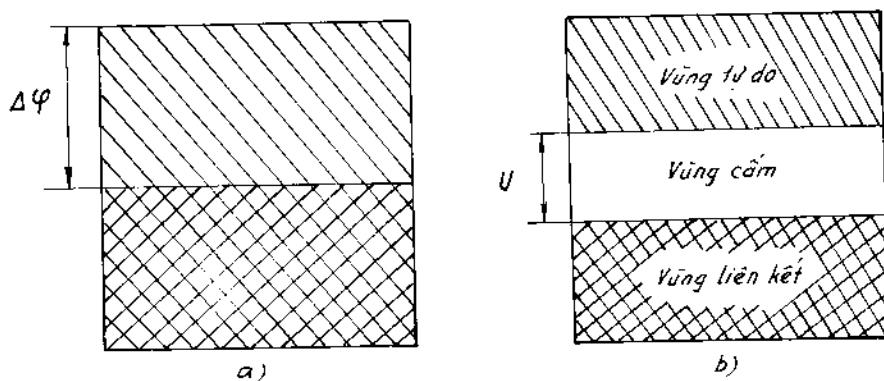
Hình 9-10. Sơ đồ các vùng năng lượng của kim loại (a) và chất bán dẫn (b):
