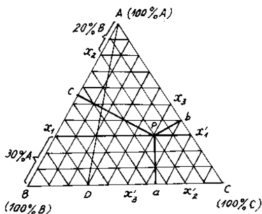
Hình 4-20. Biểu diễn thành phần của hệ ba cấu tử (tam giác thành phần).
