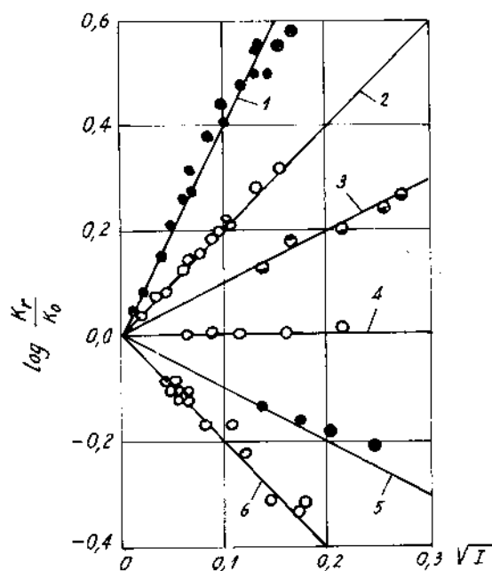
Hình 9-2. Sự phụ thuộc \log \frac{k}{k_0} vào \sqrt{I} của một số phản ứng:
