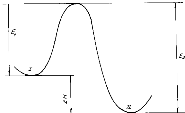
Hình 7-10. Biến thiên năng lượng trong quá trình biến đổi hoá học.
