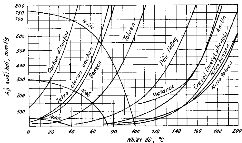
Hình 5-15. Biểu đồ áp suất hơi của các chất hữu cơ chưng theo hơi nước.
