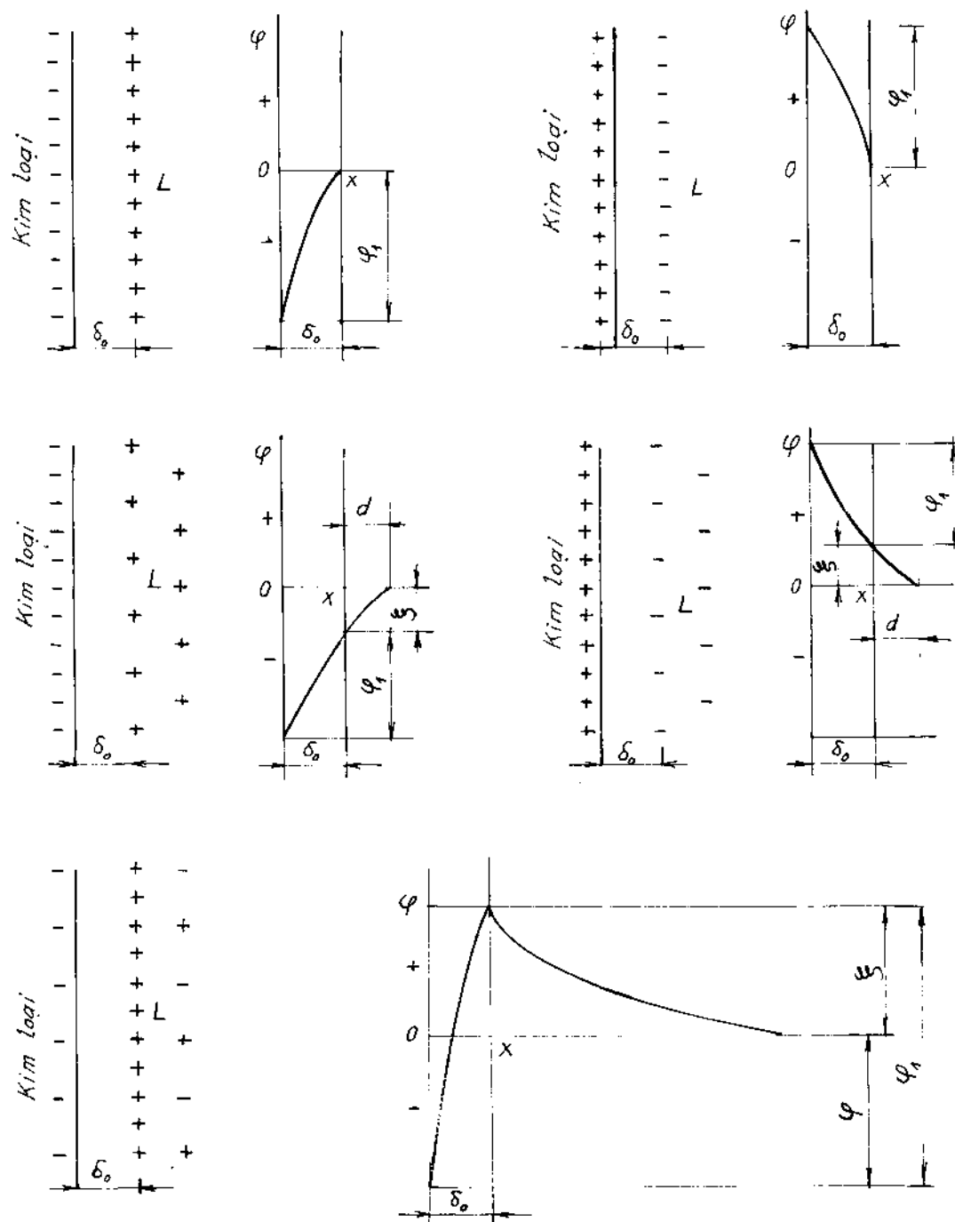
Hình 11-5. Sơ đồ cấu tạo lớp kép và sự biến đổi điện thế phụ thuộc khoảng cách x tính từ bề mặt điện cực.
