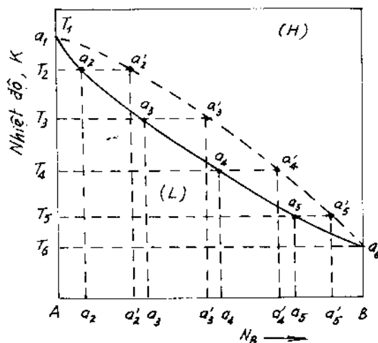
Hình 5-4. Biểu đồ "nhiệt độ sôi - thành phần"
