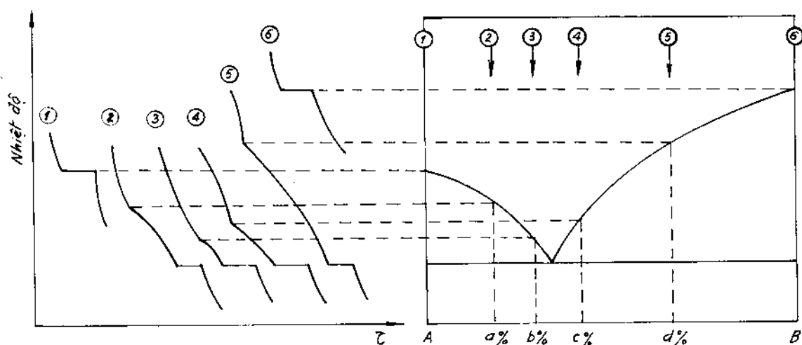
Hình 4-27. Đường lạnh của các hệ.
