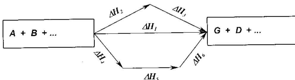
Hình 1-3. Sơ đồ minh họa định luật Hess.
