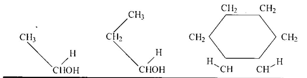
Hình 9-4. Sơ đồ minh họa cắt liên kết theo thuyết đa vị.
