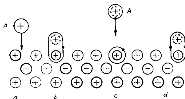
Hình 9-11. Sơ đồ hình thành các liên kết giữa A và bề mặt chất bán dẫn.
