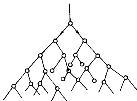
Hình 7-12. Sơ đồ phản ứng dây chuyền phân nhánh.
