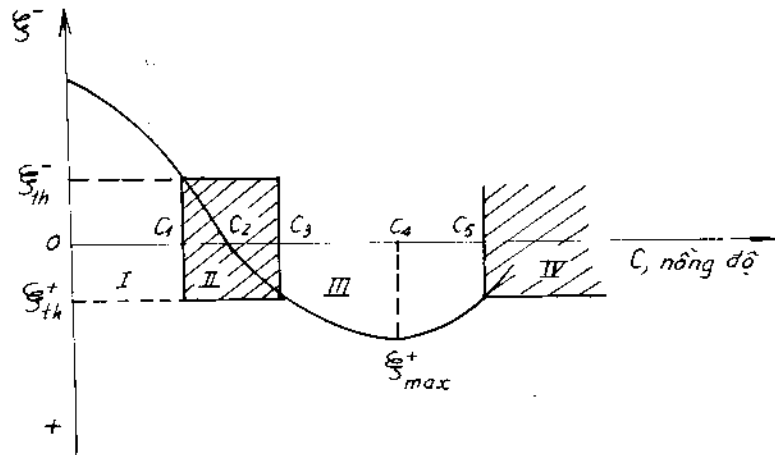
Hình 13-17. Hiện tượng keo tụ vùng.
