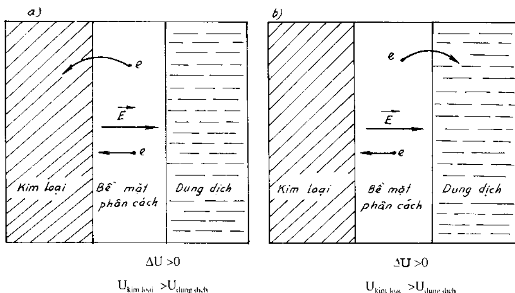
Hình 12-7. Sơ đồ chuyển dịch electron thuận lợi (a), bị cản trở (b):
