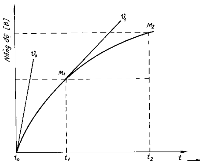
Hình 7-1. Minh hoạ cách xác định tốc độ phản ứng.
