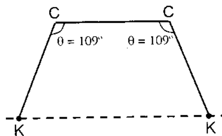
Hình 9-5. Sơ đồ hấp phụ etylen trên hai tâm xúc tác, C: cacbon, K: tâm xúc tác.
