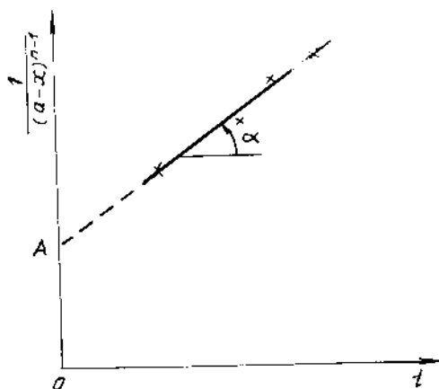
Hình 7-5. Biểu đồ xác định bậc phản ứng bậc n.
