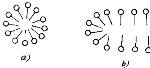
Hình 14-6. Mixen dạng hình cầu (a).
