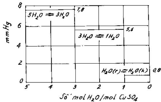
Hình 3-1. Sự biến đổi áp suất H 2 O trong quá trình phân ly CuSO 4 .5H 2 O.
