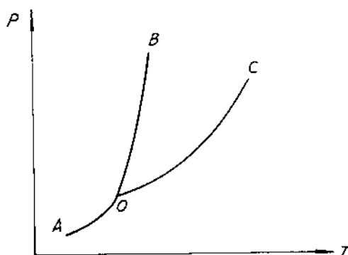
Hình 4-5. Biểu đồ trạng thái ( P - T ) của hệ có \Delta V = V_l - V_r > 0 .
