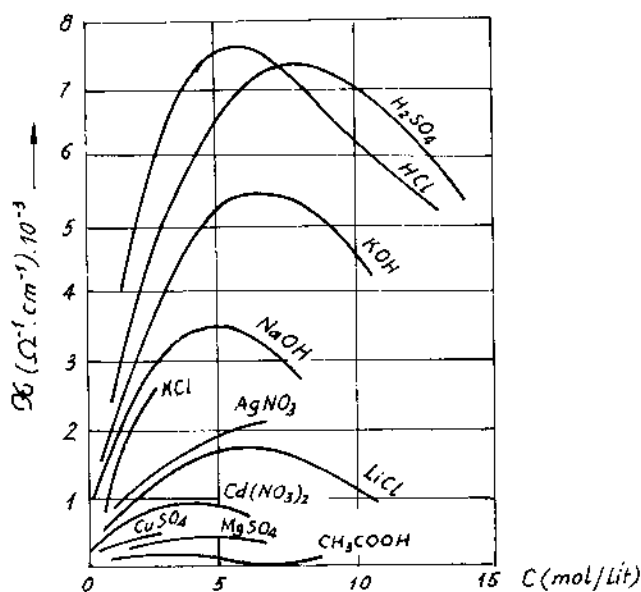
Hình 10-5. Sự phụ thuộc của độ dẫn điện riêng \kappa vào nồng độ dung dịch điện ly.
