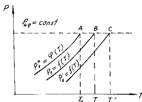
Hình 5-18. Sự phụ thuộc áp suất hơi của dung môi nguyên chất và dung dịch vào nhiệt độ.
