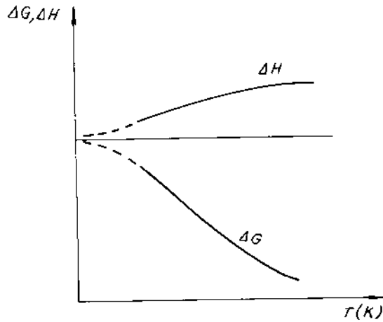
Hình 3-2. Sự phụ thuộc của \Delta G , \Delta H vào nhiệt độ trong miền nhiệt độ thấp.
