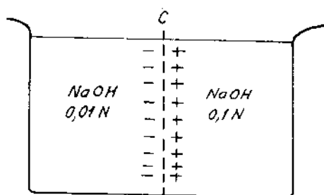
Hình 11-3. Sơ đồ xuất hiện điện thế khuếch tán giữa hai dung dịch.
