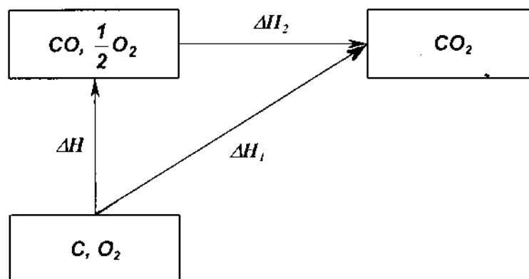
Hình 1-4. Ứng dụng định luật Hess để tính nhiệt sinh của CO.
