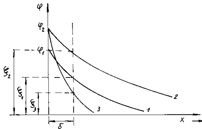
Hình 13-15. Sơ đồ biến đổi \varphi và \xi :
