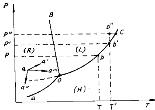
Hình 4-4. Biểu đồ trạng thái (P - T) của H 2 O ở áp suất thấp.
