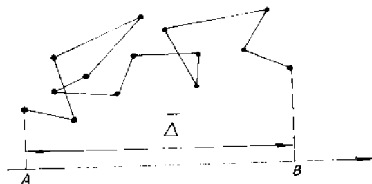
Hình 13-6. Sơ đồ chuyển động Brown của hạt keo.
