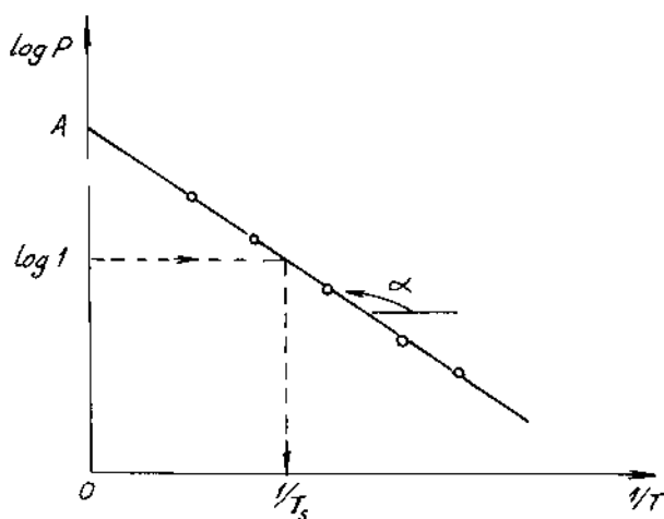
Hình 4-2. Sự phụ thuộc của \log P vào \frac{1}{T} .
