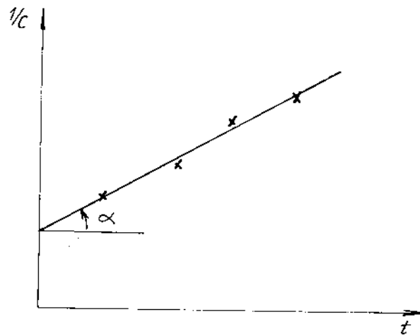
Hình 13-19. Đồ thị xác định hằng số tốc độ keo tụ.
