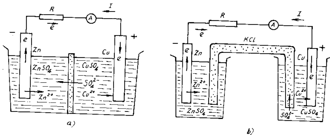
Hình 11-8. Sơ đồ cấu tạo pin Cu - Zn:
