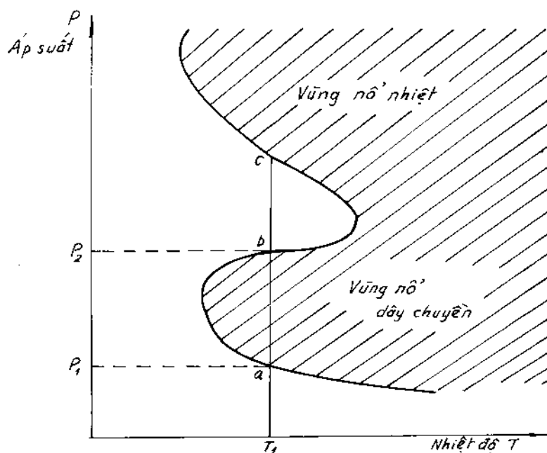
Hình 7-13. Giới hạn của các miền nổ.
