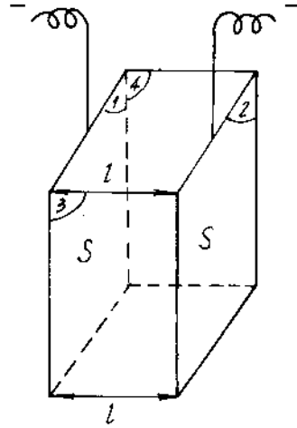
Hình 10-2. Sơ đồ bình đo độ dẫn điện:
