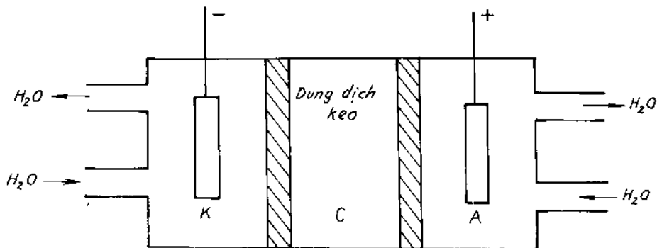
Hình 13-5. Sơ đồ bình điện thẩm tích.
