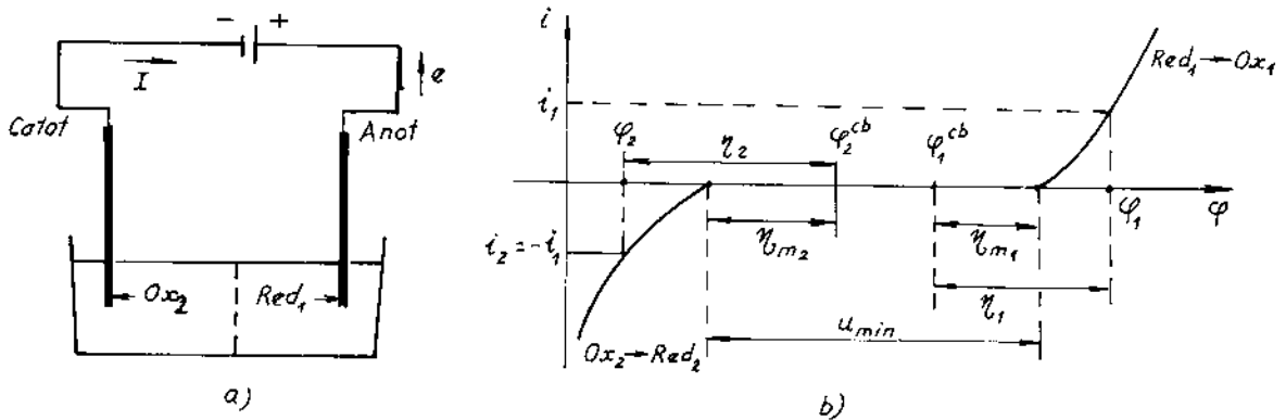
Hình 12-9. Sơ đồ bình điện phân (a), đường cong phân cực (b).
