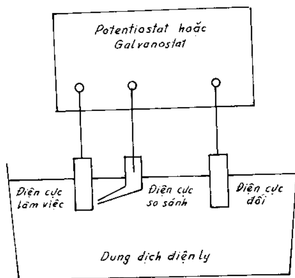
Hình 12-6. Sơ đồ đo các đường cong phân cực.
