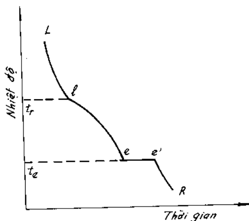
Hình 4-26. Sự phụ thuộc của nhiệt độ vào thời gian trong quá trình làm lạnh hệ hai cấu tử.
