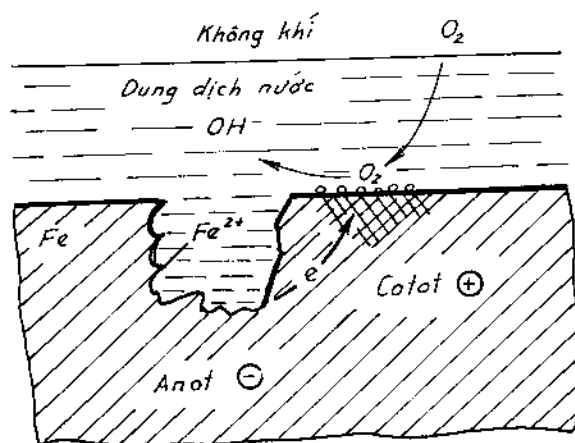
Hình 12-12. Sơ đồ ăn mòn của sắt trong môi trường nước.
