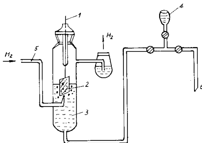
Hình 11-6. Sơ đồ điện cực hydro.
