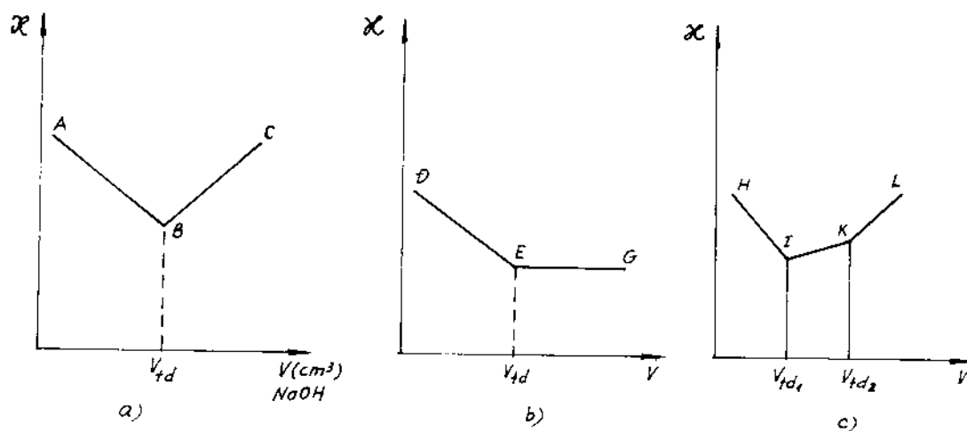
Hình 10-10. Minh hoạ sự định phân bằng phương pháp đo độ dẫn điện.
