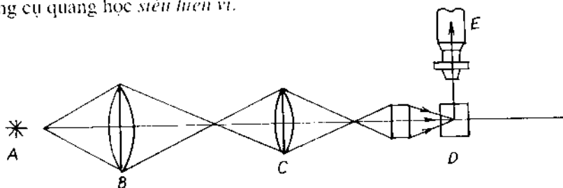
Hình 13-9. Sơ đồ dụng cụ siêu hiển vi.
