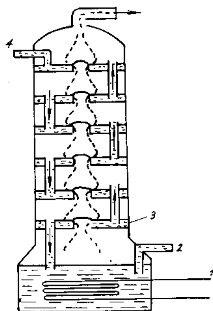
Hình 5-7. Sơ đồ tháp tinh luyện.
