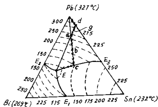
Hình 4-23. Hình chiếu của biểu đồ không gian đa nhiệt (T - C) của hệ Pb - Bi - Sn xuống tam giác thành phần.
