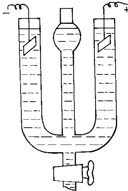
Hình 13-12. Sơ đồ dụng cụ xác định \xi bằng điện di.
