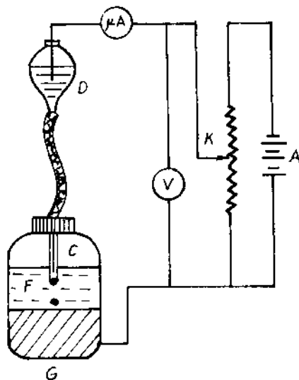
Hình 12-13: Sơ đồ máy cực phổ:
