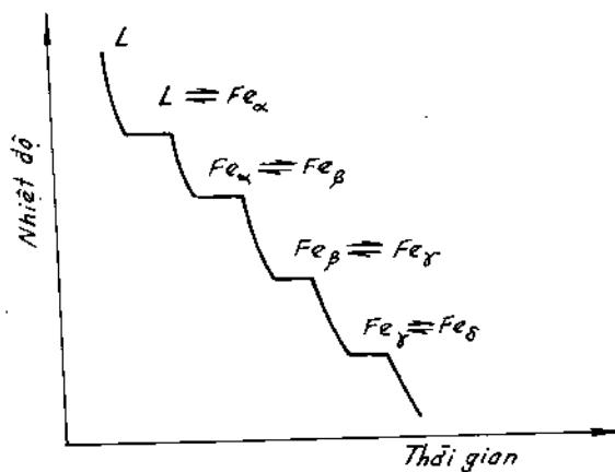
Hình 4-25. Sự phụ thuộc của nhiệt độ vào thời gian trong quá trình làm lạnh Fe.
