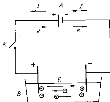
Hình 10-1. Sơ đồ hoạt động dẫn dòng điện của dây dẫn loại 2:
