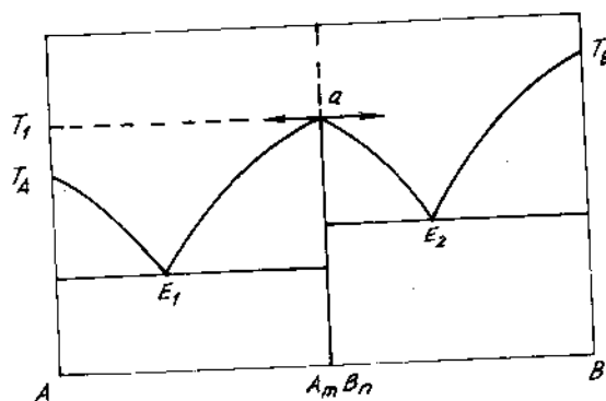
Hình 4-15. Biểu đồ đẳng áp (T - C) của hệ hai cấu tử tạo thành hợp chất hoá học bền không phân ly và không tạo thành dung dịch rắn
