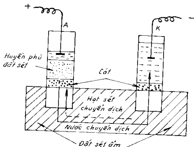
Hình 13-11. Sơ đồ thí nghiệm của Reyss.
