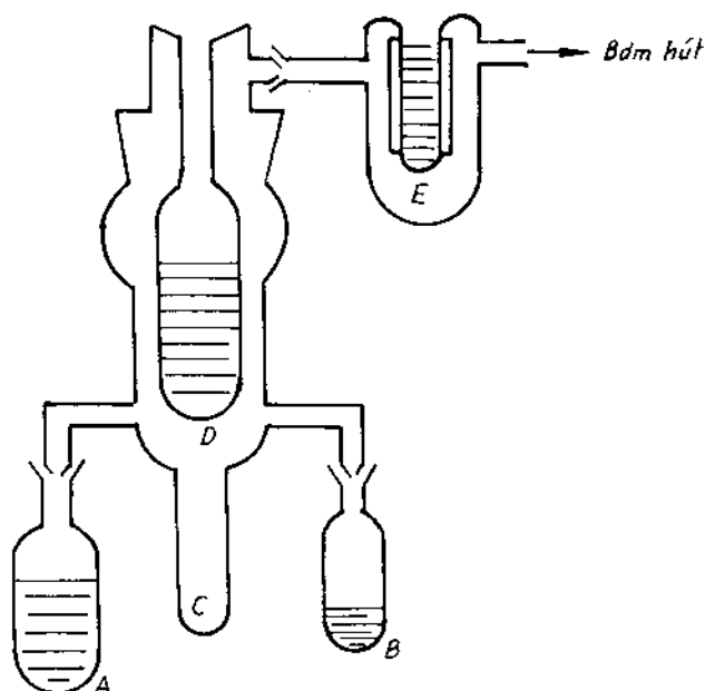
Hình 13-2. Sơ đồ dụng cụ điều chế keo bằng phương pháp ngưng tụ hơi.
