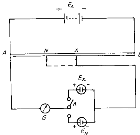
Hình 11-9 Sơ đồ đo Sđđ của pin:
