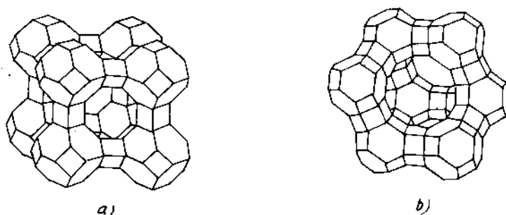
Hình 6-9. Hình thể học (topologie) của zeolit A (a) của zeolit Y (b).
