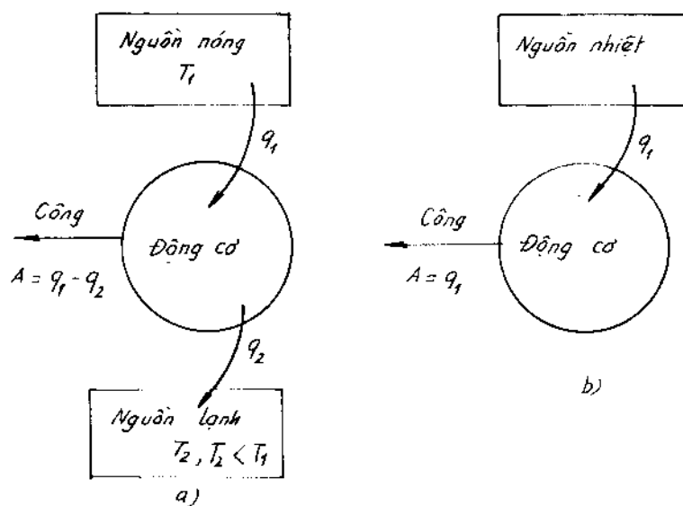
Hình 2-3. Sơ đồ chuyển nhiệt thành công.
