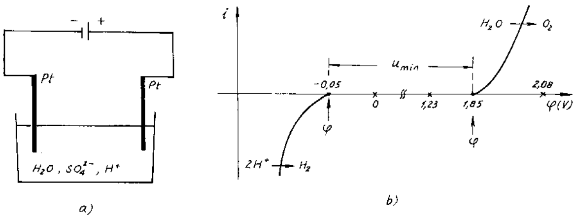
Hình 12-10. (a) Bình điện phân.
