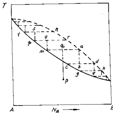
Hình 5-6. Biểu đồ "nhiệt độ sôi - thành phần" dùng để minh họa nguyên tắc chưng luyện.
