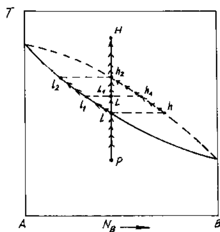
Hình 5-5. Biểu đồ minh họa quá trình sôi.
