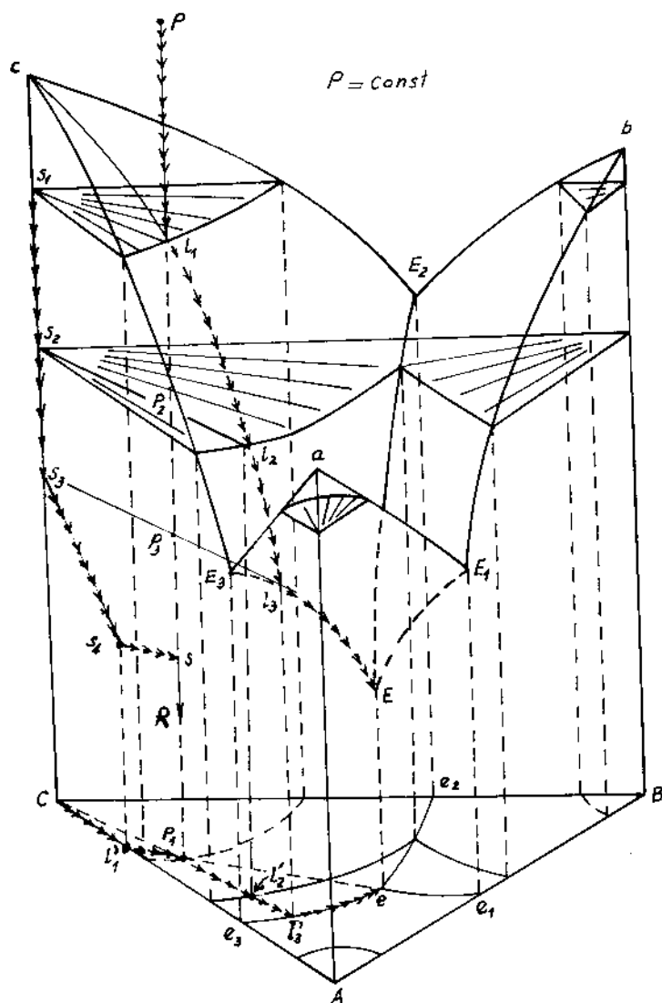
Hình 4-22. Biểu đồ không gian "nhiệt độ - thành phần" của hệ 3 cấu tử.
