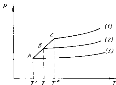
Hình 5-19. Sự phụ thuộc áp suất hơi vào nhiệt độ.
