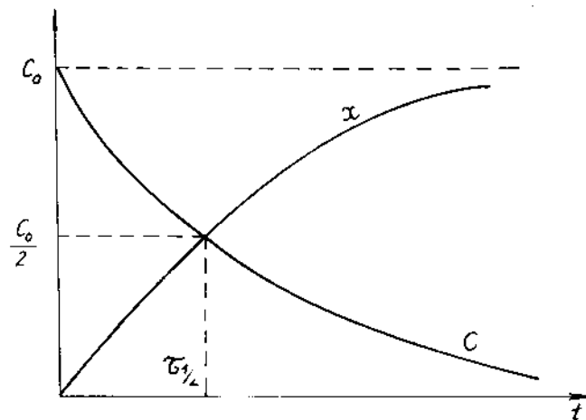
Hình 7-2. Biến thiên nồng độ của chất A theo thời gian.
