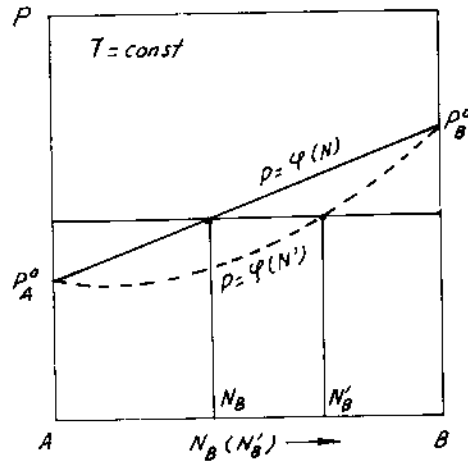
Hình 5-2. Biểu đồ "áp suất hơi - thành phần" [đường P = f(N') ].
