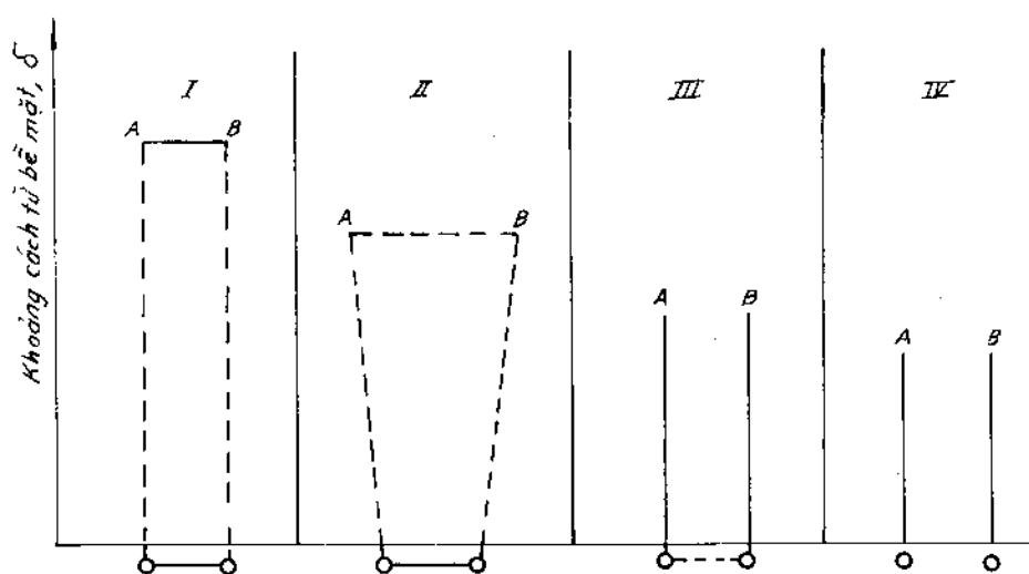
Hình 9-3. Sơ đồ về các kiểu liên kết hấp phụ.
