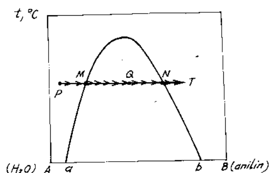
Hình 4-9. Biểu đồ đẳng áp (T – C) dùng để minh họa quá trình thêm đẳng nhiệt anilin.
