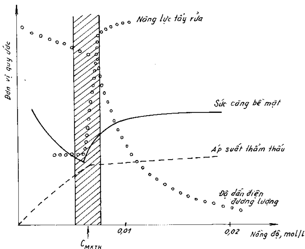
Hình 14-3. Sự biến đổi một vài tính chất của dung dịch sulfat dodexyl natri qua điểm C_{MXTH} ở 298K.
