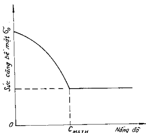
Hình 14-2. Sự biến đổi scbm theo nồng độ chất HĐBM.
