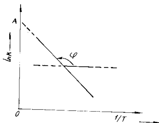
Hình 7-8. Quan hệ giữa \ln k và \frac{1}{T} của phản ứng.
