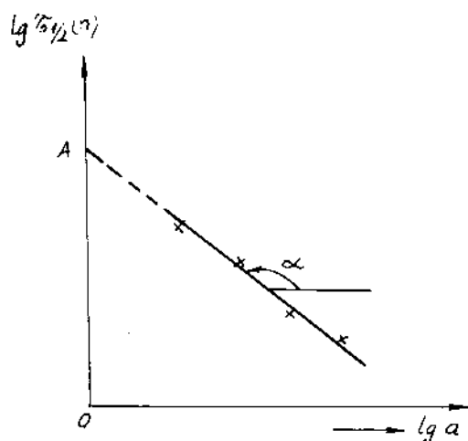
Hình 7-6. Biểu đồ xác định bậc phản ứng theo phương pháp chu kỳ bán huỷ.
