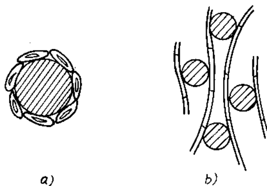
Hình 14-15. Sơ đồ bảo vệ keo kỵ lỏng bằng các CPT bị solvat hoá mạnh:
