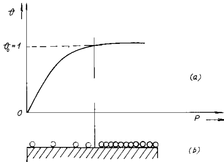
Hình 6 -1: Sơ đồ hấp phụ theo phương trình Langmuir :
