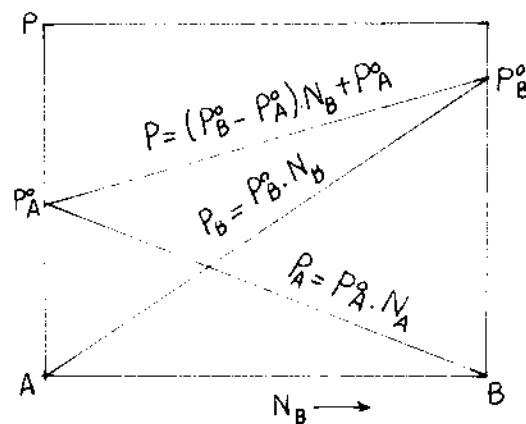
Hình 5-1. Đồ thị áp suất hơi - thành phần lỏng.
