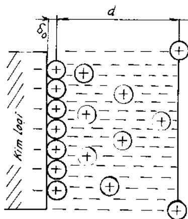
Hình 11-4. Sơ đồ hình thành lớp kép trên bề mặt phân cách kim loại - dung dịch.
