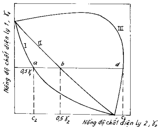
Hình 13-18. Keo tụ bằng hỗn hợp chất điện ly.
