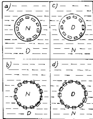
Hình 14-13. Ổn định nhũ tương bằng các chất nhũ hoá bột:
