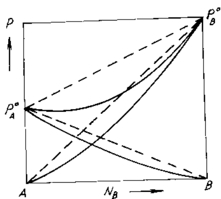
Hình 5-10. Biểu đồ "áp suất hơi - thành phần" của dung dịch sai khác âm.
