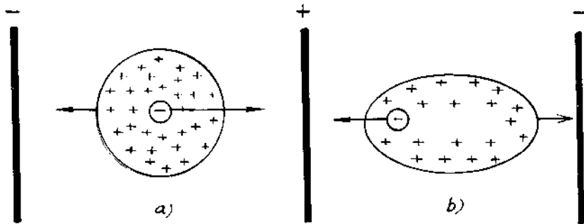
Hình 10-9. Sơ đồ minh họa hiệu ứng điện di (a) và hiệu ứng bất đối (b).
