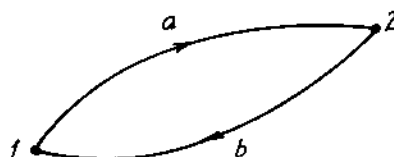
Hình 1-1. Sơ đồ biến thiên hàm trạng thái
