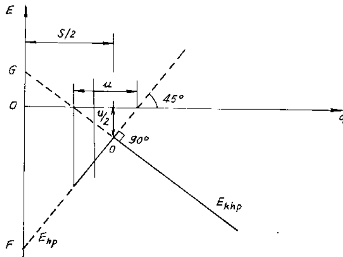
Hình 9-7. Quan hệ E - q trong phản ứng thu nhiệt:
