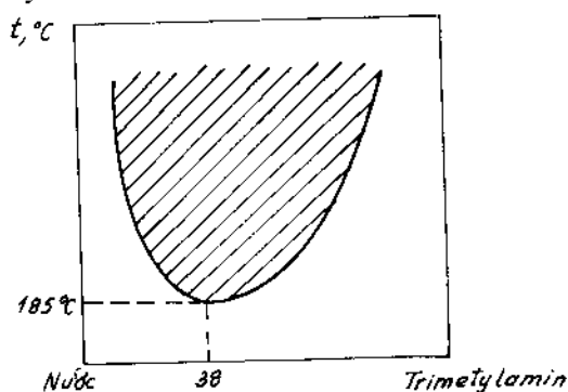
Hình 4-10. Biểu đồ đẳng áp (T – C) của hệ H 2 O – trimetylamin.
