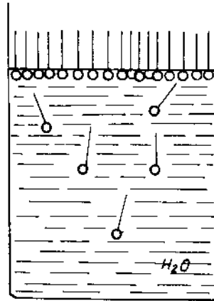
Hình 6-11. Sơ đồ hấp phụ chất IIĐBM trên bề mặt lỏng - khí.
