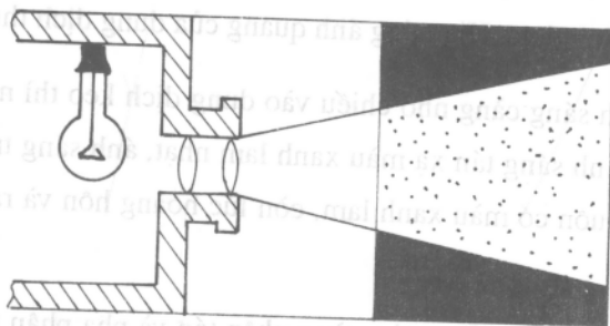
Hình 13-8. Sơ đồ minh họa hiệu ứng Faraday - Tyndall.
