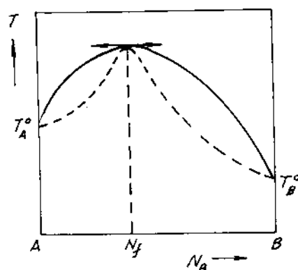
Hình 5-13. Biểu đồ "nhiệt độ sôi - thành phần" của hệ có cực tiểu trên đường áp suất hơi.
