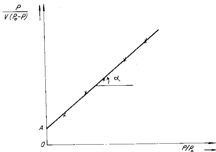
Hình 6-4: Đồ thị dùng để xác định bề mặt riêng theo phản ứng BET.
