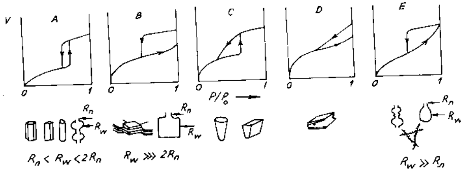
Hình 6-8: Mô hình các dạng mao quản tương ứng với các “vòng trễ” theo De Boer.
