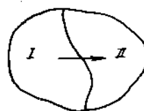
Hình 2-7. Sơ đồ chuyển chất từ pha I sang pha II.
