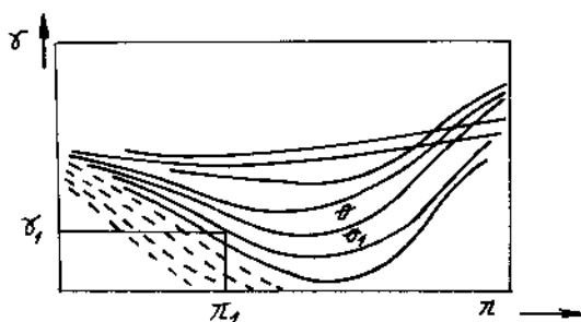
Hình 2-6. Sự phụ thuộc của hệ số fugat vào áp suất và nhiệt độ rút gọn \gamma = f(\pi, \theta)
