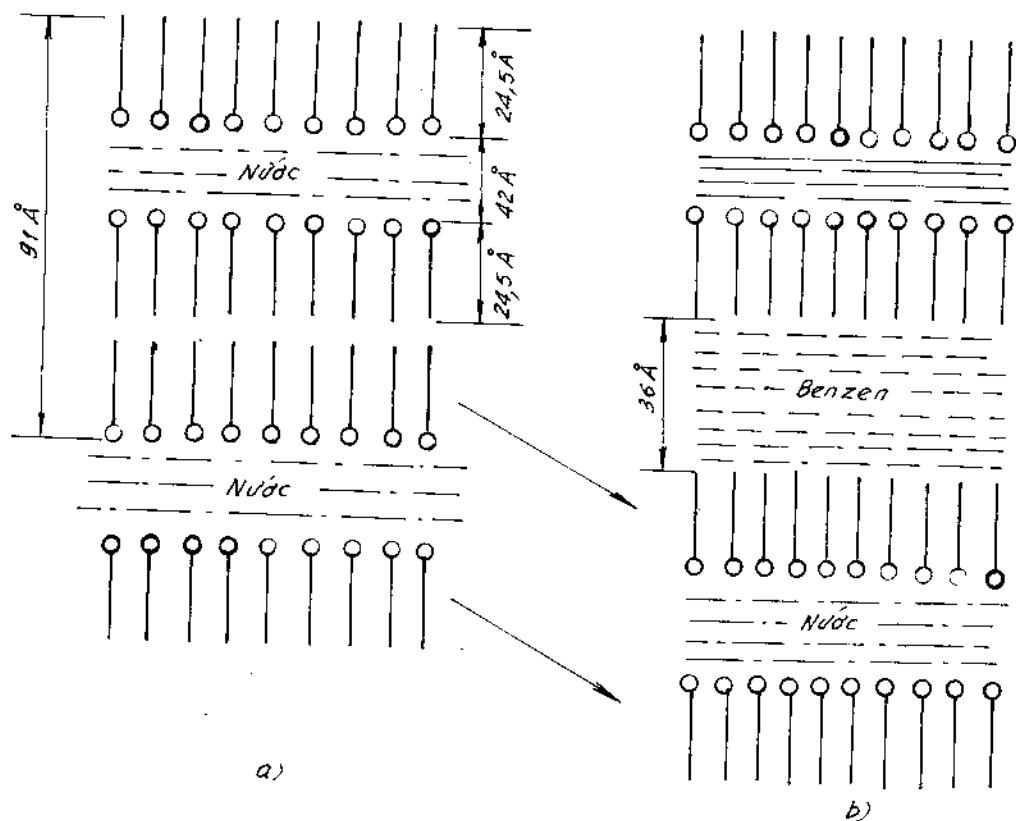
Hình 14-10. Hoà tan benzen trong mixen oleat natri:
