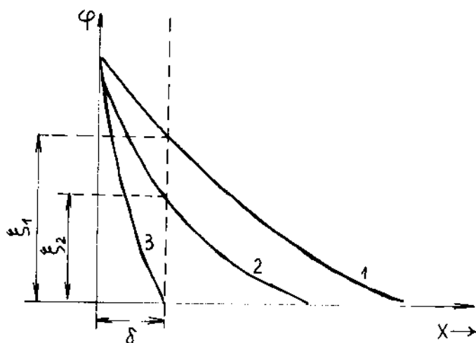
Hình 13-14. Sơ đồ minh hoạ sự giảm \xi theo nồng độ chất điện ly lạ:
