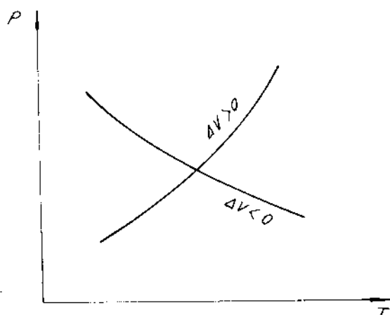
Hình 4-1. Sự phụ thuộc của nhiệt độ nóng chảy vào áp suất
