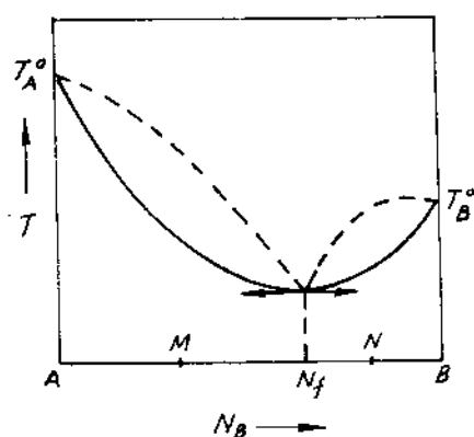
Hình 5-12. Biểu đồ "nhiệt độ sôi - thành phần" của hệ có cực đại trên đường áp suất hơi.
