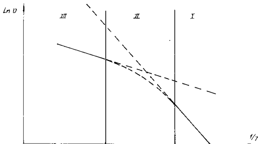
Hình 8-4. Quan hệ giữa \ln v và 1/T trong các miền phản ứng:
