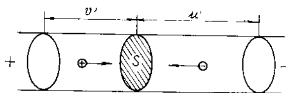
Hình 10-7. Sơ đồ chuyển vận ion trong dung dịch điện ly dưới tác dụng của điện trường.
