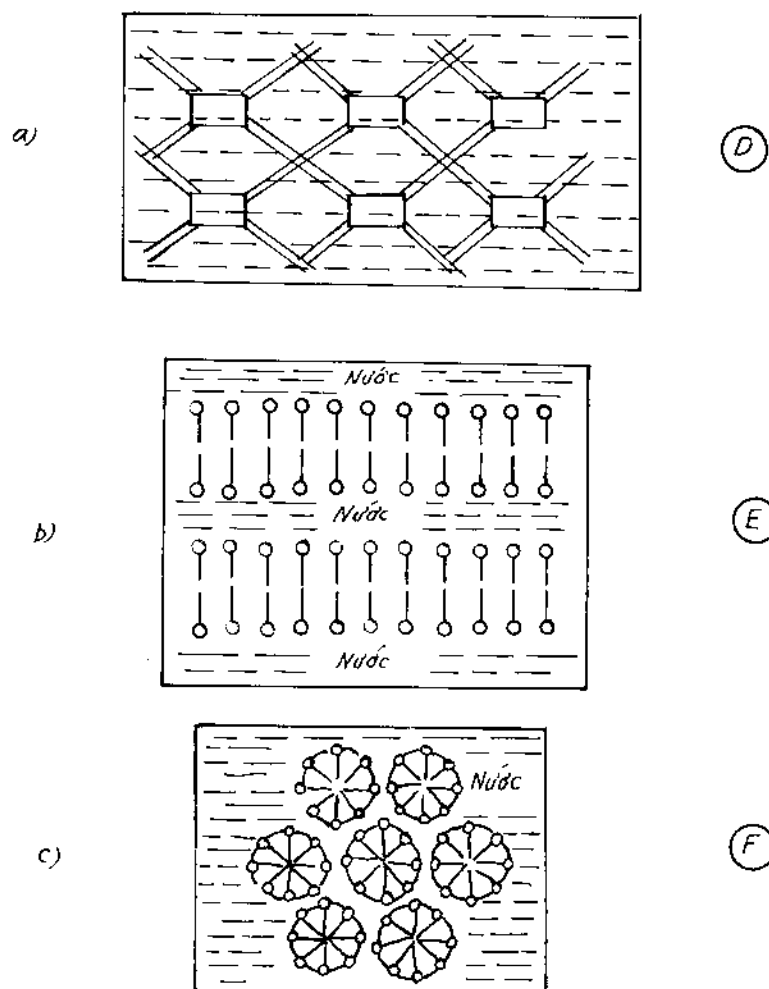
Hình 14-7. Pha lập phương (a), pha hình tấm (b) và pha 6 cạnh (c).
