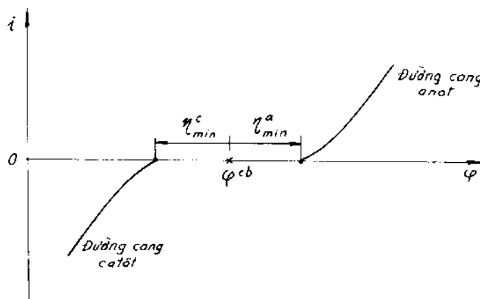
Hình 12-4. Đường cong phân cực chậm:
