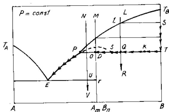
Hình 4-18. Biểu đồ đẳng áp (T - C) của hệ hai cấu tử tạo thành hợp chất hoá học không bền và không tạo thành dung dịch rắn.
