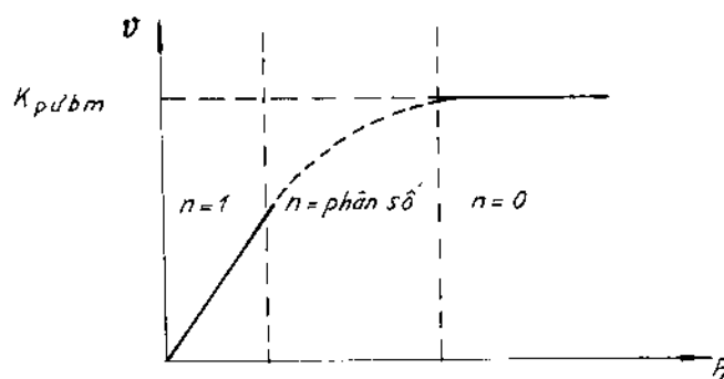
Hình 8-5. Sự biến đổi bậc phản ứng theo áp suất chất A.
