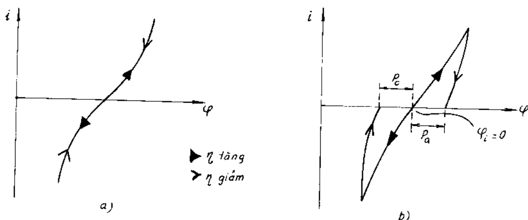
Hình 12-5. Đường cong phân cực thuận nghịch (a), bất thuận nghịch (b):
