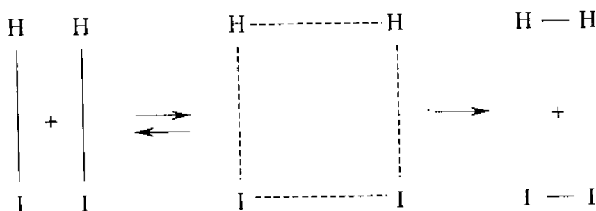
Hình 7-10A. Sự hình thành phức trung gian.
