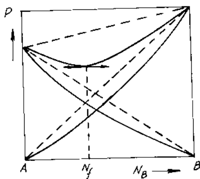
Hình 5-11. Biểu đồ "áp suất hơi - thành phần" của dung dịch sai khác âm có cực tiểu.
