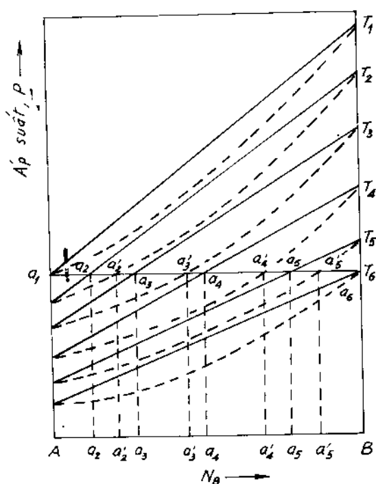
Hình 5-3. Biểu đồ "áp suất hơi - thành phần" ở các nhiệt độ khác nhau.
