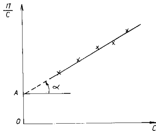
Hình 14-14. Sự phụ thuộc \frac{\Pi}{C} vào nồng độ dung dịch.
