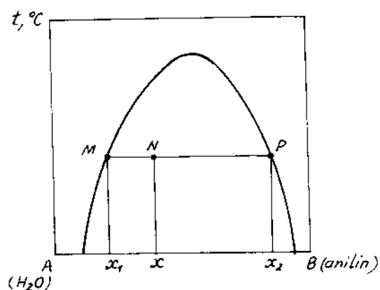
Hình 4-7. Biểu đồ đẳng áp (T - C) dùng để minh họa quy tắc đòn bẩy.
