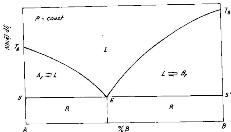
Hình 4-12. Biểu đồ đẳng áp (T - C) của hệ hai cấu tử không tạo thành hợp chất hoá học và dung dịch rắn.
