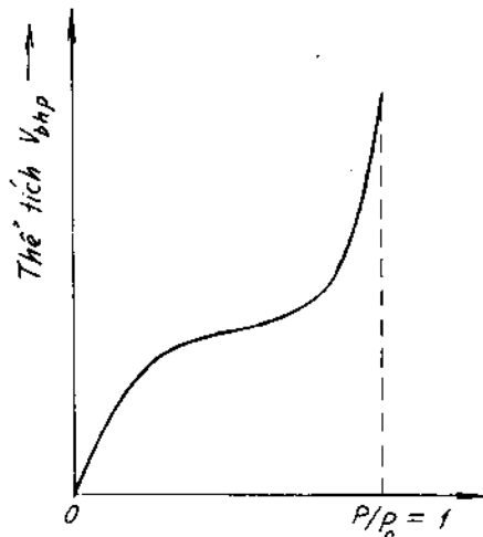
Hình 6 -2: Đường cong hấp phụ dạng chữ S:
