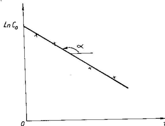
Hình 7-4. Biểu đồ xác định bậc phản ứng bậc 1.
