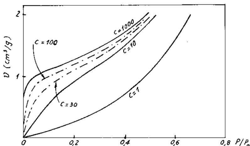
Hình 6-5: Ảnh hưởng của giá trị C đến dáng của đường đẳng nhiệt hấp phụ.
