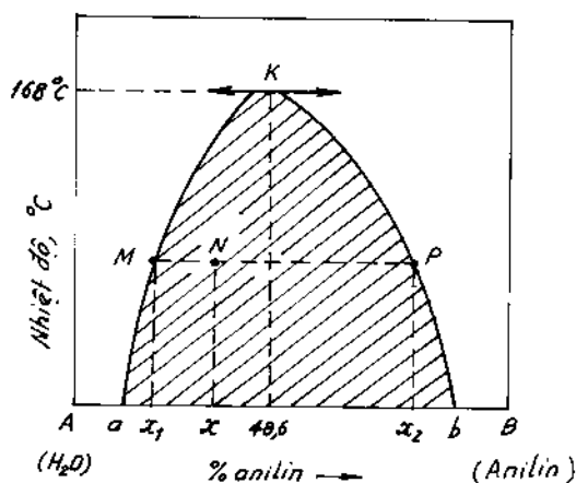
Hình 4-6. Biểu đồ đẳng áp (T - C) của hệ H_2O - anilin.
