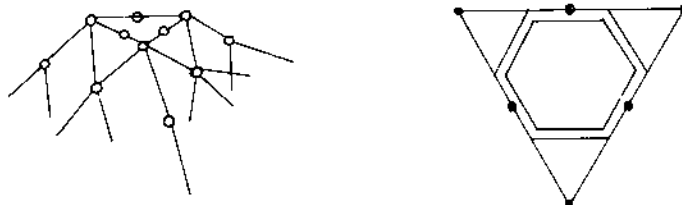
Hình 9-6. Sơ đồ tương ứng hình học của benzen và các nguyên tử bạch kim trên một mạng tinh thể.
