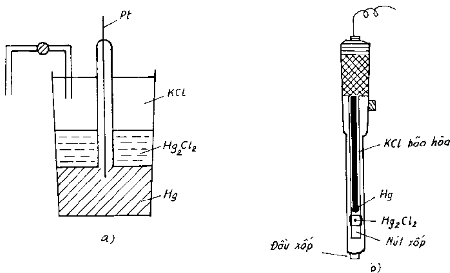
Hình 11-7. Điện cực calomen tự chế tạo (a).
