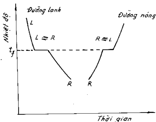
Hình 4-24. Sự phụ thuộc của nhiệt độ vào thời gian trong quá trình làm lạnh và đun nóng hệ một cấu tử (chất nguyên chất).
