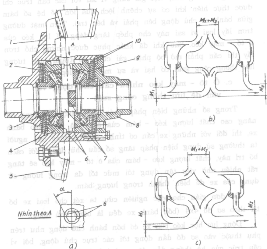
Hình XI-3. Cấu tạo của vi sai có ma sát trong lớn nhỏ ly hợp ma sát và sơ đồ phân bố mômen cho các bánh trục
