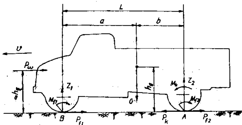
Hình 11-10. Sơ đồ lực tác dụng lên ô tô-máy kéo bánh xe chuyển động trên đường nằm ngang
