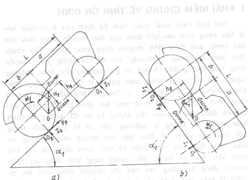
Hình VII-1. Sơ đồ lực và mômen tác dụng lên ô tô, máy kéo bánh hơi khi đứng yên.
