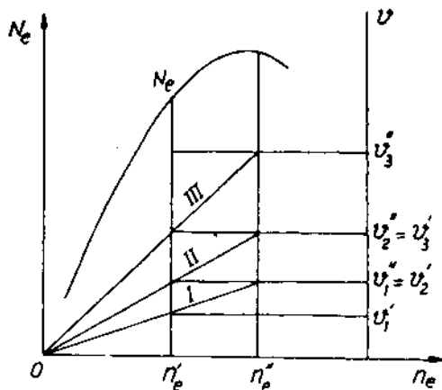
Hình IV-18. Đồ thị sang số của ô tô có hộp số 3 cấp bố trí theo cấp số nhân
