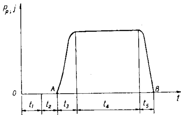
Hình IX-12. Giảm đồ phanh.
