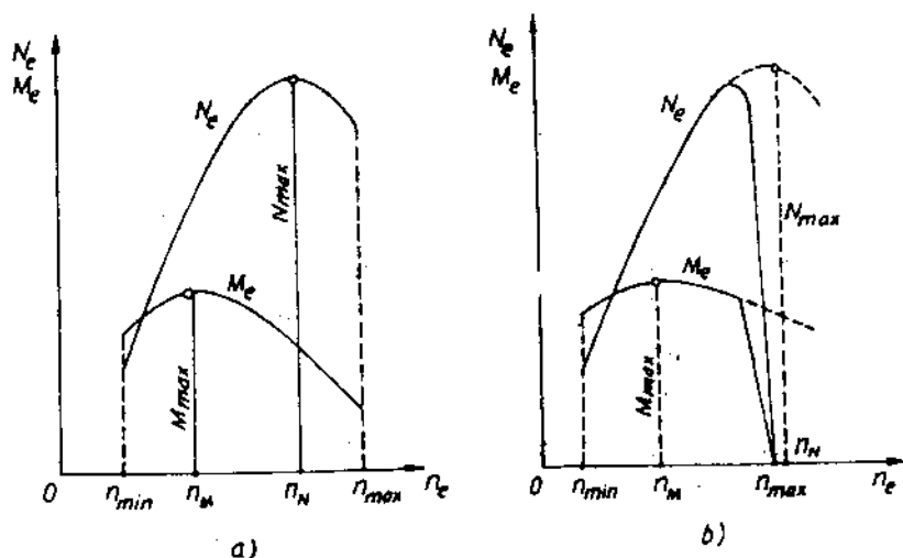
Hình I-1 Đường đặc tính ngoài của động cơ xăng a. Không hạn chế số vòng quay; b. Có hạn chế số vòng quay.
