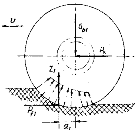
Hình II-4 Sơ đồ lực tác dụng lên bánh xe cũng lăn trên đường biến dạng
