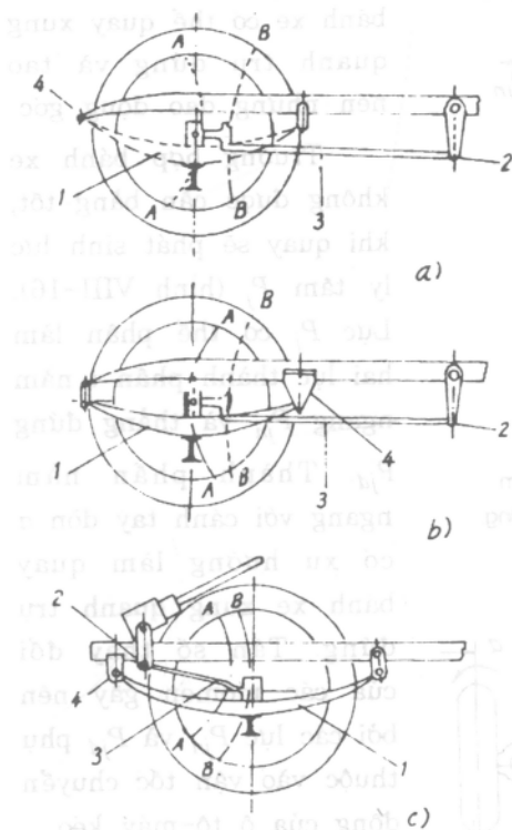
Hình VIII-18. Sơ đồ về sự phối hợp động học giữa hệ thống treo nhíp và dẫn động lái.
