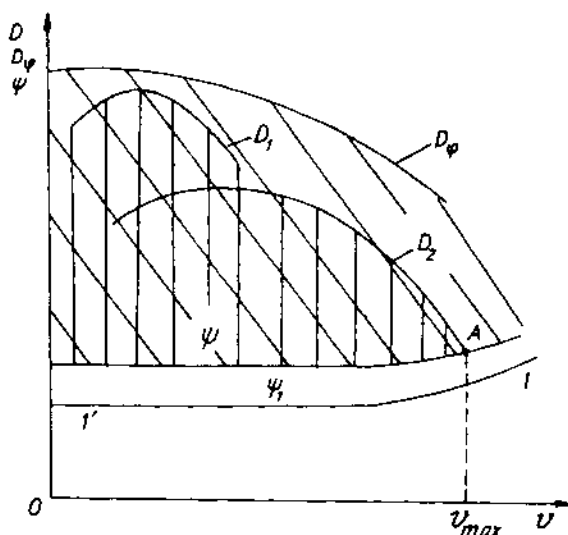
Hình IV-6 Vùng sử dụng đồ thị nhân tố động lực học D theo điều kiện bám của bánh xe chủ động và điều kiện sức cản của mặt đường
