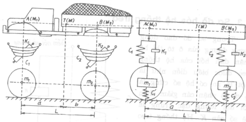
Hình X-6. Sơ đồ dao động tương đương của ô tô
