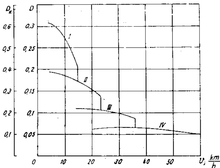
Hình IV-15 Đồ thị nhân tố động lực học của ô tô, có 4 số truyền khi chuyển động với tải trọng đầy G và khi có G_x = 0,5G
