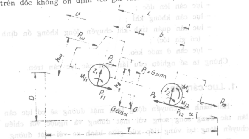
Hình I-5 Lực và mômen tác dụng lên ô tô chuyển động tăng tốc ở trên dốc
