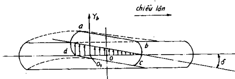
Hình VIII-4. Sơ đồ bánh xe lăn khi lớp bị biến dạng dưới tác động của lực bên.
