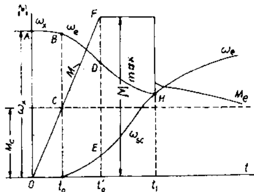
Hình V-11. Đồ thị khởi hành và tăng tốc liên hợp máy kéo.
