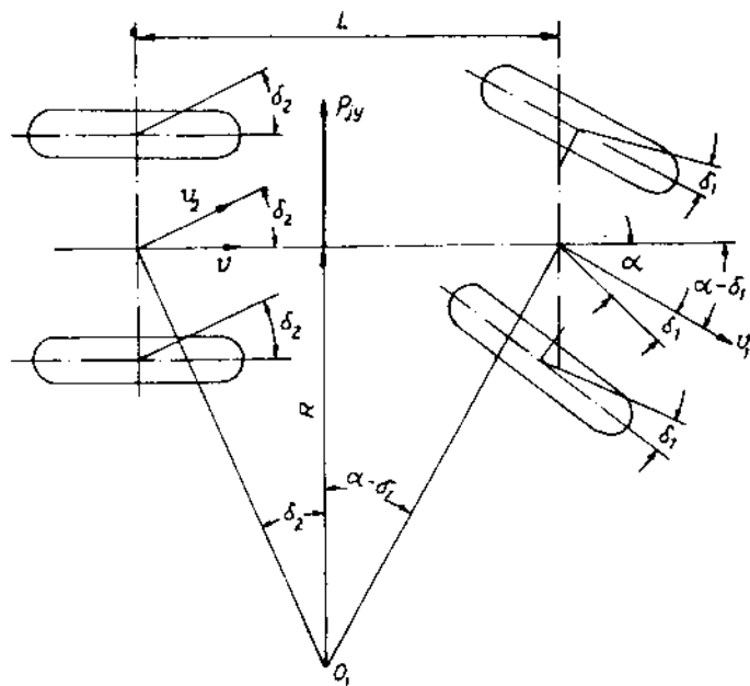
Hình VIII-8. Sơ đồ chuyển động quay vòng của ô tô - máy kéo khi lóp bị biến dạng bên
