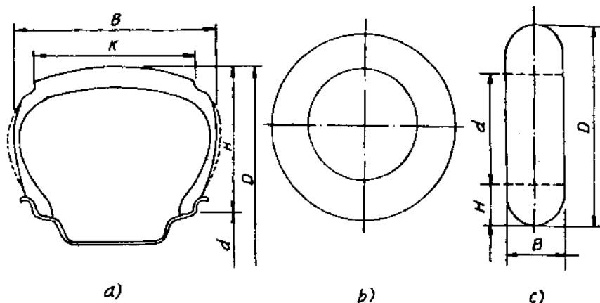
Hình 11-1 Sơ đồ kích thước hình học của lốp
