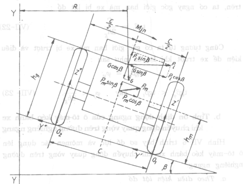
Hình VII-8. Sơ đồ lực và mômen tác dụng lên ô tô-máy kéo bánh xe khi chuyển động quay vòng trên đường nghiêng ngang.
