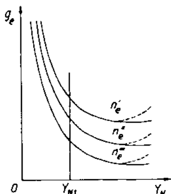
Hình VI-2. Đồ thị đặc tính tải trọng của động cơ ( n_e^I > n_e^II > n_e^III ).
