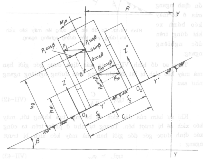
Hình VII-13. Sơ đồ lực và mômen tác dụng lên máy kéo xích khi chuyển động quay vòng trên đường nghiêng ngang.
