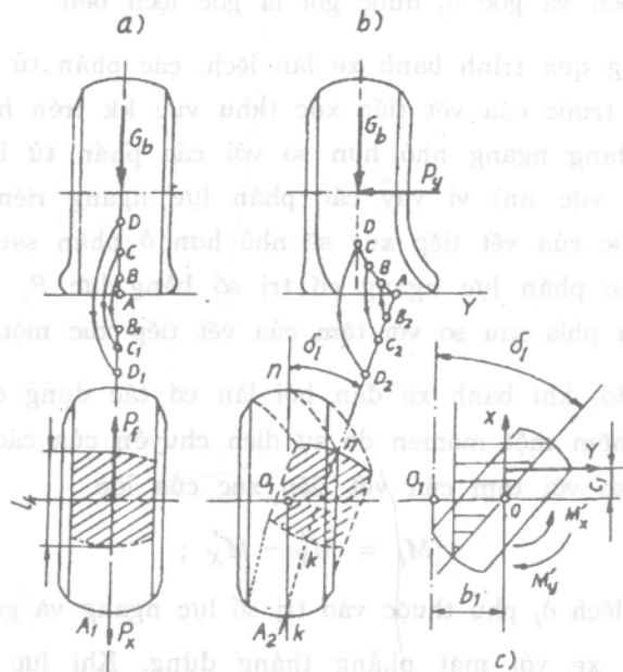
Hình II-6. Sơ đồ minh họa sự lăn của bánh xe đàn hồi:
