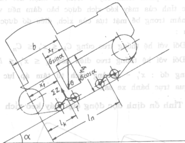
Hình VII-9. Sơ đồ máy kéo xích có hệ thống treo điều hòa đứng trên dốc.
