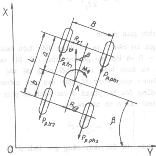
Hình IX-15. Sơ đồ lực tác dụng lên ô tô khi phanh mà bị quay ngang
