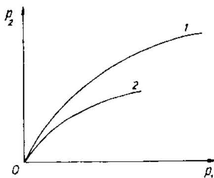
Hình IX-6. Đồ thị chỉ quan hệ giữa áp suất trong dẫn động phanh sau và dẫn động phanh trước để đảm bảo sự phanh lý tưởng. 1- Đầy tải ; 2- Không tải
