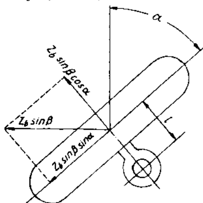
Hình VIII-10. Sơ đồ phân tích phản lực của đường tạo nên mômen ổn định.
