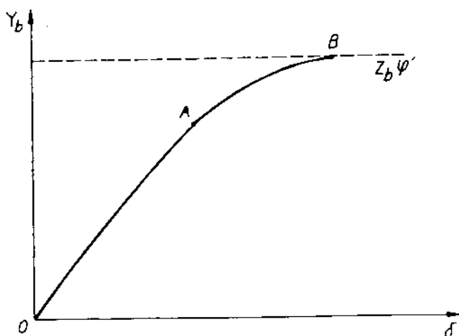
Hình VIII-5. Đồ thị quan hệ giữa phản lực bên Y_b và góc lệch bên \delta của lốp.
