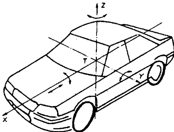
Hình X-2. Hệ dao động không gian của ô tô hai cầu.
