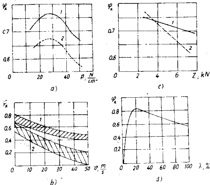
Hình 1-4 Các yếu tố ảnh hưởng đến hệ số bám 1 đường khô, 2 đường ướt
