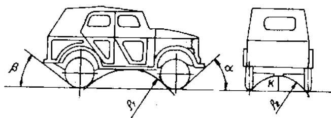
Hình XI-1. Các thông số hình học và tính năng cơ động của ô tô.
