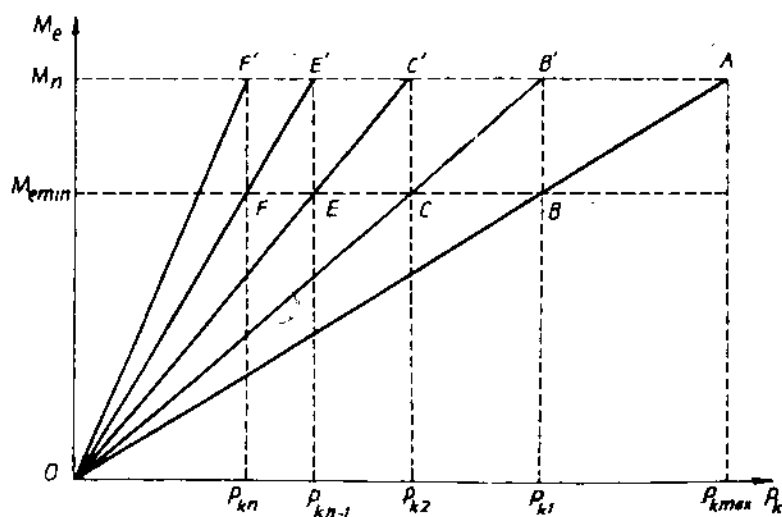
Hình V-2. Đồ thị biểu thị quan hệ M_e = f(P_k) khi dãy tỷ số truyền bố trí theo cấp số nhân.
