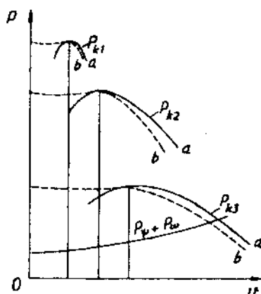
Hình IV-21 Đồ thị đặc tính kéo của ô tô a- Khi đặt ly hợp ma sát b- Khi đặt ly hợp thủy lực.
