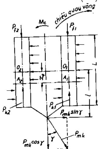
Hình VIII-21. Sơ đồ các lực tác động lên máy kéo khi quay vòng.
