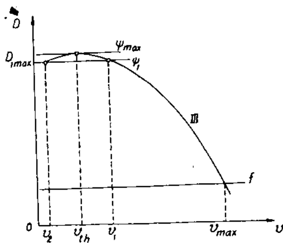
Hình IV-7 Khu vực làm việc của nhân tố động lực học
