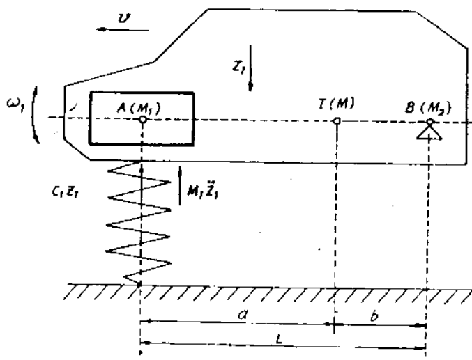
Hình X-11. Sơ đồ dao động độc lập của ô tô tại cầu trước
