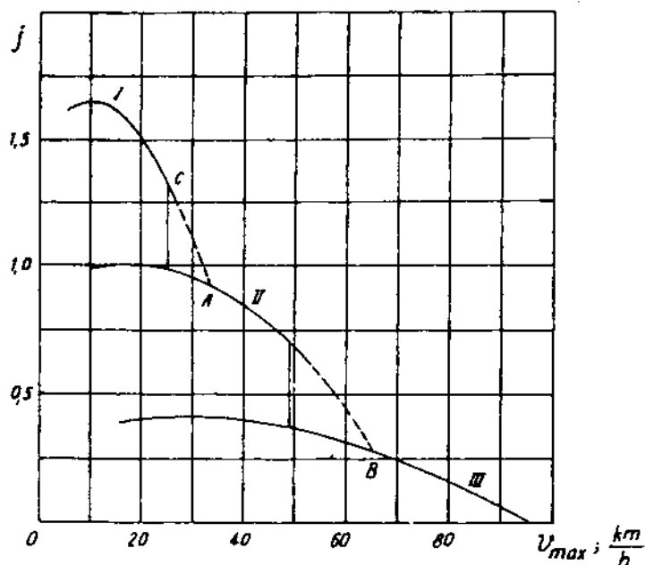
Hình IV-8 Đồ thị biểu diễn gia tốc của ô tô có 3 số truyền
