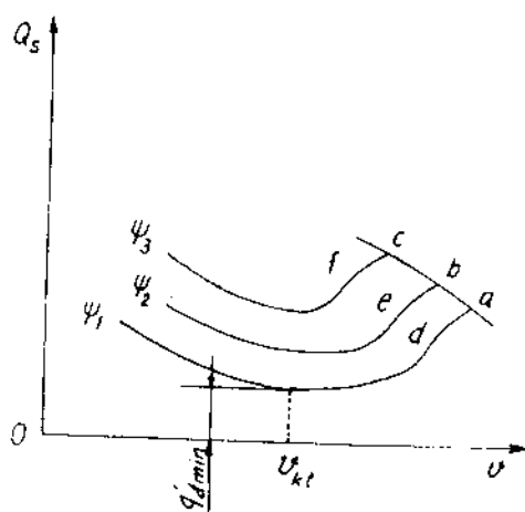
Hình VI-4. Đồ thị đặc tính tiêu hao nhiên liệu của ô tô khi chuyển động ổn định.
