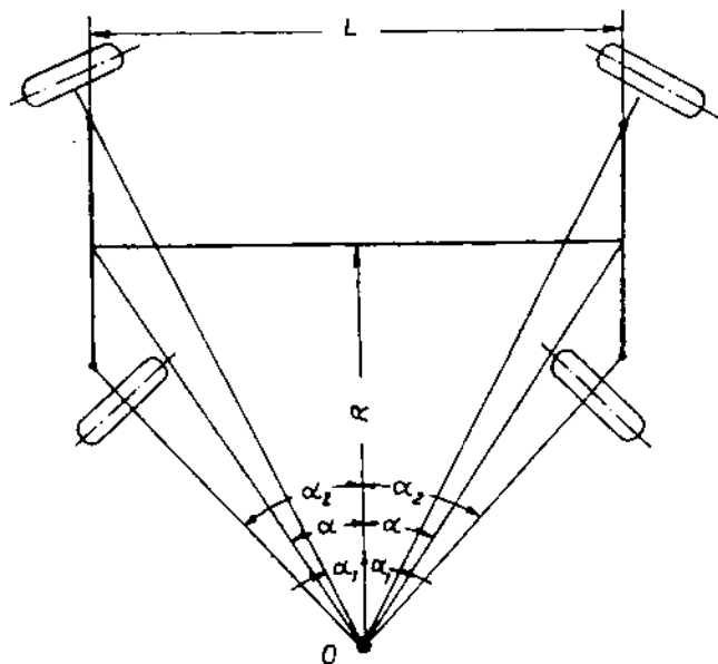
Hình VIII-3. Sơ đồ quay vòng của ô tô máy kéo có bốn bánh dẫn hướng.
