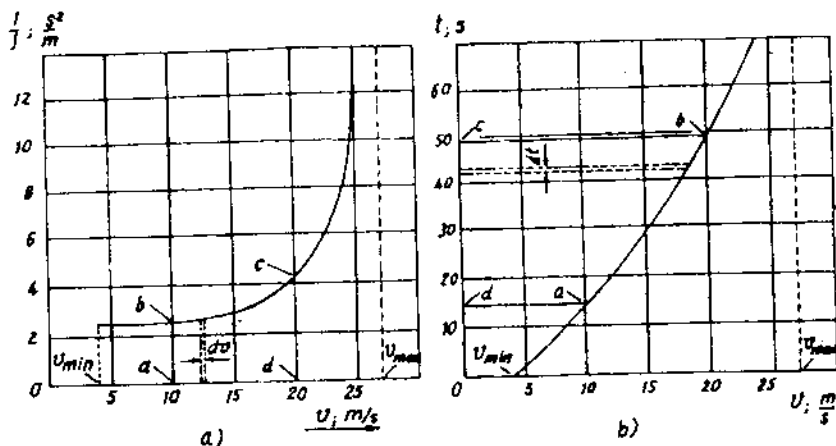
Hình IV-12 Đồ thị xác định thời gian tăng tốc của ô tô
