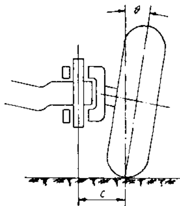
Hình VIII-13. Góc đoang của bánh xe dẫn hướng phía trước.
