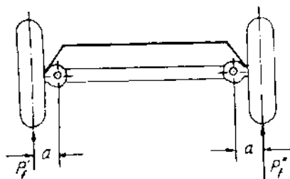
Hình VIII-15. Sơ đồ các lực cân lẫn có trị số khác nhau tác động lên hai bánh dẫn hướng
