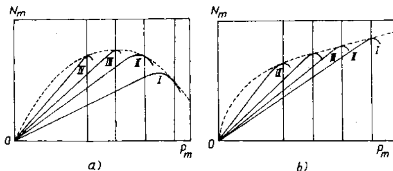
Hình V-9. Đồ thị công suất kéo có ích ở mức kéo có 4 số truyền.
