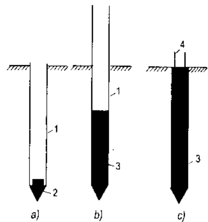
Hình 3.7. Cọc bê tông đổ tại chỗ
