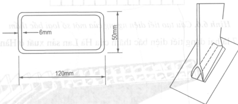
Hình 6.8c. Tiết diện cần cẩu bắc thấm và neo
