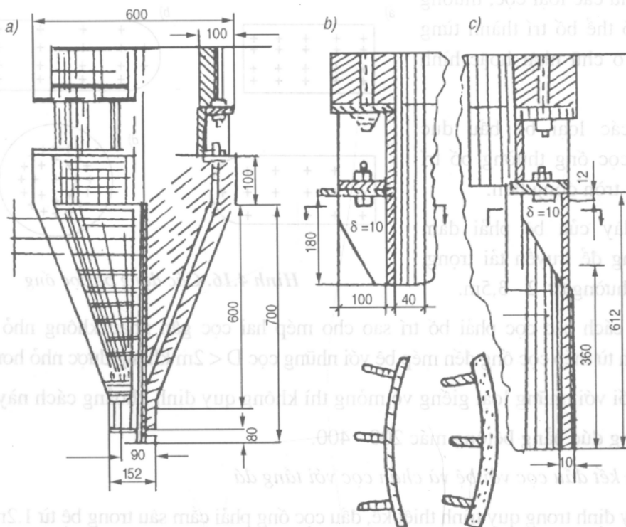
Hình 4.15. Cấu tạo chân cọc ống
