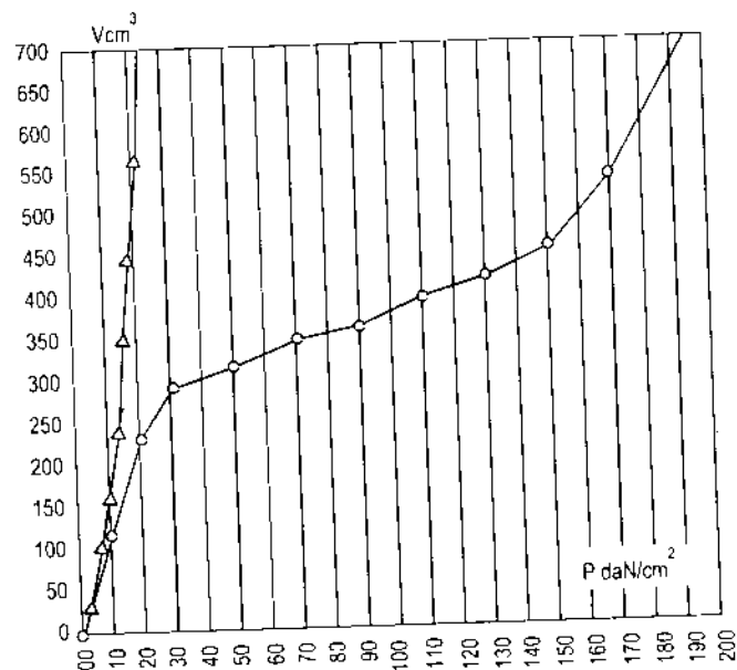
Hình 1.8. Đường cong nén ngang
