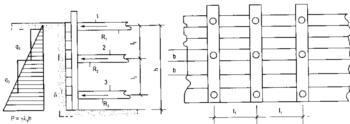
Hình 2.25. Tính toán ván lát
