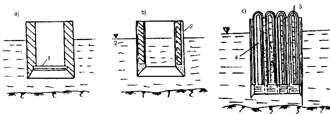
Hình 5.21. a) Giếng chìm có đáy tạm; b) Giếng với các lỗ rỗng; c) Giếng chìm với các ống thép. 1- Sàn đáy tạm bằng gỗ; 2- Bê tông; 3- Ống thép; 4- Mức nước.
