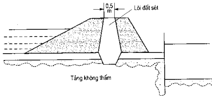
Hình 2.31. Vòng vây đất có lõi đất sét
