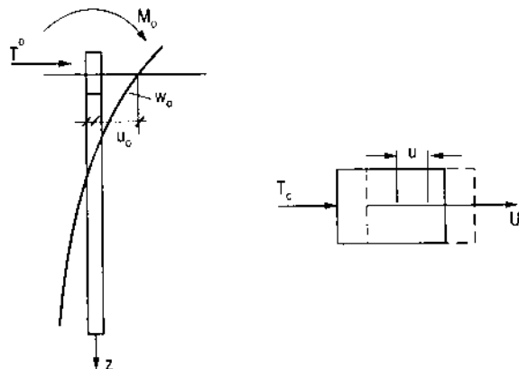
Hình 3.24. Sơ đồ biến dạng của cọc dưới tác dụng lực ngang.
