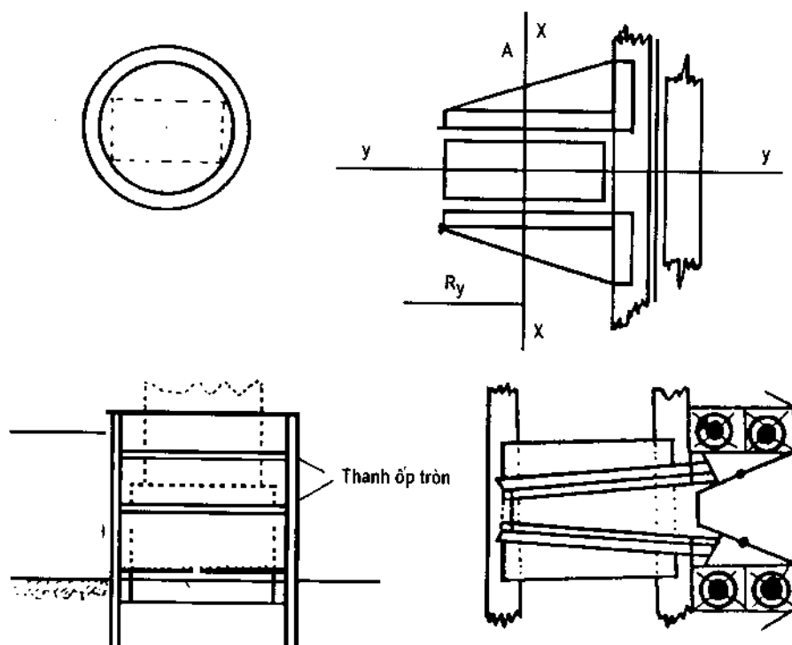
Hình 2.35. Vòng vây cọc ván thép tròn
