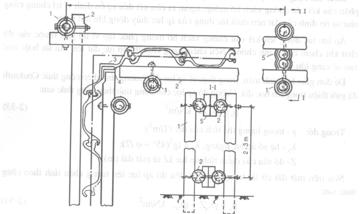
Hình 2.23. Khung định hướng dùng khi đóng cọc ván thép 1- Cọc định vị; 2- Khung định hướng; 3- Cọc ván thép.
