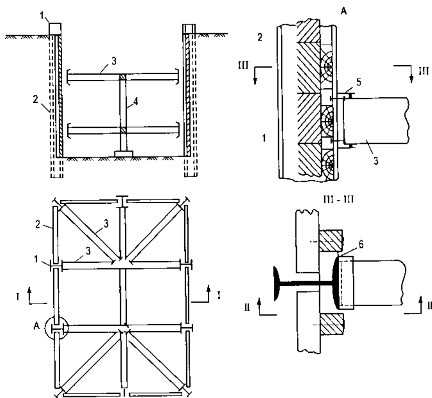
Hình 2.18. Cấu tạo ván lát kiểu chống bằng sắt chữ I 1- Thanh sắt chữ I; 2- Vách lát ngang; 3- Thanh chống ngang; 4- Thanh chống đứng; 5- Nêm gỗ; 6- Bulông.
