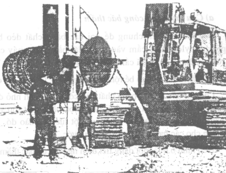
Hình 6.8b. Máy cẩu bắc thấm đang hoạt động
