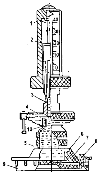
Hình 2.52. Dụng cụ xác định độ tách nước
