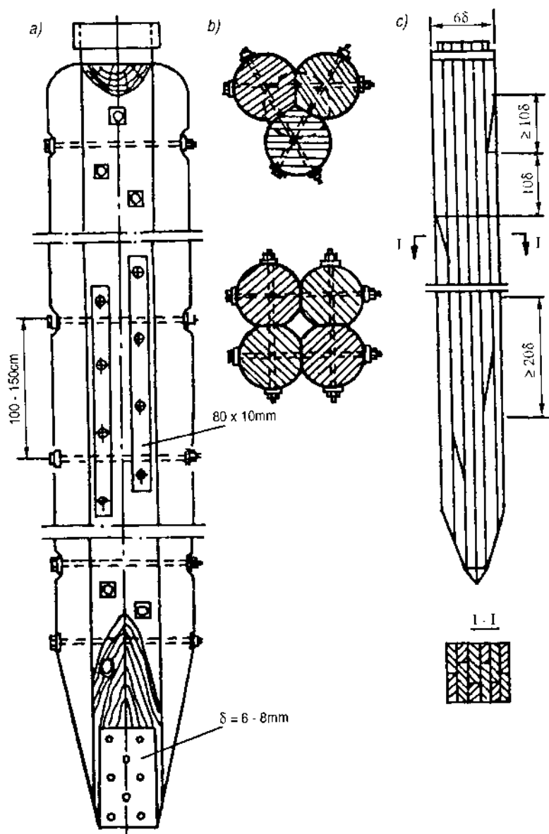
Hình 3.4. Cọc tổ hợp
