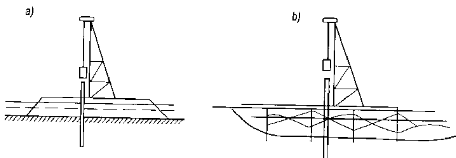
Hình 3.55. Đóng cọc nơi có mặt nước nông a) Đóng cọc trên đảo đất; b) Đóng cọc trên sàn tạm.
