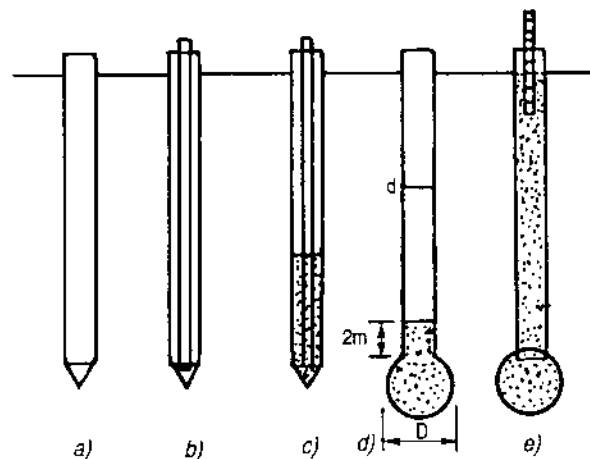
Hình 3.8. Cọc nổ mìn
