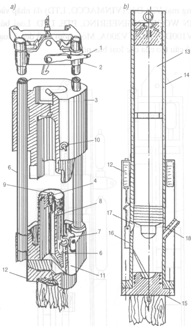
Hình 3.47. Búa diesel a) Kiểu cột dẫn; b) Kiểu ống.
