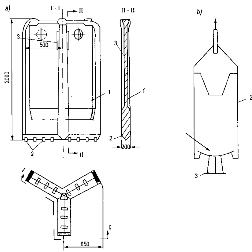
Hình 4.29. Thùng lấy bùn 1- Nắp dây hình mặt cầu; 2- Thùng hình ống; 3- Đế hàn liền với nắp; 4- Đáy hình mặt cầu.
