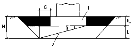
Hình 6.1. Móng trên đệm cát 1- Móng; 2- Đệm cát
