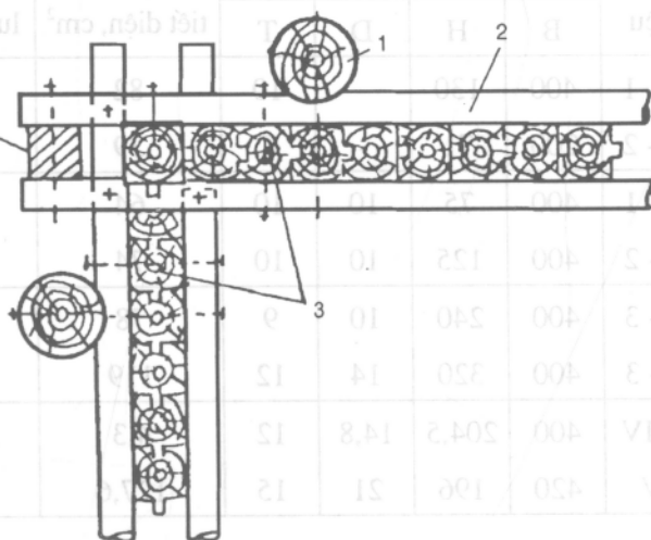
Hình 2.21. Khung định hướng 1- Cọc định vị; 2- Khung định hướng; 3- Cọc ván.
