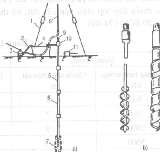
Hình 1.1. Thiết bị, dụng cụ khoan
