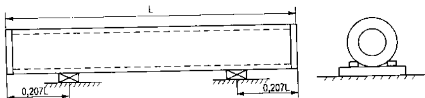
Hình 4.20. Kê cọc ống khi vận chuyển
