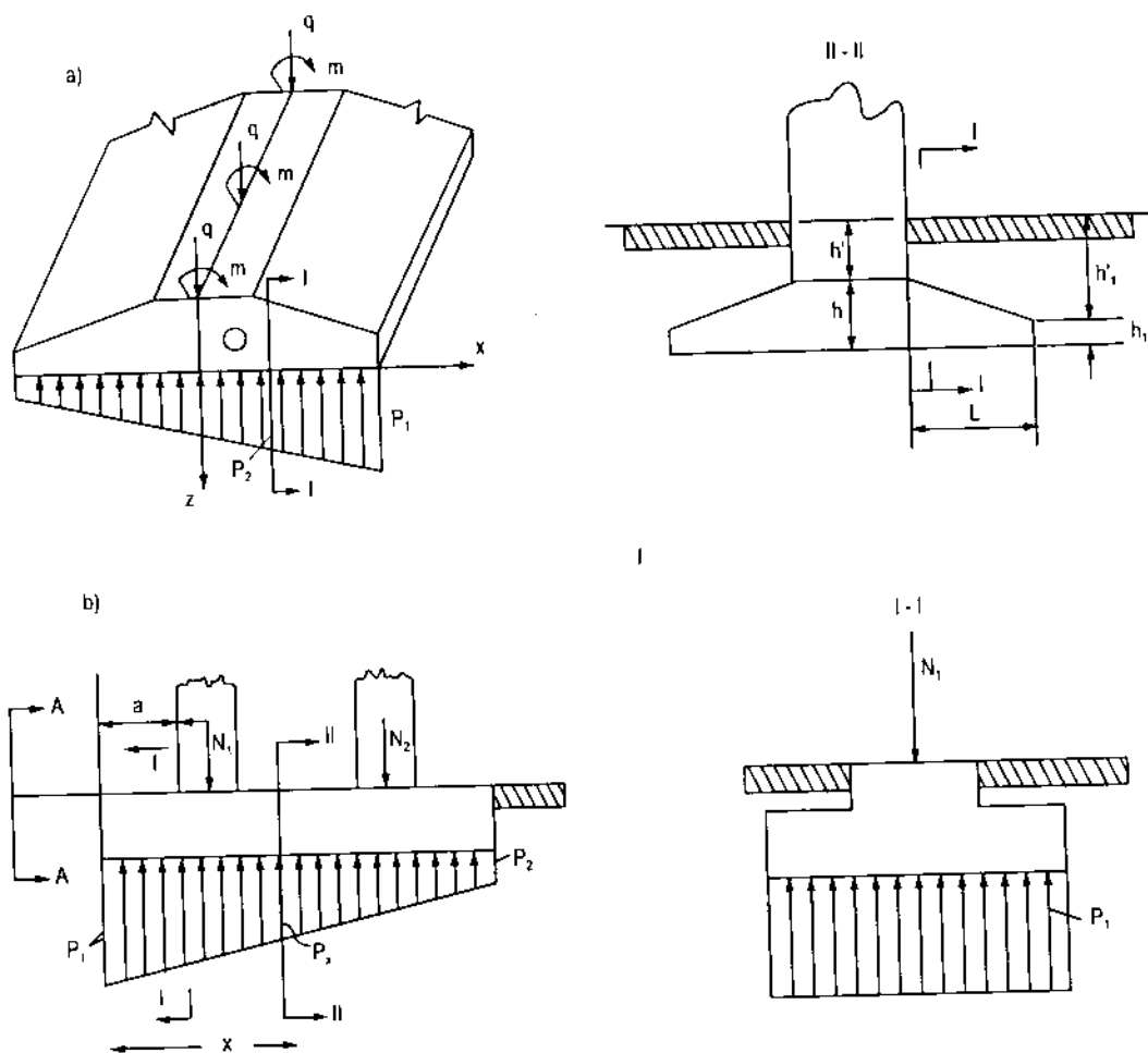
Hình 2.13. Sơ đồ tính toán móng.
