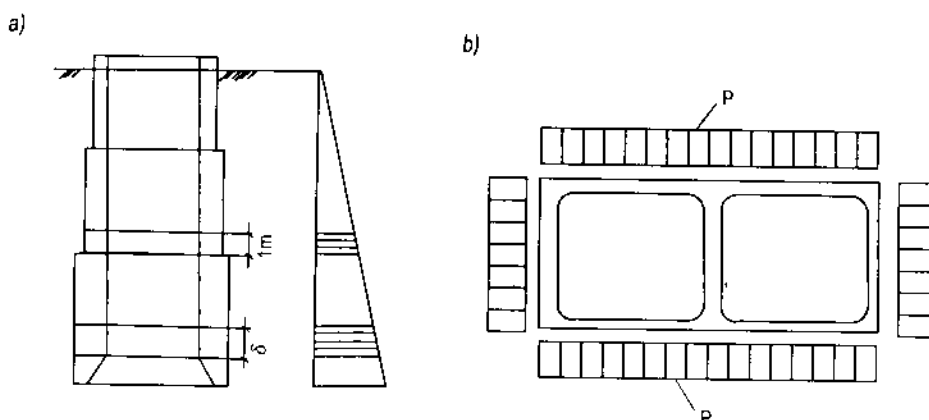
Hình 5.15. Tính tường giếng
