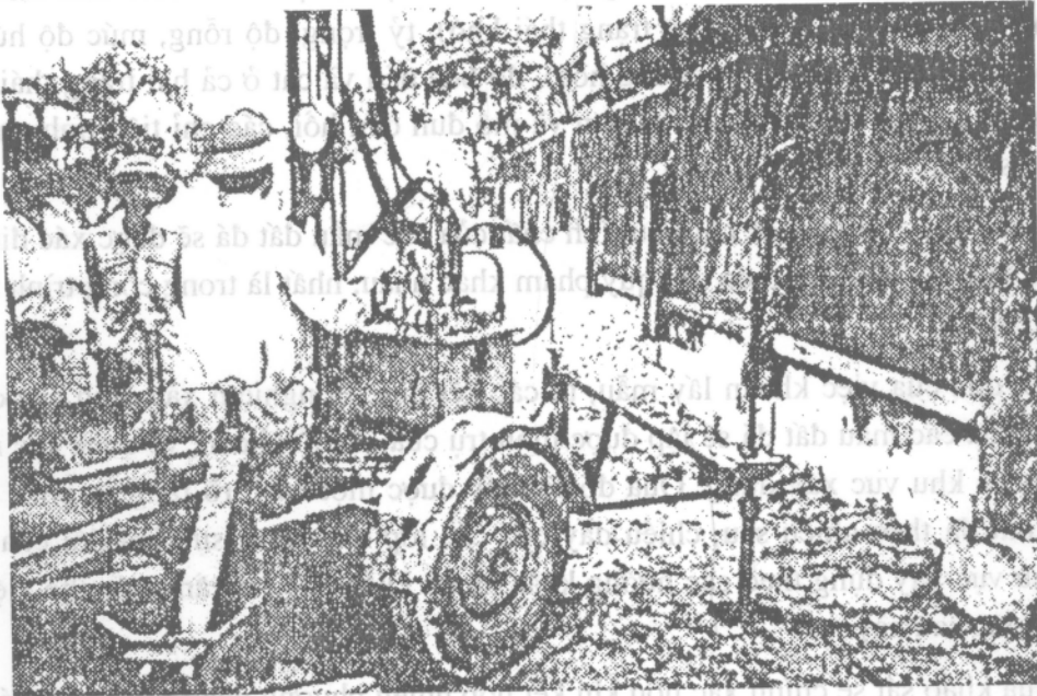
Hình 1.3. Máy xuyên tĩnh Gouda
