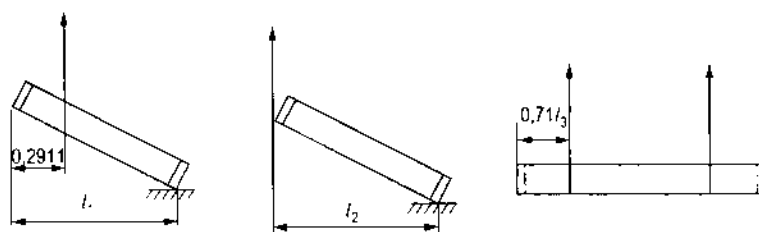
Hình 4.22. Sơ đồ treo trục cọc ống
