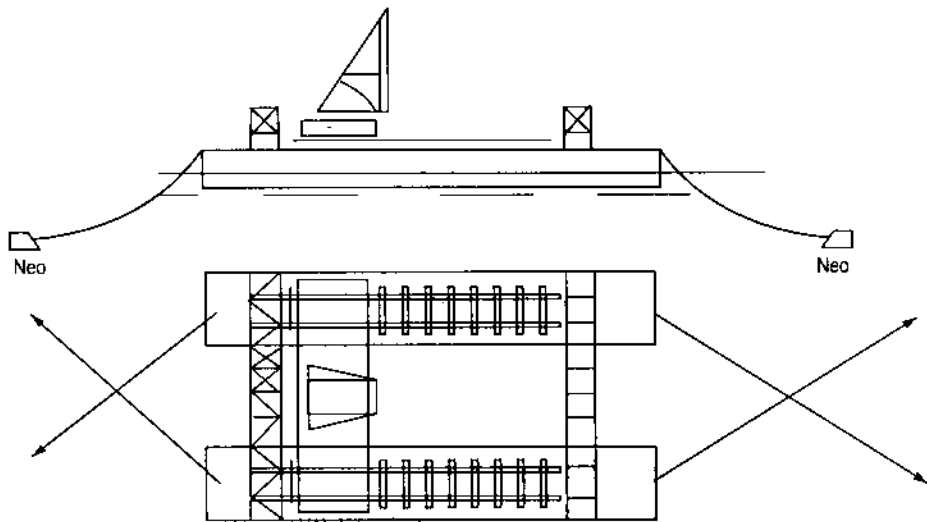
Hình 3.57. Búa đóng cọc trên hai phao
