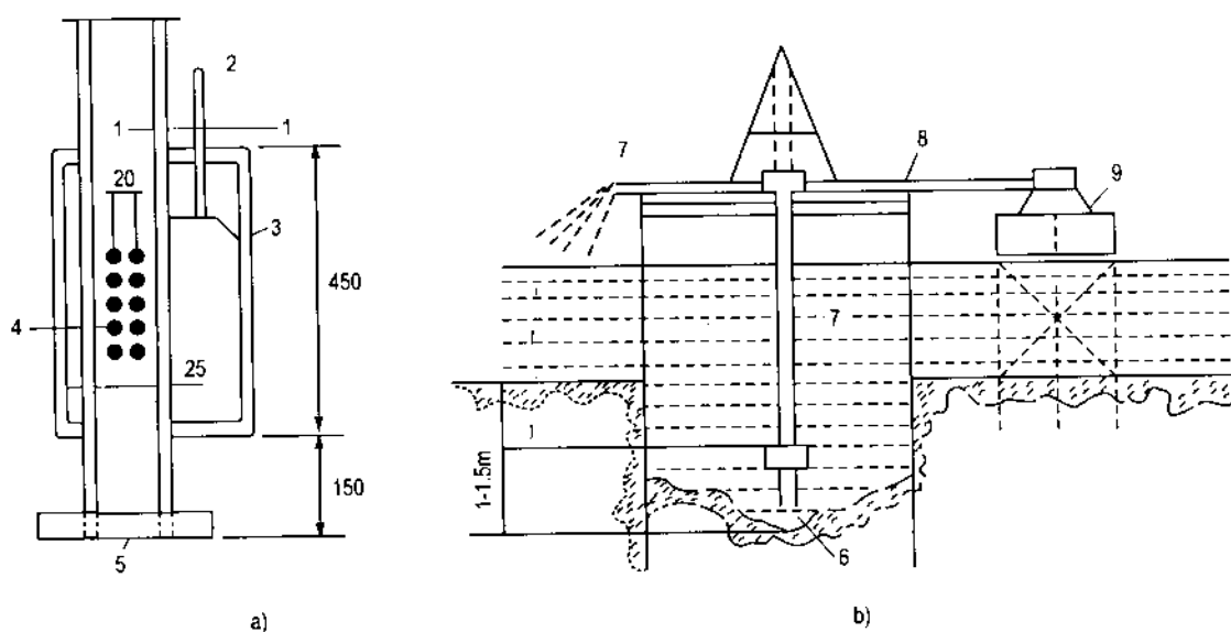
Hình 2.39. a) Máy hút bùn khí ép; b) Bố trí máy hút bùn khí ép trong vòng vây.
