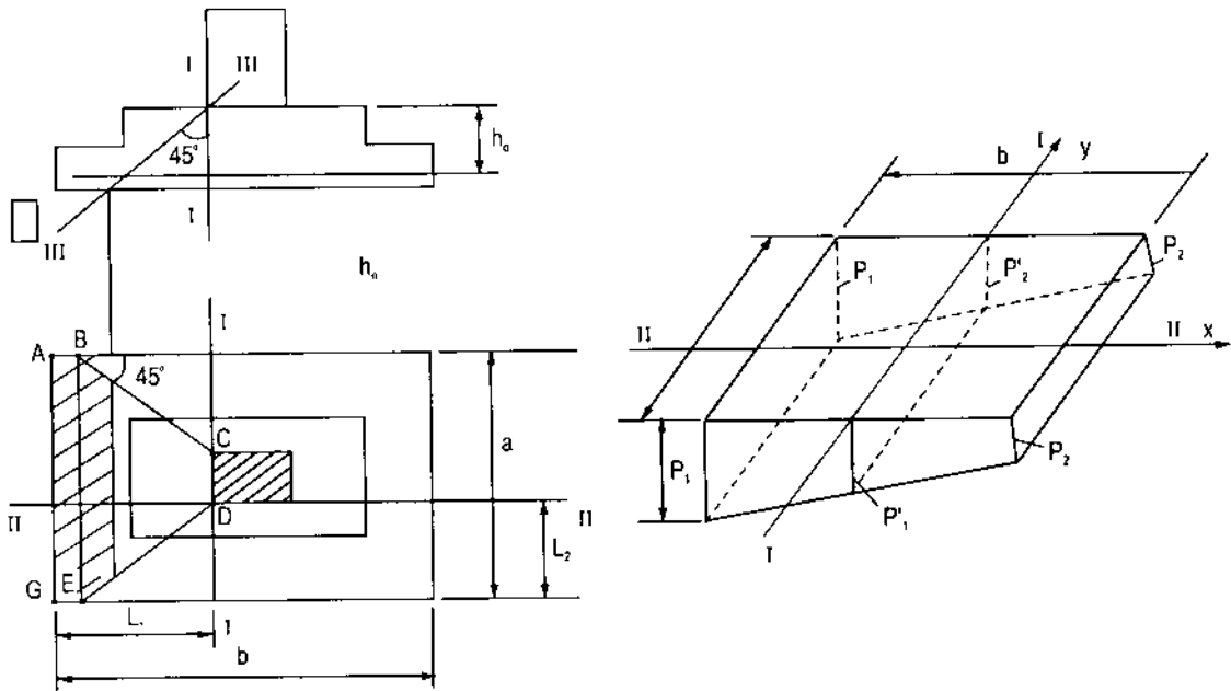
Hình 2.14. Sơ đồ tính toán mômen đế cột.
