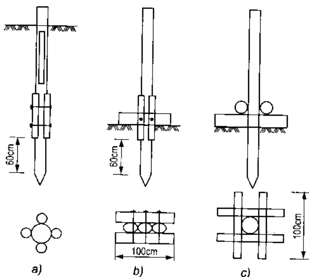
Hình 3.5. Cọc gỗ tăng cường
