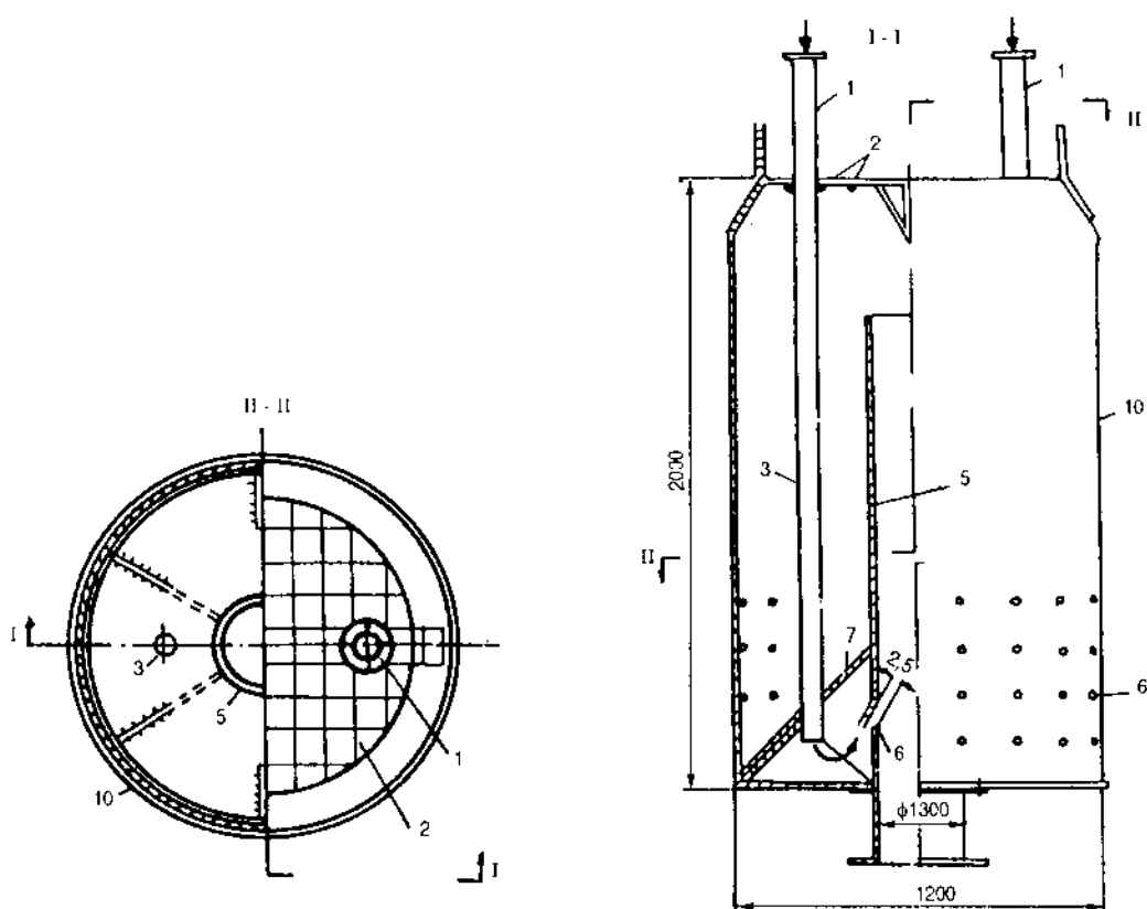
Hình 4.26. Thùng hút đá cuội sỏi
