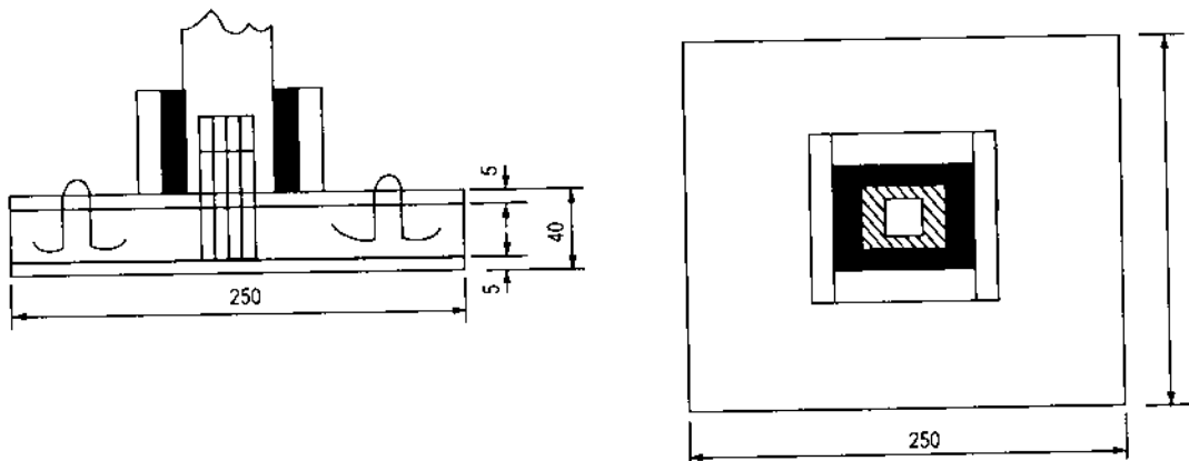
Hình 2.6. Móng bê tông cốt thép chân cầu vượt
