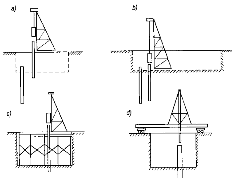
Hình 3.54. Các sơ đồ móng cọc
