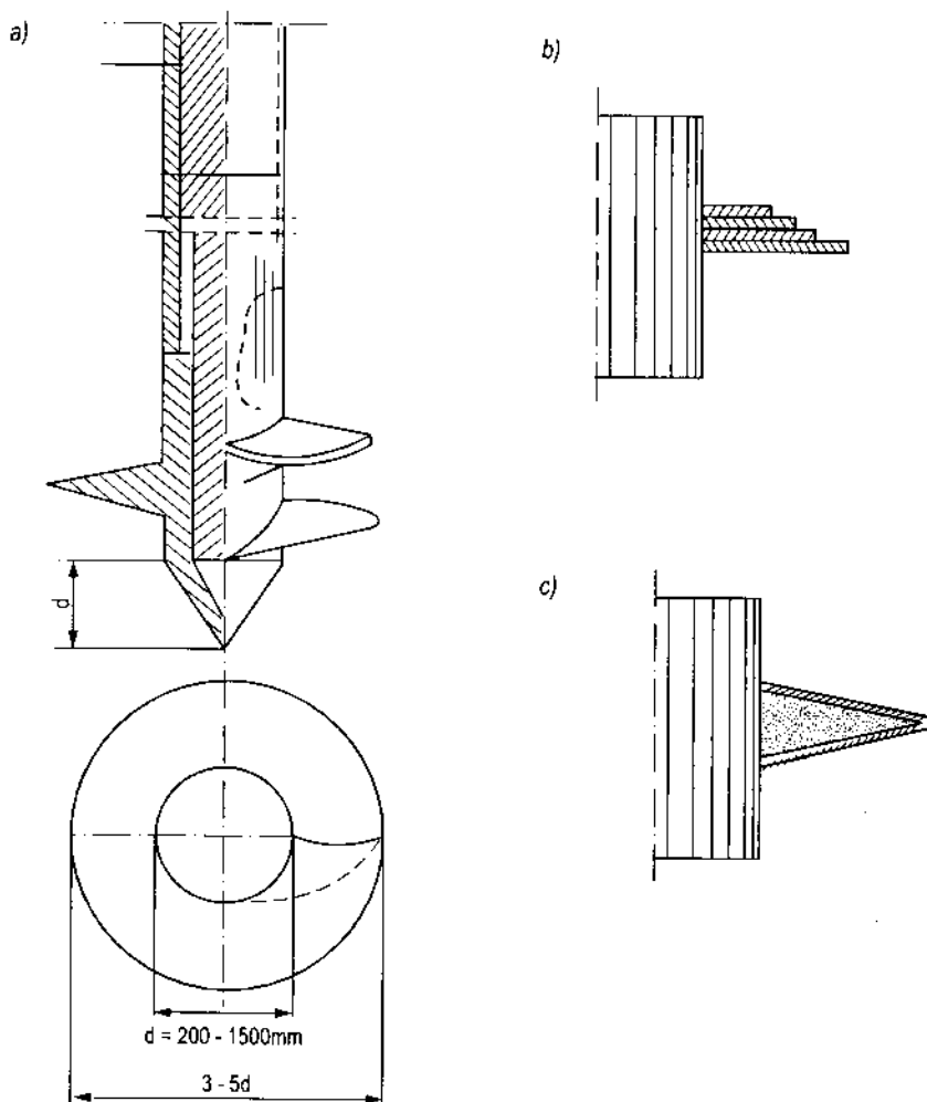
Hình 3.10. Cọc xoắn ốc
