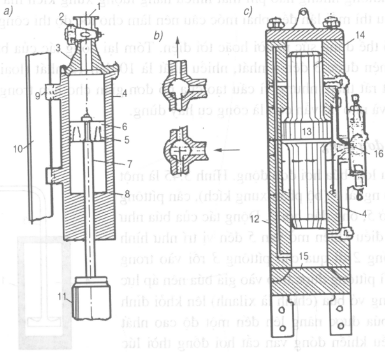
Hình 3.46. Búa hơi: a) Búa hơi đơn động; b) Sơ đồ van ba chiều trong búa hơi đơn động; c) Búa hơi song động. 1- Lỗ xả hơi; 2- Van 3 chiều; 3- Phần trên của xilanh; 4- Xilanh; 5 -Pittông; 6- Vòng nén; 7- Cán dẫn hướng; 8 - Lỗ để không khí và nước ngưng tụ thoát ra; 9- Ngàm trượt; 10- Cán dẫn hướng giá búa; 11- Cọc; 12- Xilanh; 13- Pittông; 14- Đầu pittông; 15- Đế xilanh; 16- Van điều chỉnh hơi nước.
