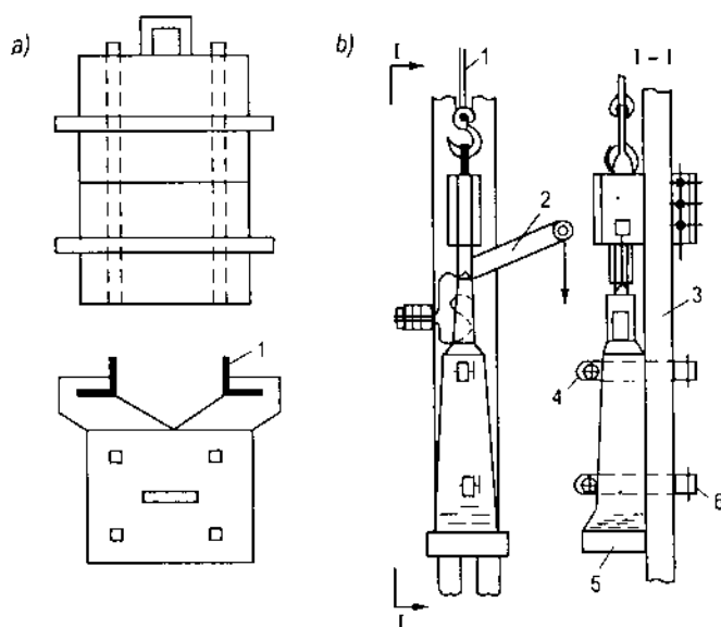
Hình 3.44. Búa kéo tay
