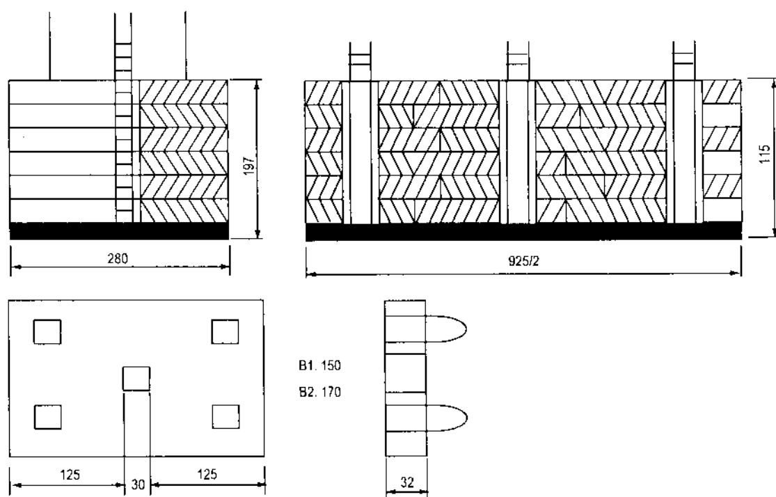
Hình 2.5. Móng bê tông lắp ghép khối lớn
