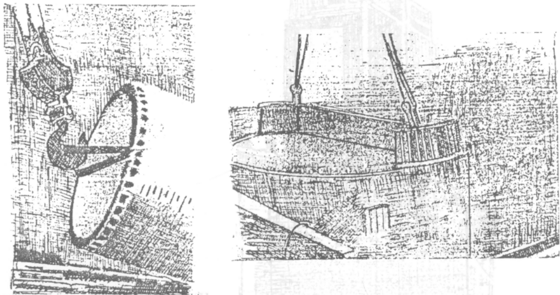
Hình 4.23. Dầm để nâng các loại cọc ống
