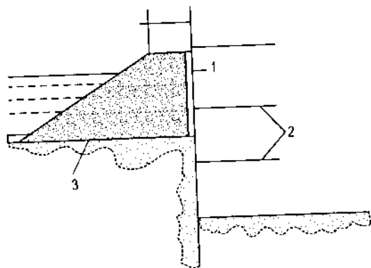
Hình 2.32. Cọc ván gỗ chống đơn
