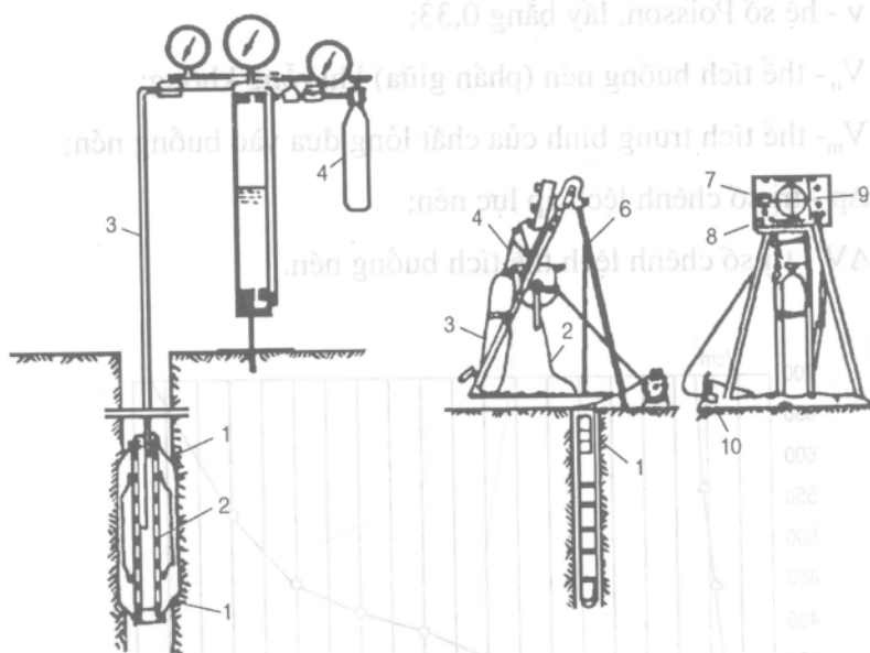
Hình 1.7. Thiết bị nén ngang các loại
