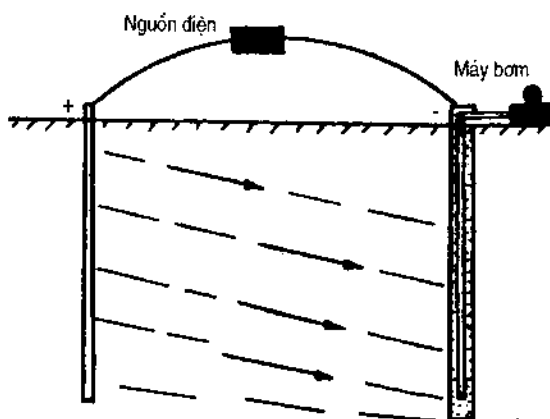
Hình 6.12. Phương pháp điện thấm
