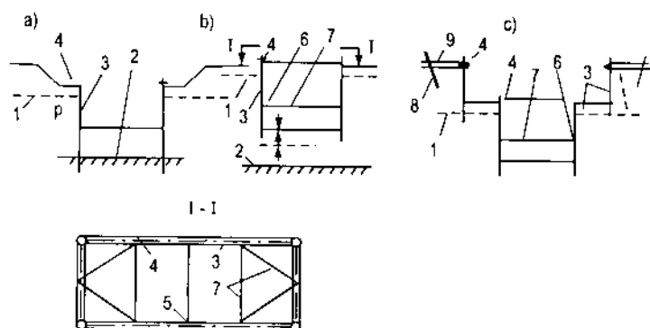
Hình 2.19. Sơ đồ chống hố móng
