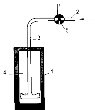
Hình 3.45. Búa đơn động
