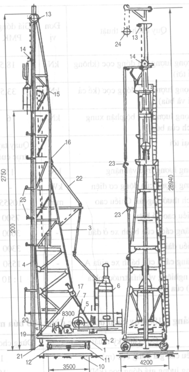
Hình 3.52. Giá đóng cọc vạn năng
