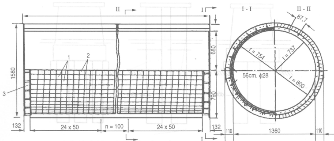
Hình 4.13. Cấu tạo cọc ống và cốt thép
