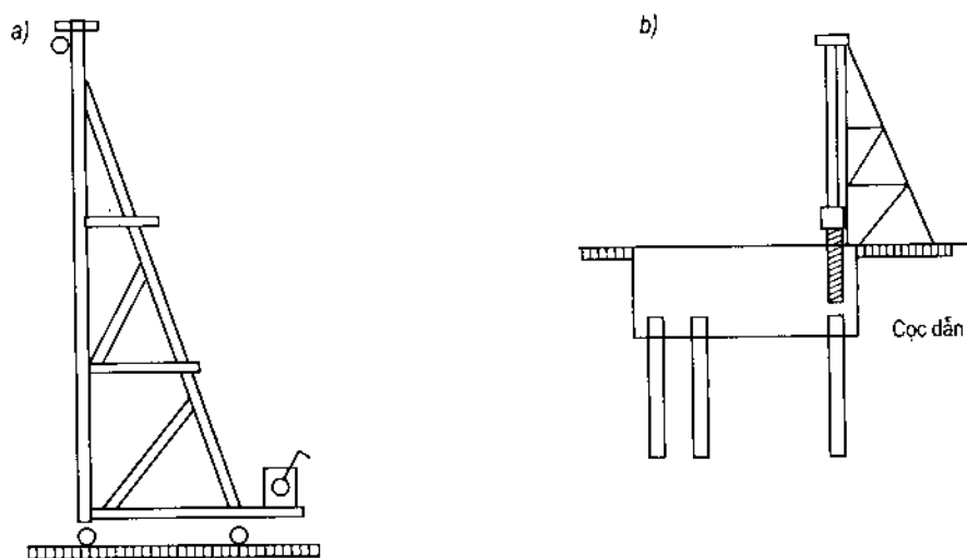
Hình 3.50. Giá gỗ tháo lắp
