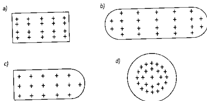
Hình 4.16. Các dạng bệ cọc ống
