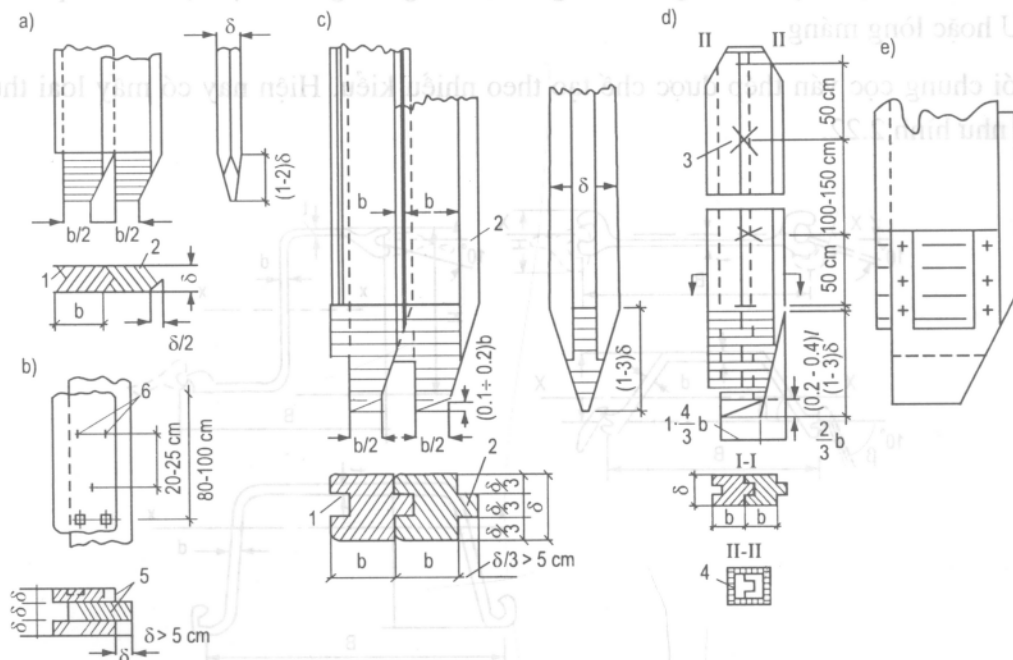
Hình 2.20. Cấu tạo cọc ván gỗ
