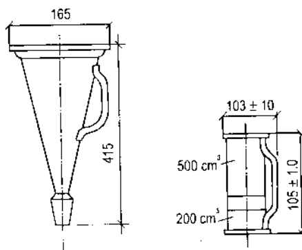
Hình 2.50. Phễu đo độ nhớt
