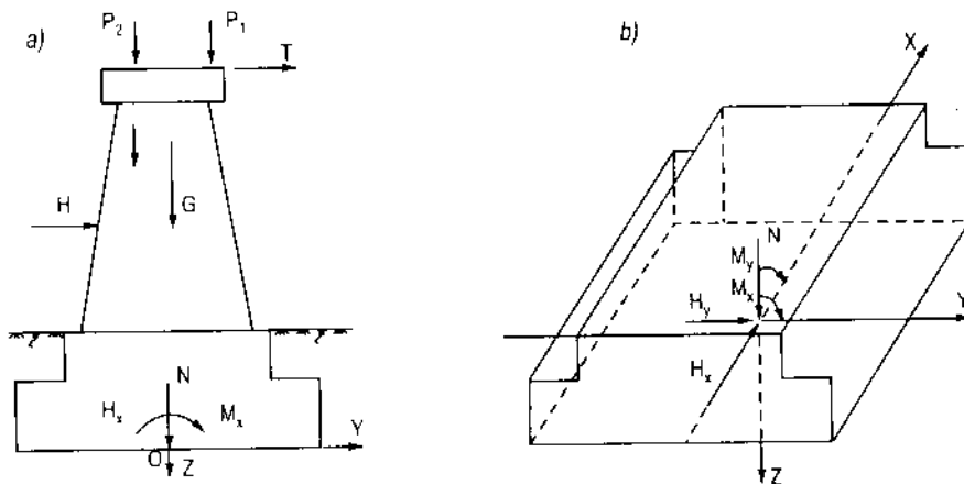
Hình 2.7. Chuyển các lực bên trên về trọng tâm đáy móng
