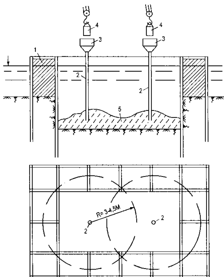
Hình 2.40. Sơ đồ đổ bê tông dưới nước
