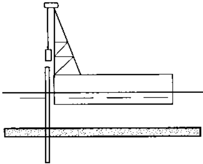
Hình 3.56. Đóng cọc trên phao
