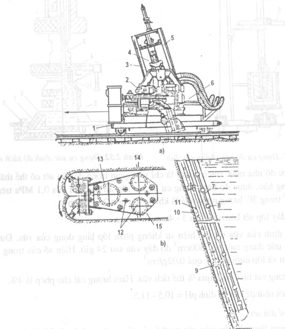
Hình 2.53. Máy đào bằng phương pháp xới và hút bùn
