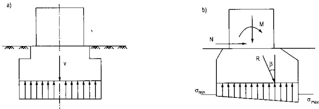
Hình 2.2. a) Lực tác dụng đúng tâm, cấu tạo móng đối xứng; b) Lực tác dụng lệch tâm, cấu tạo móng không đối xứng.
