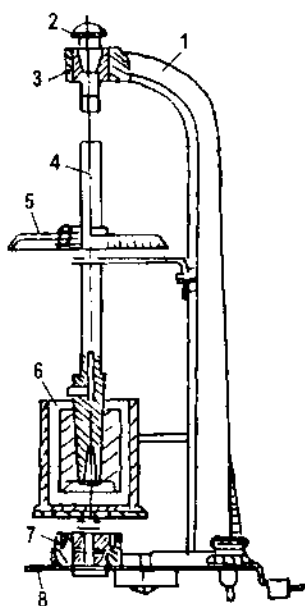
Hình 2.51. Dụng cụ đo sức chống cắt tĩnh
