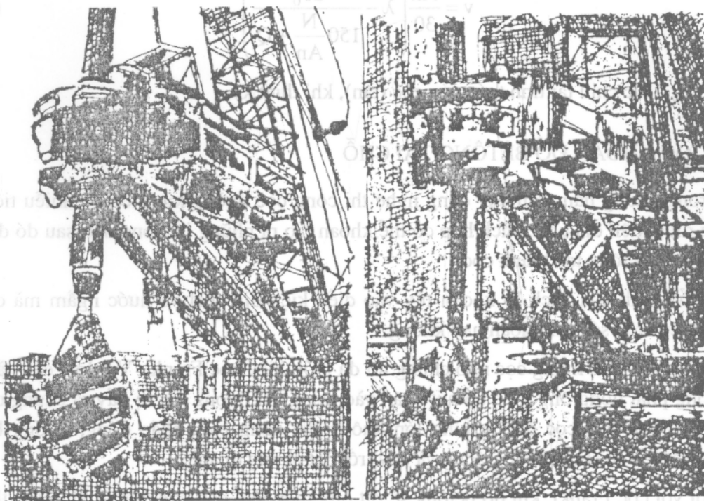
Hình 4.30. Mũi khoan xoắn tạo lỗ cọc
