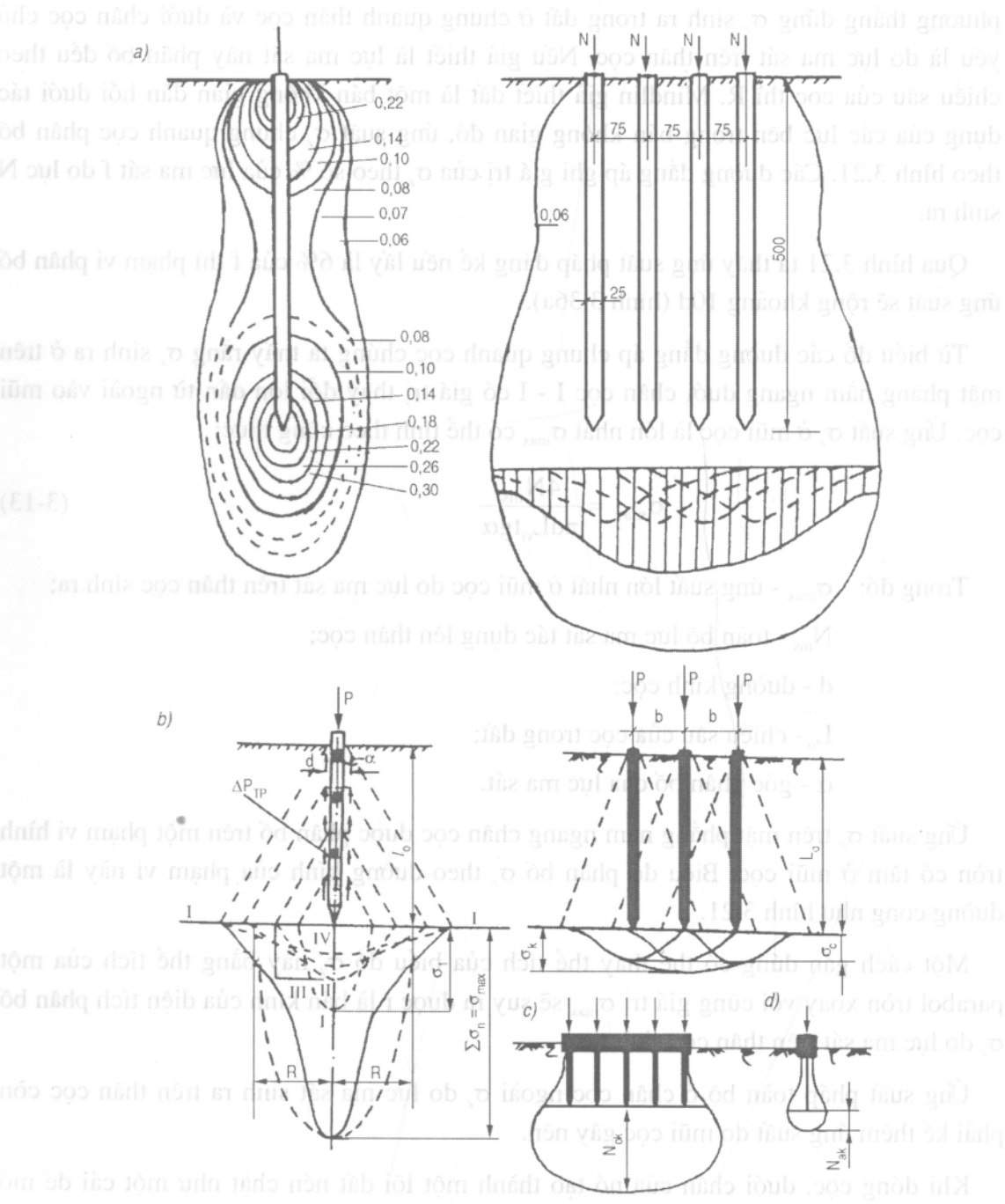
Hình 3.21. a) Biểu đồ phân bố ứng suất chung quanh thân cọc; b) Phân bố ứng suất dưới chân cọc đứng một mình.
