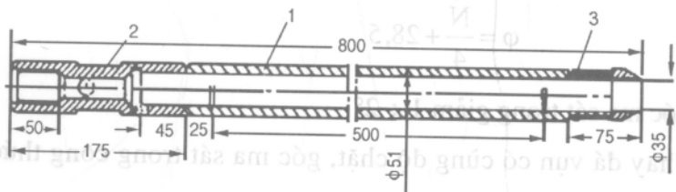
Hình 1.5. Thí nghiệm xuyên tiêu chuẩn SPT 1- Ống mẫu chế; 2- Đầu nối; 3- Mũi thép.
