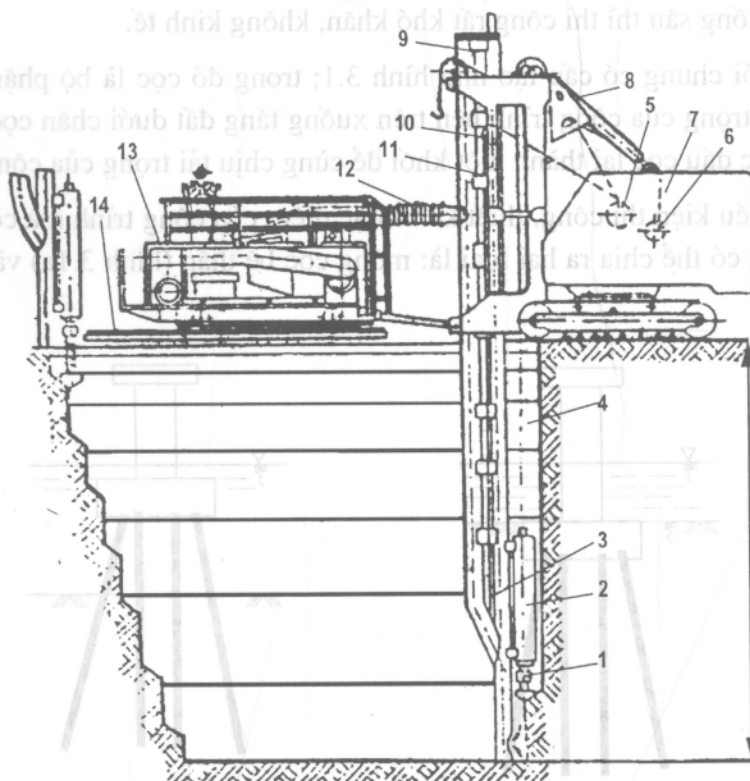
Hình 2.55. Một kiểu máy đào hào.
