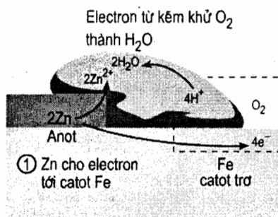
(b) Bảo vệ catot
