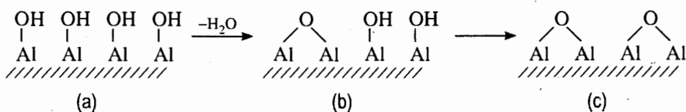
Hình 7.20. a) Nhôm oxit “hydroxyl hoá”, b) “Nhôm oxit “đề hydroxyl hoá từng phần” c) Nhôm oxit “đề hydroxyl hoá”
