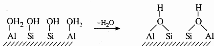
Hình 7.21. Sự hình thành tâm axit Brønsted ở nhôm silicat
