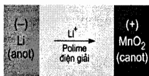
Hình 9.5. Pin liti rắn
