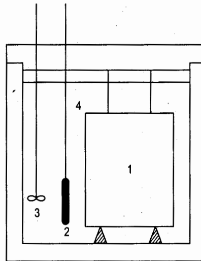
Hình 1.4. Sơ đồ một nhiệt lượng kế đơn giản
