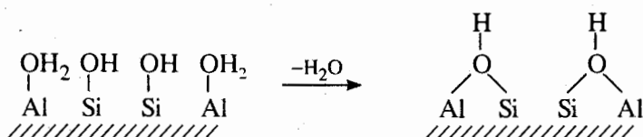
Hình 7.21. Sơ hình thành tâm axit Brostet ở nhôm silicat
