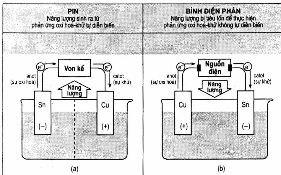
Hình 9.10. a) Phản ứng giữa Sn và Cu 2+ tự diễn biến ở pin sinh ra điện thế 0,48 V.
