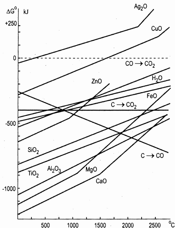
Hình 9.13. Giảm đồ Ellingham đối với sự khử oxit kim loại
