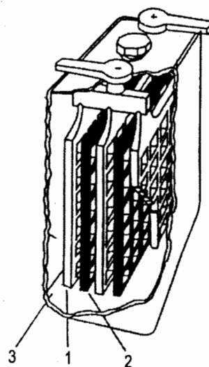
Hình 9.3. Ắc quy chì
