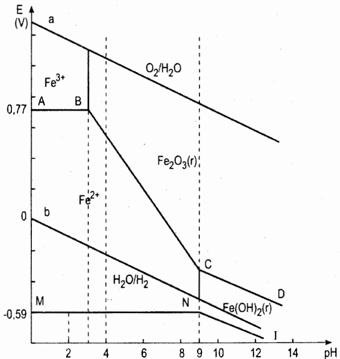
Hình 9.17. Giảm đồ E - pH của sắt
