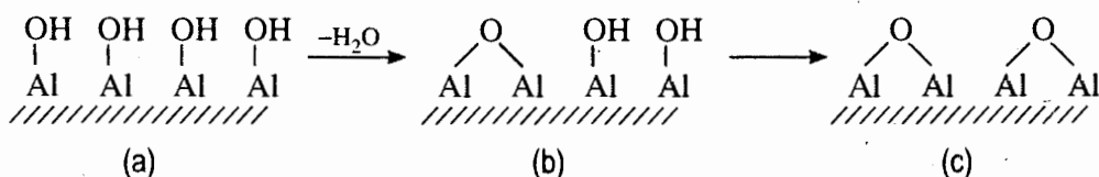
Hình 7.20. a) Nhôm oxit “hiđroxyl hoá”, b) “Nhôm oxit “đề hiđroxyl hoá từng phần” c) Nhôm oxit “đề hiđroxyl hoá”
