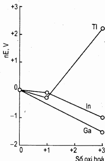
Hình 8.17. Biểu đồ Frost đối với các kim loại họ p nhóm gali
