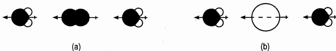
Hình 6.11. Phân tử nước gây ra lưỡng cực cảm ứng ở oxi (a) và ở argon (b)
