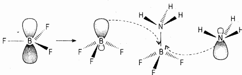
Hình 7.16. Tương tác giữa LUMO của BF_3 với HOMO của NH_3
