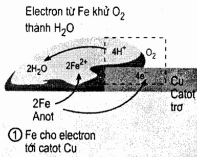
(a) Tăng cường ăn mòn
