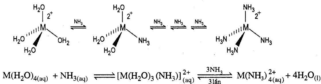
Hình 6.24. Sự thay thế nước từng nấc bởi amoniac
