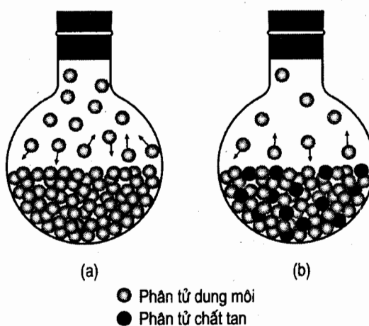
Hình 6.18 a) Dung môi nguyên chất b) Dung dịch chất tan không bay hơi
