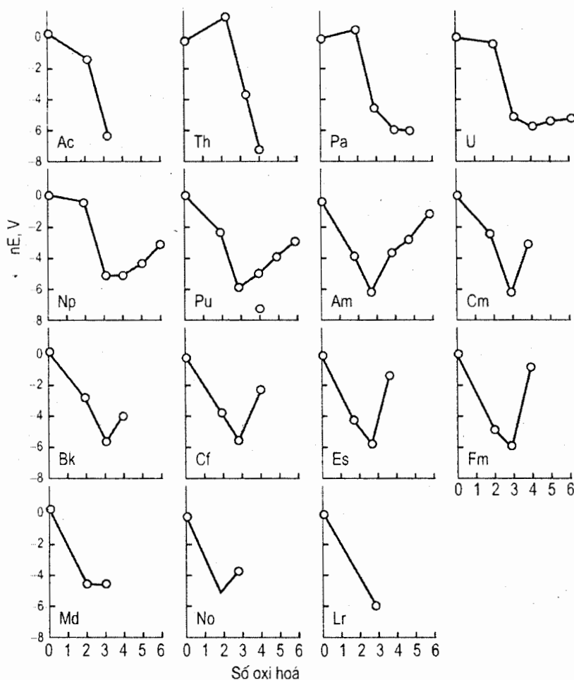
Hình 8.18. Giảm đồ Frost đối với một vài kim loại họ actini
