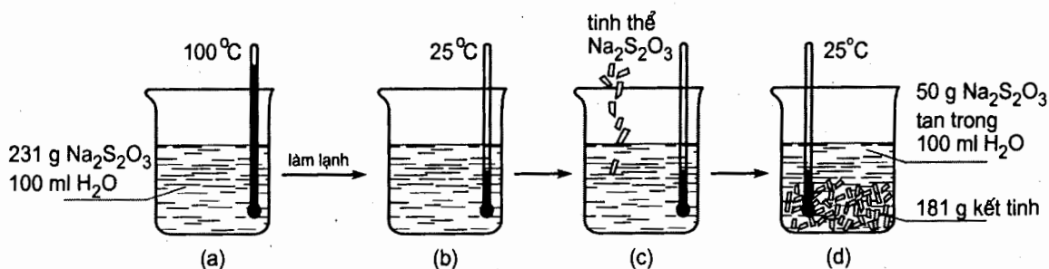
Hình 6.1. a) Dung dịch bão hoà ở 100 °C ; b) Dung dịch quá bão hoà (ở 25 °C chứa 231 g Na 2 S 2 O 3 trong 100 ml H 2 O ; c) Gây mầm tinh thể ; d ) 181 g Na 2 S 2 O 3 kết tinh còn lại dung dịch bão hoà ở 25 °C chứa 50 g Na 2 S 2 O 3 trong 100 ml H 2 O
