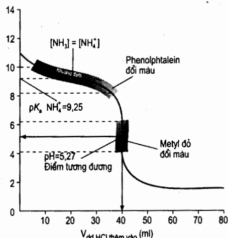
Hình 7.14. Chuẩn độ 40 ml dung dịch \text{NH}_3 0,1M bằng dung dịch \text{HCl} 0,1M
