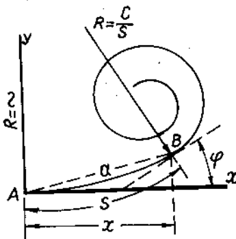
Hình 3-9. Đường cong chuyển tiếp dạng cloithoide
