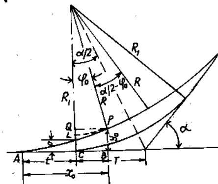
Hình 3-10. Cấu tạo đường cong chuyển tiếp dạng cloithoide
