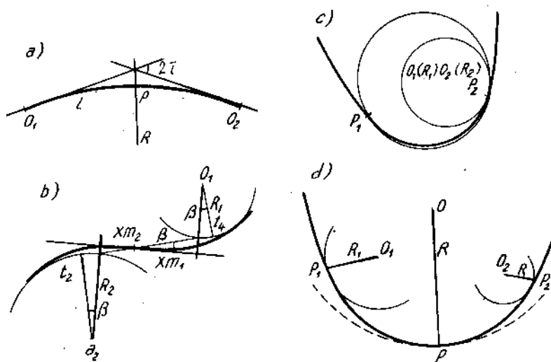
Hình 6-10. Các trường hợp vận dụng đường cong clothoide.
