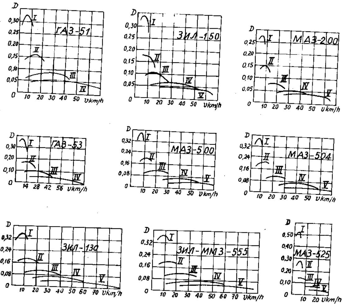
Hình 2-5a. Một số biểu đồ nhân tố động lực xe tải.
