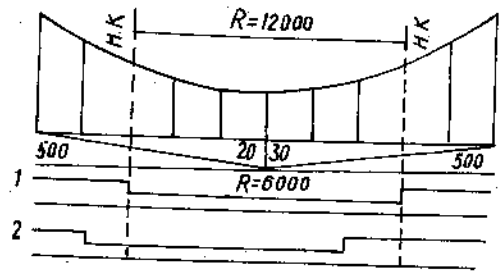
Hình 6-18. Phối hợp đường cong nằm và đường cong đứng. 1 - nền lồi ; 2 - cho phép.
