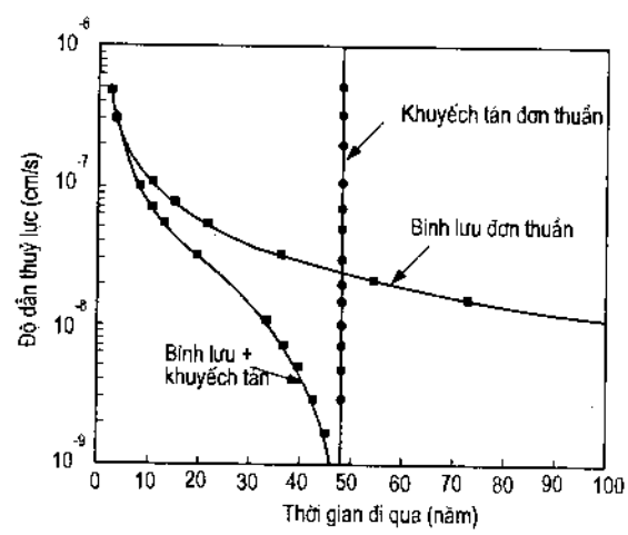
Hình 11.14: Thời gian chuyển qua tương ứng C/C_0 = 0,5 như là một hàm của độ dẫn thủy lực cho lớp sét lớt giả thuyết dày 3ft với độ rỗng trung bình là 0,50 và chịu gradient thủy lực là 1,33. Giả thiết hệ số khuếch tán là 6 \times 10^{-6} cm 2 /s (theo Shackelford, 1988)
