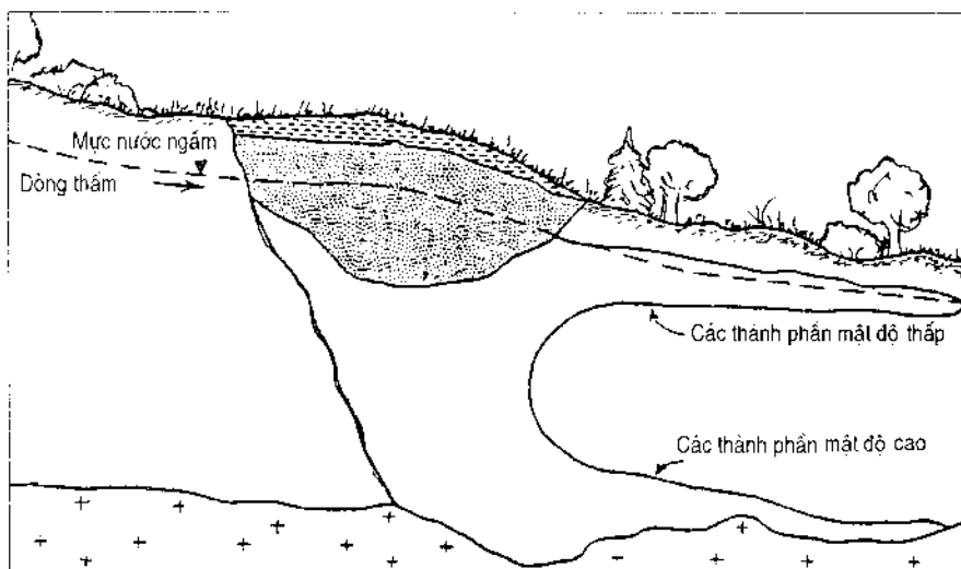
Hình 9.4: Sơ đồ di chuyển điển hình của chất ô nhiễm có mật độ biến đổi ở dưới đất (Hội Bảo vệ môi trường Mỹ, 1985)
