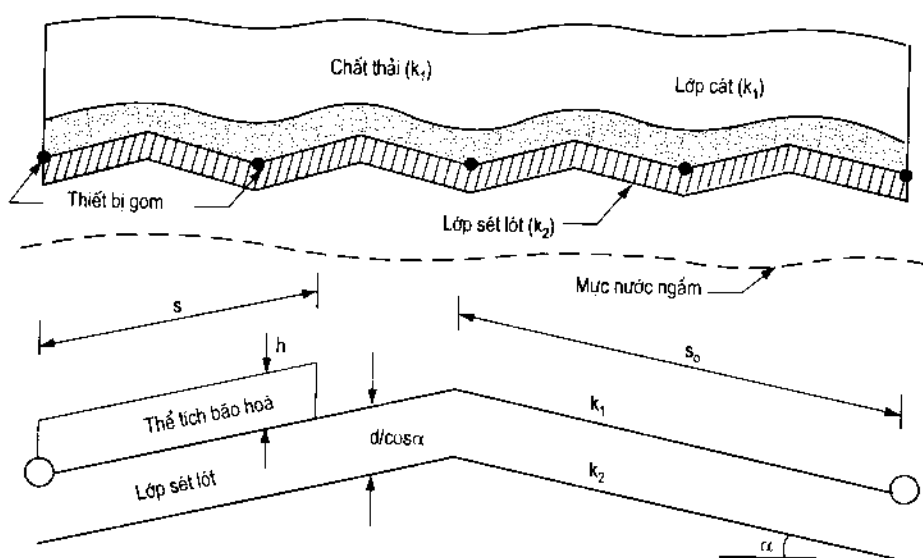
Hình 11.6: Sơ đồ mô hình bãi chứa rác thải cho thấy các thông số thích ứng hệ thu gom chất rửa lũa (Wong, 1977)
