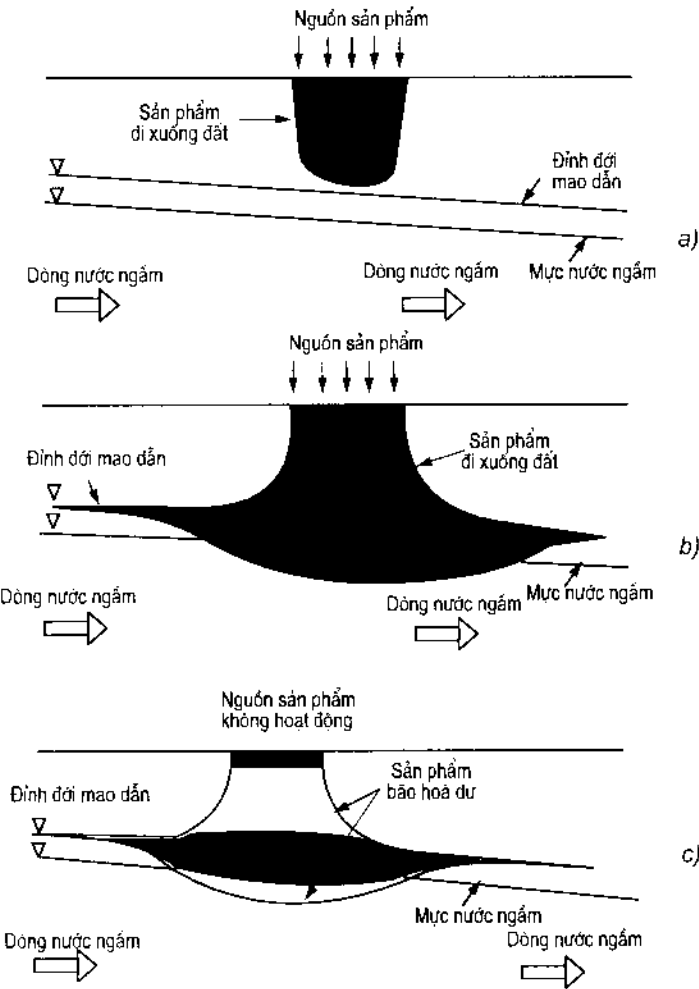
Hình 5.8: Chuyển động LNAPLs ở dưới mặt đất
