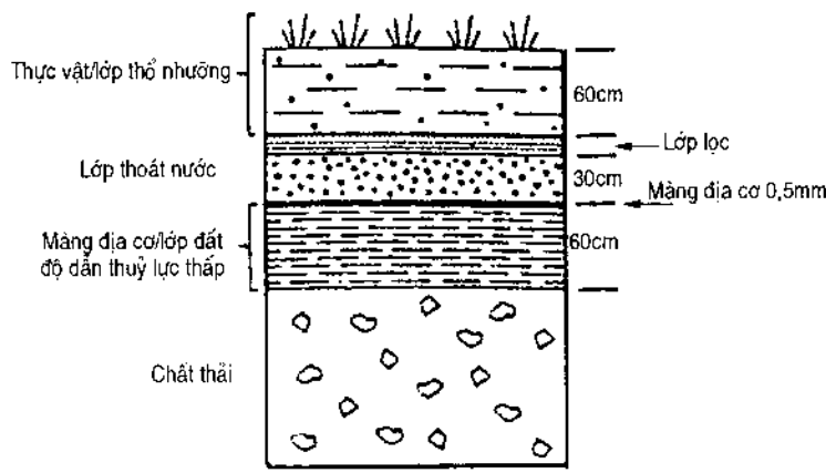
Hình 10.2: Hệ nắp phủ để nghị cho bãi chứa rác thải (Hội Bảo vệ môi trường Mỹ, 1991)
