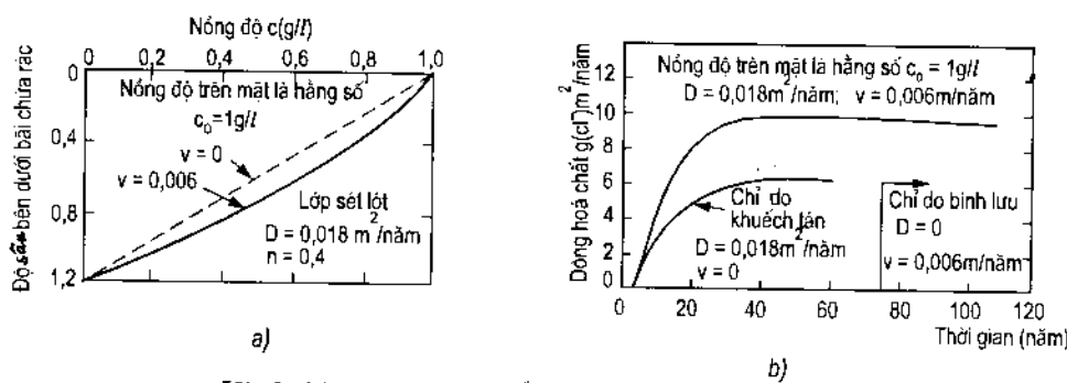
Hình 11.12: Vận chuyển khối qua các lớp sét lớt a) Mặt cắt nồng độ ở trạng thái ổn định trong lớp sét lớt dày 1 - 2m; b) Các dòng rửa lũ phụ thuộc thời gian tồn tại lớp lớt (theo Rowe, 1987)
