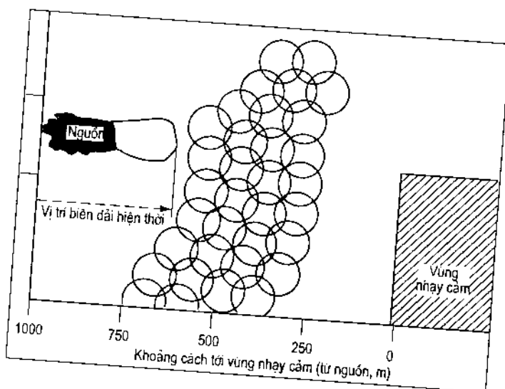
Hình 9.9: Sự sắp xếp có thể có của các điểm tác động để khống chế dòng di chuyển chất ô nhiễm về phía đôn nhạy cảm (Inyang, 1992)
