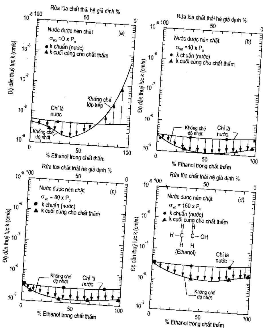
Hình 12.9: Độ dẫn thủy lực của đất sét đầm chặt được hỗn hợp chất rửa lựa của chất thải rắn thành phố - ethanol thấm kế tiếp đất sét ẩm chịu ứng suất trước tại các mức ứng suất hiệu quả thẳng đứng khác nhau (Fernandez và Quigley, 1991)
