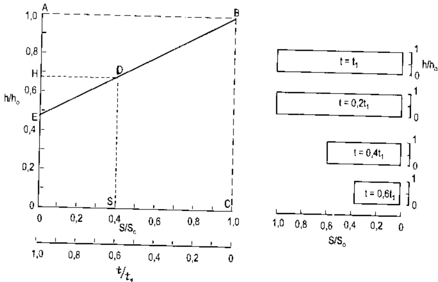
Hình 11.7: Lời giải cho bài toán kết hợp rò rỉ qua vật chất và thu gom chất rửa lũa:
