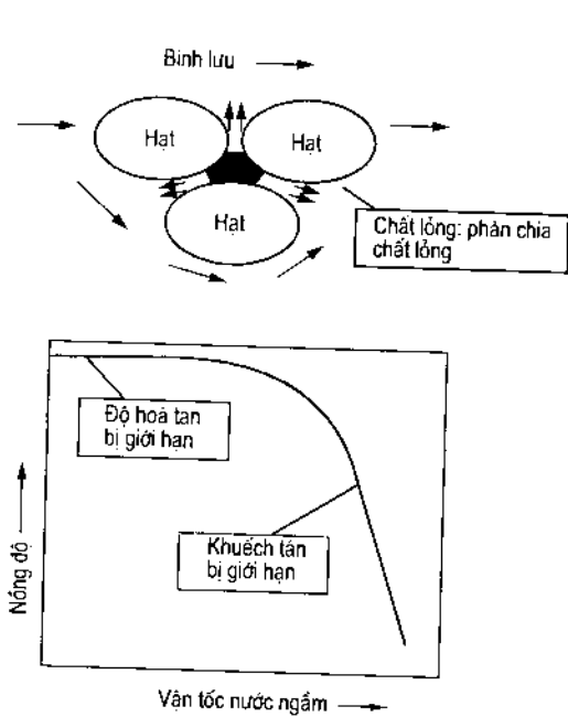
Hình 8.3: Sơ đồ mô tả các giới hạn độ hoà tan và độ khuếch tán cho các hệ bơm và xử lí (Keeley, 1989)
