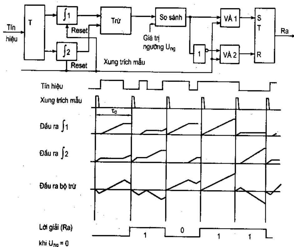
Hình 14-3 : Sơ đồ khối và đồ thị của trích mẫu phương pháp tích phân.
