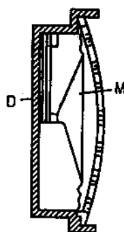
Hình 3-17 : Cấu tạo micro áp điện.
