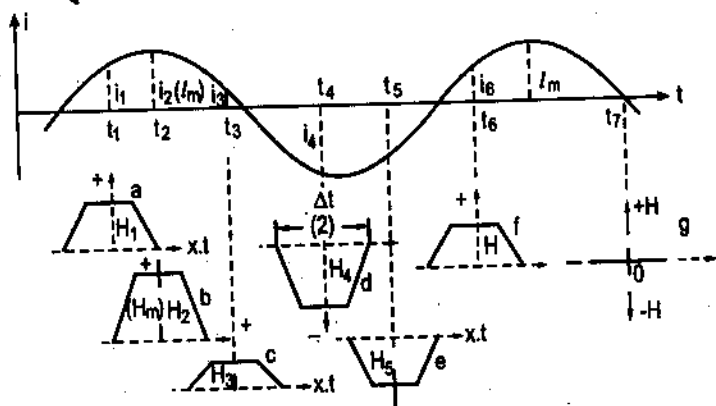
Hình 5-7 : Xung trường đầu từ ghi âm ở tần số thấp.
