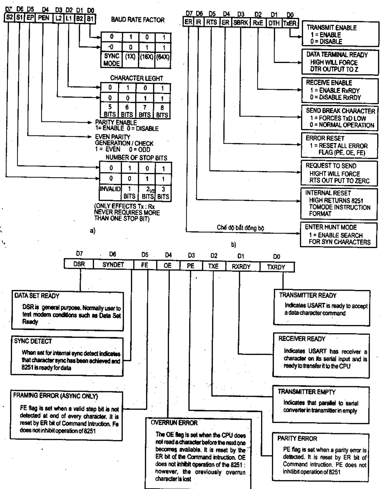
Hình 15-7 : Đặc điểm tín hiệu 8251A
