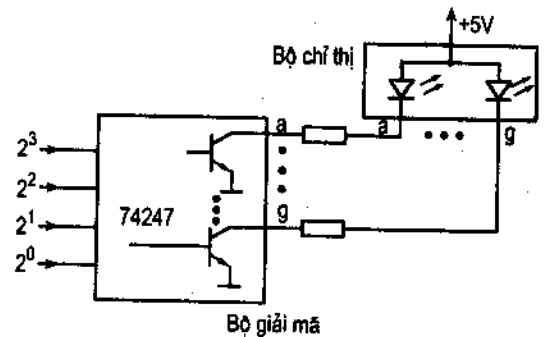
Hình 10-5 : Mạch giải mã đầu nối với LED 7 thanh.
