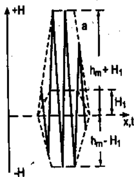
Hình 5-10 : Dạng xung đầu từ ghi âm có thiên từ.
