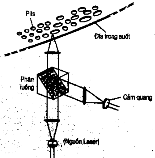
Hình 6-2 : Dùng tia laser để đọc tín hiệu trên C.D. (Nguồn laser như cái đèn, phần tử cảm quang như con mắt, dòng pit như dòng chữ).
