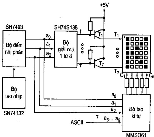
Hình 10-7 : Sơ đồ điều khiển ma trận 5 \times 7 LED.
