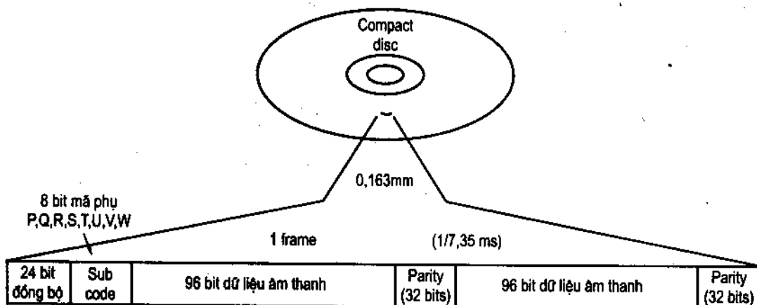
Hình 6-3 : Một khung số liệu trên đĩa trước EFM và cài xen (288 bit). Trừ 24 bit đồng bộ, số liệu còn lại trong khung phải EFM để tạo ra tổng số 588 bit mã hóa.
