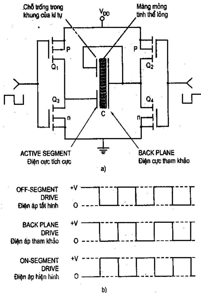
Hình 10-2 : Sơ đồ mạch tạo tín hiệu E cho LCD : a) mạch ; b) tín hiệu.
