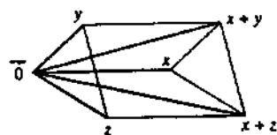
Tính chất 5): tính bất biến qua phép tịnh tiến
