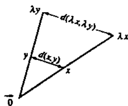
Tính chất 4): tính thuần nhất dương
