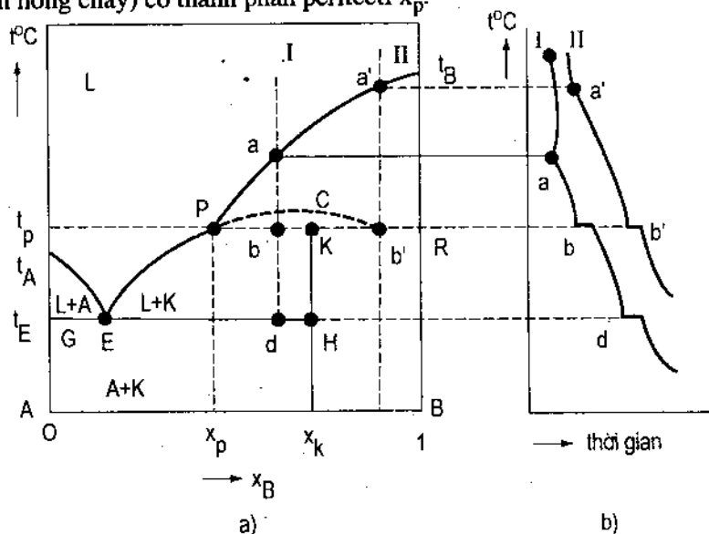
Hình XIV-9. a) Giản đồ pha hệ 2 cấu tử có hợp chất nóng chảy không hoàn nguyên ; b) đường nguội.
