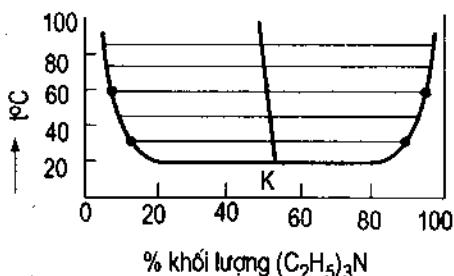
Hình XIV-14. Hệ nước - trietylamin có điểm hoà tan tối hạn dưới
