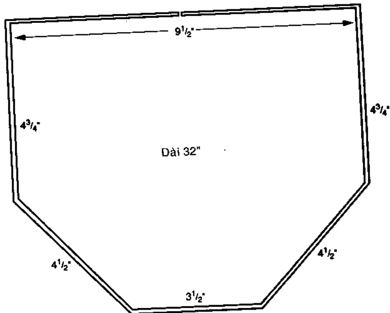
Hình 8.6. Hình chiếu đứng của khung uốn từ thanh nhôm 1/8" \times 1/2" \times 32" .
