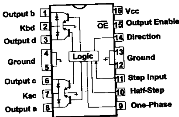
Hình 10.7. Vi mạch UCN-5804 của bộ điều khiển động cơ bước.
