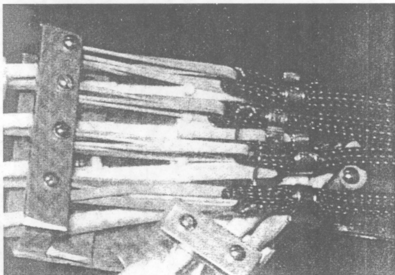
Hình 16.26. Cơ bắp không khí, dây cao su, và phần kéo ngón tay được nối với nhau trong bàn tay máy hoàn chỉnh.
