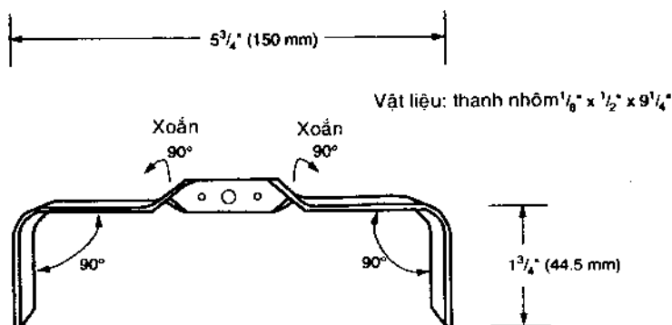
Hình 11.9. Chân giữa.
