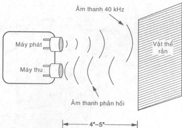
Hình 5.34. Sơ đồ thiết bị phát hiện va chạm bằng sóng siêu âm.
