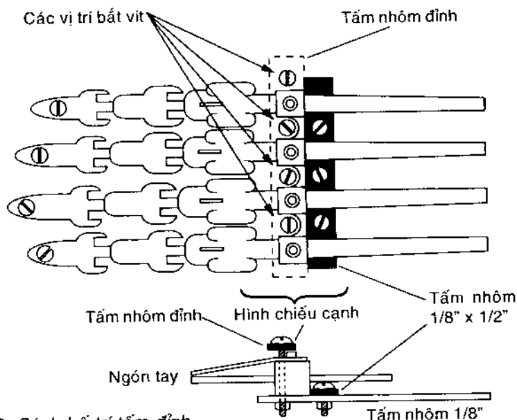
Hình 16.22. Cách bố trí tấm nhôm.
