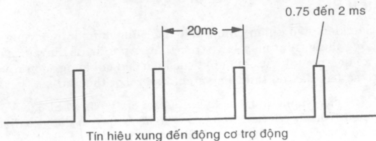
Hình 9.3. Chiều rộng xung được dùng để điều khiển động cơ trợ động.
