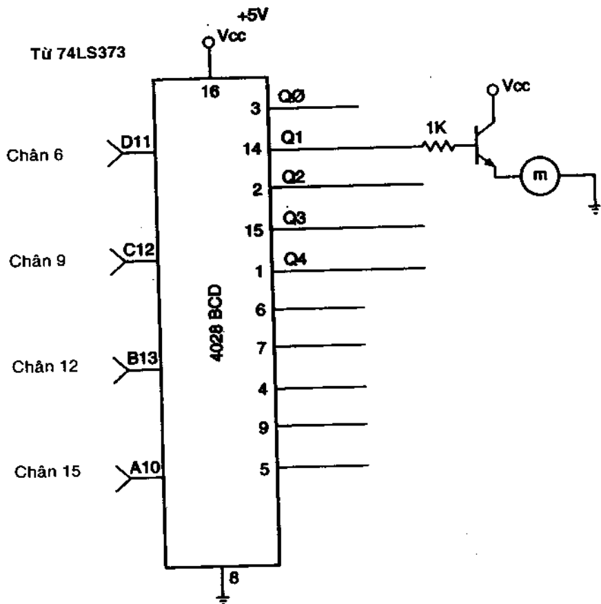
Hình 7.6. Mạch giao diện dùng cho xe R/C cải tiến.
