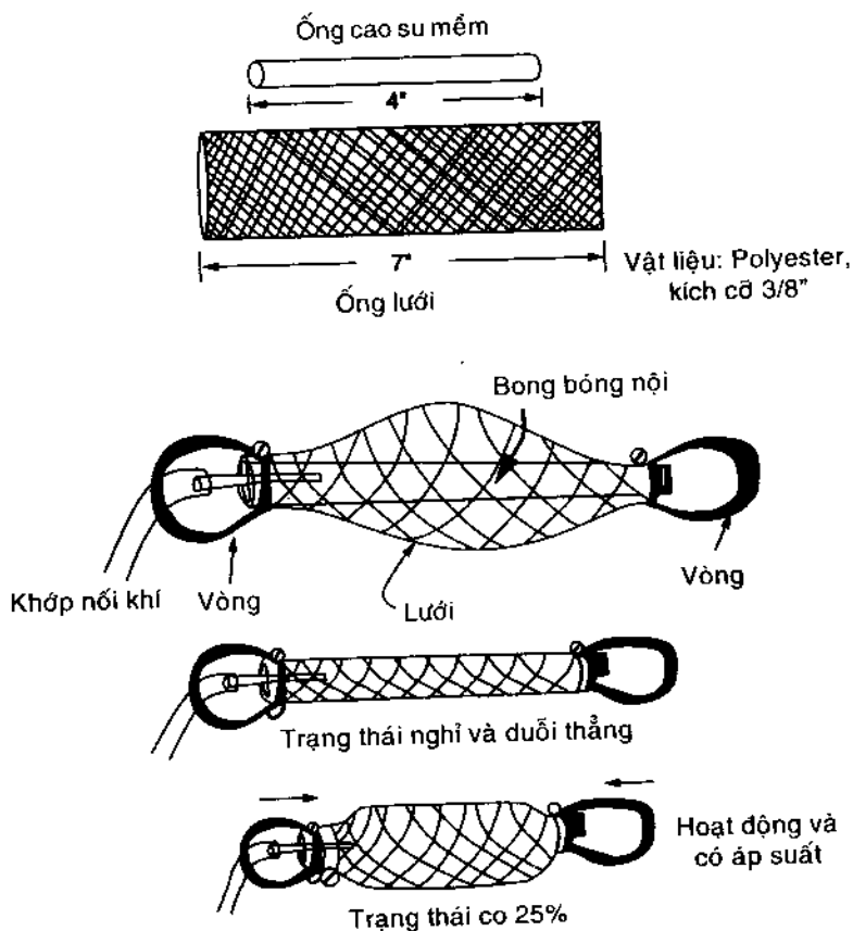
Hình 4.1. Chức năng và cấu tạo của cơ bắp khí.
