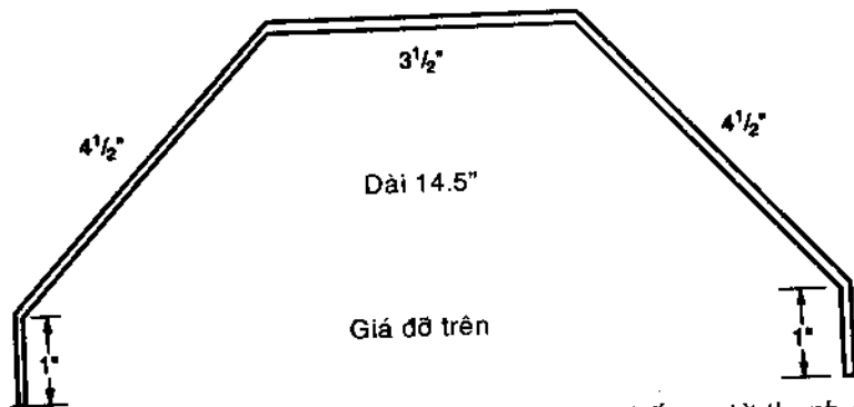
Hình 8.8. Hình chiếu cạnh của giá đỡ trên được chế tạo từ thanh nhôm 1/8" \times 1/2" \times 14.5" .
