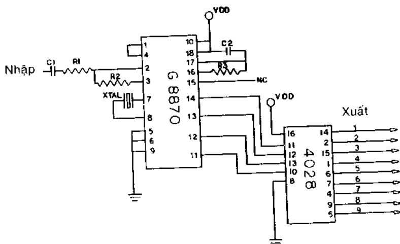
Hình 5.26. Sơ đồ thiết bị nhận DTMF với bộ chuyển đổi BCD-thập phân.
