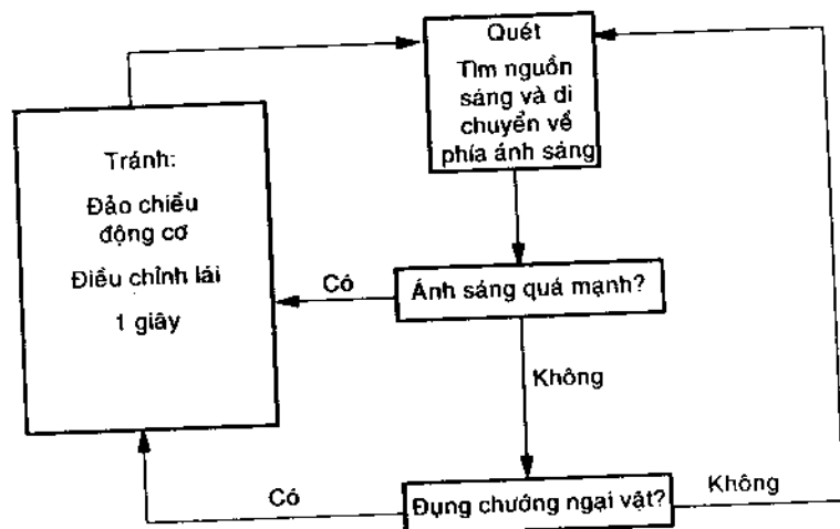
Hình 8.17. Lưu đồ chương trình.
