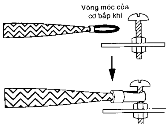
Hình 16.25. Cách gắn đầu đối diện của cơ bắp không khí với ốc máy để kéo đuôi cơ bắp không khí.
