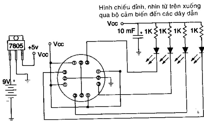
Hình 5.30. Mạch thử nghiệm la bàn digital sử dụng bốn LED.
