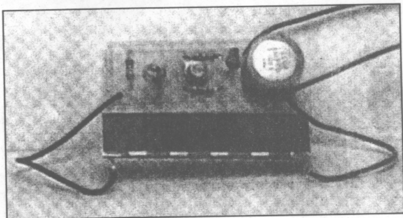
Hình 3.4. Động cơ mặt trời hoàn chỉnh
