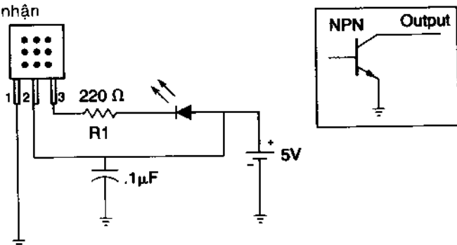
Hình 5.12. Sơ đồ thiết bị nhận hồng ngoại.
