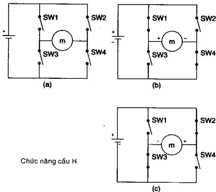
Hình 4.16 Cầu-H sử dụng các công tắc.
