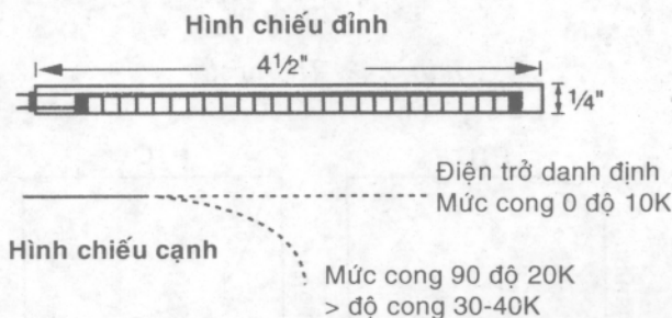
Hình 5.41. Đồ thị điện trở của bộ cảm biến uốn cong.
