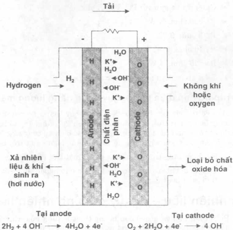
Hình 3.9. Pin nhiên liệu kiềm (KOH)
