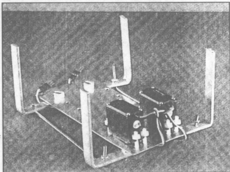
Hình 11.11. Mặt dưới robot sáu chân với hai động cơ trợ động phía trước.
