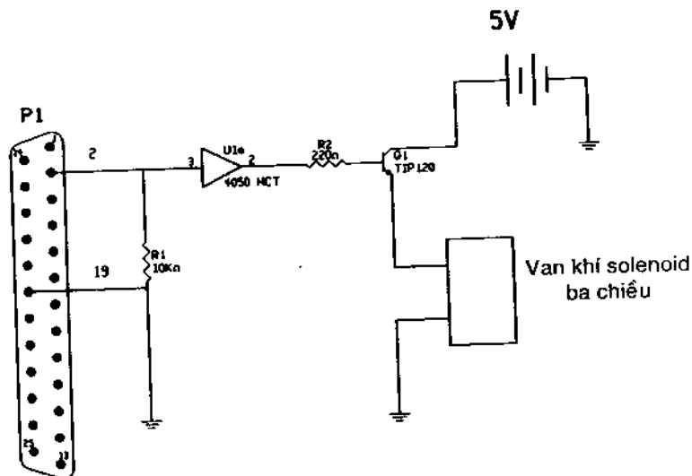
Hình 16.16. Sơ đồ bộ điều khiển van khí.
