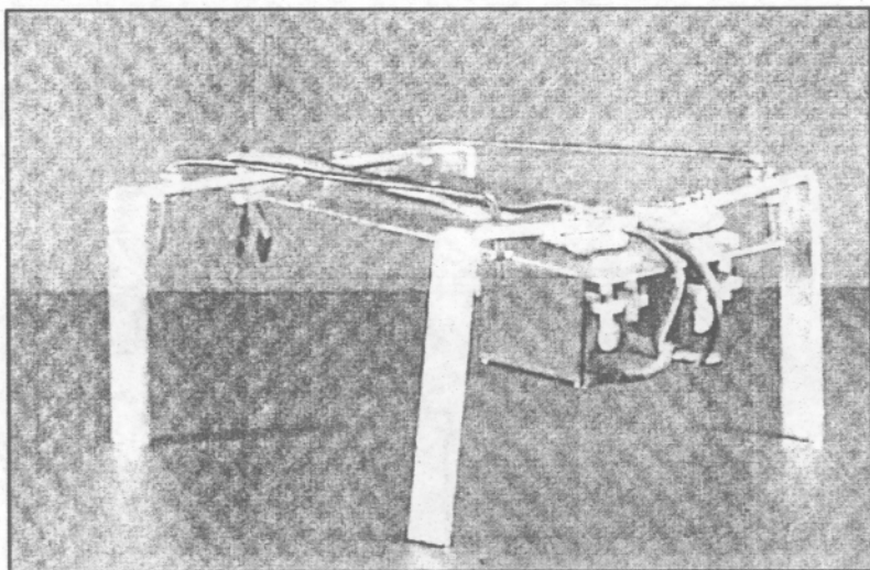
Hình 11.12. Robot sáu chân đang lắp ráp với hai động cơ trợ động ở phía trước.
