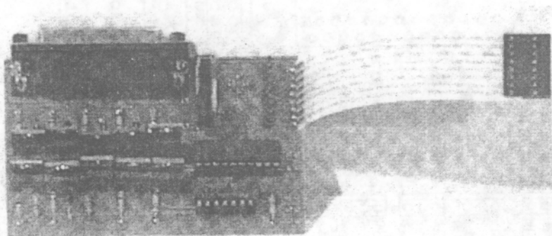
Hình 15.7. Giao diện PC sau khi lắp ráp (mặt trên).
