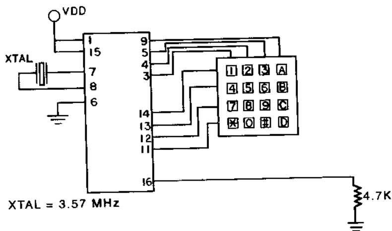
Hình 5.18. Mạch điện mã hóa DTMF sử dụng ma trận bàn phím 3 x 4.
