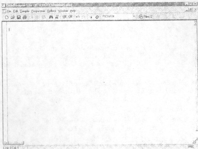
Hình 6.17. CodeDesigner Lite
