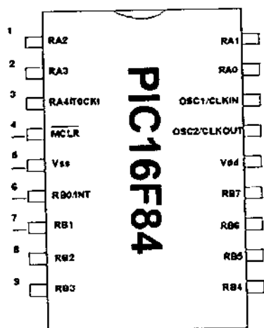
Hình 6.3. Bộ vi điều khiển 16F84
