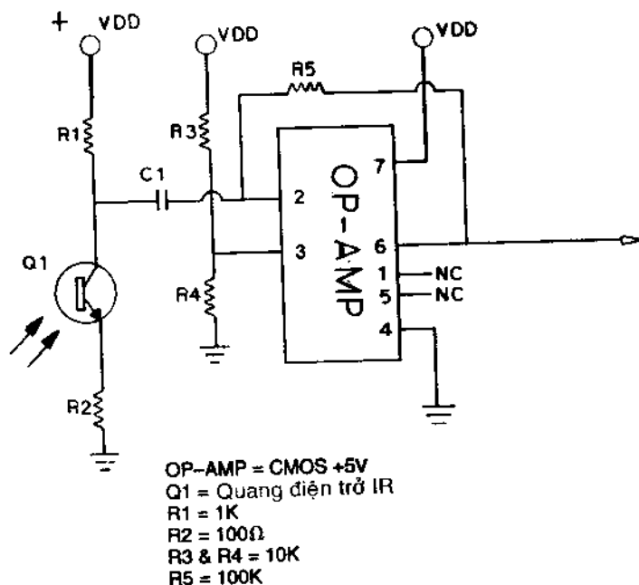
Hình 5.25. Sơ đồ mặt trước của thiết bị nhận DTMF IR
