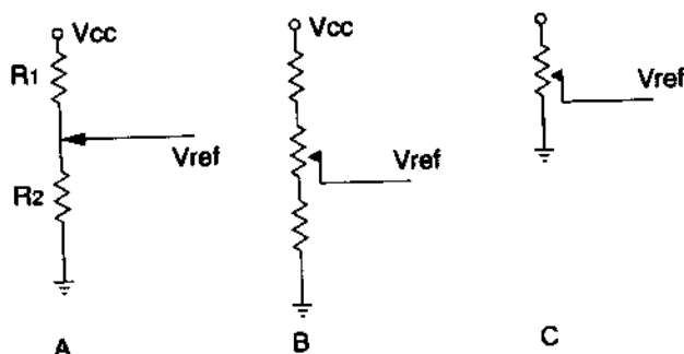
Hình 5.2. Các bộ chia điện áp A, B, và C.
