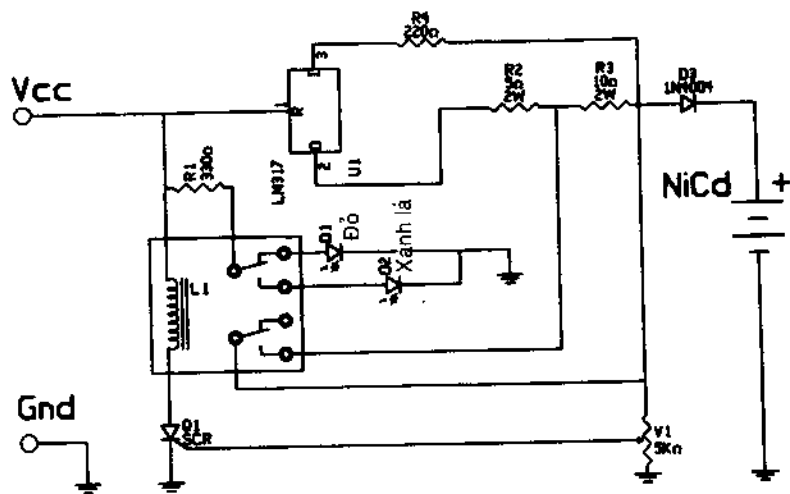
Hình 3.8. Sơ đồ mạch của bộ nạp điện
