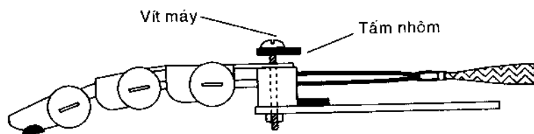
Hình 16.24. Sơ đồ gắn cơ bắp không khí đuôi thẳng với bộ phận kéo ngón tay.
