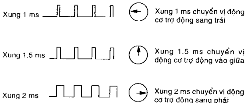
Hình 4.10. Tín hiệu xung của động cơ trở động.
