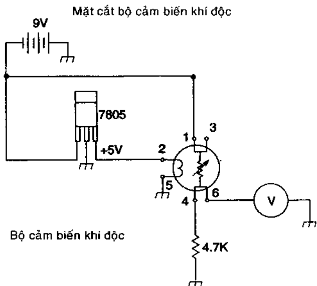
Hình 5.46. Mạch thử nghiệm của bộ cảm biến khí độc.
