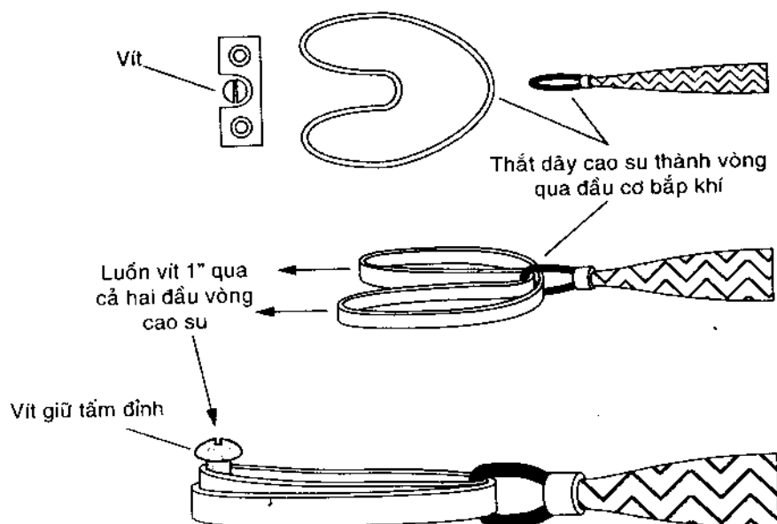
Hình 16.23. Móc dây cao su qua một đầu của cơ bấp không khí và gắn đầu đối diện với ốc vít giữ tấm nhôm.
