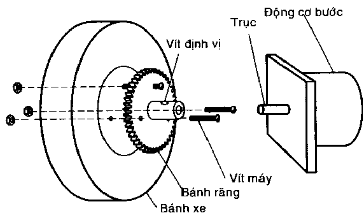
Hình 10.9. Lắp ráp bánh xe với trục động cơ.
