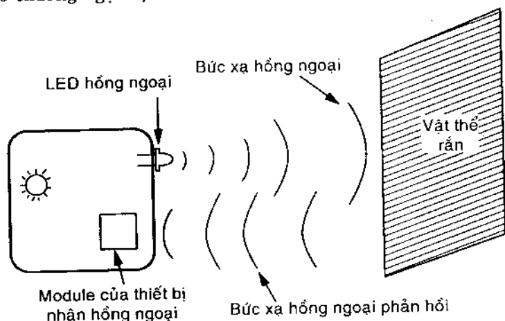
Hình 5.10. Thiết bị dò chương ngại vật bằng hồng ngoại.
