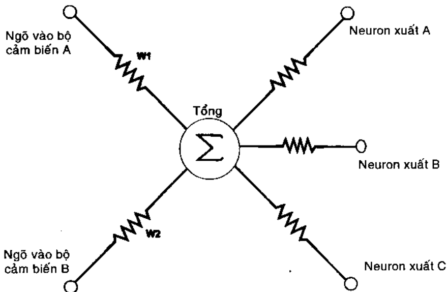
Hình 6.36. Sơ đồ tế bào neuron ba-mức đơn giản.
