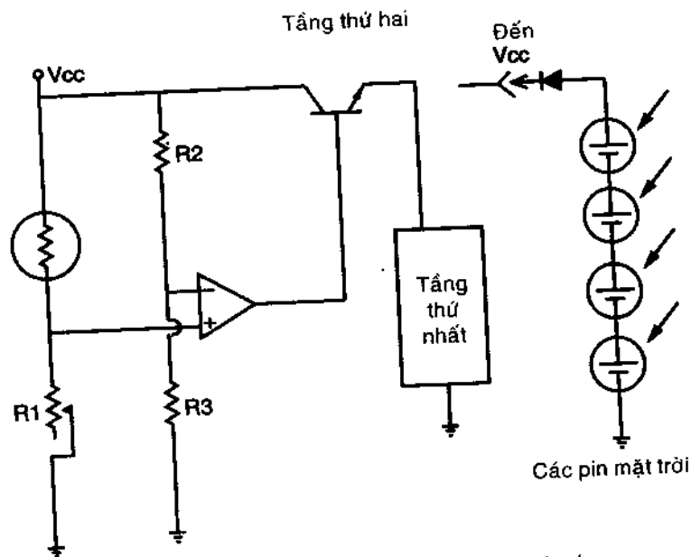
Hình 8.23. Mạch điện bộ so sánh hành vi.
