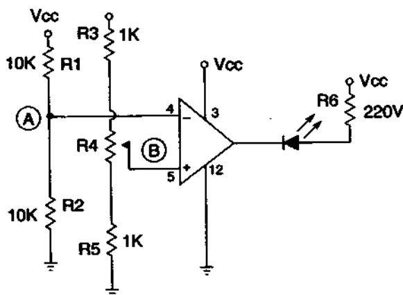
Hình 5.3. Sơ đồ mạch thử nghiệm bộ so sánh op-amp.
