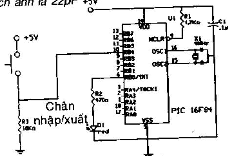
Hình 6.22. Sơ đồ mạch điện đọc - công tắc - cao.
