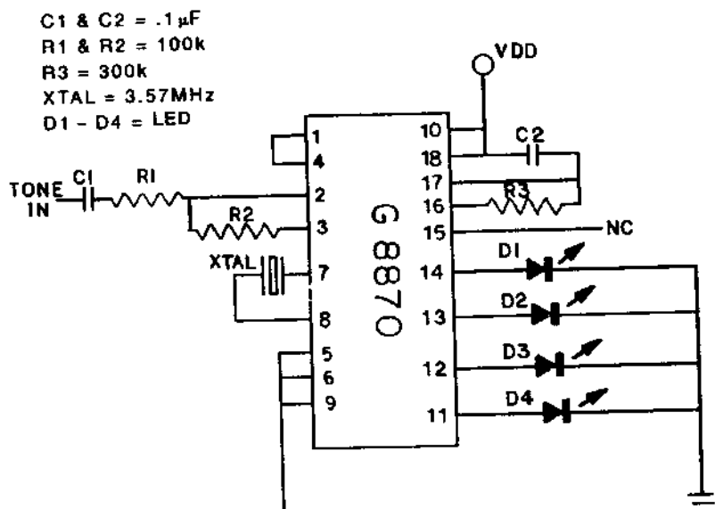
Hình 5.22. Sơ đồ mạch nhận với tín hiệu ra nhị phân 4-bit .
