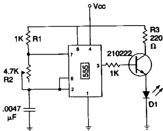
Hình 5.11. Sơ đồ máy phát hồng ngoại.
