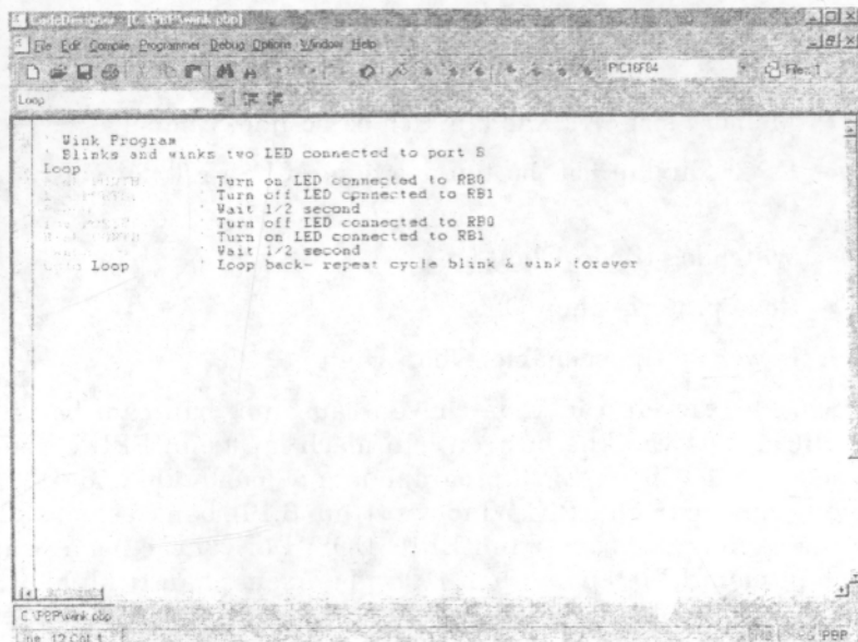
Hình 6.18. Chương trình PICBASIC Pro được viết trong CodeDesigner.
