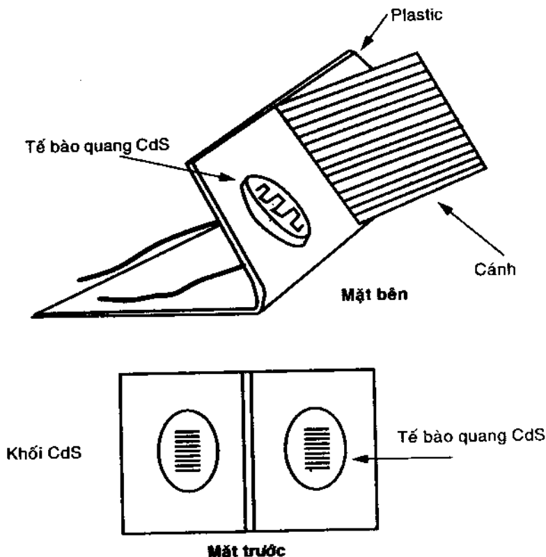
Hình 8.14. Hình vẽ tấm cảm biến với kích thước thật.
