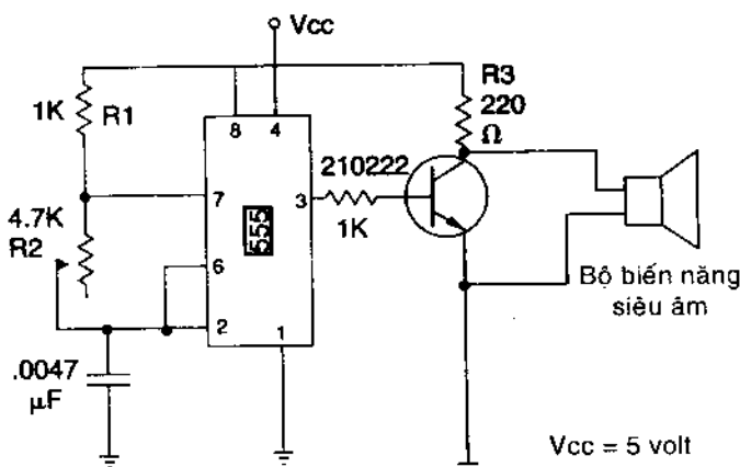
Hình 5.36. Mạch máy phát siêu âm.
