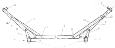
Khung võng xếp của tác giả Lâm Tấn Lợi được Cục SHTT cấp Bằng độc quyền GPHI số 314
