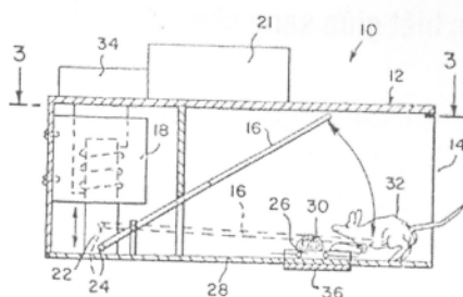
Một kiểu bẫy chuột được Cục Patent và Nhân hàng Hoa kỳ cấp Bằng độc quyền sáng chế số 5.107.619 (28.4.1992).
