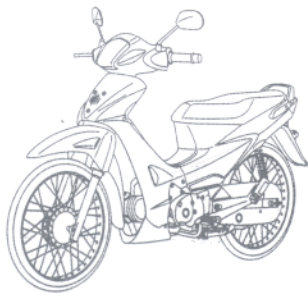
Kiểu dáng xe máy của Honda Việt nam được cấp Bảng độc quyền kiểu dáng công nghiệp số 4036
